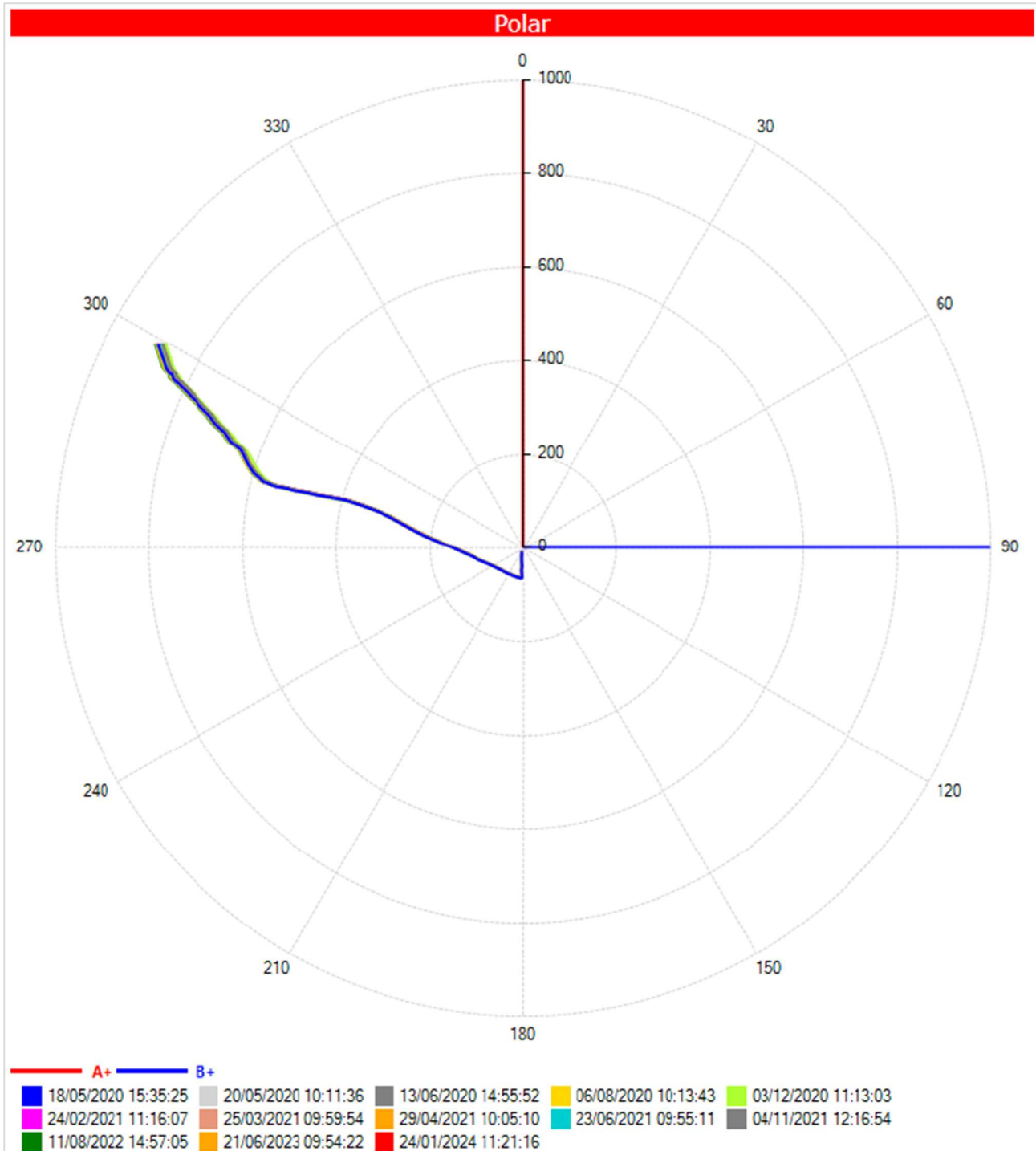
Figura 5.102 – Deslocamentos em relação a coordenadas polares acumulados do INC-01 (ref. 24/01/2024).
