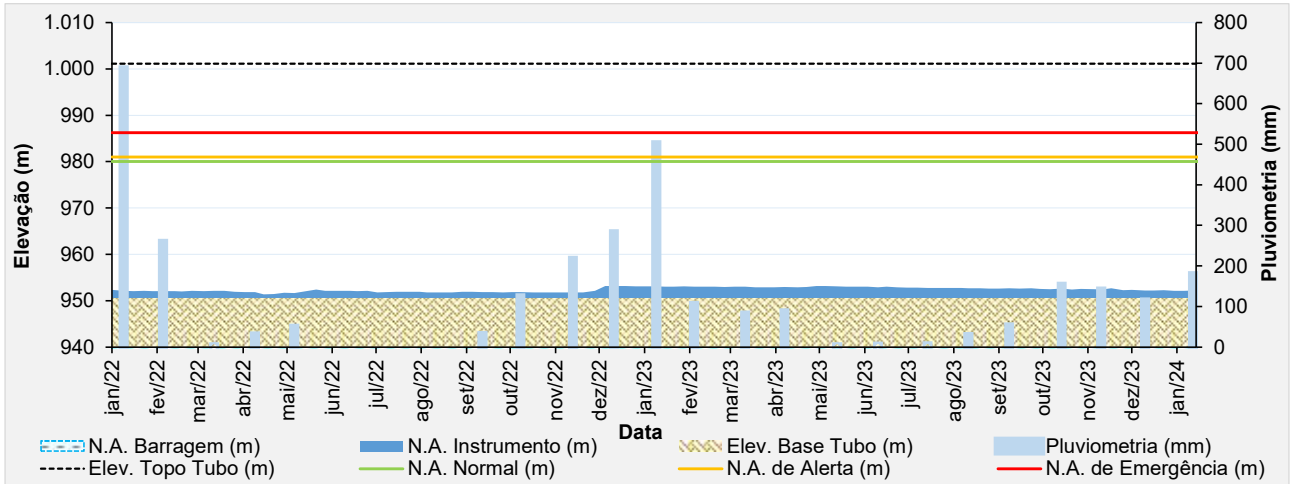
Figura 5.51 – Desempenho do piezômetro de tubo aberto - PZ-21.
