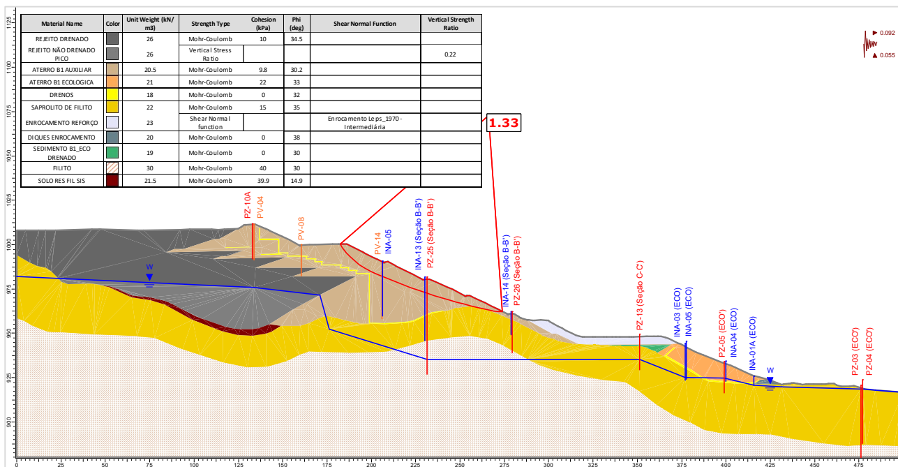
Figura 5.111 – Seção A-A' – Análise Não Drenada – Superfície de ruptura plano-circular otimizada – Freática 29/01/2024 – Razão de resistência não drenada de pico + sismo ↑ (critério CDA).
