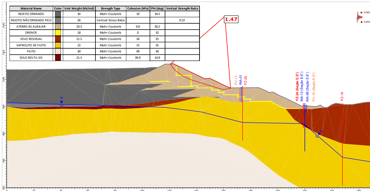
Figura 5.146 – Seção F-F' – Análise Não Drenada – Superfície de ruptura plano-circular otimizada – Freática 29/01/2024 – Razão de resistência não drenada de pico + sismo ↑ (critério CDA).
