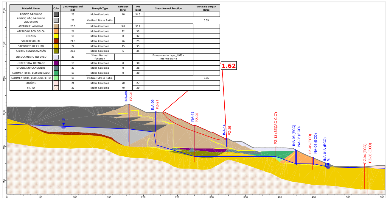
Figura 5.117 – Seção B-B' – Análise Não Drenada – Superfície de ruptura plano-circular otimizada – Freática 29/01/2024 – Razão de resistência não drenada liquefeita.
