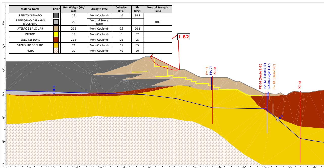
Figura 5.145 – Seção F-F' – Análise Não Drenada – Superfície de ruptura plano-circular otimizada – Freática 29/01/2024 – Razão de resistência não drenada liquefeita.
