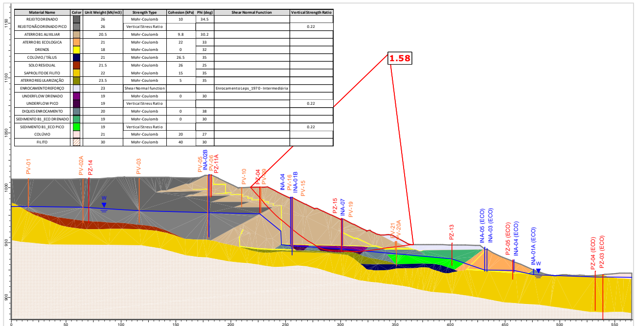
Figura 5.123 – Seção C-C' – Análise Não Drenada – Superfície de ruptura plano-circular otimizada – Freática 29/01/2024 – Razão de resistência não drenada de pico.
