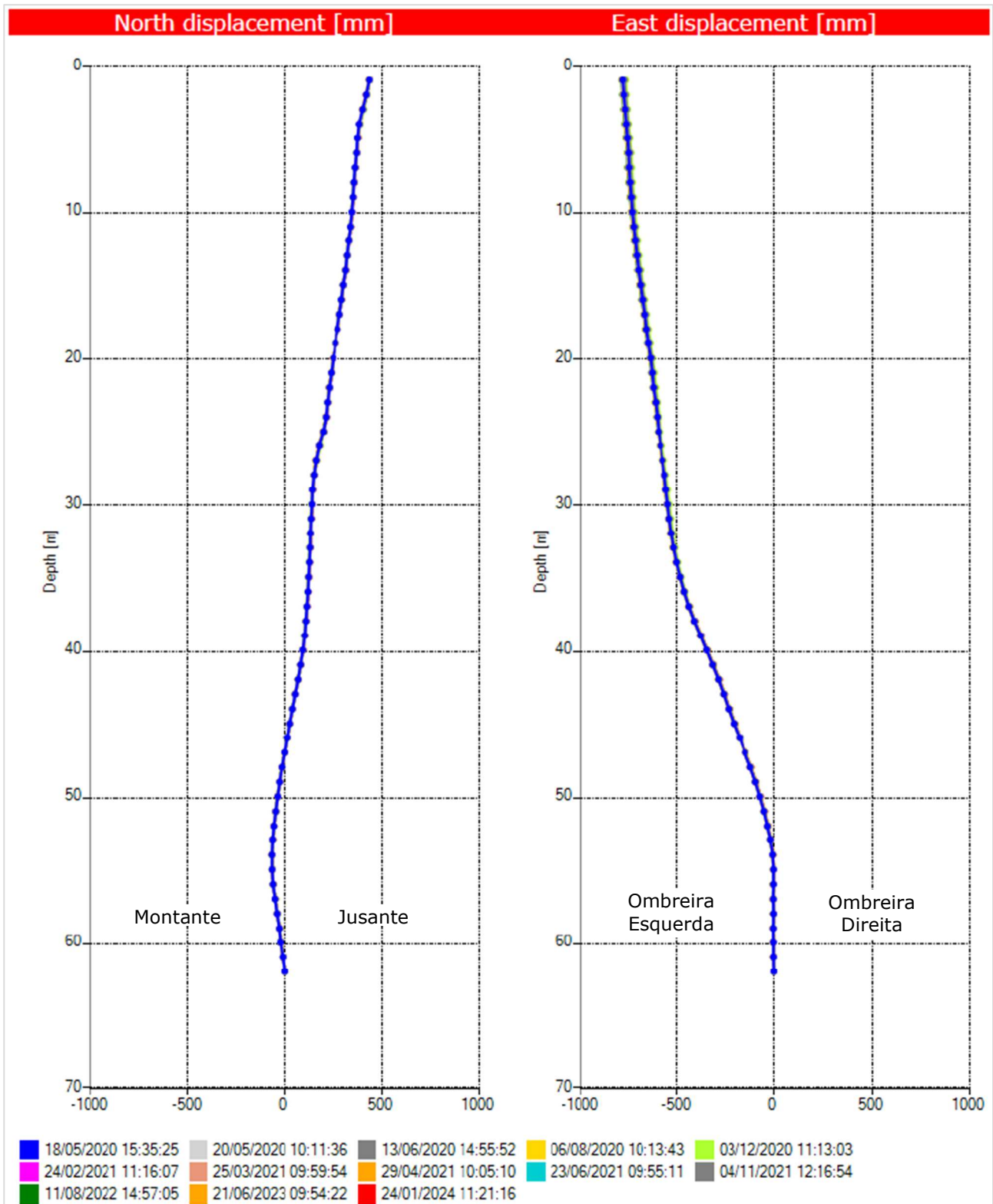
Figura 5.101 – Deslocamentos horizontais acumulados do INC-01 (ref. 24/01/2024).
