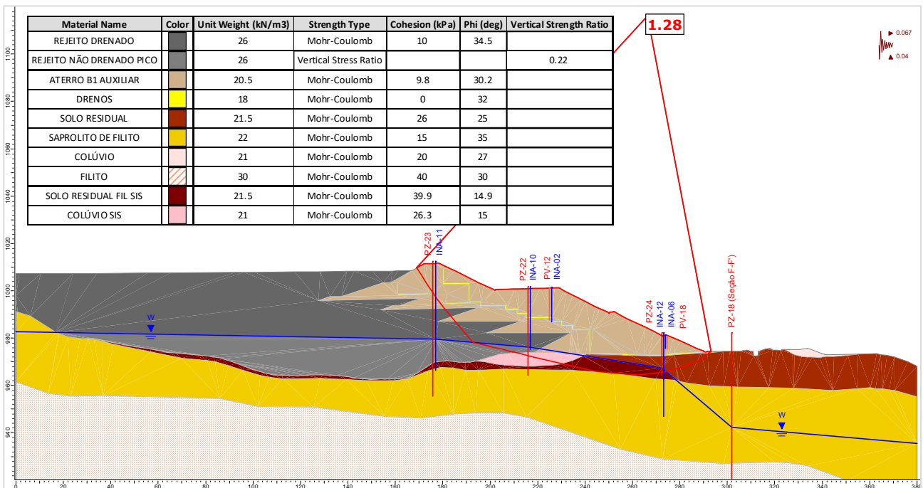
Figura 5.141 – Seção E-E' – Análise Não Drenada – Superfície de ruptura plano-circular otimizada – Freática 29/01/2024 – Razão de resistência não drenada de pico + sismo ↑ (critério vida útil).
