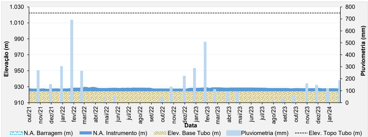
Figura 5.46 – Desempenho do piezômetro de tubo aberto - PZ-16.
