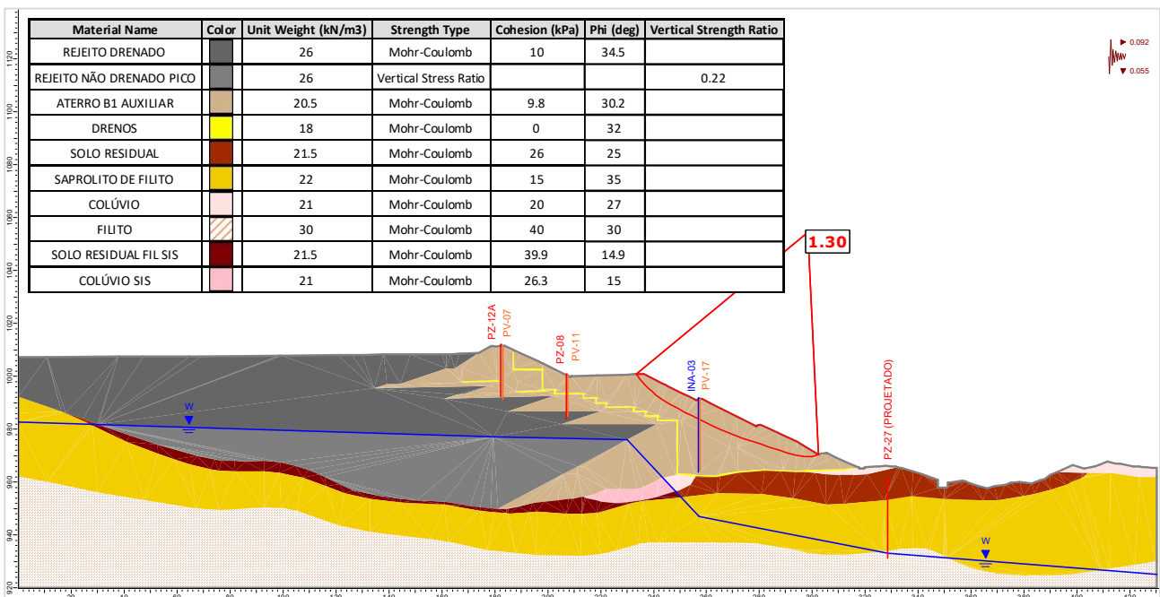
Figura 5.133 – Seção D-D' – Análise Não Drenada – Superfície de ruptura plano-circular otimizada – Freática 29/01/2024 – Razão de resistência não drenada de pico + sismo ↓ (critério CDA).
