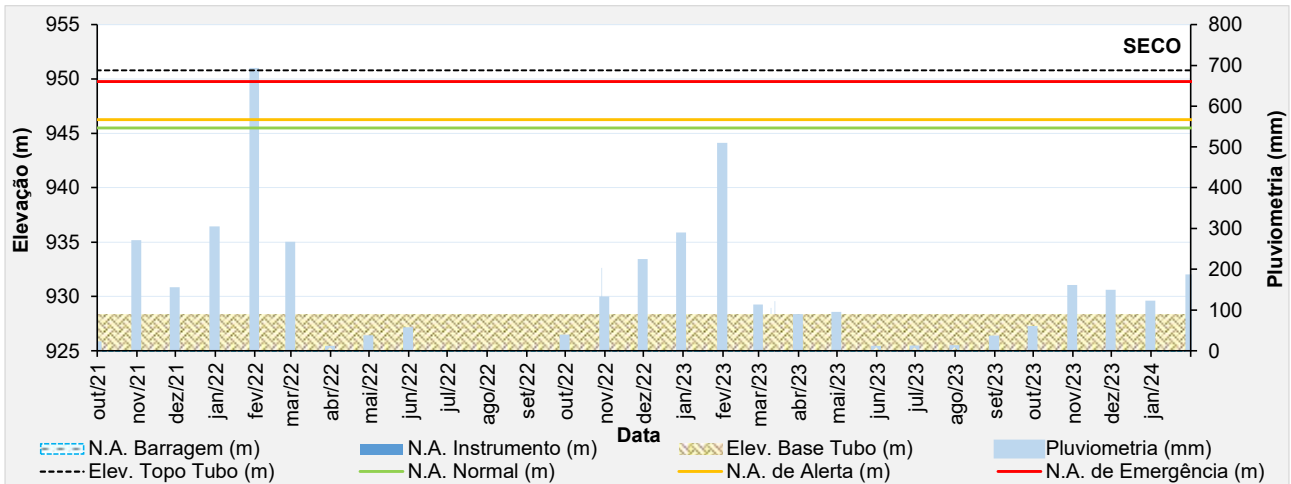
Figura 5.36 – Desempenho do piezômetro elétrico - PV-20A.
