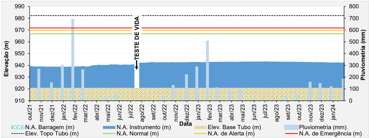
Figura 5.48 – Desempenho do piezômetro de tubo aberto - PZ-18.
