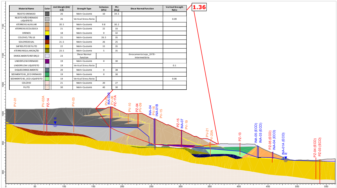
Figura 5.124 – Seção C-C' – Análise Não Drenada – Superfície de ruptura plano-circular otimizada – Freática 29/01/2024 – Razão de resistência não drenada liquefeita.
