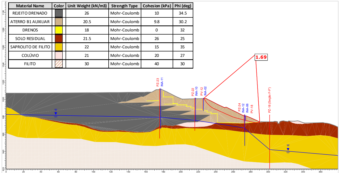
Figura 5.136 – Seção E-E' – Análise Drenada – Superfície de ruptura plano-circular otimizada – Freática 29/01/2024.
