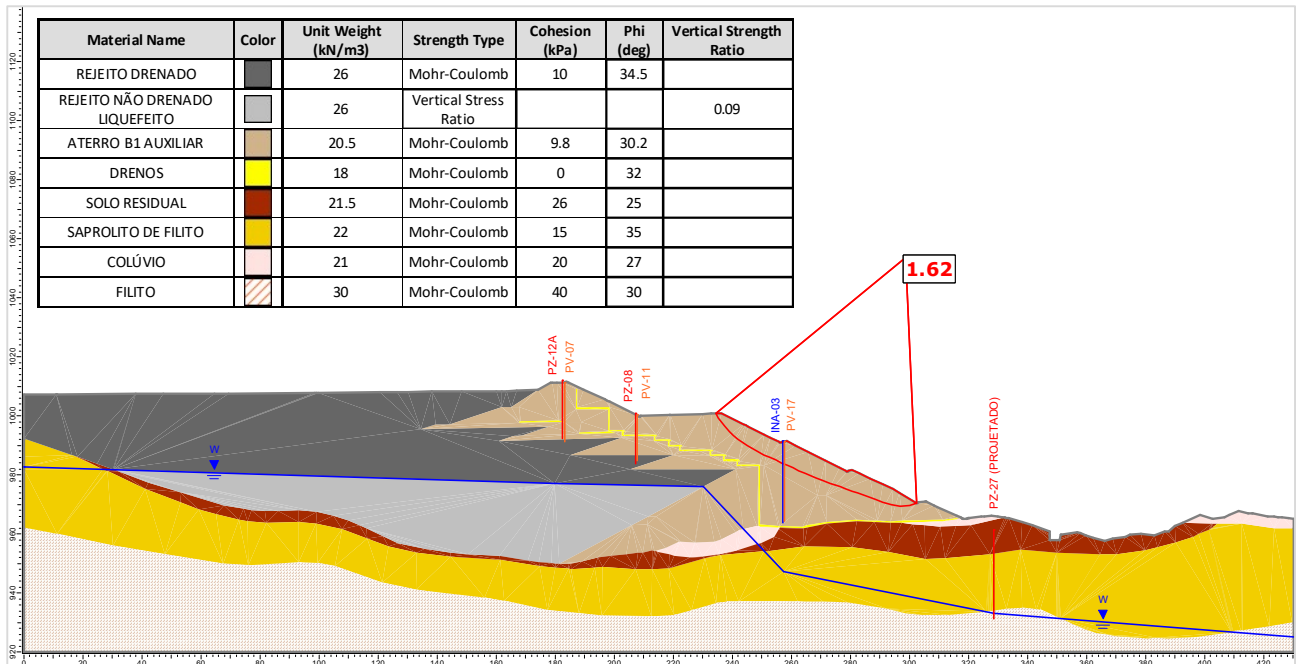
Figura 5.131 – Seção D-D' – Análise Não Drenada – Superfície de ruptura plano-circular otimizada – Freática 29/01/2024 – Razão de resistência não drenada liquefeita.
