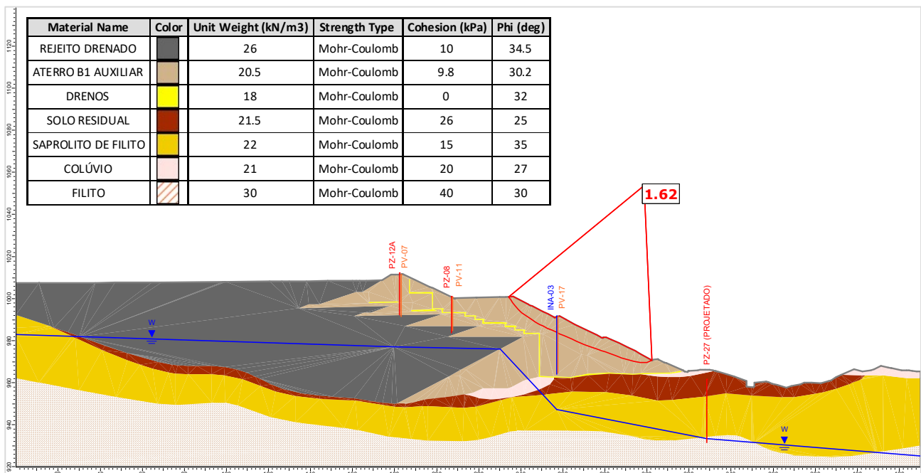
Figura 5.129 – Seção D-D' – Análise Drenada – Superfície de ruptura plano-circular otimizada – Freática 29/01/2024.
