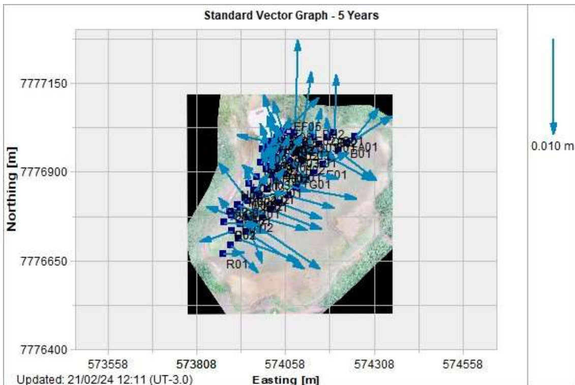
Figura 5.84 – Registros vetores deslocamento dos prismas.
