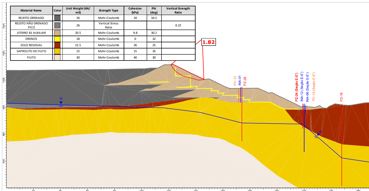
Figura 5.144 – Seção F-F' – Análise Não Drenada – Superfície de ruptura plano-circular otimizada – Freática 29/01/2024 – Razão de resistência não drenada de pico.
