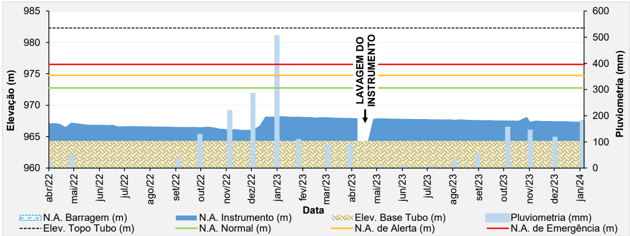
Figura 5.54 – Desempenho do piezômetro de tubo aberto - PZ-24.
