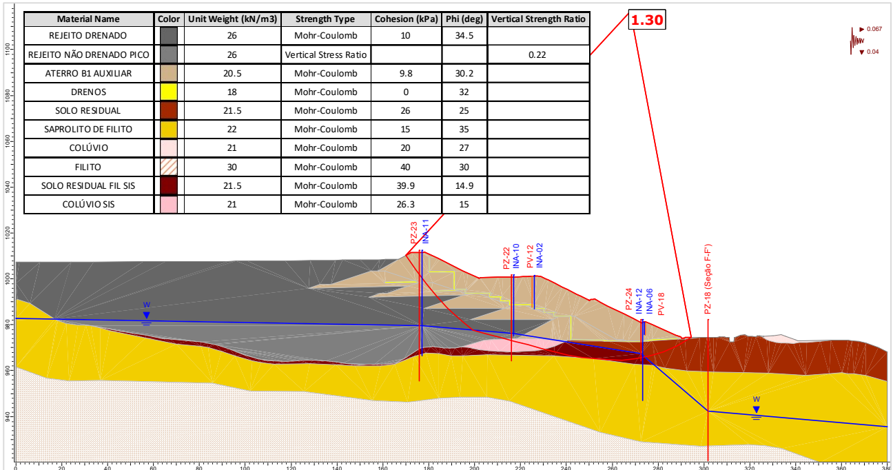
Figura 5.142 – Seção E-E' – Análise Não Drenada – Superfície de ruptura plano-circular otimizada – Freática 29/01/2024 – Razão de resistência não drenada de pico + sismo ↓ (critério vida útil).
