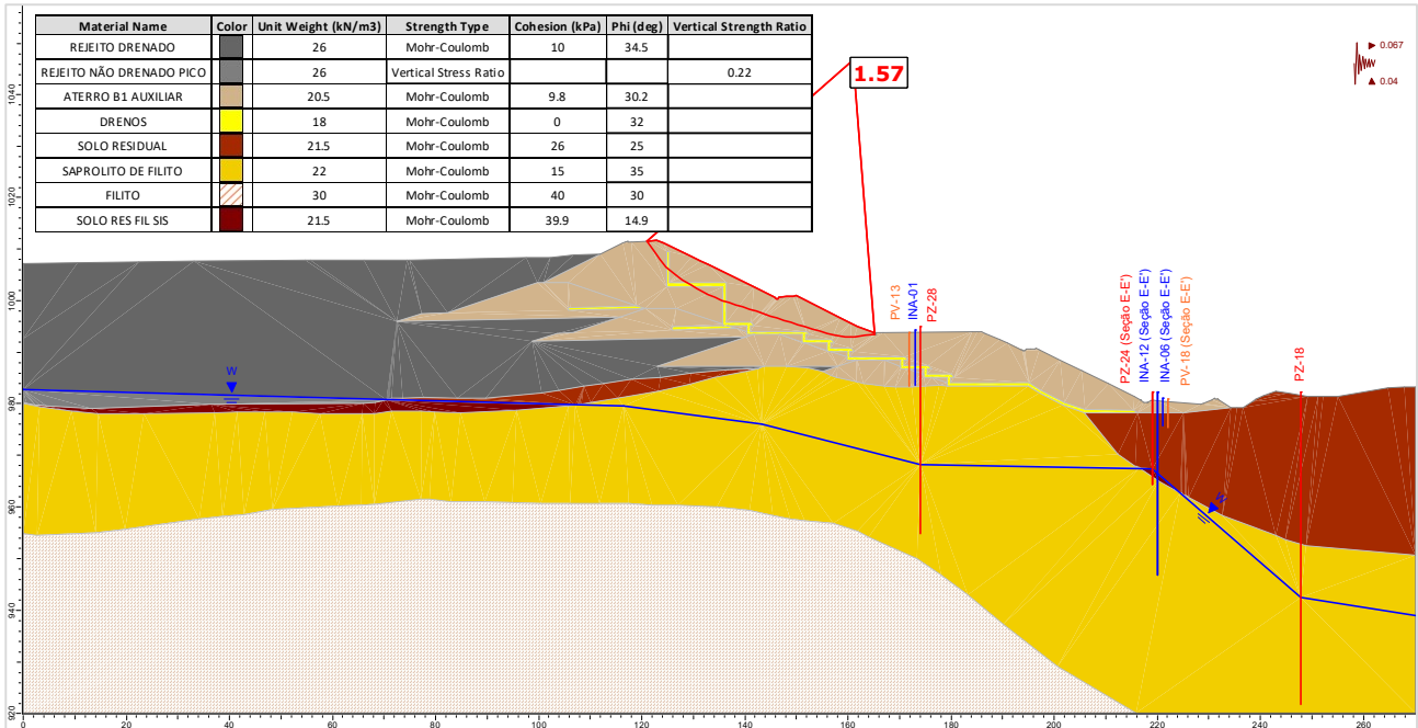
Figura 5.148 – Seção F-F' – Análise Não Drenada – Superfície de ruptura plano-circular otimizada – Freática 29/01/2024 – Razão de resistência não drenada de pico + sismo ↑ (critério vida útil).
