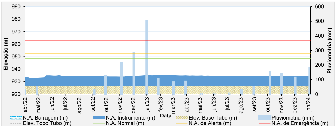
Figura 5.55 – Desempenho do piezômetro de tubo aberto - PZ-25.
