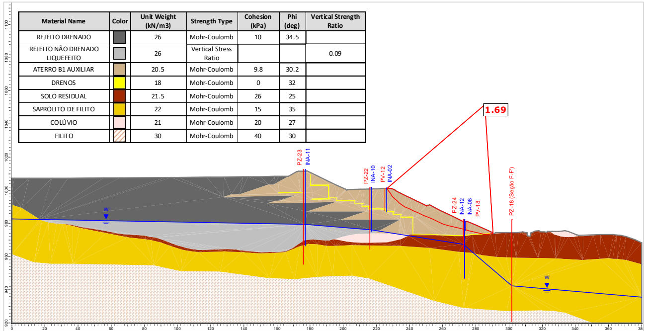
Figura 5.138 – Seção E-E' – Análise Não Drenada – Superfície de ruptura plano-circular otimizada – Freática 29/01/2024 – Razão de resistência não drenada liquefeita.
