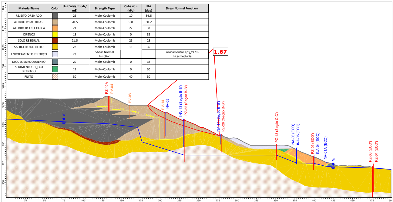
Figura 5.108 – Seção A-A' – Análise Drenada – Superfície de ruptura plano-circular otimizada – Freática 29/01/2024.
