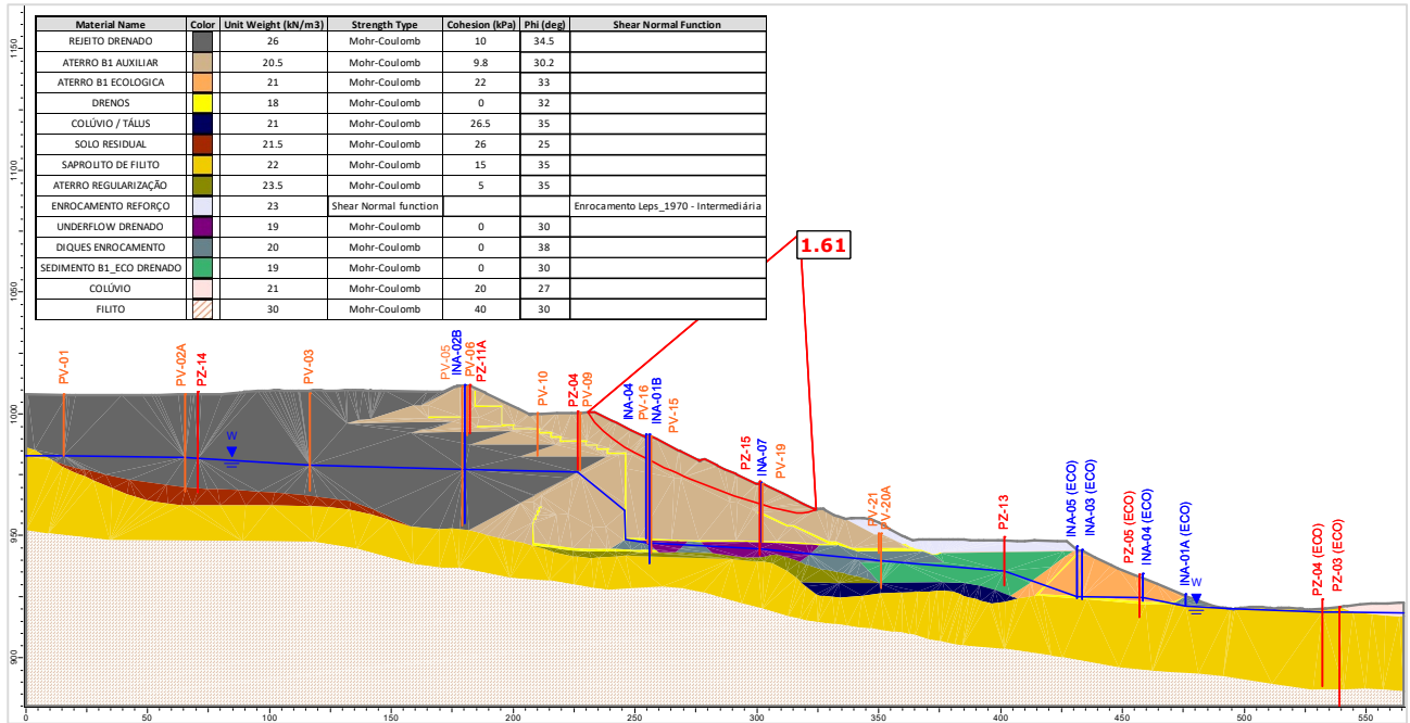
Figura 5.122 – Seção C-C' – Análise Drenada – Superfície de ruptura plano-circular otimizada – Freática 29/01/2024.
