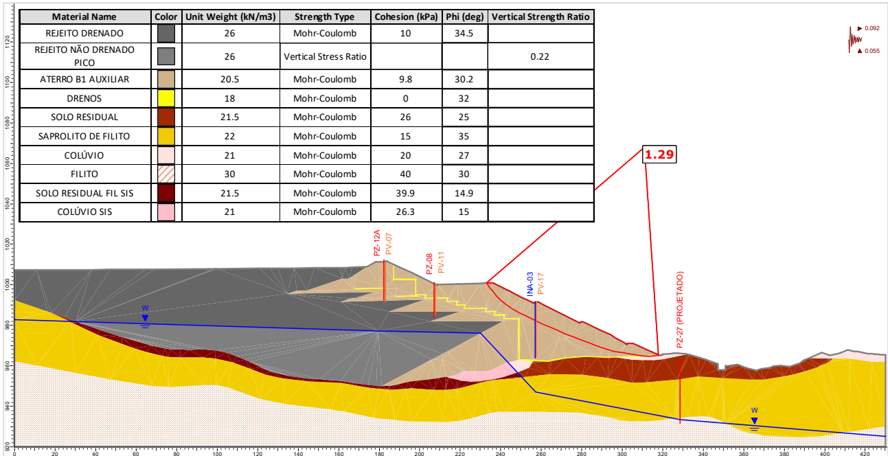
Figura 5.132 – Seção D-D' – Análise Não Drenada – Superfície de ruptura plano-circular otimizada – Freática 29/01/2024 – Razão de resistência não drenada de pico + sismo ↑ (critério CDA).
