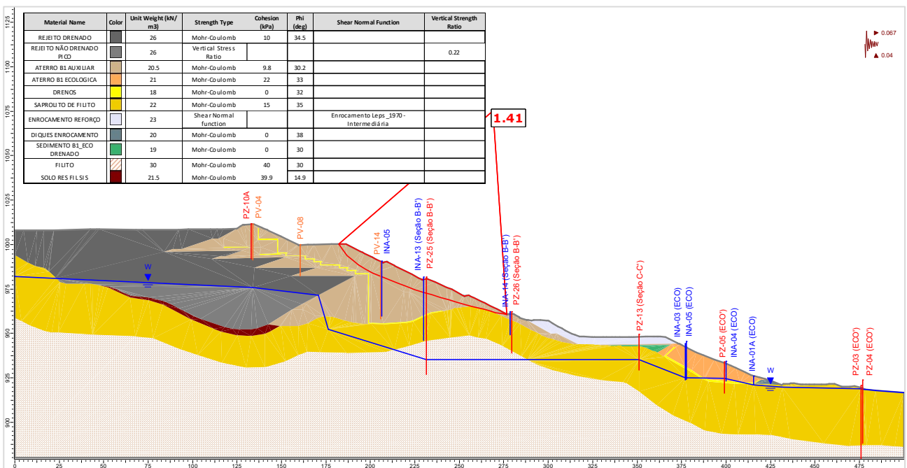
Figura 5.113 – Seção A-A' – Análise Não Drenada – Superfície de ruptura plano-circular otimizada – Freática 29/01/2024 – Razão de resistência não drenada de pico + sismo ↑ (critério vida útil).
