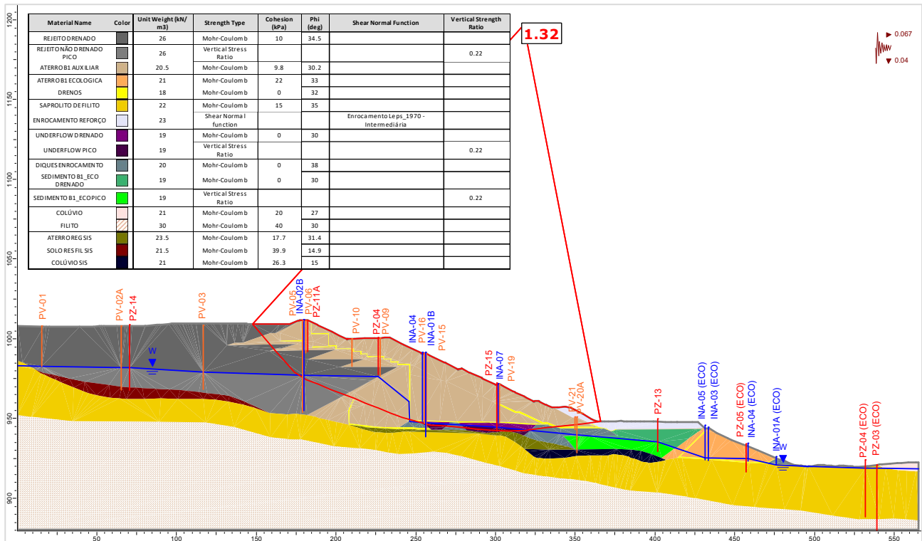
Figura 5.128 – Seção C-C' – Análise Não Drenada – Superfície de ruptura plano-circular otimizada – Freática 29/01/2024 – Razão de resistência não drenada de pico + sismo ↓ (critério vida útil).
