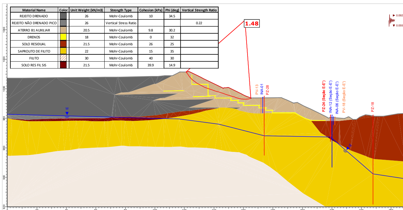
Figura 5.147 – Seção F-F' – Análise Não Drenada – Superfície de ruptura plano-circular otimizada – Freática 29/01/2024 – Razão de resistência não drenada de pico + sismo ↓ (critério CDA).
