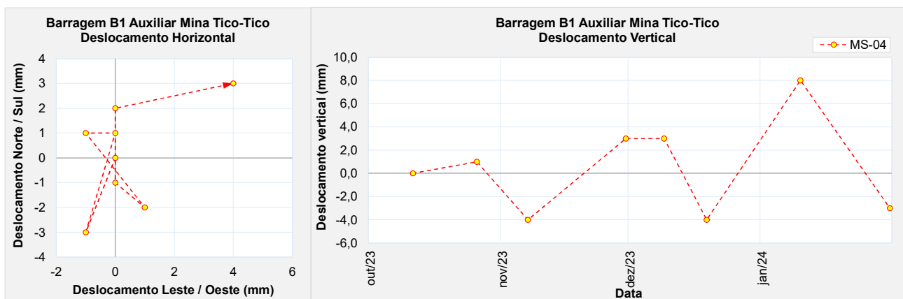
Figura 5.96 – Marco de controle de deformação – MS-04.
