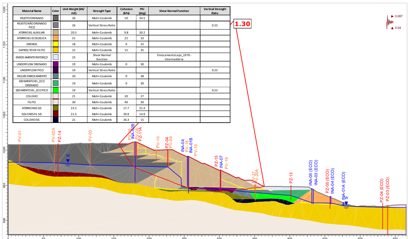
Figura 5.127 – Seção C-C' – Análise Não Drenada – Superfície de ruptura plano-circular otimizada – Freática 29/01/2024 – Razão de resistência não drenada de pico + sismo ↑ (critério vida útil).
