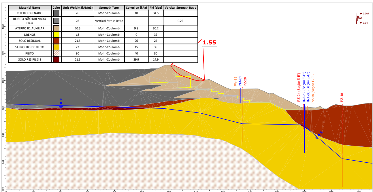
Figura 5.149 – Seção F-F' – Análise Não Drenada – Superfície de ruptura plano-circular otimizada – Freática 29/01/2024 – Razão de resistência não drenada de pico + sismo ↓ (critério vida útil).
