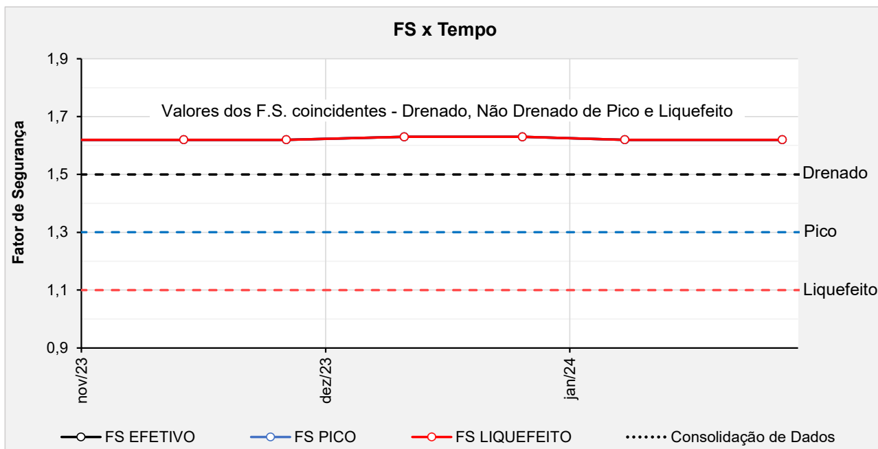
Figura 5.153 – Seção D-D' - Histórico dos F.S. obtidos nas análises de estabilidade no período avaliado.
