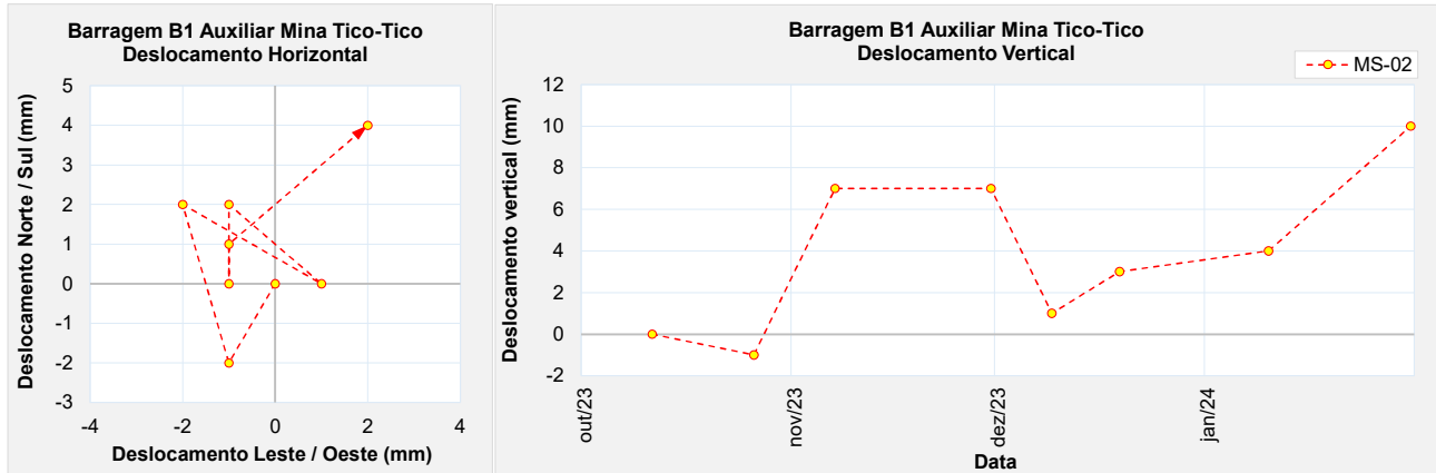
Figura 5.94 – Marco de controle de deformação – MS-02.
