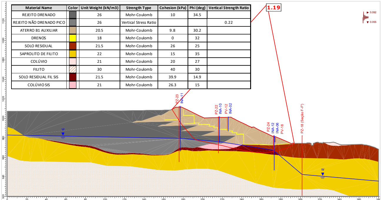
Figura 5.140 – Seção E-E' – Análise Não Drenada – Superfície de ruptura plano-circular otimizada – Freática 29/01/2024 – Razão de resistência não drenada de pico + sismo ↓ (critério CDA).
