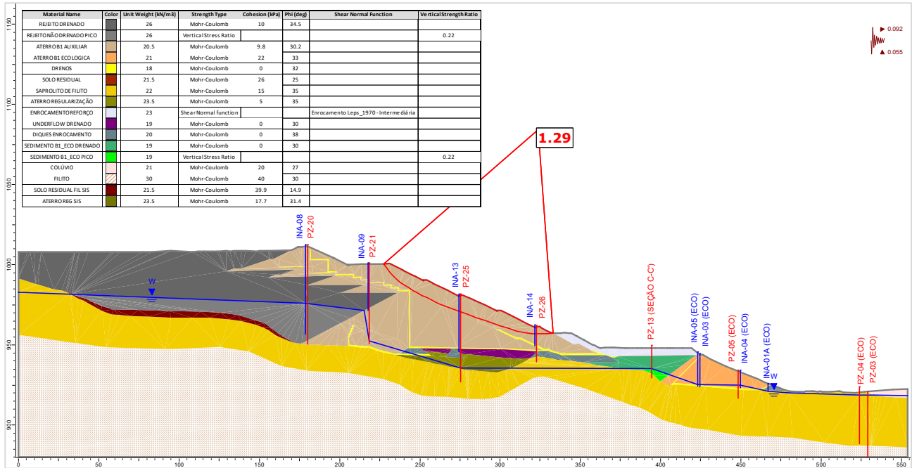
Figura 5.118 – Seção B-B' – Análise Não Drenada – Superfície de ruptura plano-circular otimizada – Freática 29/01/2024 – Razão de resistência não drenada de pico + sismo ↑ (critério CDA).
