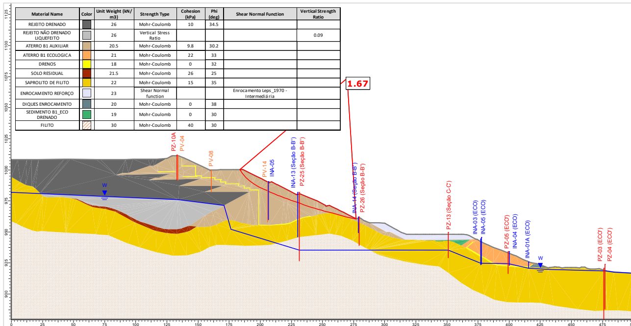
Figura 5.110 – Seção A-A' – Análise Não Drenada – Superfície de ruptura plano-circular otimizada – Freática 29/01/2024 – Razão de resistência não drenada liquefeita.
