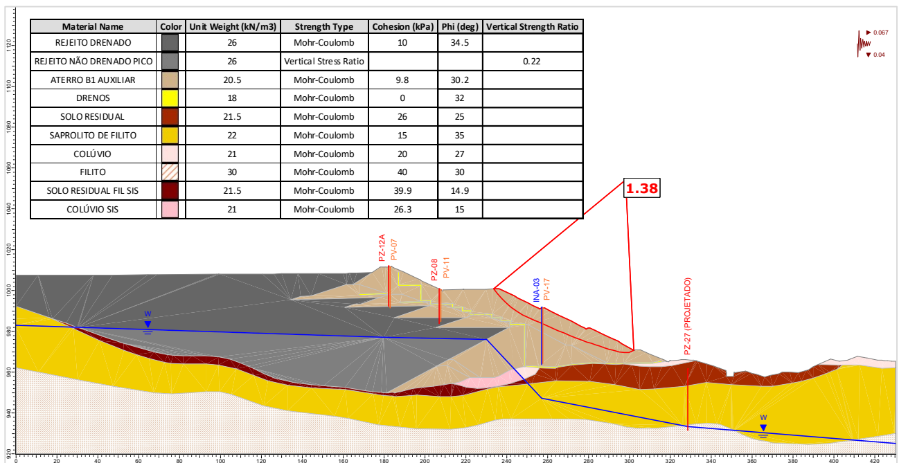
Figura 5.135 – Seção D-D' – Análise Não Drenada – Superfície de ruptura plano-circular otimizada – Freática 29/01/2024 – Razão de resistência não drenada de pico + sismo ↓ (critério vida útil).
