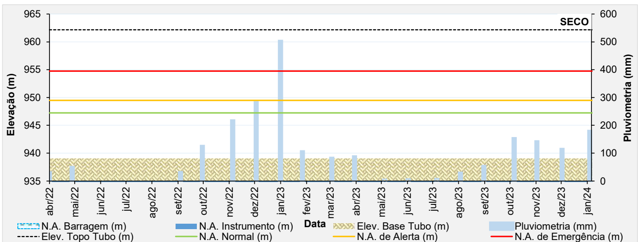
Figura 5.56 – Desempenho do piezômetro de tubo aberto - PZ-26.
