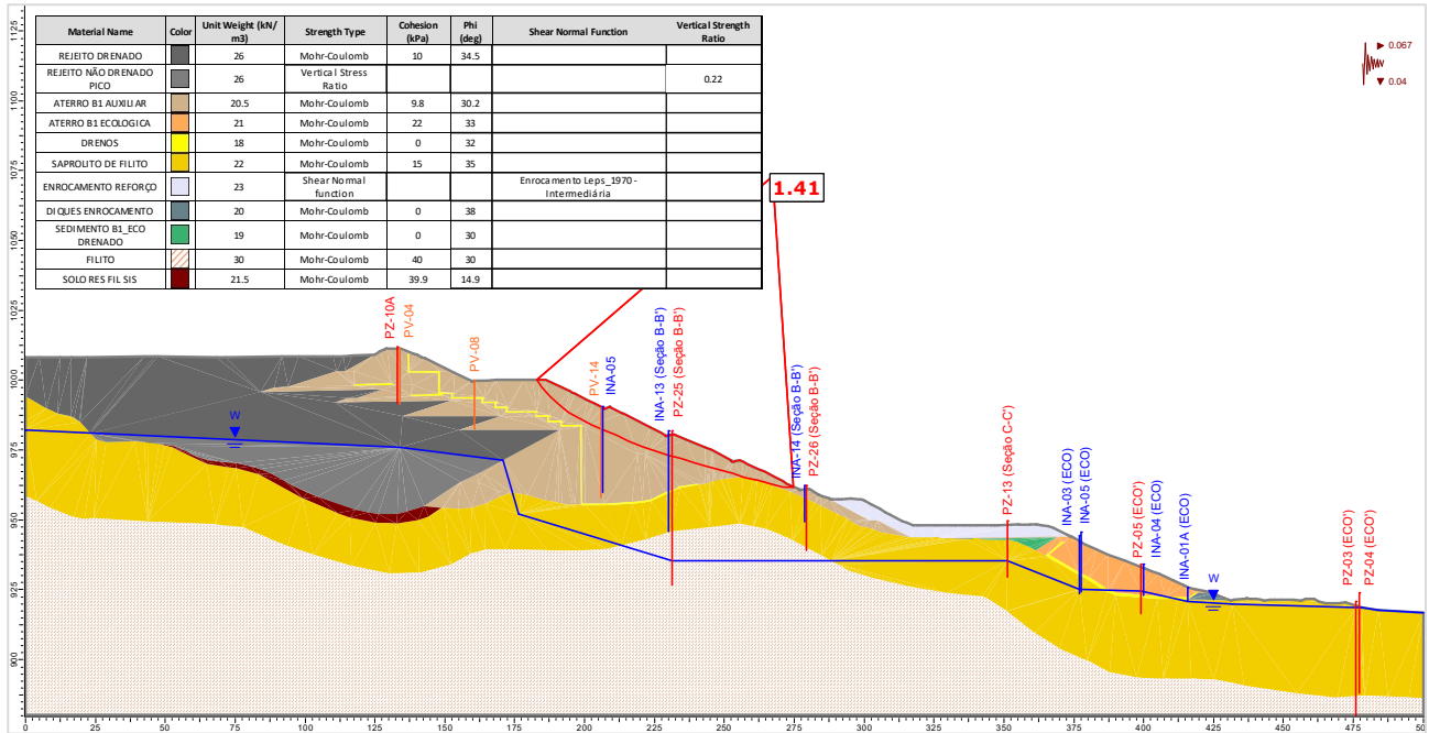
Figura 5.114 – Seção A-A’ – Análise Não Drenada – Superfície de ruptura plano-circular otimizada – Freática 29/01/2024 – Razão de resistência não drenada de pico + sismo ↓ (critério vida útil).
