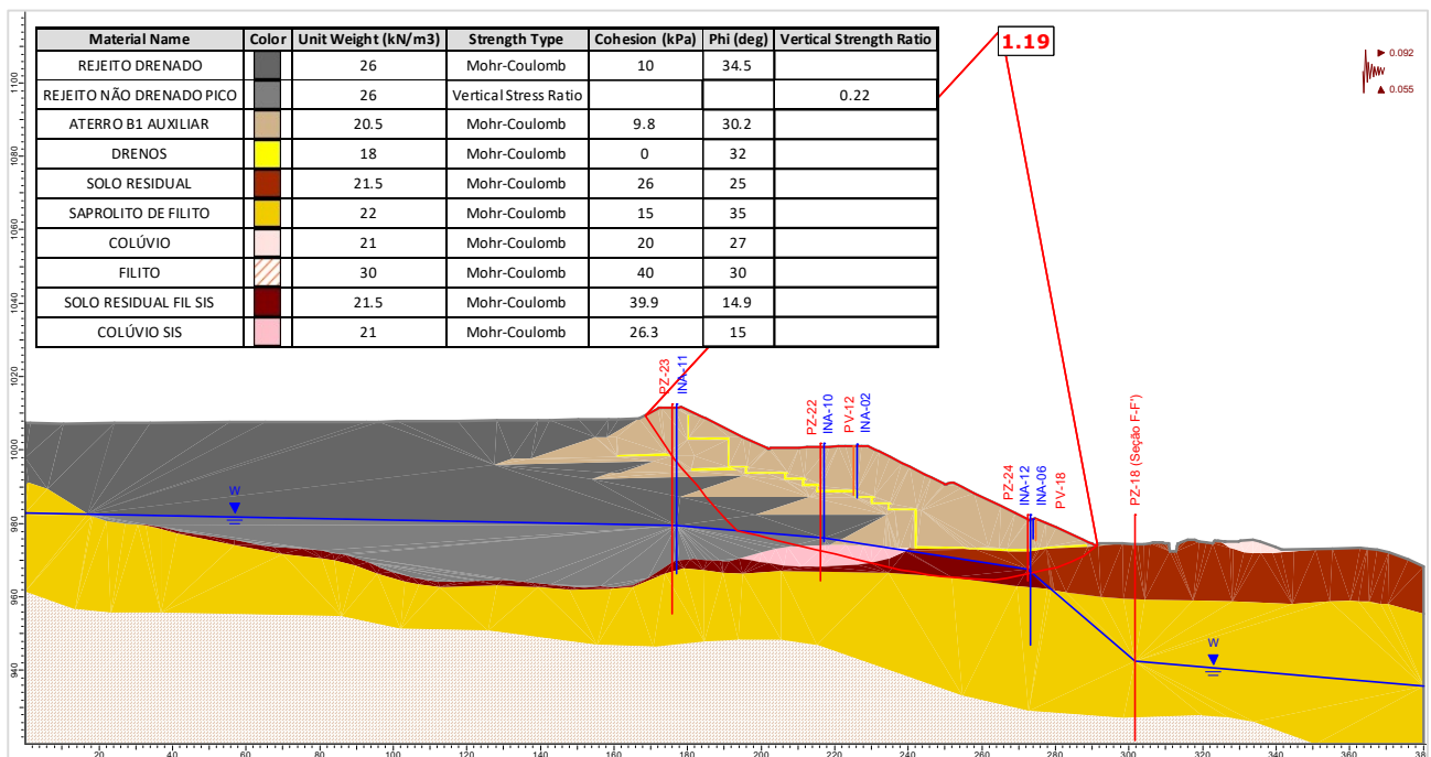
Figura 5.139 – Seção E-E' – Análise Não Drenada – Superfície de ruptura plano-circular otimizada – Freática 29/01/2024 – Razão de resistência não drenada de pico + sismo ↑ (critério CDA).
