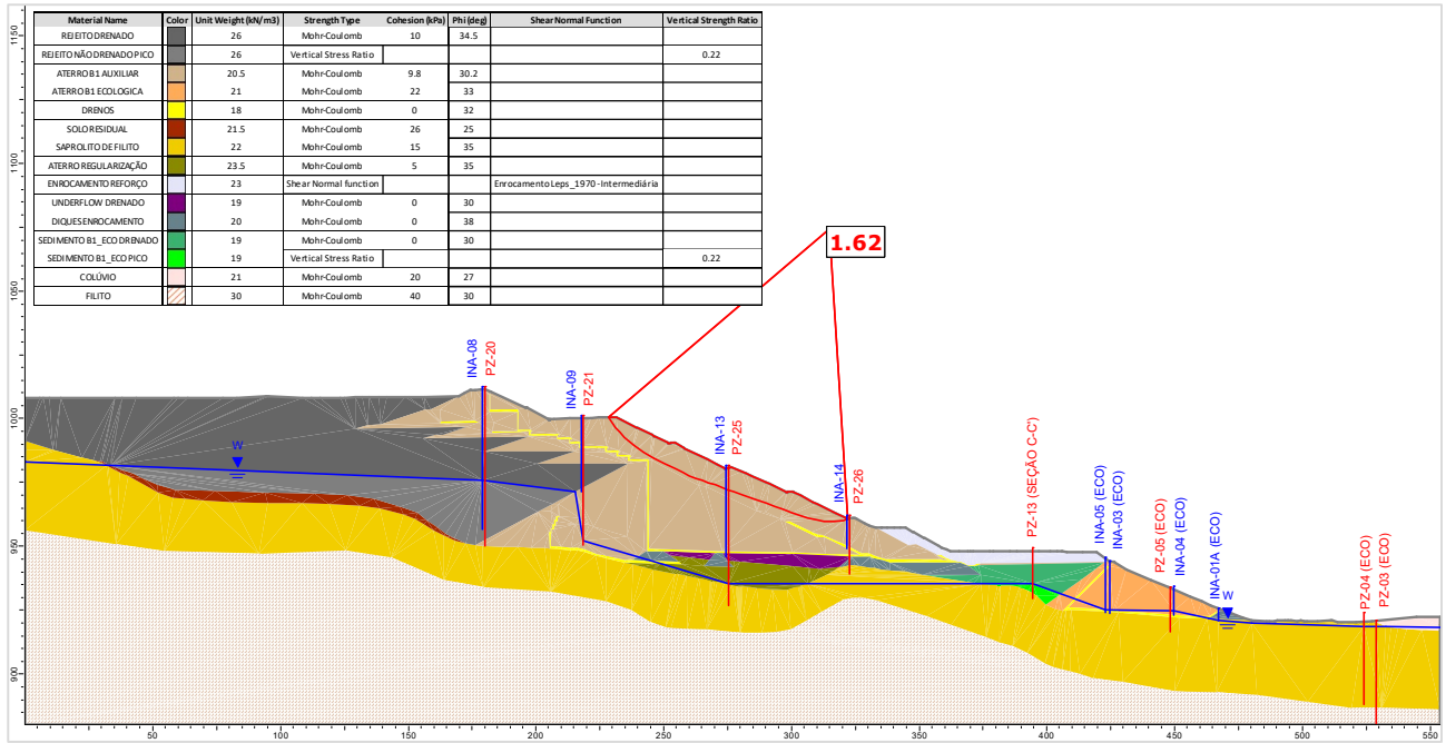
Figura 5.116 – Seção B-B' – Análise Não Drenada – Superfície de ruptura plano-circular otimizada – Freática 29/01/2024 – Razão de resistência não drenada de pico.
