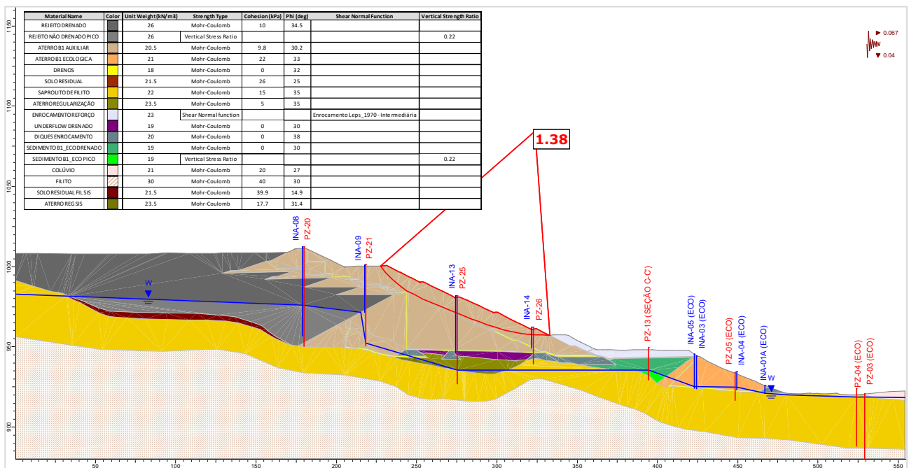
Figura 5.121 – Seção B-B' – Análise Não Drenada – Superfície de ruptura plano-circular otimizada – Freática 29/01/2024 – Razão de resistência não drenada de pico + sismo ↓ (critério vida útil).
