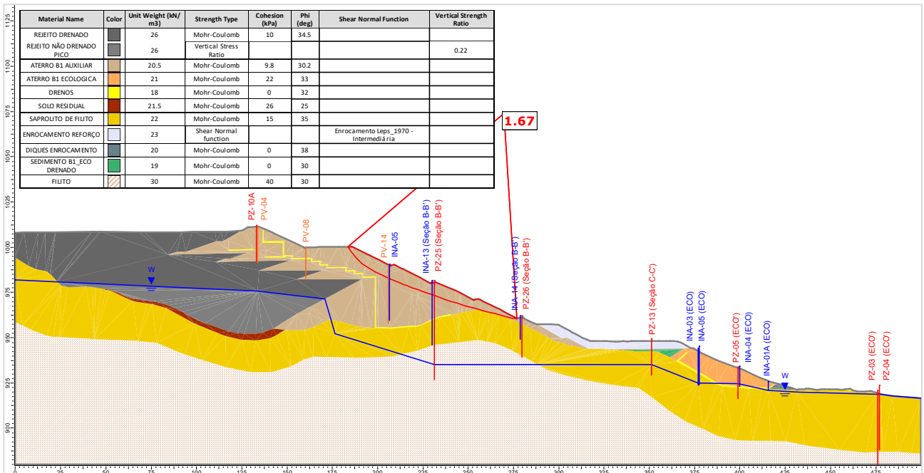
Figura 5.109 – Seção A-A' – Análise Não Drenada – Superfície de ruptura plano-circular otimizada – Freática 29/01/2024 – Razão de resistência não drenada de pico.
