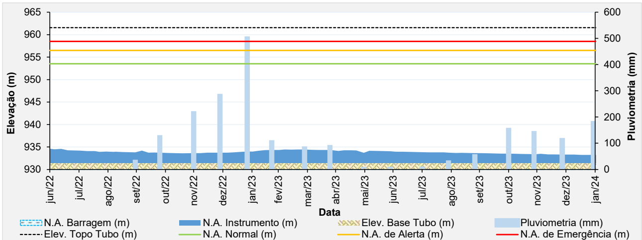
Figura 5.57 – Desempenho do piezômetro de tubo aberto - PZ-27.
