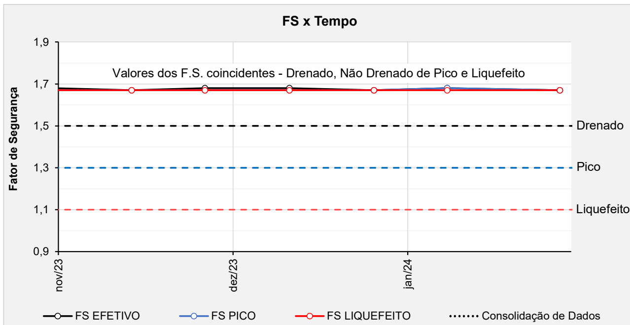
Figura 5.150 – Seção A-A' - Histórico dos F.S. obtidos nas análises de estabilidade no período avaliado.
