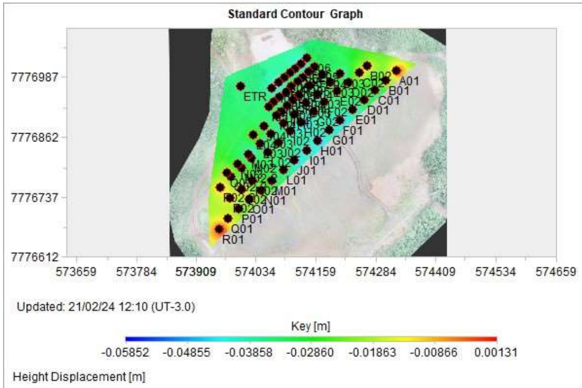
Figura 5.83 – Registros deslocamentos verticais dos prismas.
