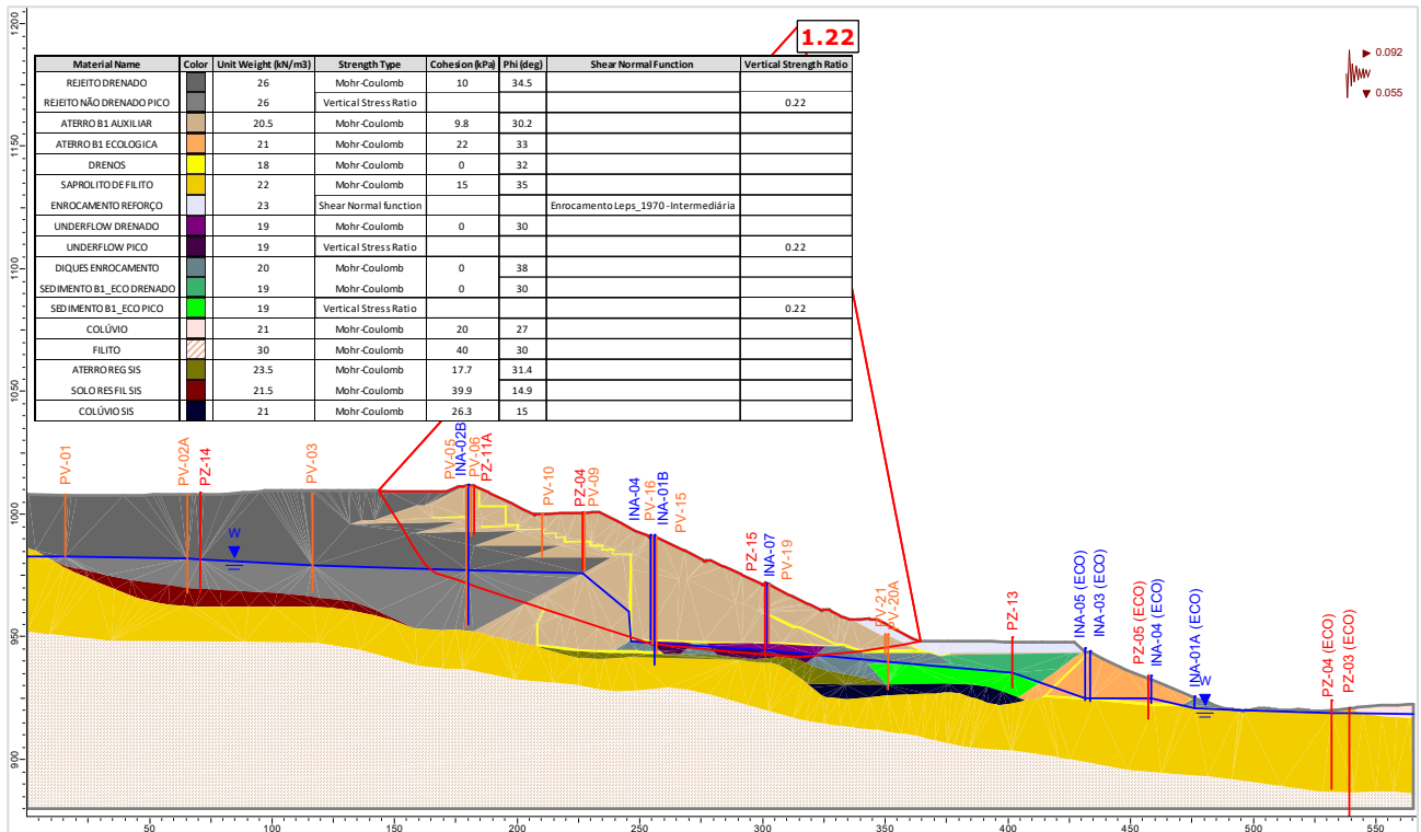
Figura 5.126 – Seção C-C' – Análise Não Drenada – Superfície de ruptura plano-circular otimizada – Freática 29/01/2024 – Razão de resistência não drenada de pico + sismo ↓ (critério CDA).
