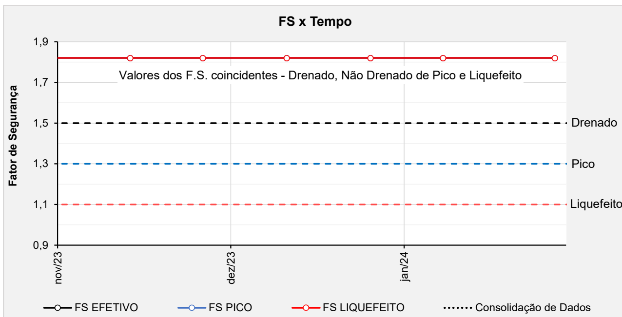
Figura 5.155 – Seção F-F' - Histórico dos F.S. obtidos nas análises de estabilidade no período avaliado.
