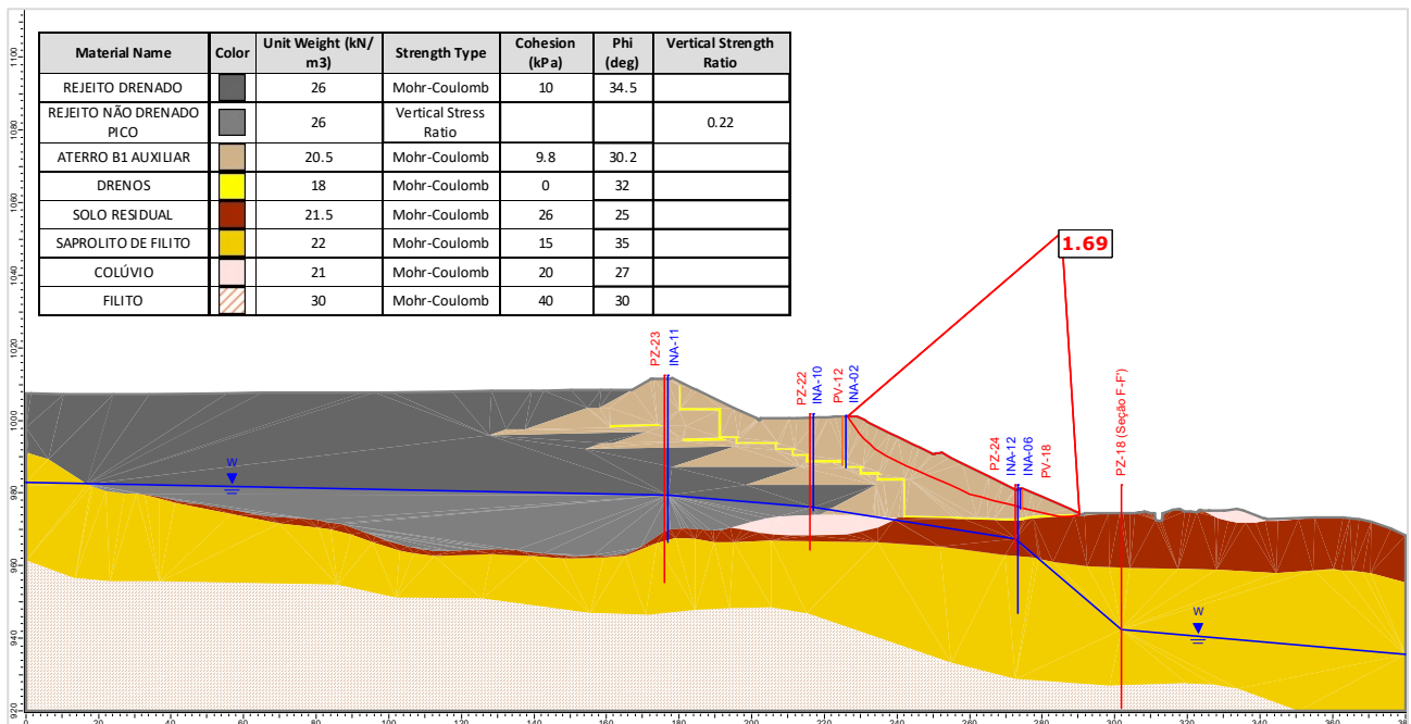
Figura 5.137 – Seção E-E' – Análise Não Drenada – Superfície de ruptura plano-circular otimizada – Freática 29/01/2024 – Razão de resistência não drenada de pico.
