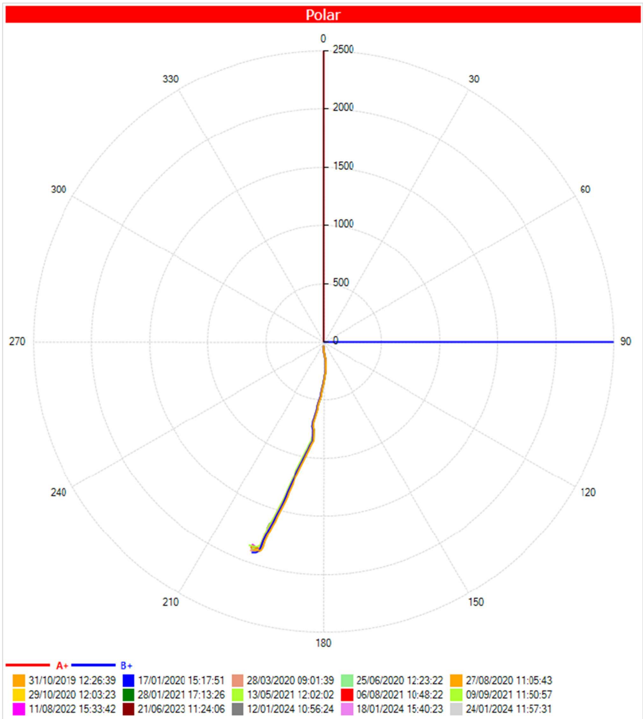
Figura 5.104 – Deslocamentos em relação a coordenadas polares acumulados do INC-02 (ref. 24/01/2024).
