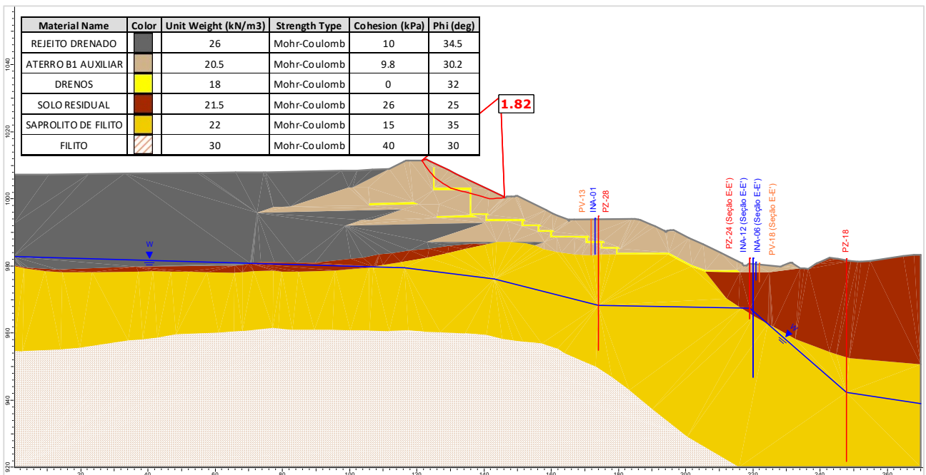
Figura 5.143 – Seção F-F' – Análise Drenada – Superfície de ruptura plano-circular otimizada – Freática 29/01/2024.
