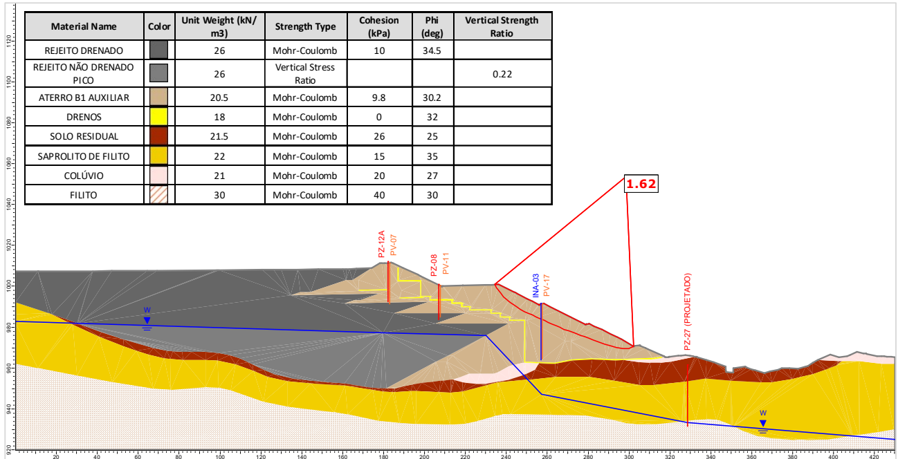
Figura 5.130 – Seção D-D' – Análise Não Drenada – Superfície de ruptura plano-circular otimizada – Freática 29/01/2024 – Razão de resistência não drenada de pico.
