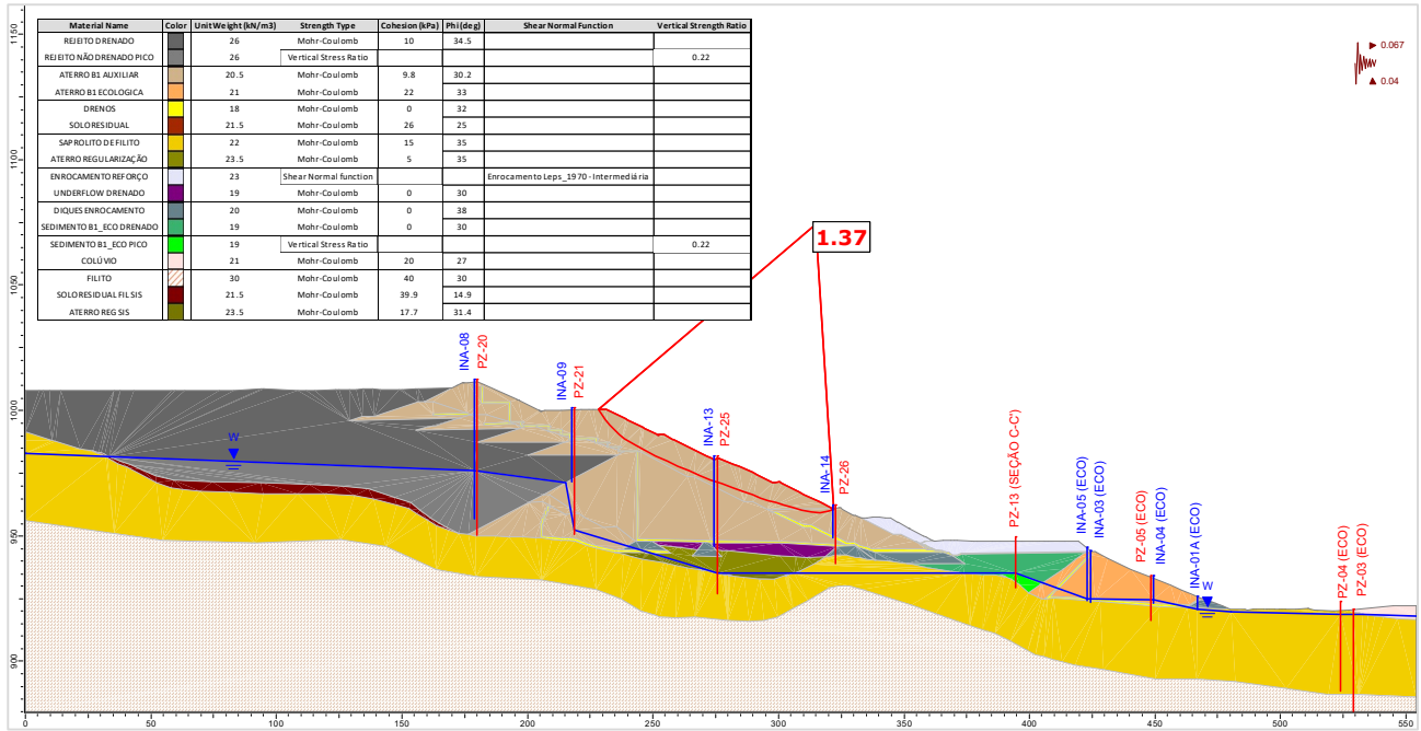
Figura 5.120 – Seção B-B' – Análise Não Drenada – Superfície de ruptura plano-circular otimizada – Freática 29/01/2024 – Razão de resistência não drenada de pico + sismo ↑ (critério vida útil).
