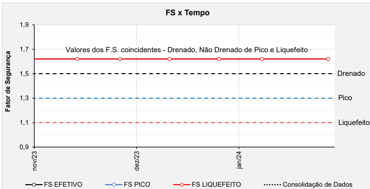
Figura 5.151 – Seção B-B' - Histórico dos F.S. obtidos nas análises de estabilidade no período avaliado.
