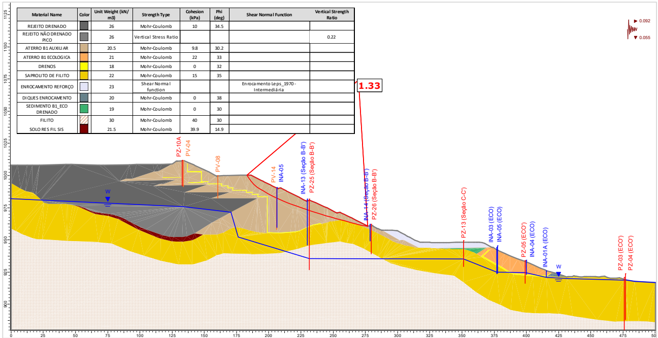
Figura 5.112 – Seção A-A' – Análise Não Drenada – Superfície de ruptura plano-circular otimizada – Freática 29/01/2024 – Razão de resistência não drenada de pico + sismo ↓ (critério CDA).
