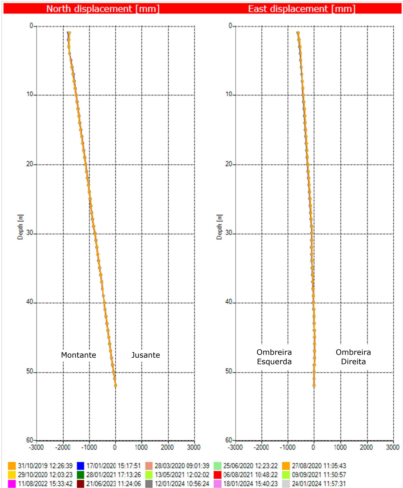
Figura 5.103 – Deslocamentos horizontais acumulados do INC-02 (ref. 24/01/2024).
