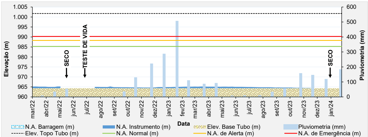
Figura 5.52 – Desempenho do piezômetro de tubo aberto - PZ-22.
