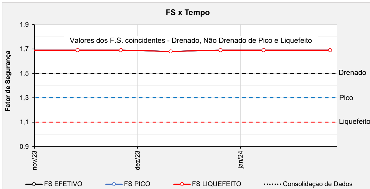
Figura 5.154 – Seção E-E' - Histórico dos F.S. obtidos nas análises de estabilidade no período avaliado.
