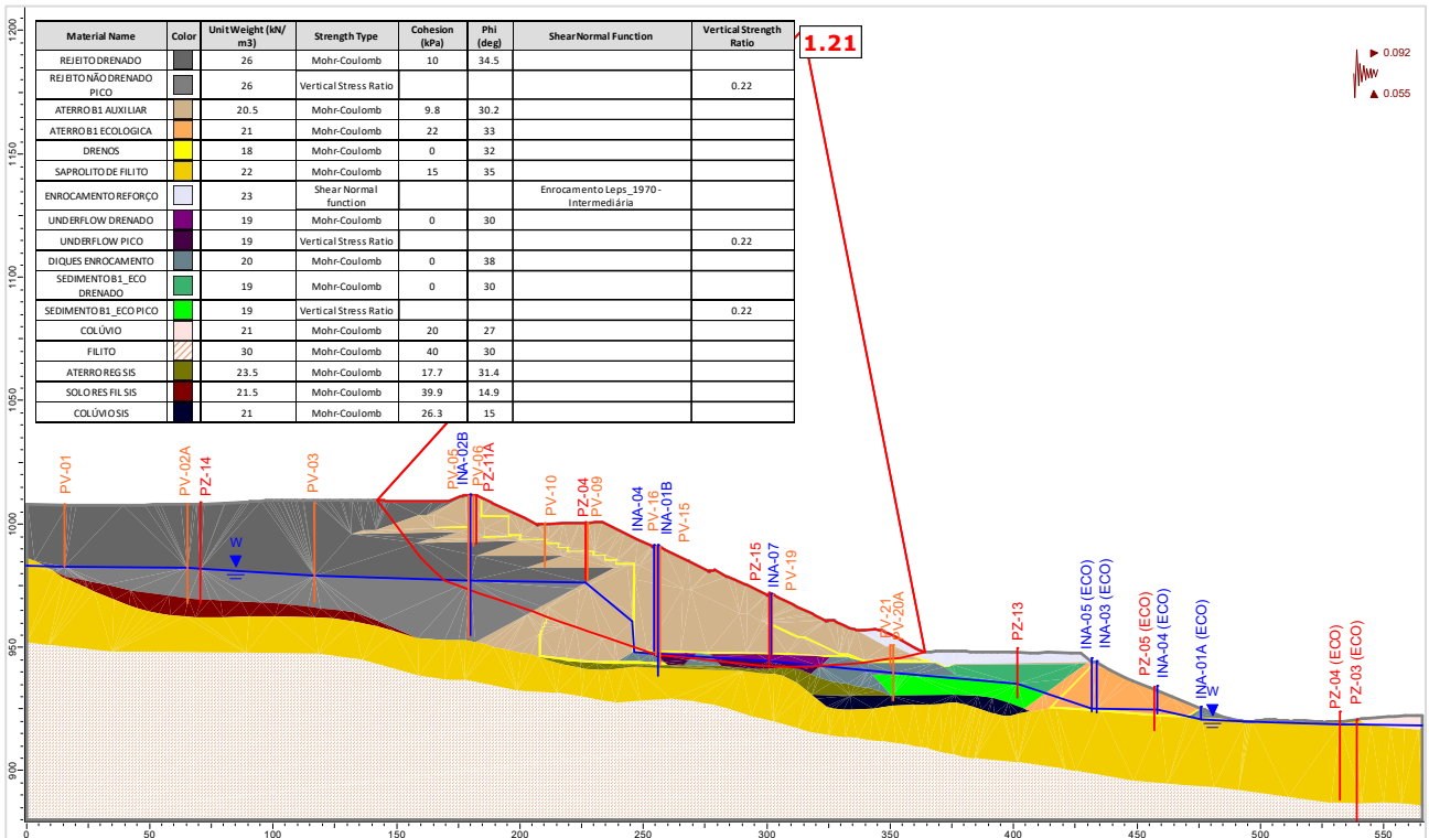
Figura 5.125 – Seção C-C' – Análise Não Drenada – Superfície de ruptura plano-circular otimizada – Freática 29/01/2024 – Razão de resistência não drenada de pico + sismo ↑ (critério CDA).
