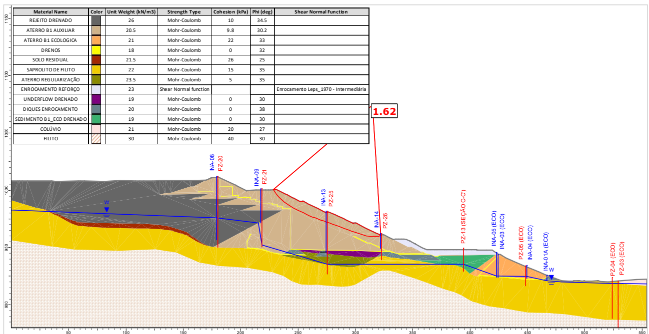
Figura 5.115 – Seção B-B’ – Análise Drenada – Superfície de ruptura plano-circular otimizada – Freática 29/01/2024.
