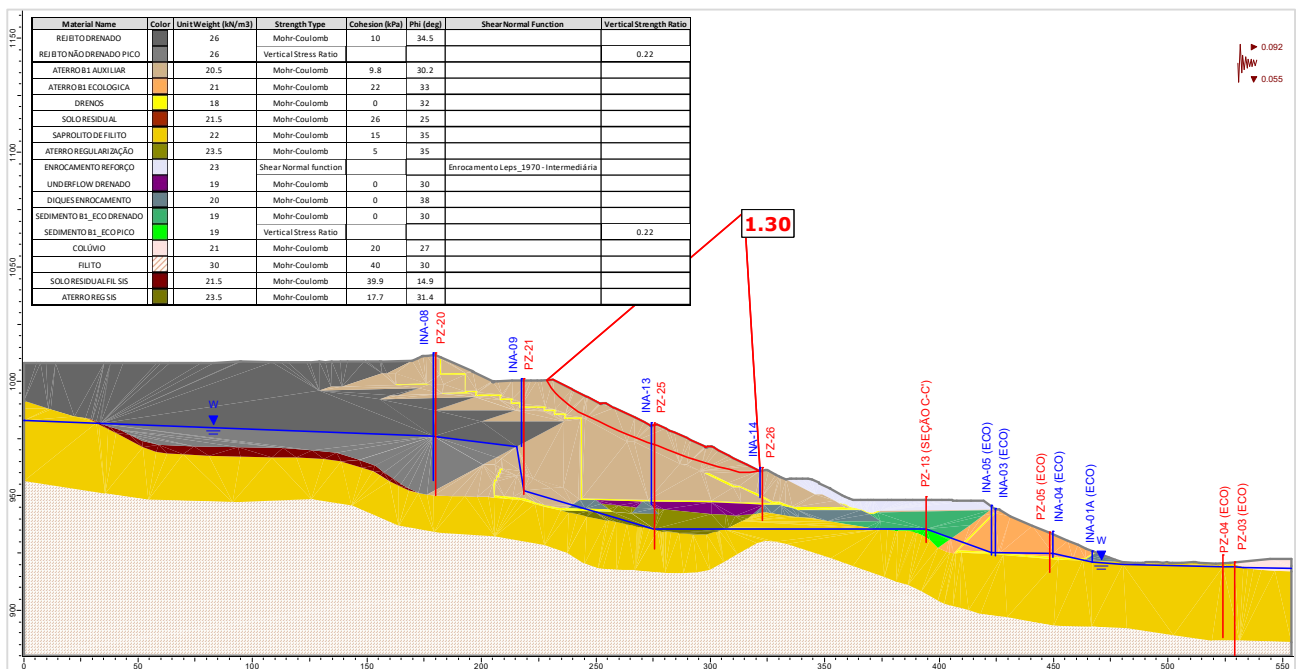
Figura 5.119 – Seção B-B' – Análise Não Drenada – Superfície de ruptura plano-circular otimizada – Freática 29/01/2024 – Razão de resistência não drenada de pico + sismo ↓ (critério CDA).
