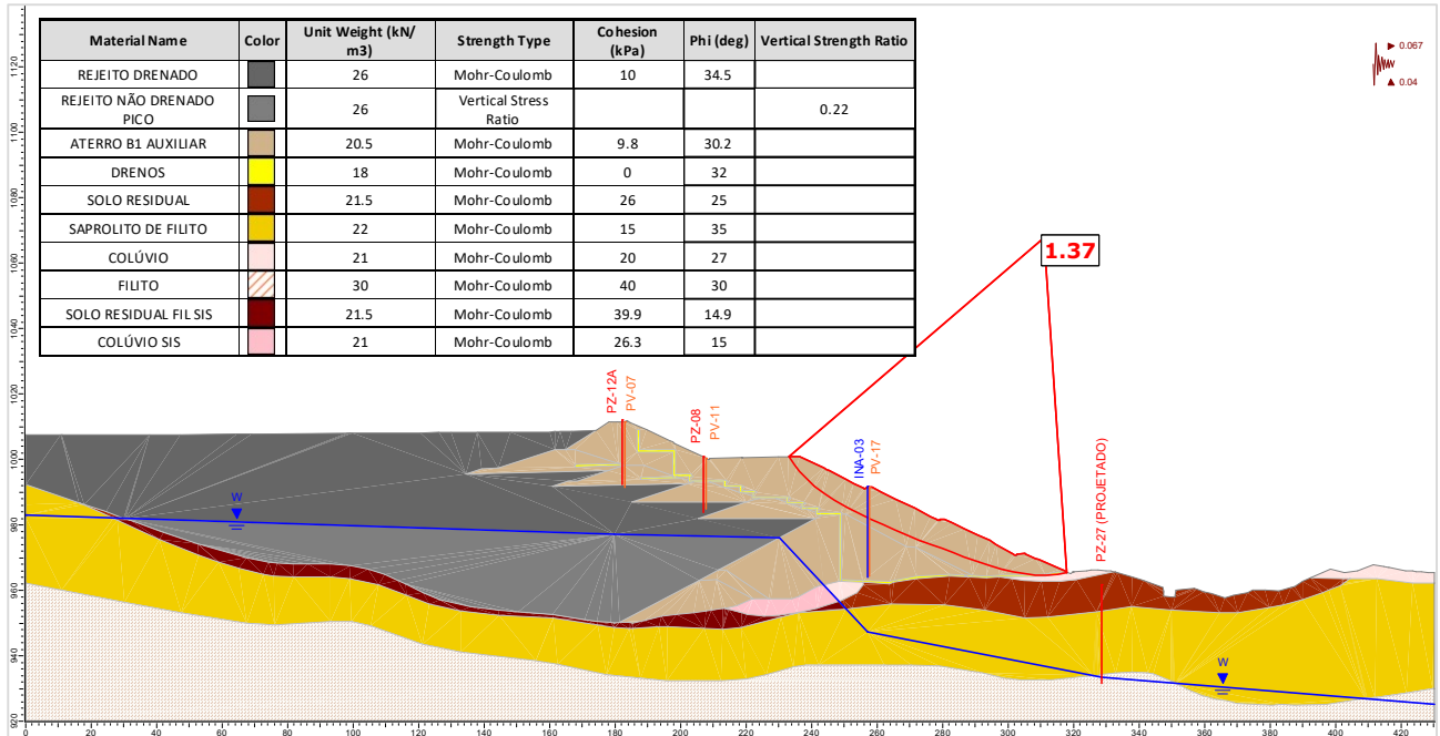
Figura 5.134 – Seção D-D' – Análise Não Drenada – Superfície de ruptura plano-circular otimizada – Freática 29/01/2024 – Razão de resistência não drenada de pico + sismo ↑ (critério vida útil).
