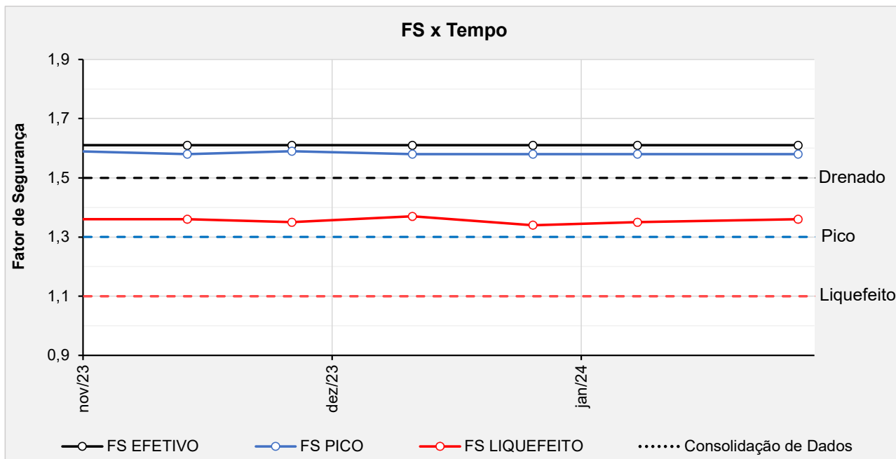
Figura 5.152 – Seção C-C' - Histórico dos F.S. obtidos nas análises de estabilidade no período avaliado.
