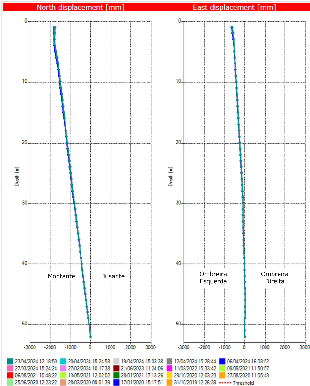
Figura 5.103 – Deslocamentos horizontais acumulados do INC-02 (ref. 23/04/2024).
