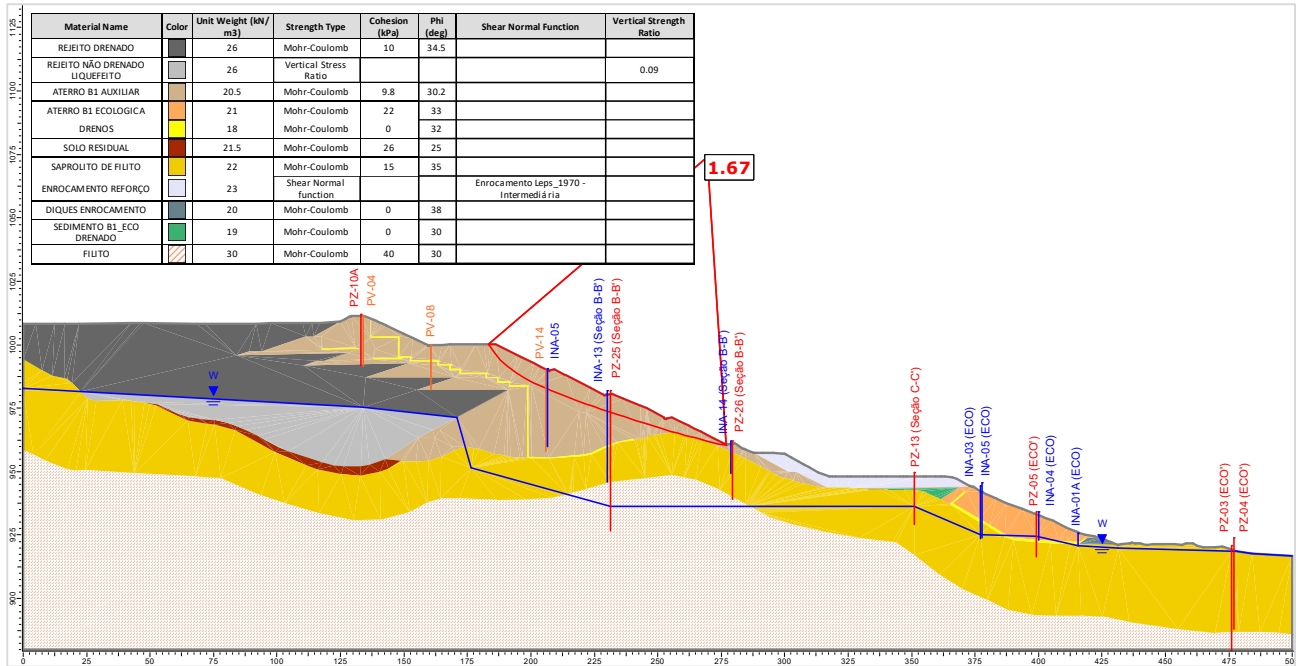
Figura 5.110 – Seção A-A' – Análise Não Drenada – Superfície de ruptura plano-circular otimizada – Freática 30/04/2024 – Razão de resistência não drenada liquefeita.
