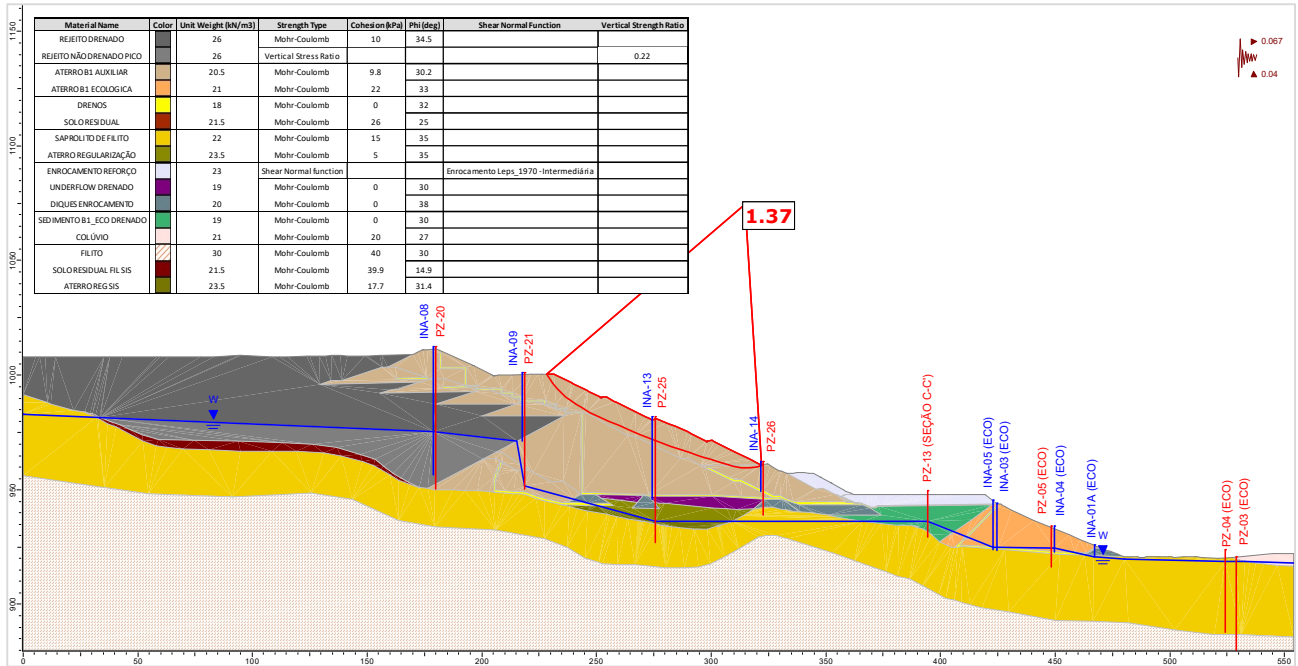
Figura 5.120 – Seção B-B' – Análise Não Drenada – Superfície de ruptura plano-circular otimizada – Freática 30/04/2024 – Razão de resistência não drenada de pico + sismo ↑ (critério vida útil).
