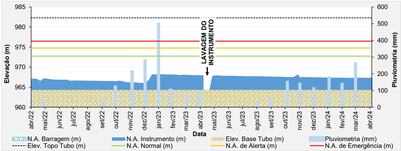
Figura 5.54 – Desempenho do piezômetro de tubo aberto - PZ-24.
