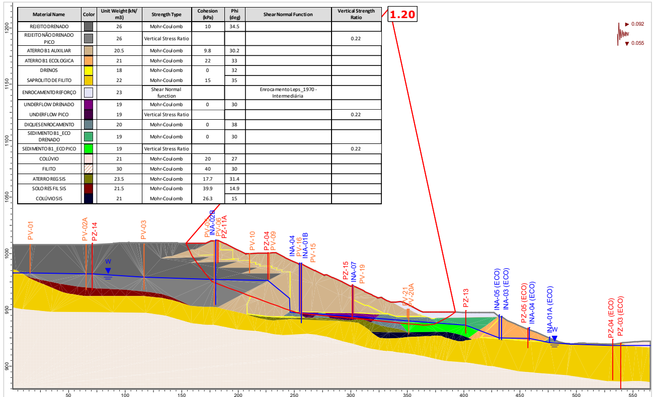
Figura 5.126 – Seção C-C' – Análise Não Drenada – Superfície de ruptura plano-circular otimizada – Freática 30/04/2024 – Razão de resistência não drenada de pico + sismo ↓ (critério CDA).
