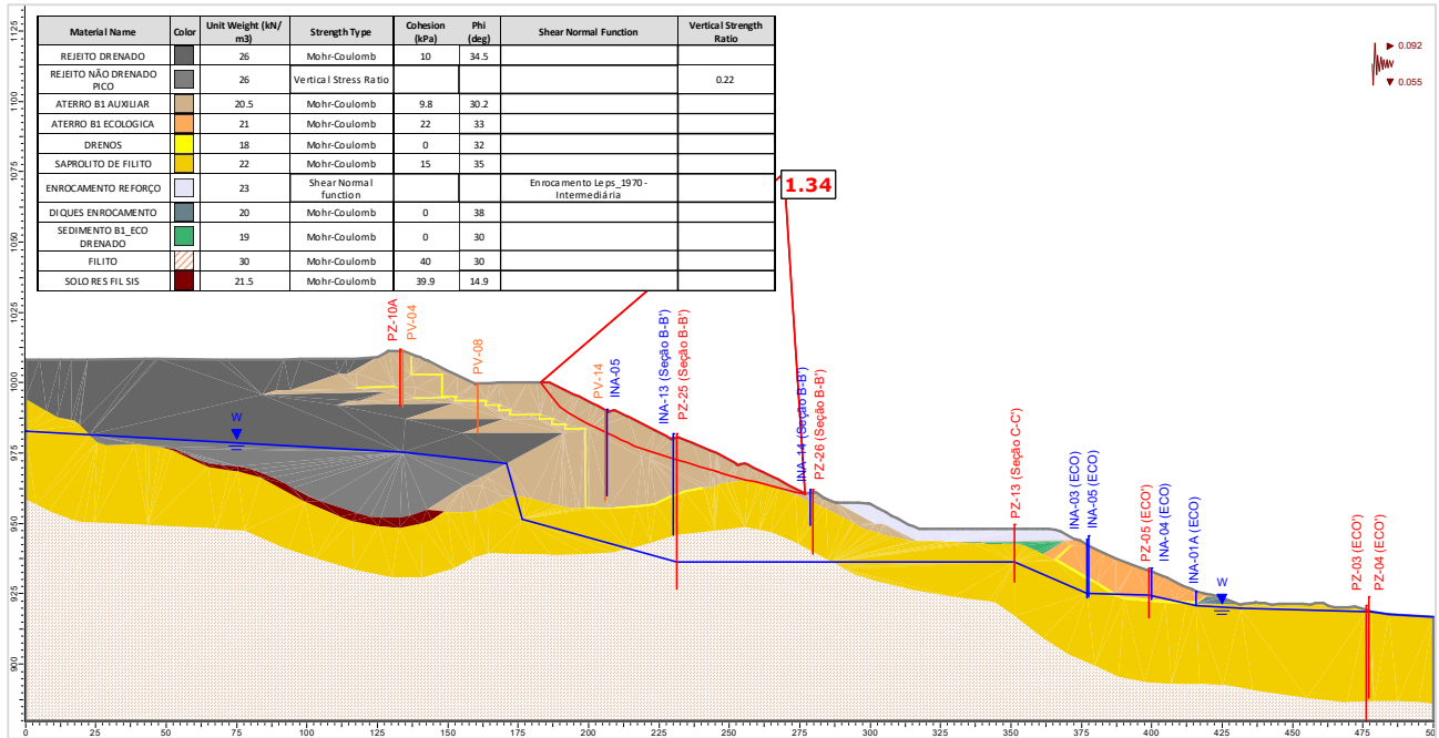
Figura 5.112 – Seção A-A' – Análise Não Drenada – Superfície de ruptura plano-circular otimizada – Freática 30/04/2024 – Razão de resistência não drenada de pico + sismo ↓ (critério CDA).
