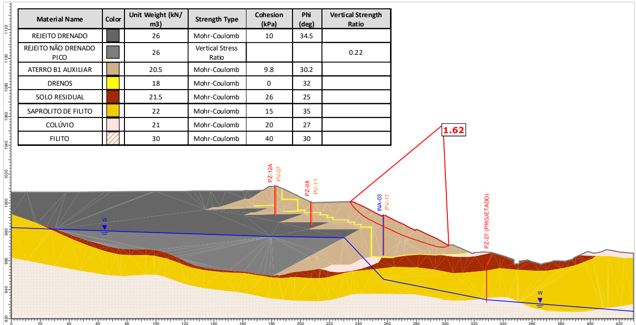
Figura 5.130 – Seção D-D' – Análise Não Drenada – Superfície de ruptura plano-circular otimizada – Freática 30/04/2024 – Razão de resistência não drenada de pico.
