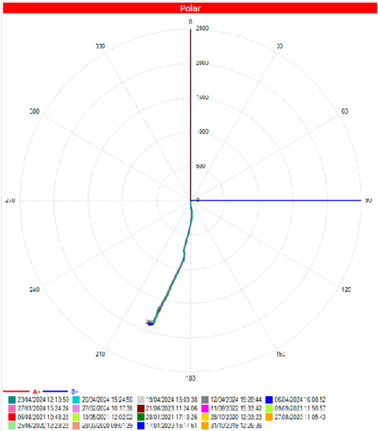
Figura 5.104 – Deslocamentos em relação a coordenadas polares acumulados do INC-02 (ref. 23/04/2024).
