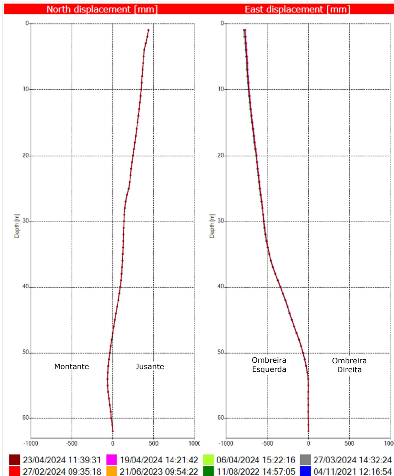
Figura 5.101 – Deslocamentos horizontais acumulados do INC-01 (ref. 23/04/2024).
