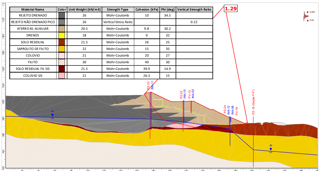
Figura 5.141 – Seção E-E' – Análise Não Drenada – Superfície de ruptura plano-circular otimizada – Freática 30/04/2024 – Razão de resistência não drenada de pico + sismo ↑ (critério vida útil).
