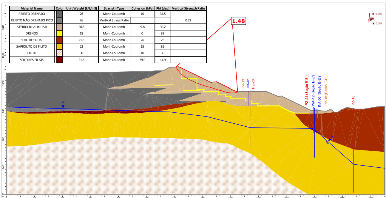
Figura 5.147 – Seção F-F' – Análise Não Drenada – Superfície de ruptura plano-circular otimizada – Freática 30/04/2024 – Razão de resistência não drenada de pico + sismo ↓ (critério CDA).
