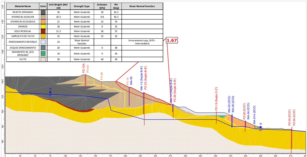
Figura 5.108 – Seção A-A' – Análise Drenada – Superfície de ruptura plano-circular otimizada – Freática 30/04/2024.
