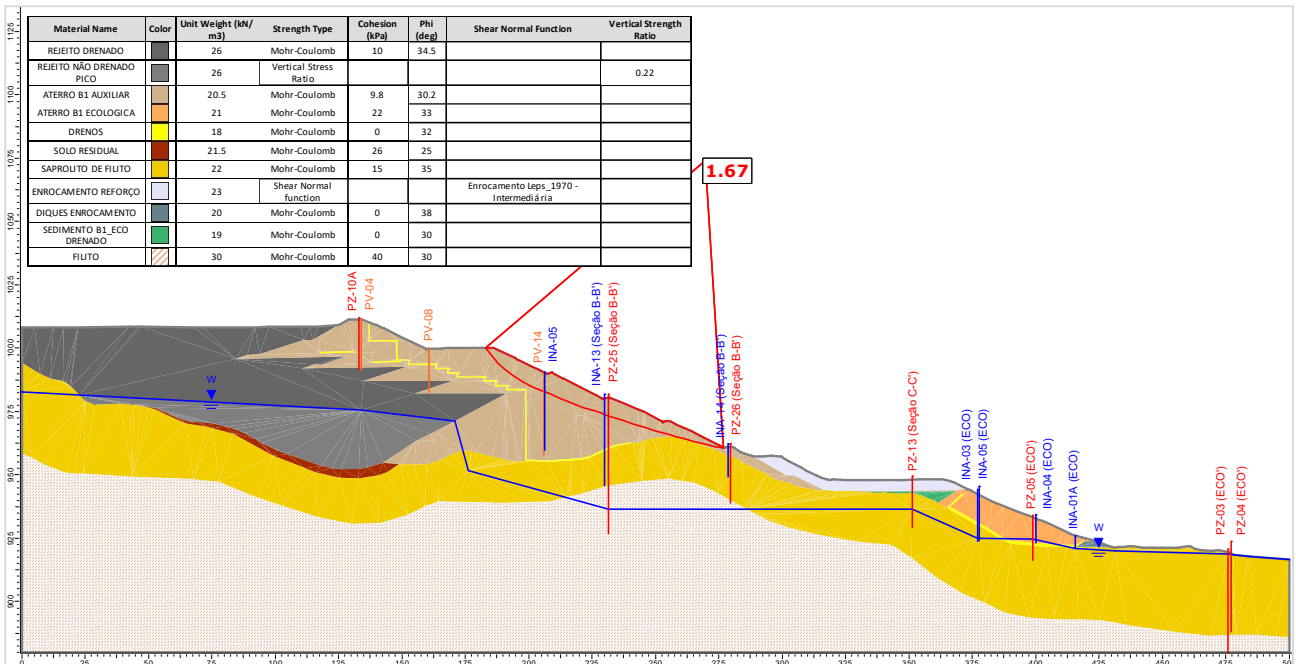
Figura 5.109 – Seção A-A' – Análise Não Drenada – Superfície de ruptura plano-circular otimizada – Freática 30/04/2024 – Razão de resistência não drenada de pico.
