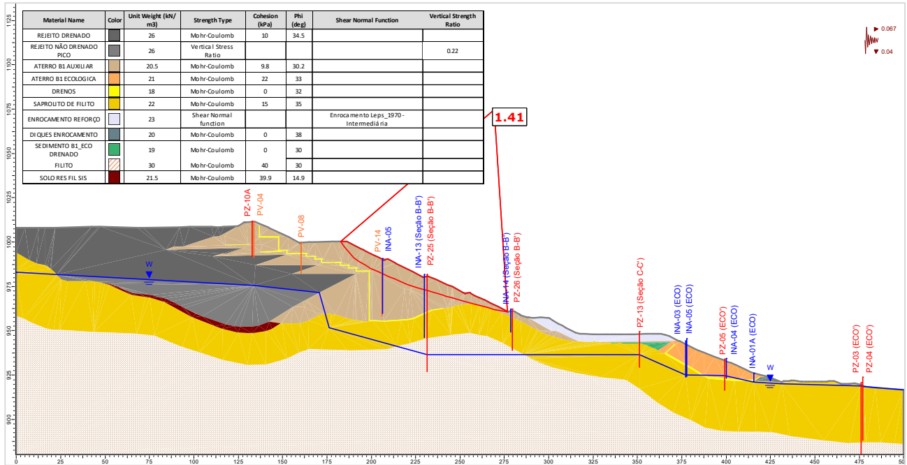
Figura 5.114 – Seção A-A’ – Análise Não Drenada – Superfície de ruptura plano-circular otimizada – Freática 30/04/2024 – Razão de resistência não drenada de pico + sismo ↓ (critério vida útil).
