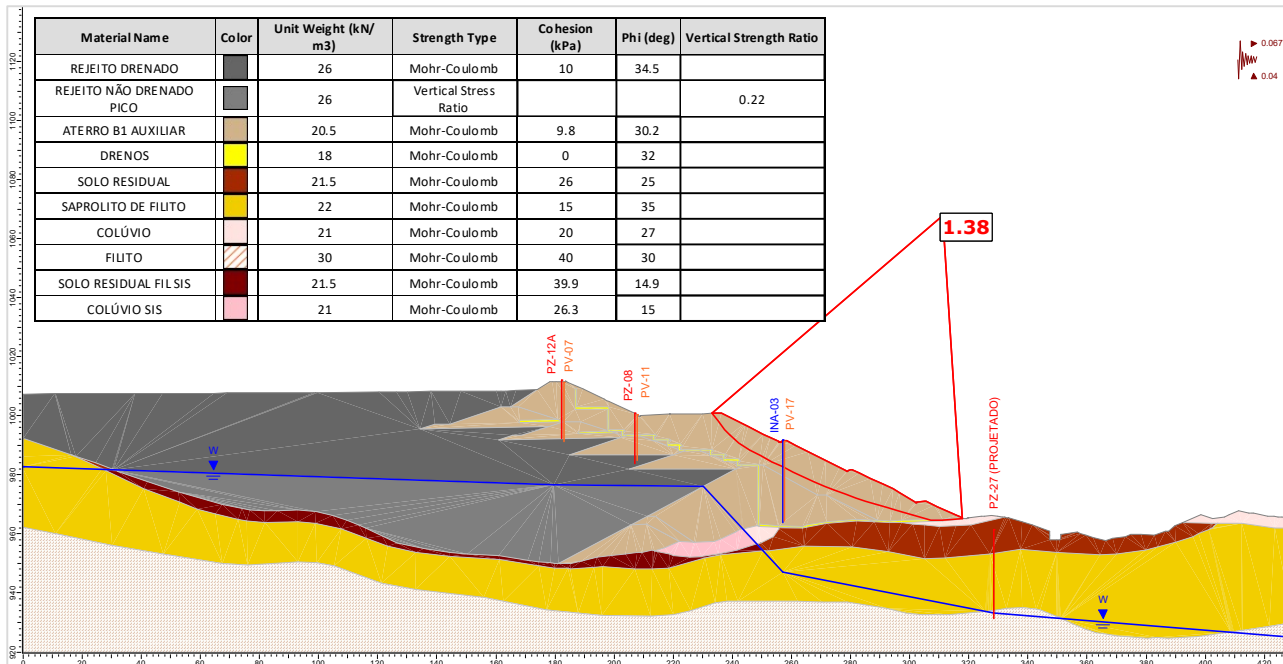
Figura 5.134 – Seção D-D' – Análise Não Drenada – Superfície de ruptura plano-circular otimizada – Freática 30/04/2024 – Razão de resistência não drenada de pico + sismo ↑ (critério vida útil).
