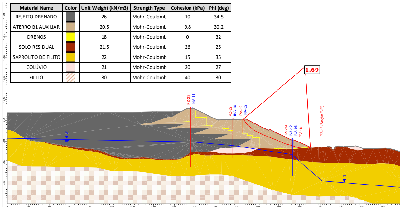
Figura 5.136 – Seção E-E' – Análise Drenada – Superfície de ruptura plano-circular otimizada – Freática 30/04/2024.
