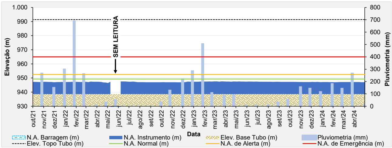
Figura 5.63 – Desempenho do indicador de nível d'água - INA-01B.
