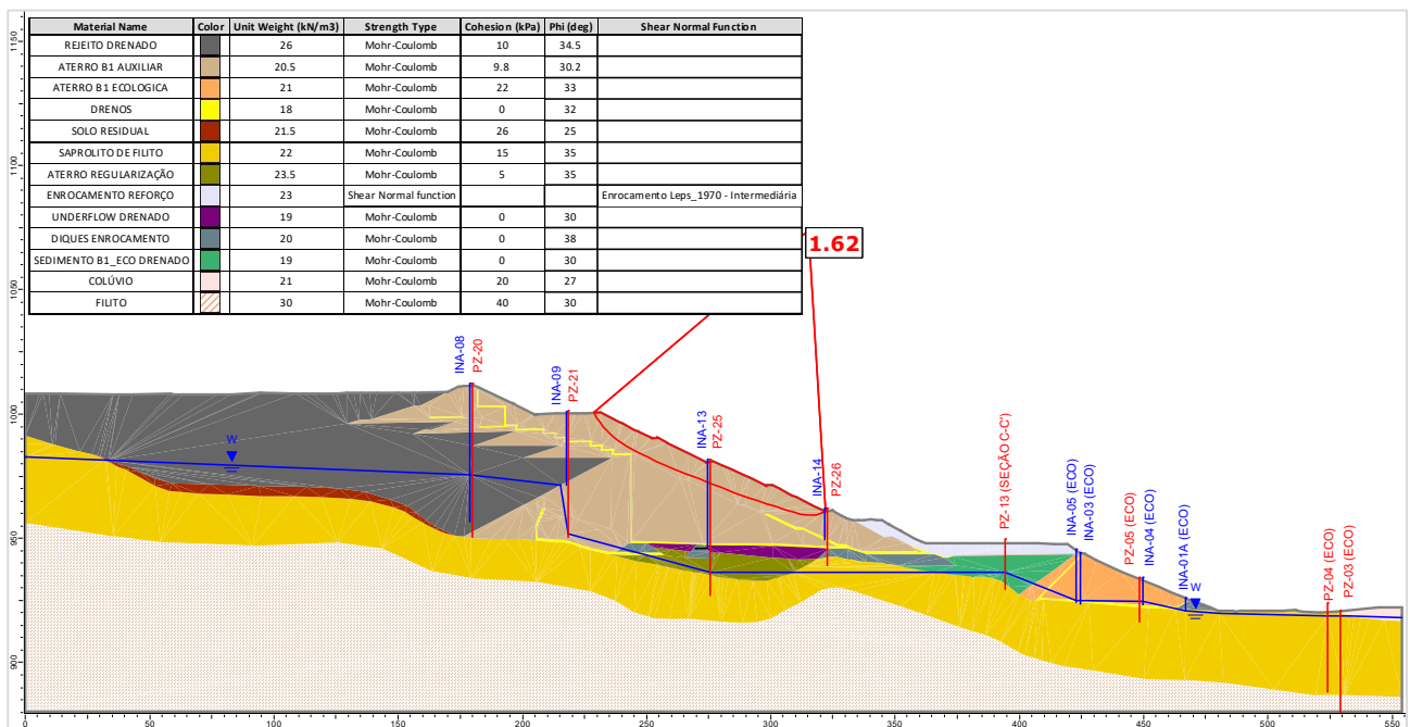
Figura 5.115 – Seção B-B’ – Análise Drenada – Superfície de ruptura plano-circular otimizada – Freática 30/04/2024.
