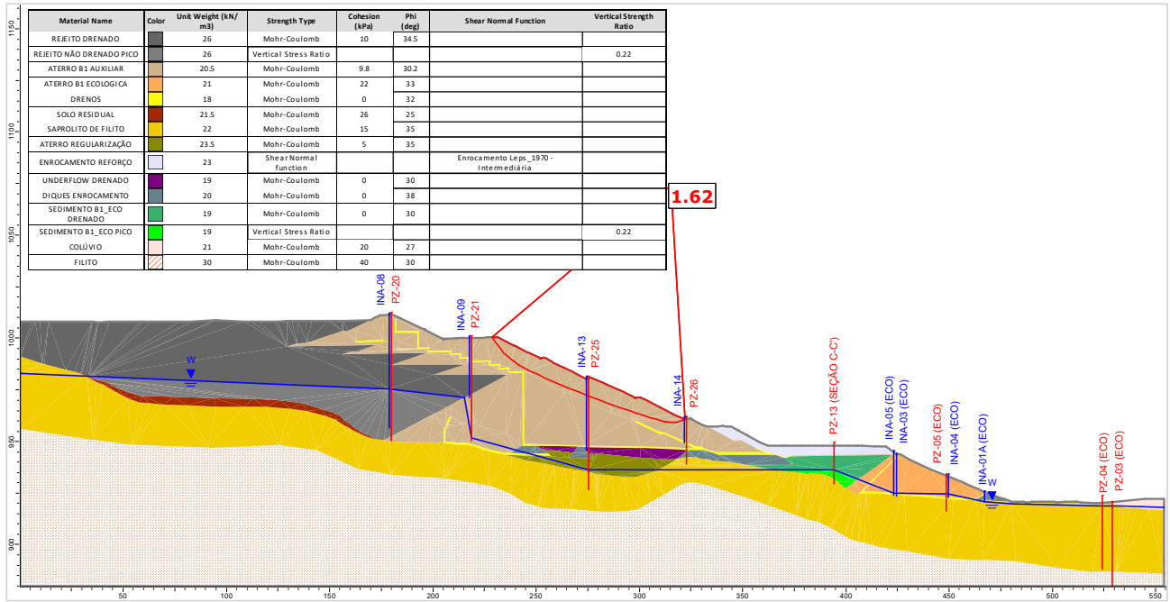
Figura 5.116 – Seção B-B' – Análise Não Drenada – Superfície de ruptura plano-circular otimizada – Freática 30/04/2024 – Razão de resistência não drenada de pico.
