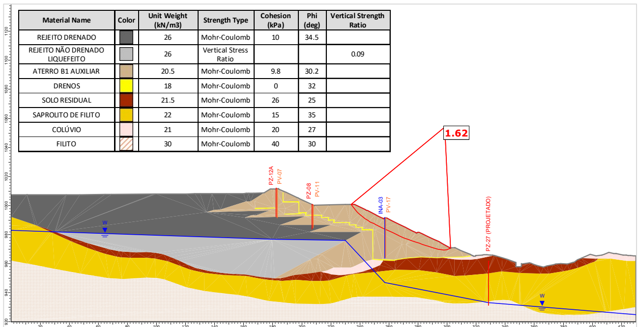
Figura 5.131 – Seção D-D' – Análise Não Drenada – Superfície de ruptura plano-circular otimizada – Freática 30/04/2024 – Razão de resistência não drenada liquefeita.
