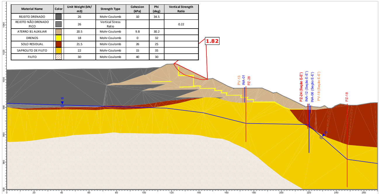
Figura 5.144 – Seção F-F' – Análise Não Drenada – Superfície de ruptura plano-circular otimizada – Freática 30/04/2024 – Razão de resistência não drenada de pico.
