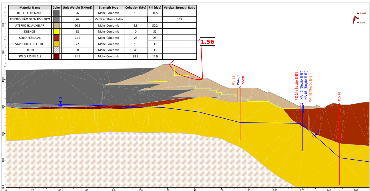
Figura 5.149 – Seção F-F' – Análise Não Drenada – Superfície de ruptura plano-circular otimizada – Freática 30/04/2024 – Razão de resistência não drenada de pico + sismo ↓ (critério vida útil).
