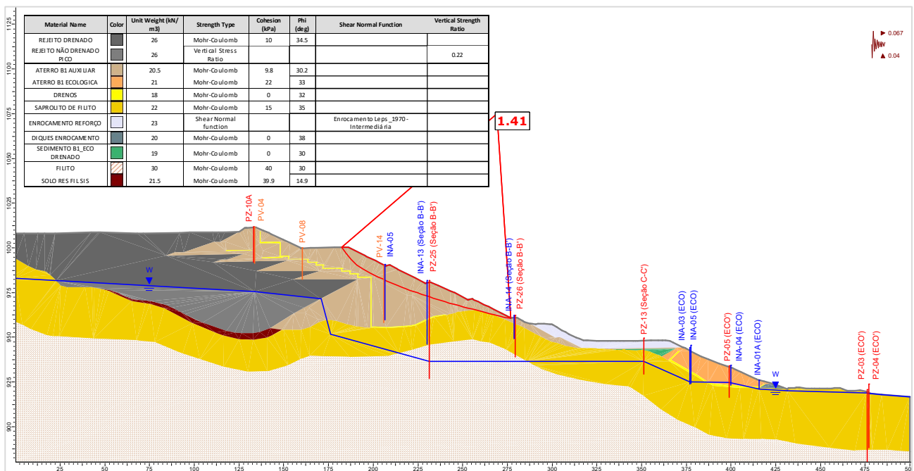
Figura 5.113 – Seção A-A' – Análise Não Drenada – Superfície de ruptura plano-circular otimizada – Freática 30/04/2024 – Razão de resistência não drenada de pico + sismo ↑ (critério vida útil).
