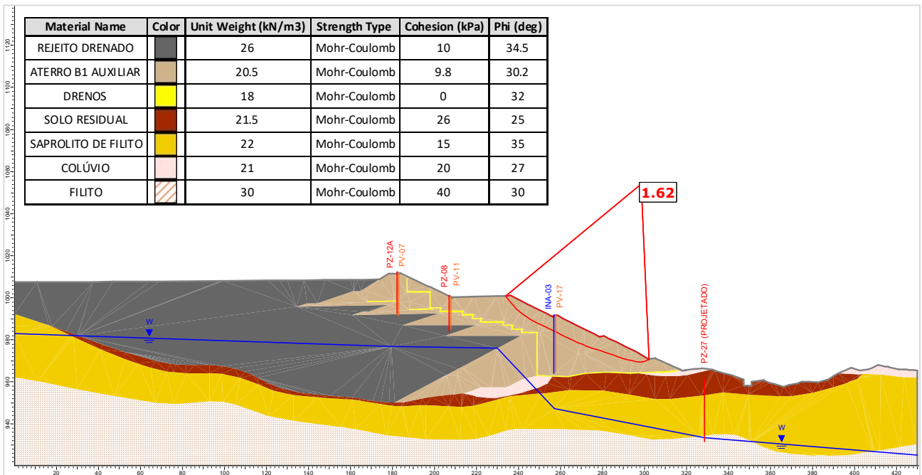
Figura 5.129 – Seção D-D' – Análise Drenada – Superfície de ruptura plano-circular otimizada – Freática 30/04/2024.
