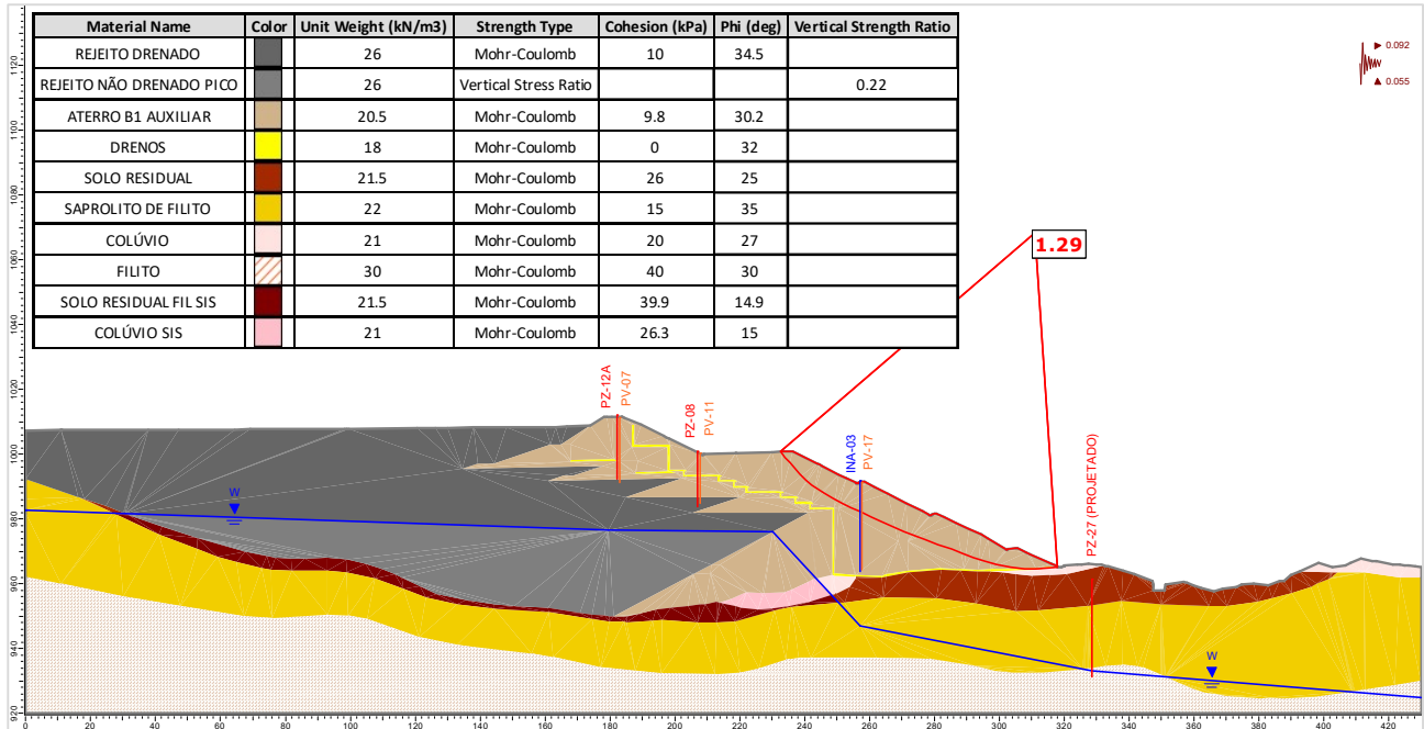
Figura 5.132 – Seção D-D' – Análise Não Drenada – Superfície de ruptura plano-circular otimizada – Freática 30/04/2024 – Razão de resistência não drenada de pico + sismo ↑ (critério CDA).
