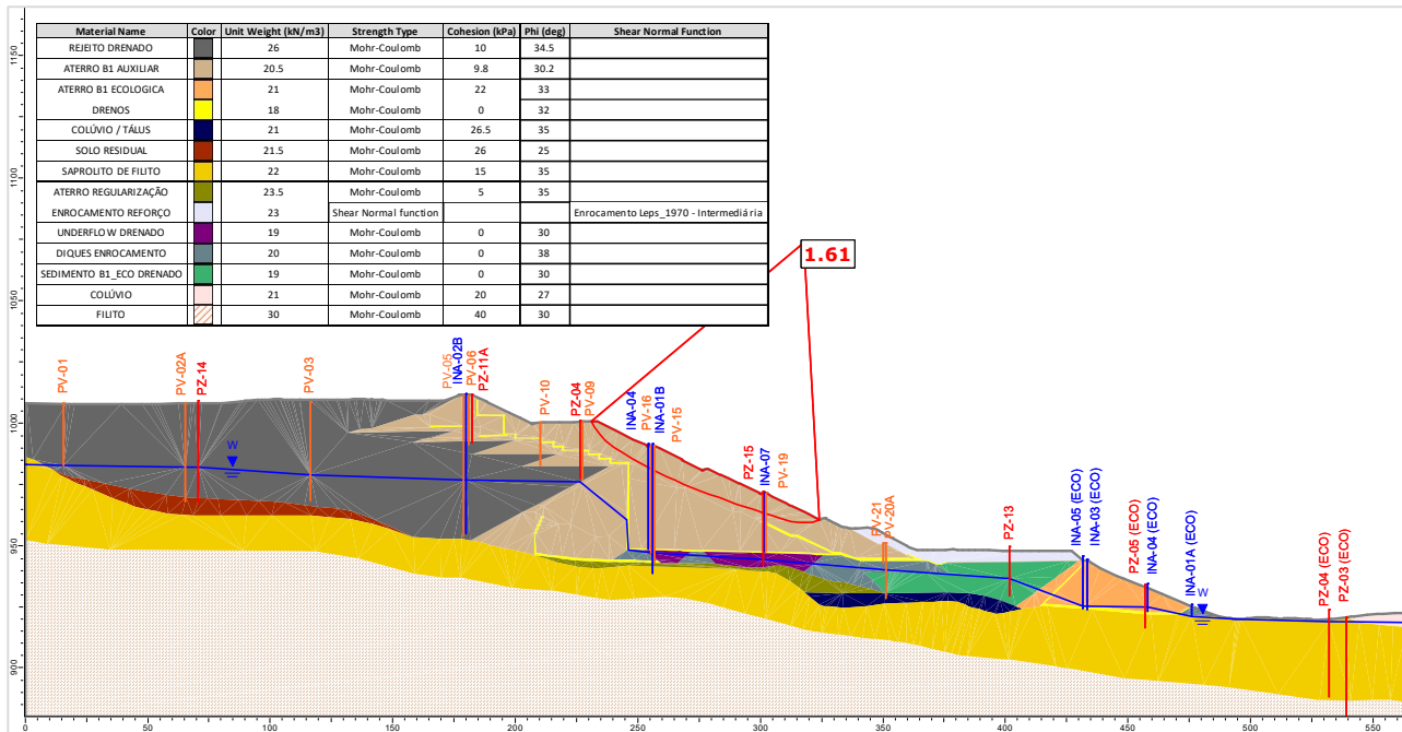
Figura 5.122 – Seção C-C' – Análise Drenada – Superfície de ruptura plano-circular otimizada – Freática 30/04/2024.
