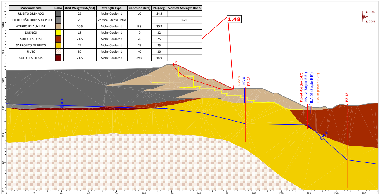
Figura 5.146 – Seção F-F' – Análise Não Drenada – Superfície de ruptura plano-circular otimizada – Freática 30/04/2024 – Razão de resistência não drenada de pico + sismo ↑ (critério CDA).
