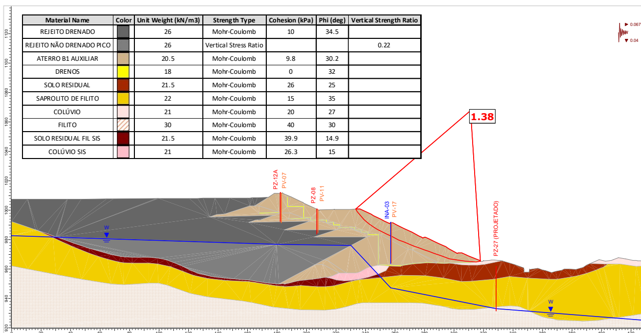
Figura 5.135 – Seção D-D' – Análise Não Drenada – Superfície de ruptura plano-circular otimizada – Freática 30/04/2024 – Razão de resistência não drenada de pico + sismo ↓ (critério vida útil).
