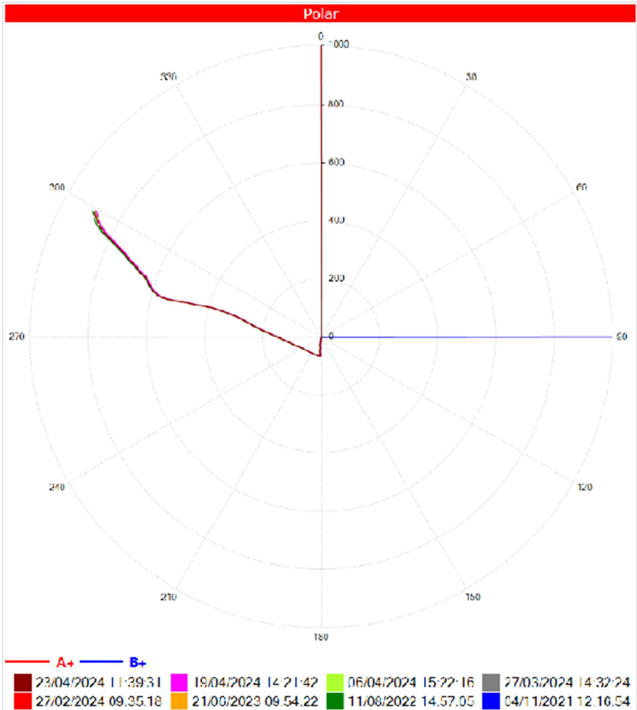
Figura 5.102 – Deslocamentos em relação a coordenadas polares acumulados do INC-01 (ref. 23/04/2024).
