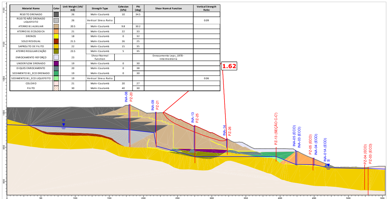
Figura 5.117 – Seção B-B' – Análise Não Drenada – Superfície de ruptura plano-circular otimizada – Freática 30/04/2024 – Razão de resistência não drenada liquefeita.
