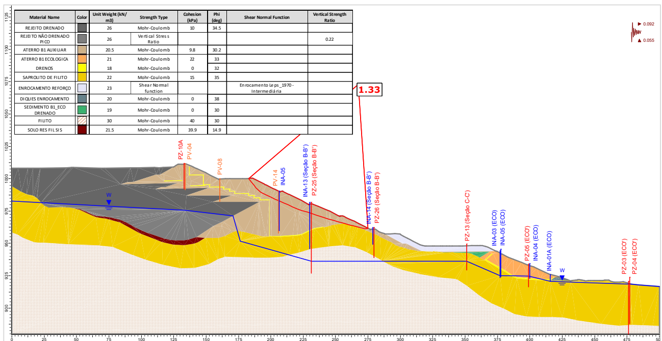
Figura 5.111 – Seção A-A' – Análise Não Drenada – Superfície de ruptura plano-circular otimizada – Freática 30/04/2024 – Razão de resistência não drenada de pico + sismo ↑ (critério CDA).
