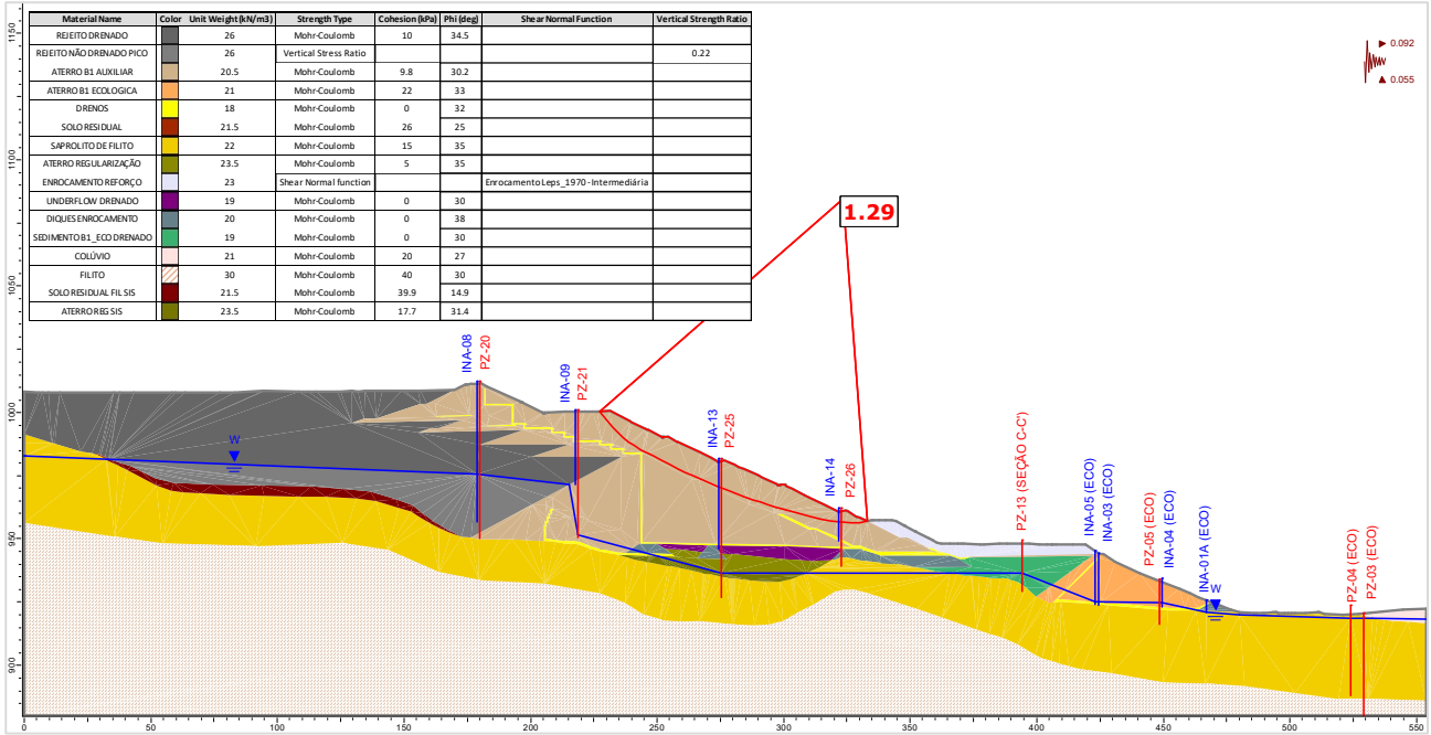
Figura 5.118 – Seção B-B' – Análise Não Drenada – Superfície de ruptura plano-circular otimizada – Freática 30/04/2024 – Razão de resistência não drenada de pico + sismo ↑ (critério CDA).
