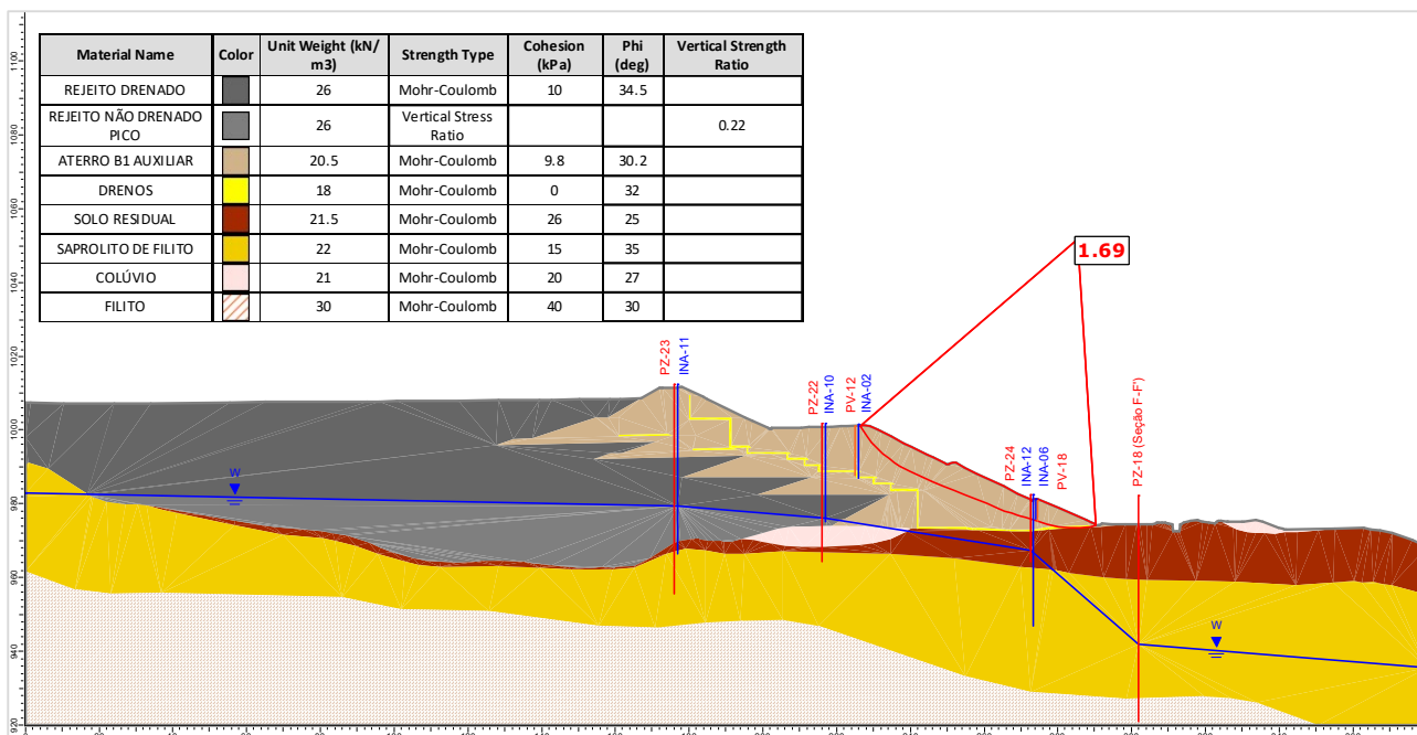
Figura 5.137 – Seção E-E' – Análise Não Drenada – Superfície de ruptura plano-circular otimizada – Freática 30/04/2024 – Razão de resistência não drenada de pico.
