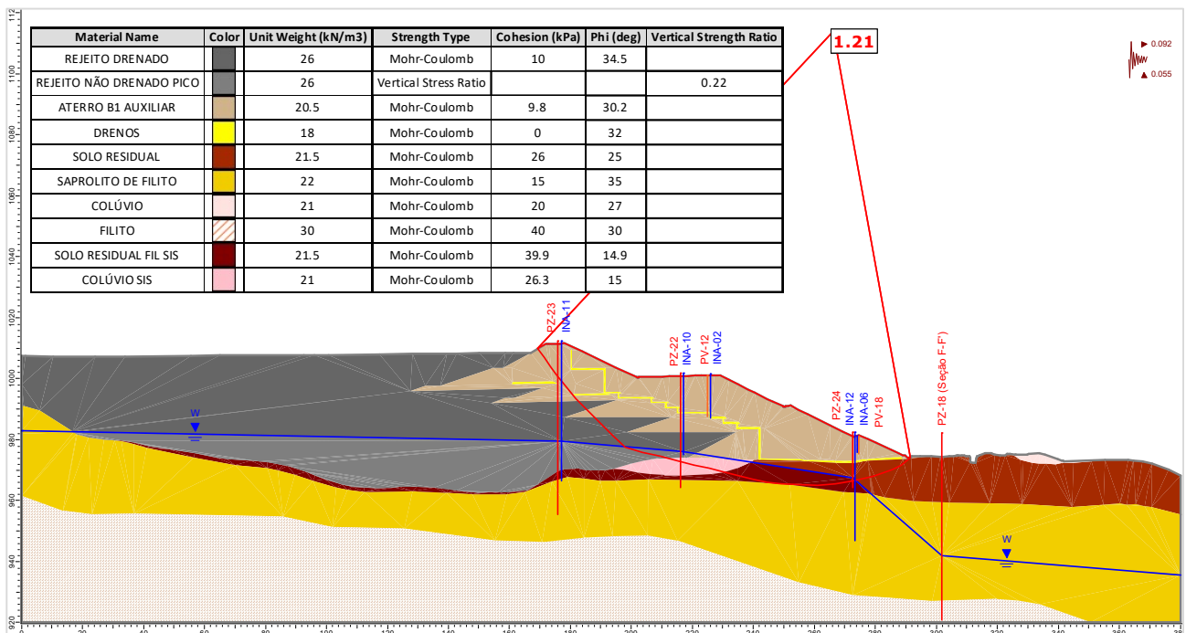
Figura 5.139 – Seção E-E' – Análise Não Drenada – Superfície de ruptura plano-circular otimizada – Freática 30/04/2024 – Razão de resistência não drenada de pico + sismo ↑ (critério CDA).
