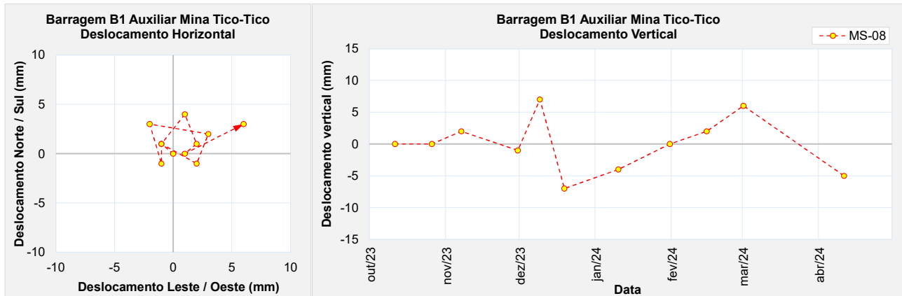
Figura 5.100 – Marco de controle de deformação – MS-08.
