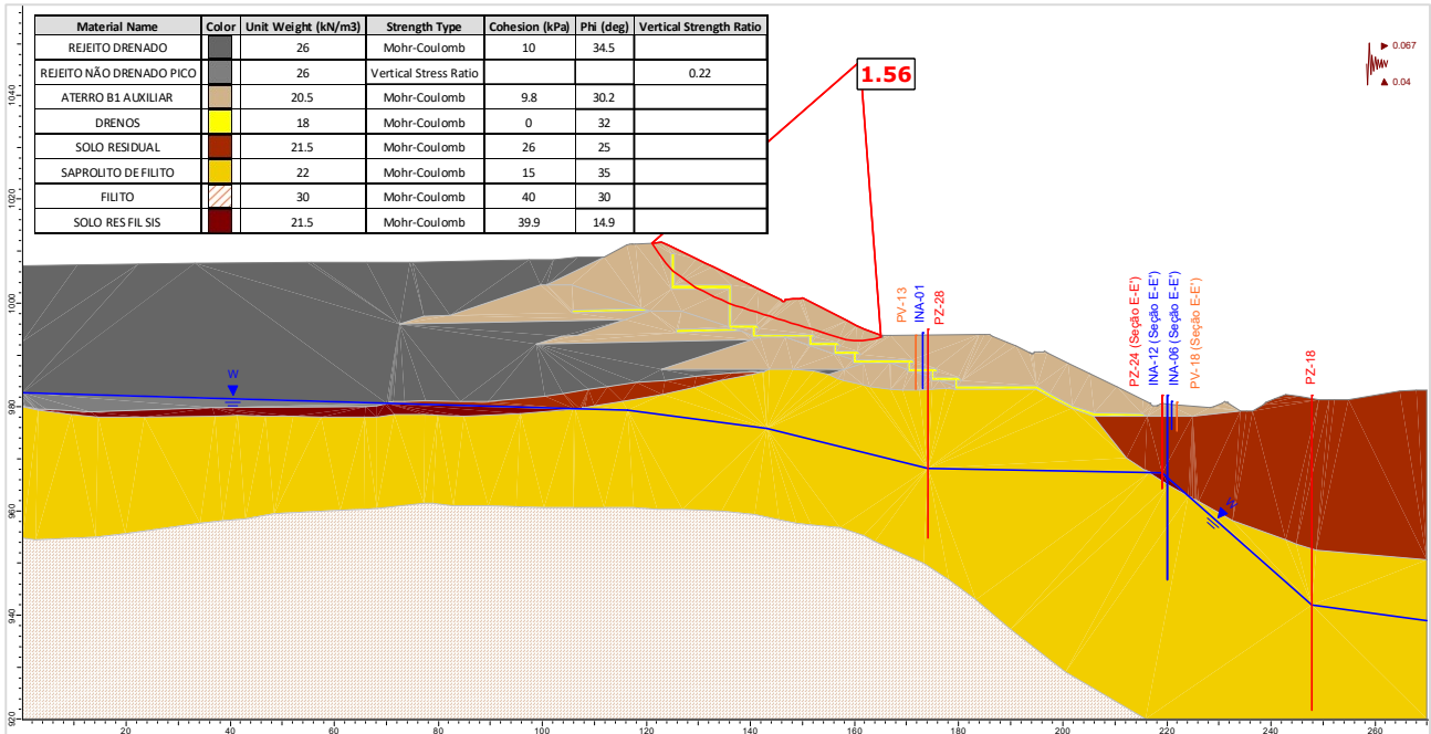
Figura 5.148 – Seção F-F' – Análise Não Drenada – Superfície de ruptura plano-circular otimizada – Freática 30/04/2024 – Razão de resistência não drenada de pico + sismo ↑ (critério vida útil).
