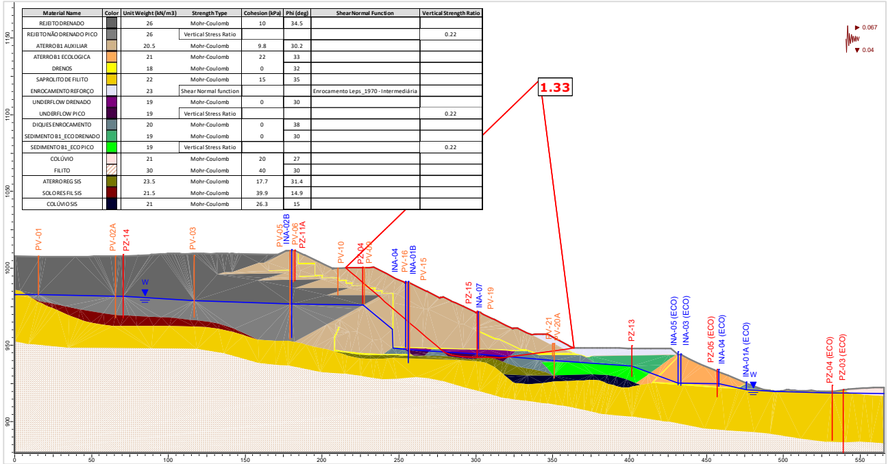
Figura 5.128 – Seção C-C' – Análise Não Drenada – Superfície de ruptura plano-circular otimizada – Freática 30/04/2024 – Razão de resistência não drenada de pico + sismo ↓ (critério vida útil).
