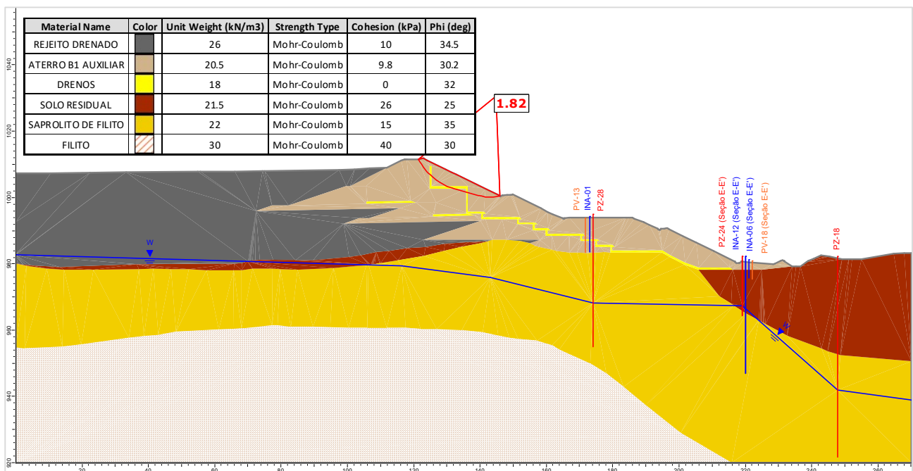
Figura 5.143 – Seção F-F' – Análise Drenada – Superfície de ruptura plano-circular otimizada – Freática 30/04/2024.
