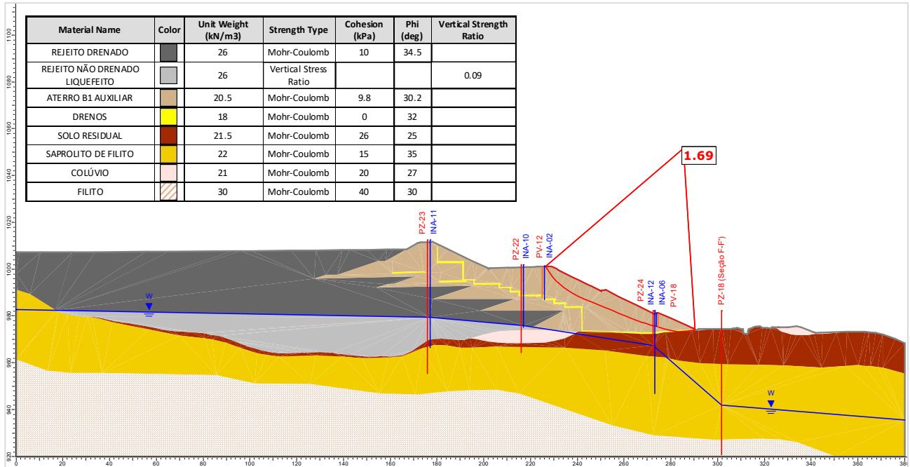
Figura 5.138 – Seção E-E' – Análise Não Drenada – Superfície de ruptura plano-circular otimizada – Freática 30/04/2024 – Razão de resistência não drenada liquefeita.
