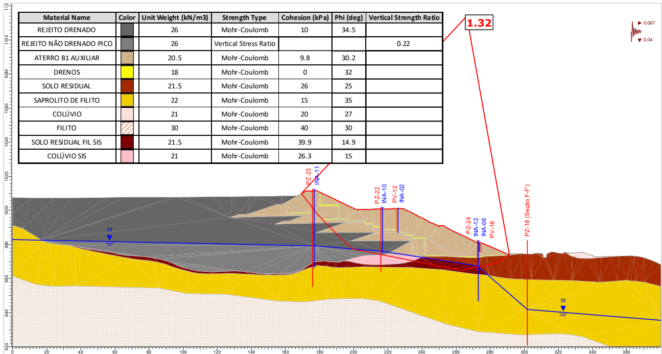
Figura 5.142 – Seção E-E' – Análise Não Drenada – Superfície de ruptura plano-circular otimizada – Freática 30/04/2024 – Razão de resistência não drenada de pico + sismo ↓ (critério vida útil).
