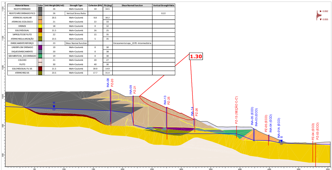
Figura 5.119 – Seção B-B' – Análise Não Drenada – Superfície de ruptura plano-circular otimizada – Freática 30/04/2024 – Razão de resistência não drenada de pico + sismo ↓ (critério CDA).
