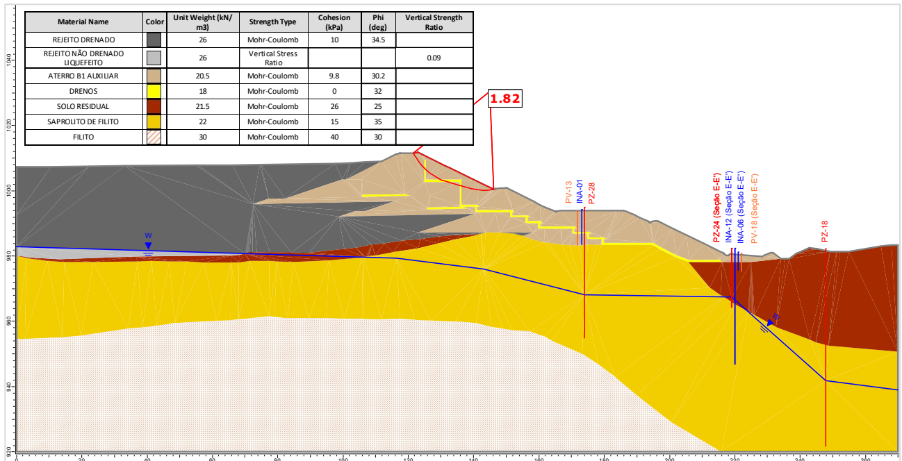
Figura 5.145 – Seção F-F' – Análise Não Drenada – Superfície de ruptura plano-circular otimizada – Freática 30/04/2024 – Razão de resistência não drenada liquefeita.
