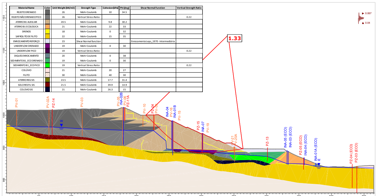
Figura 5.127 – Seção C-C' – Análise Não Drenada – Superfície de ruptura plano-circular otimizada – Freática 30/04/2024 – Razão de resistência não drenada de pico + sismo ↑ (critério vida útil).
