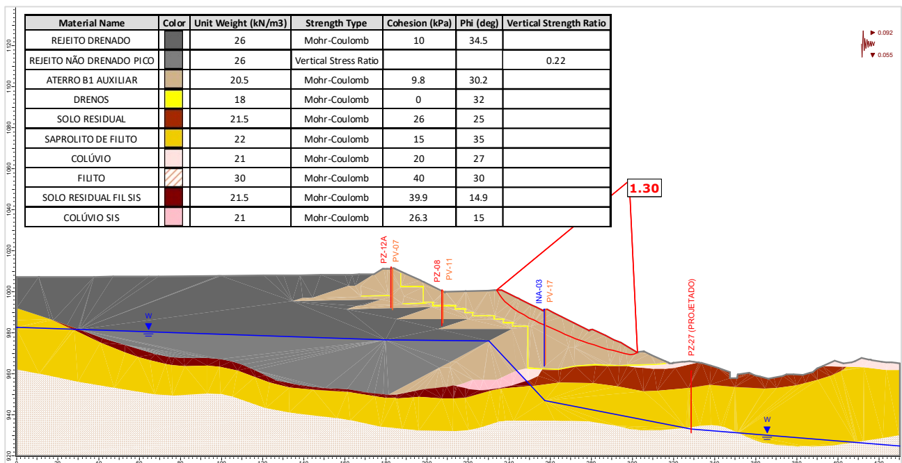
Figura 5.133 – Seção D-D' – Análise Não Drenada – Superfície de ruptura plano-circular otimizada – Freática 30/04/2024 – Razão de resistência não drenada de pico + sismo ↓ (critério CDA).
