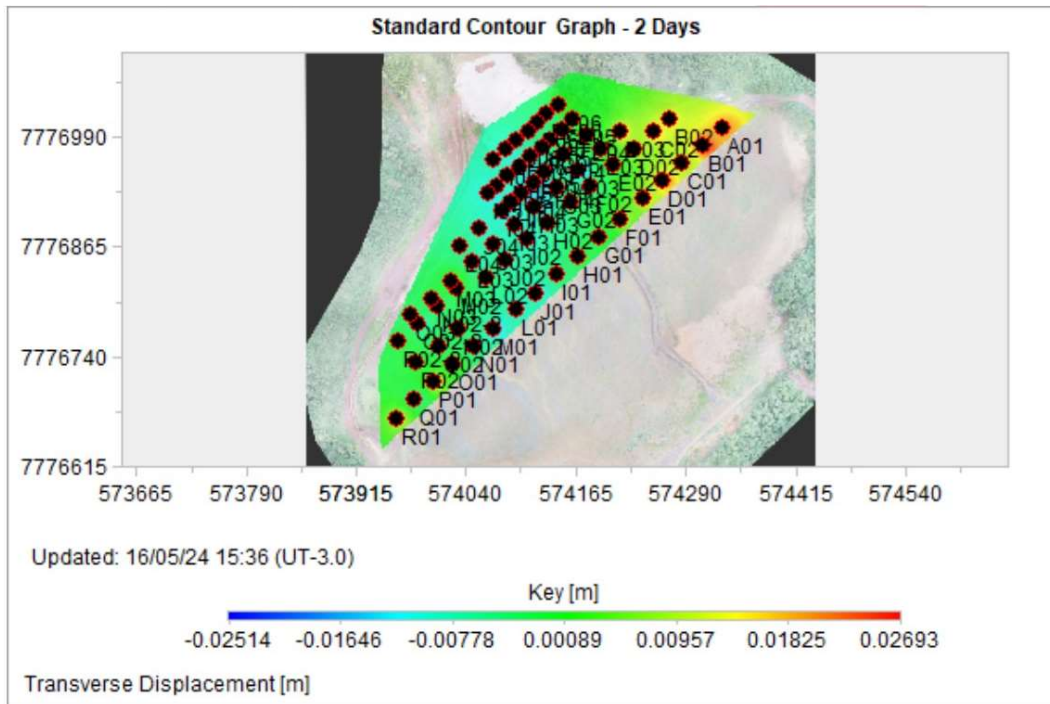
Figura 5.83 – Registros deslocamentos verticais dos prismas.
