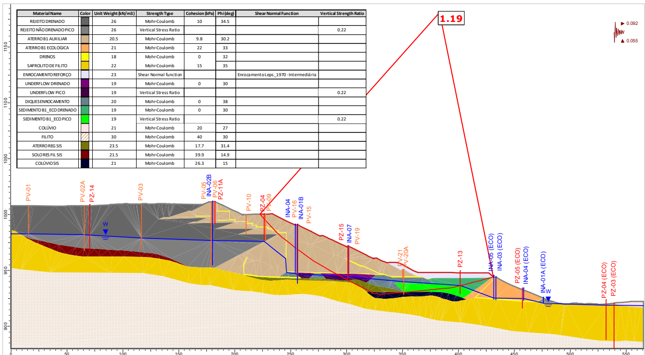
Figura 5.125 – Seção C-C' – Análise Não Drenada – Superfície de ruptura plano-circular otimizada – Freática 30/04/2024 – Razão de resistência não drenada de pico + sismo ↑ (critério CDA).
