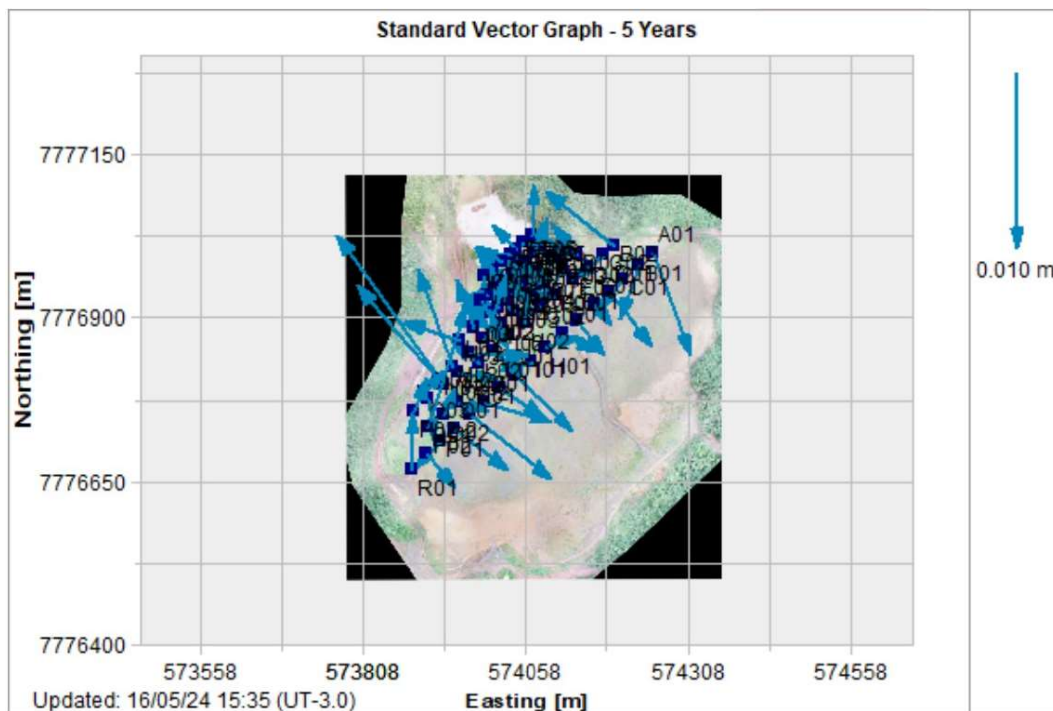
Figura 5.84 – Registros vetores deslocamento dos prismas.
