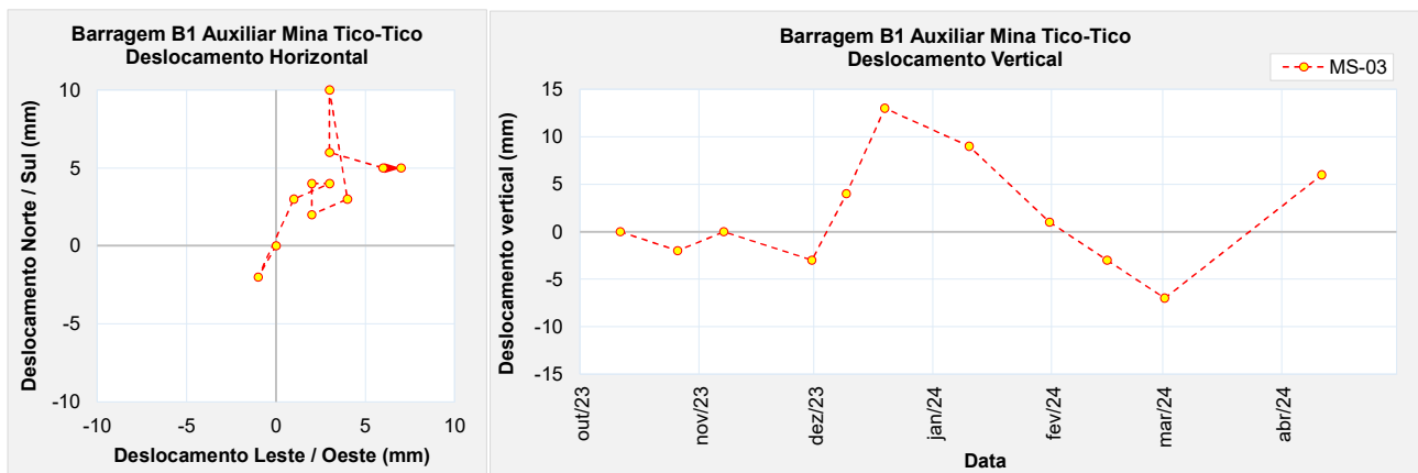
Figura 5.95 – Marco de controle de deformação – MS-03.
