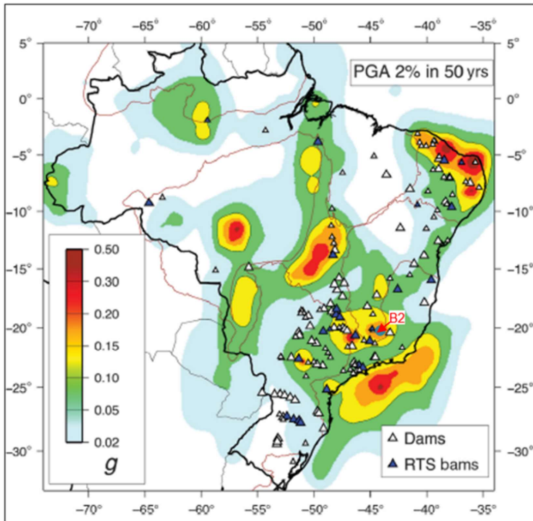
Figura 5.107 – Mapa de Ameaça Sísmica Brasileiro com probabilidade de excedência de 2% durante 50 anos (Barros Et al., 2018).
