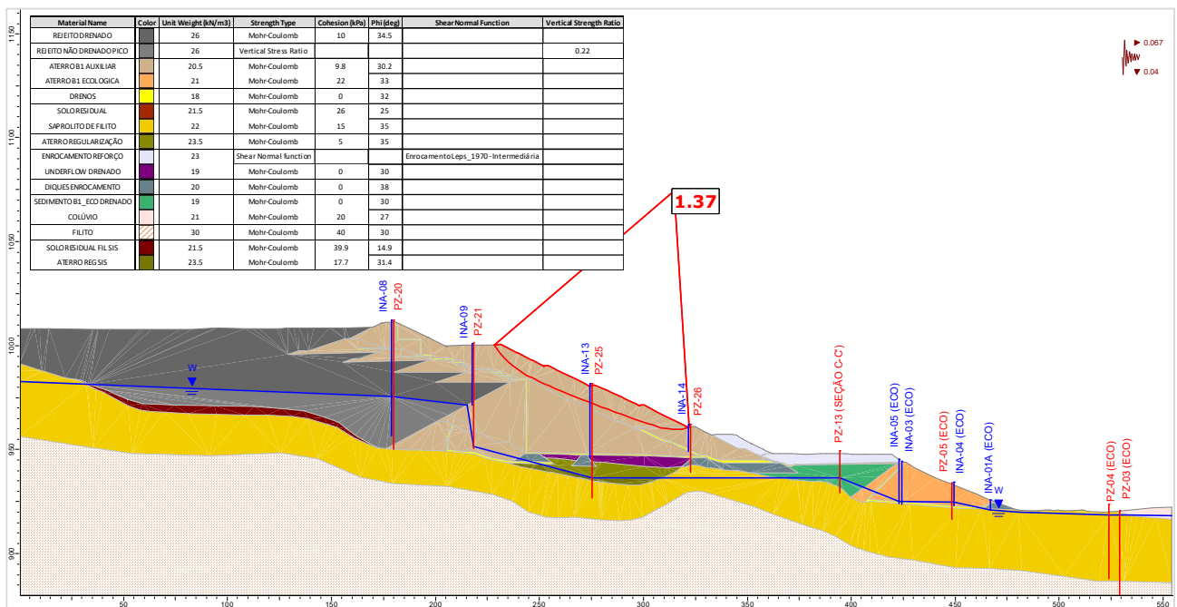
Figura 5.121 – Seção B-B' – Análise Não Drenada – Superfície de ruptura plano-circular otimizada – Freática 30/04/2024 – Razão de resistência não drenada de pico + sismo ↓ (critério vida útil).
