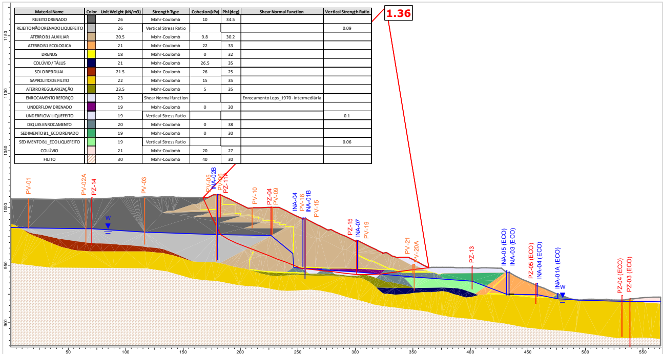
Figura 5.124 – Seção C-C' – Análise Não Drenada – Superfície de ruptura plano-circular otimizada – Freática 30/04/2024 – Razão de resistência não drenada liquefeita.
