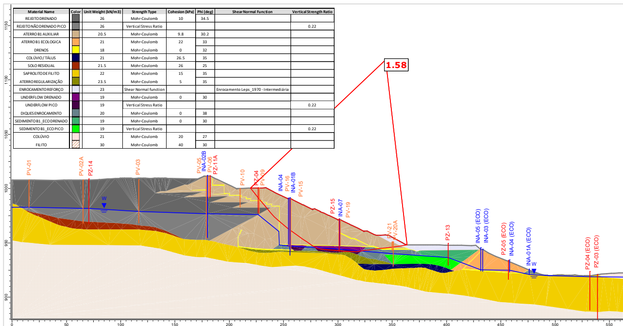
Figura 5.123 – Seção C-C' – Análise Não Drenada – Superfície de ruptura plano-circular otimizada – Freática 30/04/2024 – Razão de resistência não drenada de pico.
