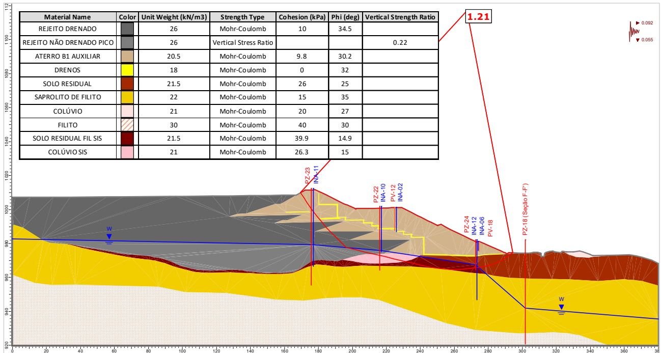
Figura 5.140 – Seção E-E' – Análise Não Drenada – Superfície de ruptura plano-circular otimizada – Freática 30/04/2024 – Razão de resistência não drenada de pico + sismo ↓ (critério CDA).
