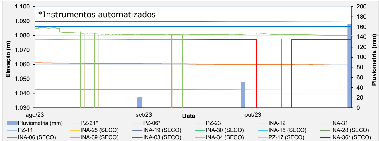
Figura 6.9 – Leituras dos instrumentos da seção de controle A-A'.
