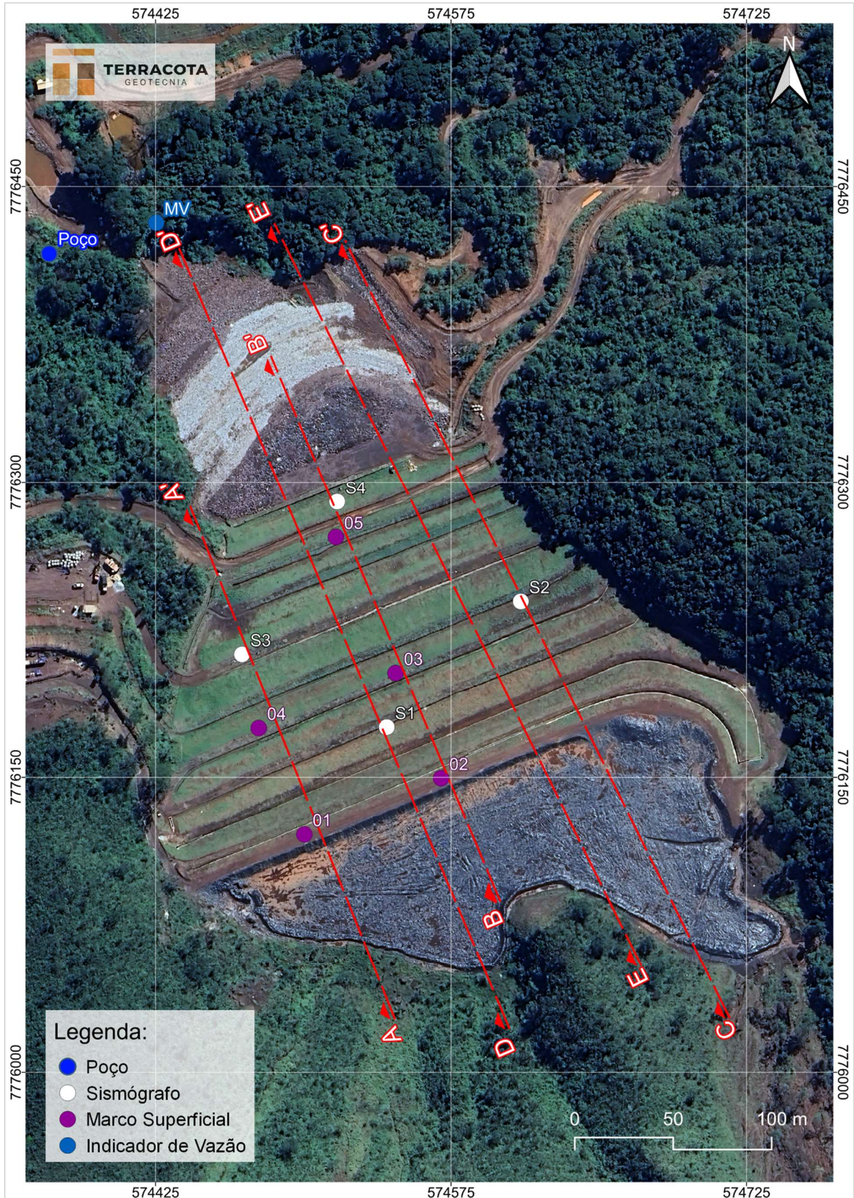
Figura 6.3 – Localização dos Marcos Superficiais, Sismógrafos e Indicador de Vazão.
