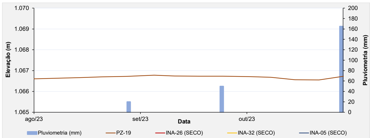
Figura 6.11 – Leituras dos instrumentos da seção de controle C-C'.
