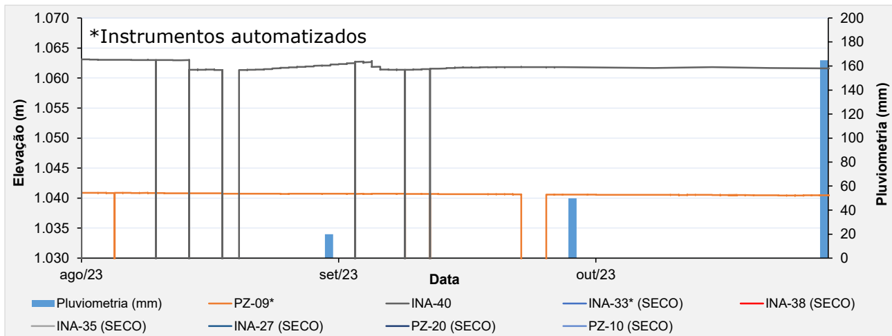
Figura 6.13 – Leituras dos instrumentos da seção de controle E-E'
