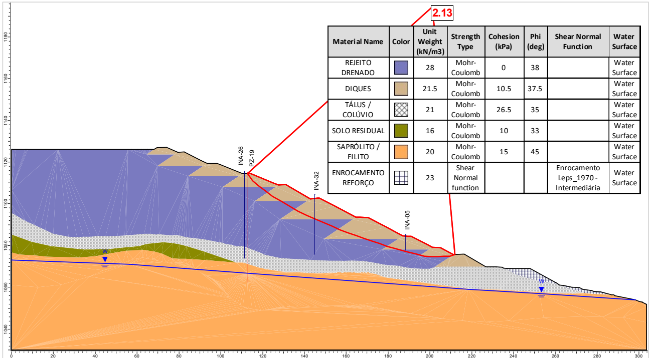
Figura 6.26 – Seção C-C’ – Análise Drenada – Superfície de ruptura plano-circular otimizada – Freática atual (31/10/2023).
