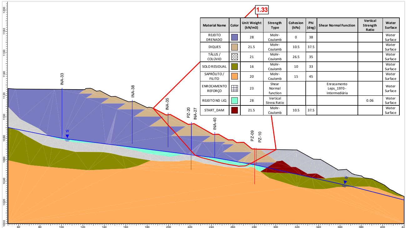
Figura 6.32 – Seção E-E' – Análise Não Drenada – Superfície de ruptura plano-circular otimizada – Freática atual (31/10/2023) – Razão de resistência não drenada liquefeita.
