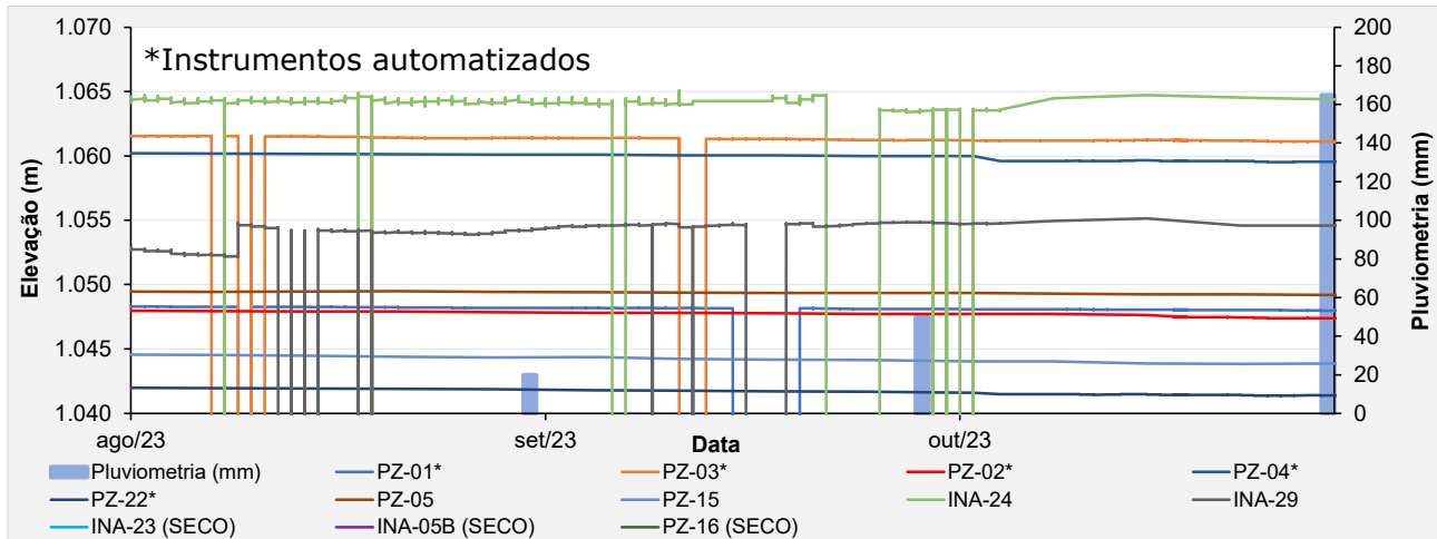
Figura 6.12 – Leituras dos instrumentos da seção de controle D-D'.
