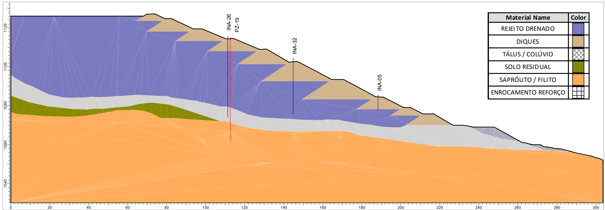
Figura 6.6 – Seção transversal de controle C-C'.
