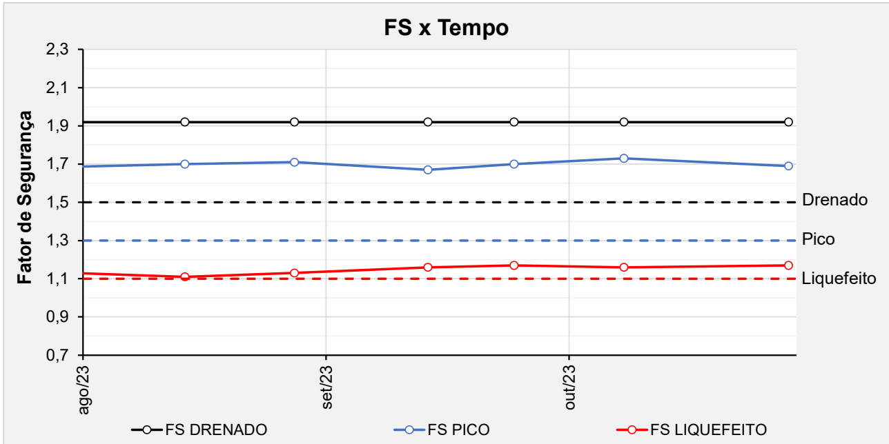
Figura 6.18 – Seção D-D' - Histórico dos F.S. obtidos nas análises de estabilidade no período avaliado.
