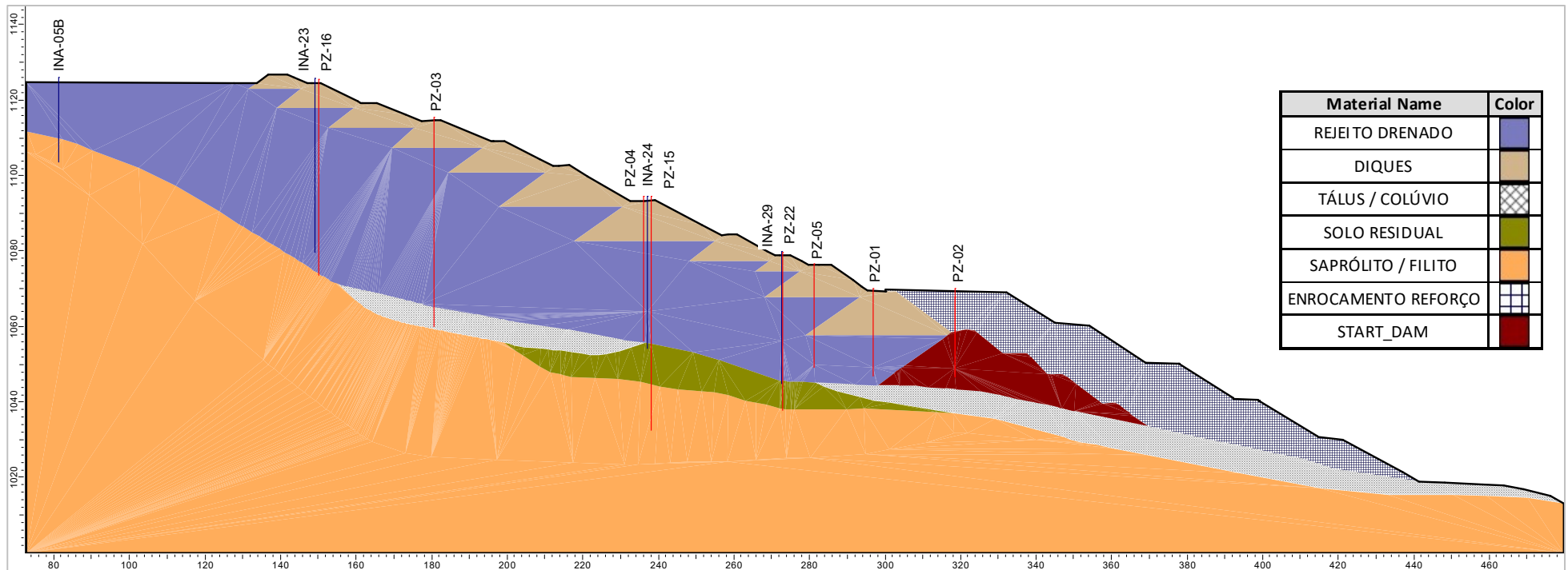
Figura 6.7 – Seção transversal de controle D-D'.
