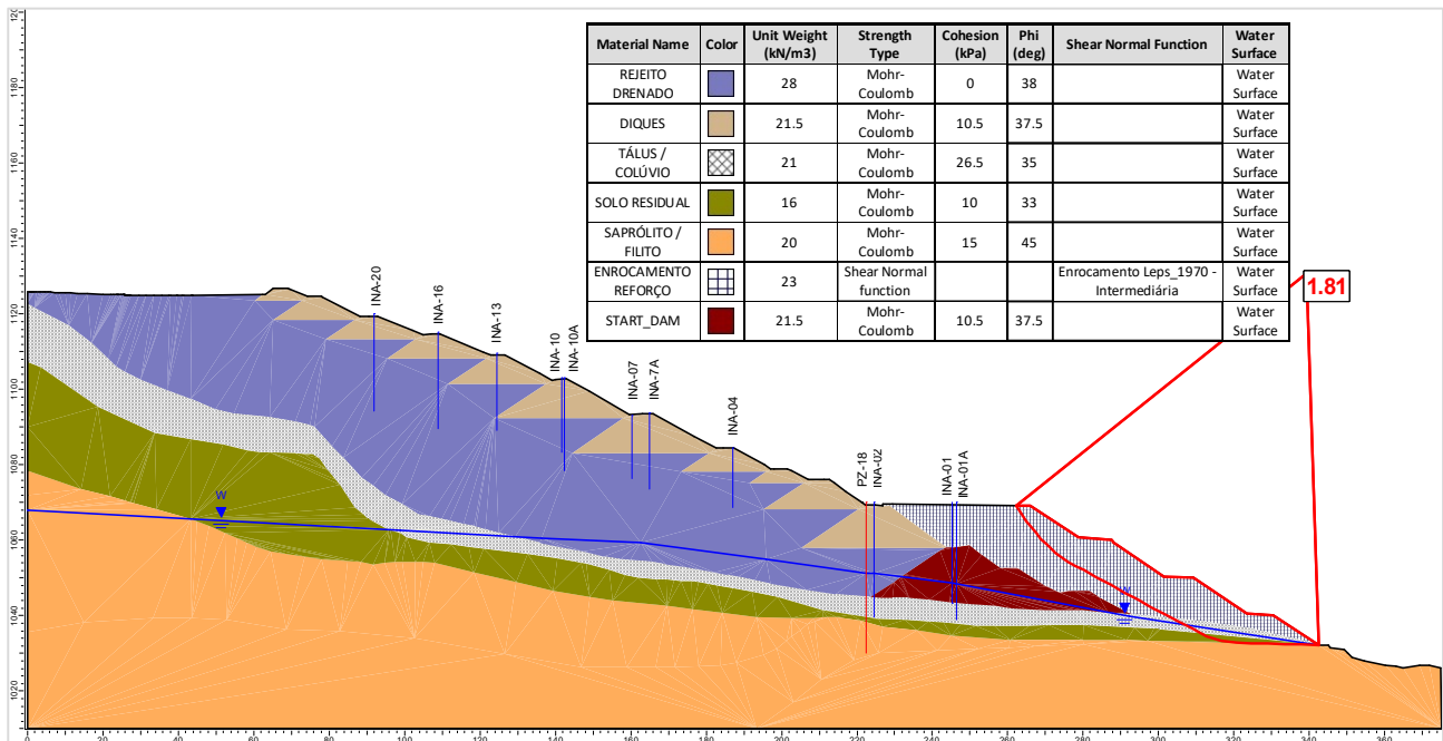
Figura 6.23 – Seção B-B' – Análise Drenada – Superfície de ruptura plano-circular otimizada – Freática atual (31/10/2023).
