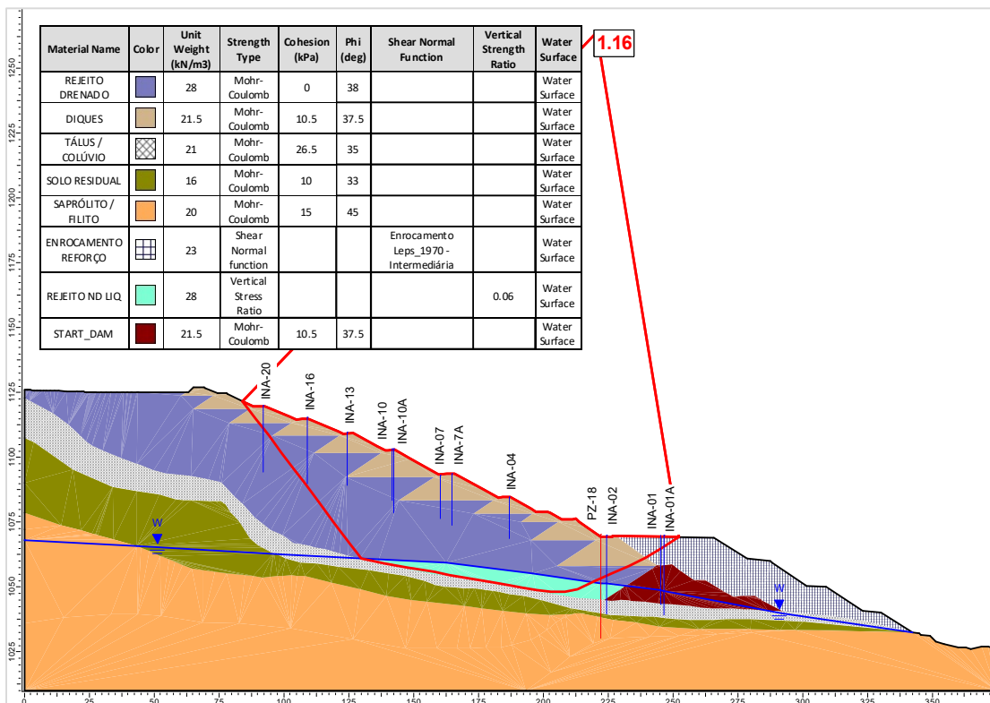
Figura 6.25 – Seção B-B' – Análise Não Drenada – Superfície de ruptura plano-circular otimizada – Freática atual (31/10/2023) – Razão de resistência não drenada liquefeita.
