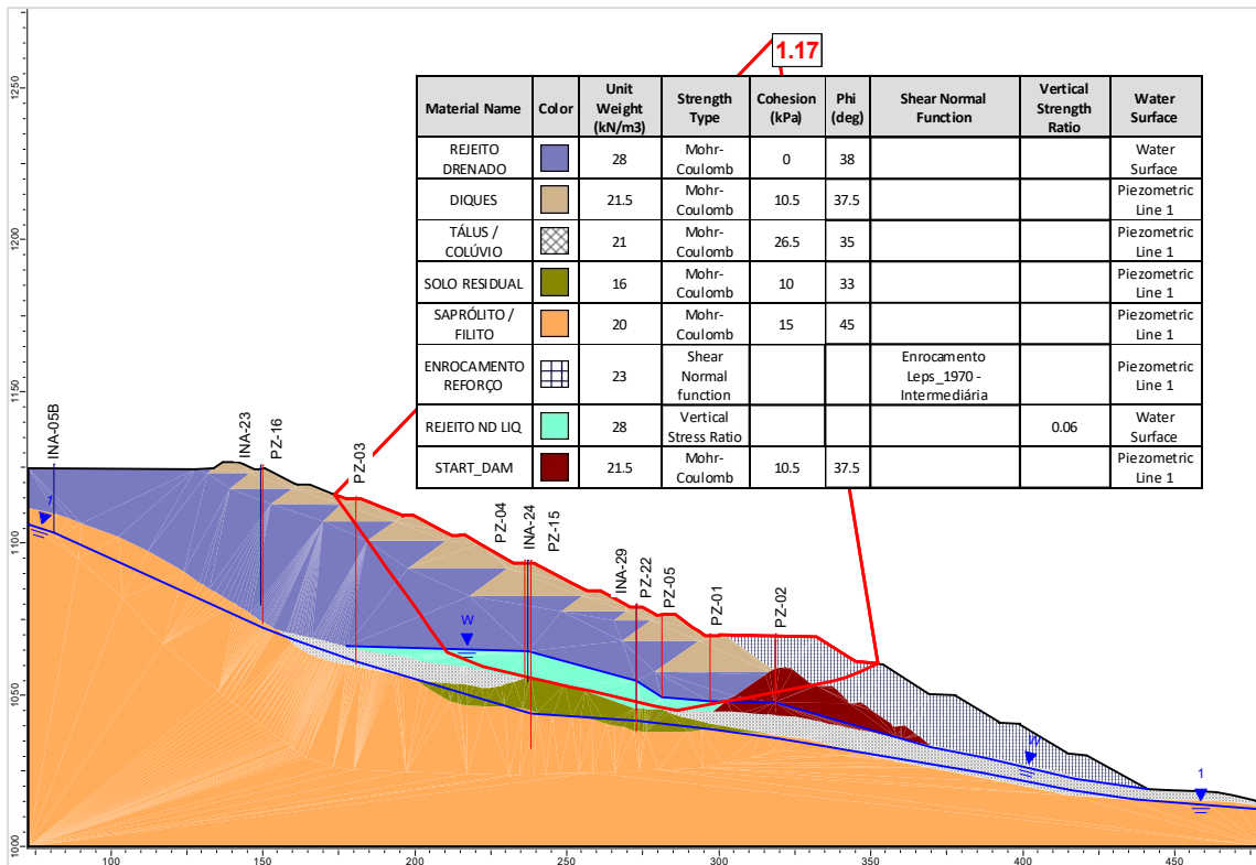
Figura 6.29 – Seção D-D' – Análise Não Drenada – Superfície de ruptura plano-circular otimizada – Freática atual (31/10/2023) – Razão de resistência não drenada liquefeita.
