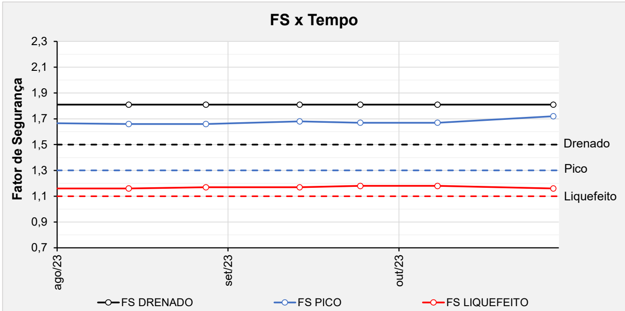
Figura 6.16 – Seção B-B' - Histórico dos F.S. obtidos nas análises de estabilidade no período avaliado.
