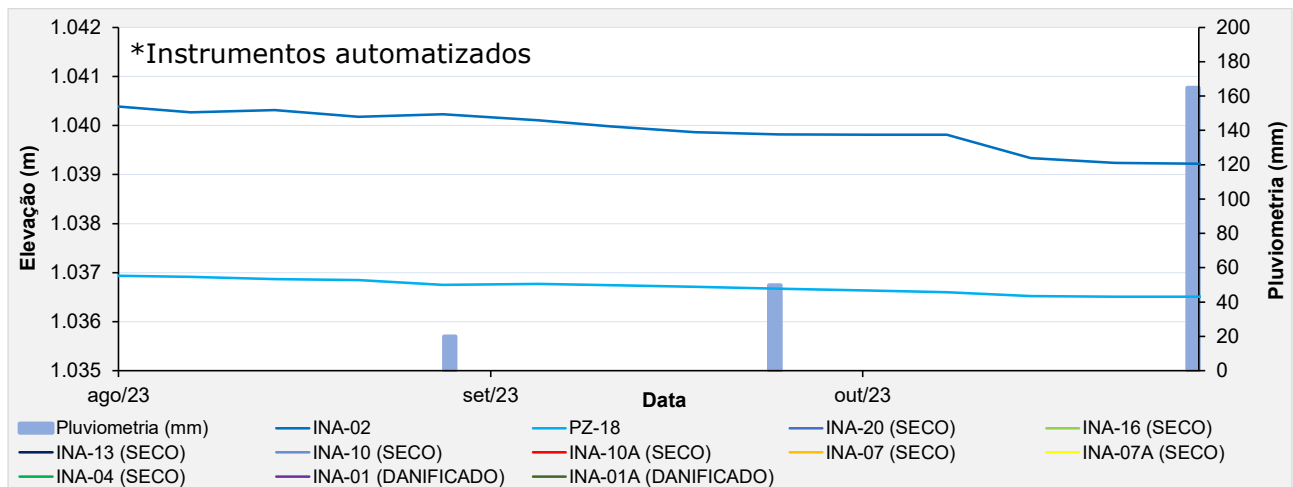
Figura 6.10 – Leituras dos instrumentos da seção de controle B-B'.
