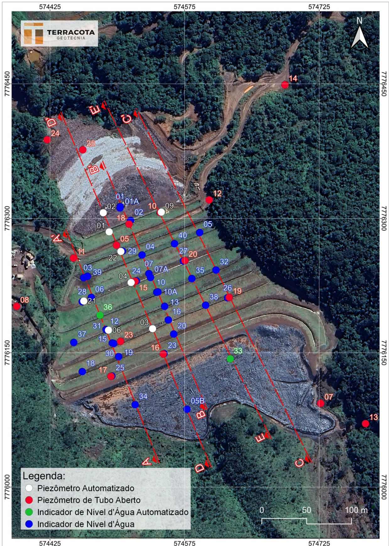
Figura 6.14 – Seções Instrumentadas Barragem B2 – Mina Tico-Tico- Planta.
