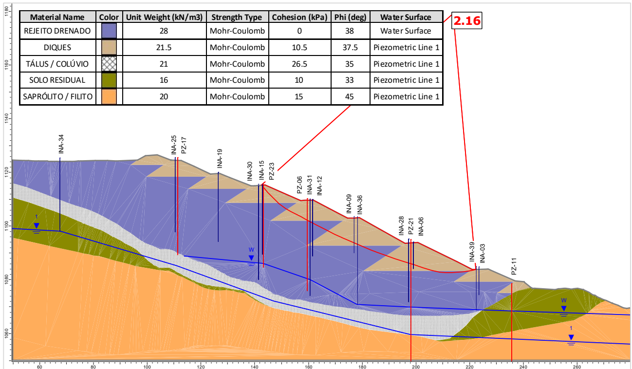
Figura 6.20 – Seção A-A' – Análise Drenada – Superfície de ruptura plano-circular otimizada – Freática atual (31/10/2023).
