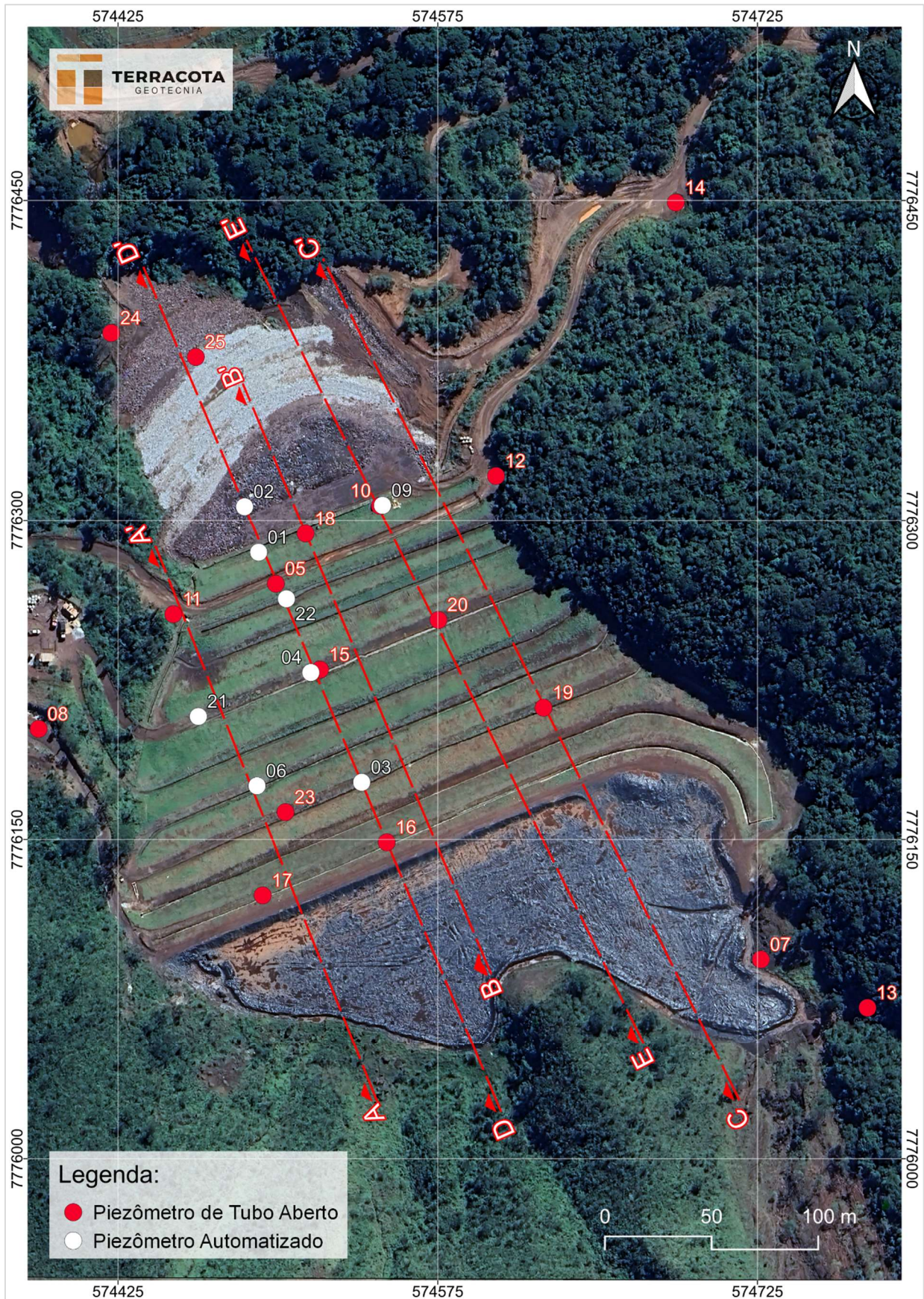
Figura 6.2 – Localização dos Piezômetros.
