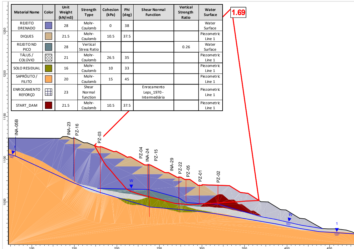
Figura 6.28 – Seção D-D' – Análise Não Drenada – Superfície de ruptura plano-circular otimizada – Freática atual (31/10/2023) – Razão de resistência não drenada de pico.
