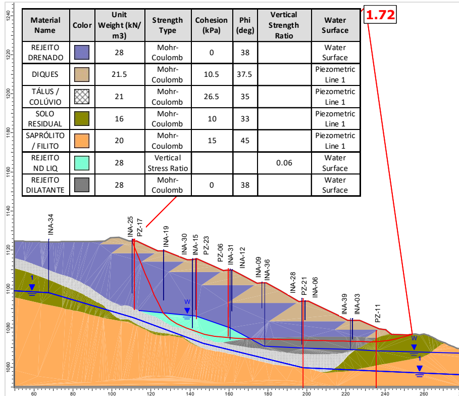
Figura 6.22 – Seção A-A' – Análise Não Drenada – Superfície de ruptura plano-circular otimizada – Freática atual (31/10/2023) – Razão de resistência não drenada liquefeita.
