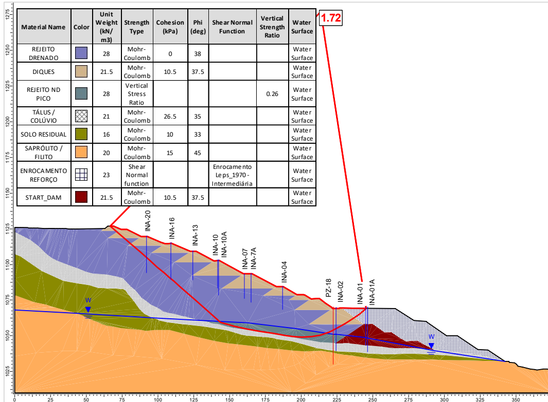
Figura 6.24 – Seção B-B' – Análise Não Drenada – Superfície de ruptura plano-circular otimizada – Freática atual (31/10/2023) – Razão de resistência não drenada de pico.
