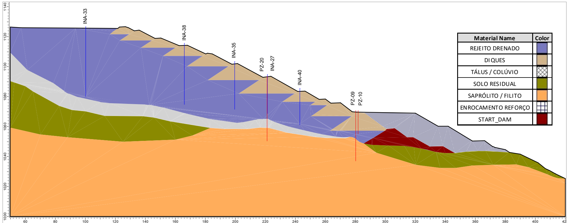
Figura 6.8 – Seção transversal de controle E-E'.
