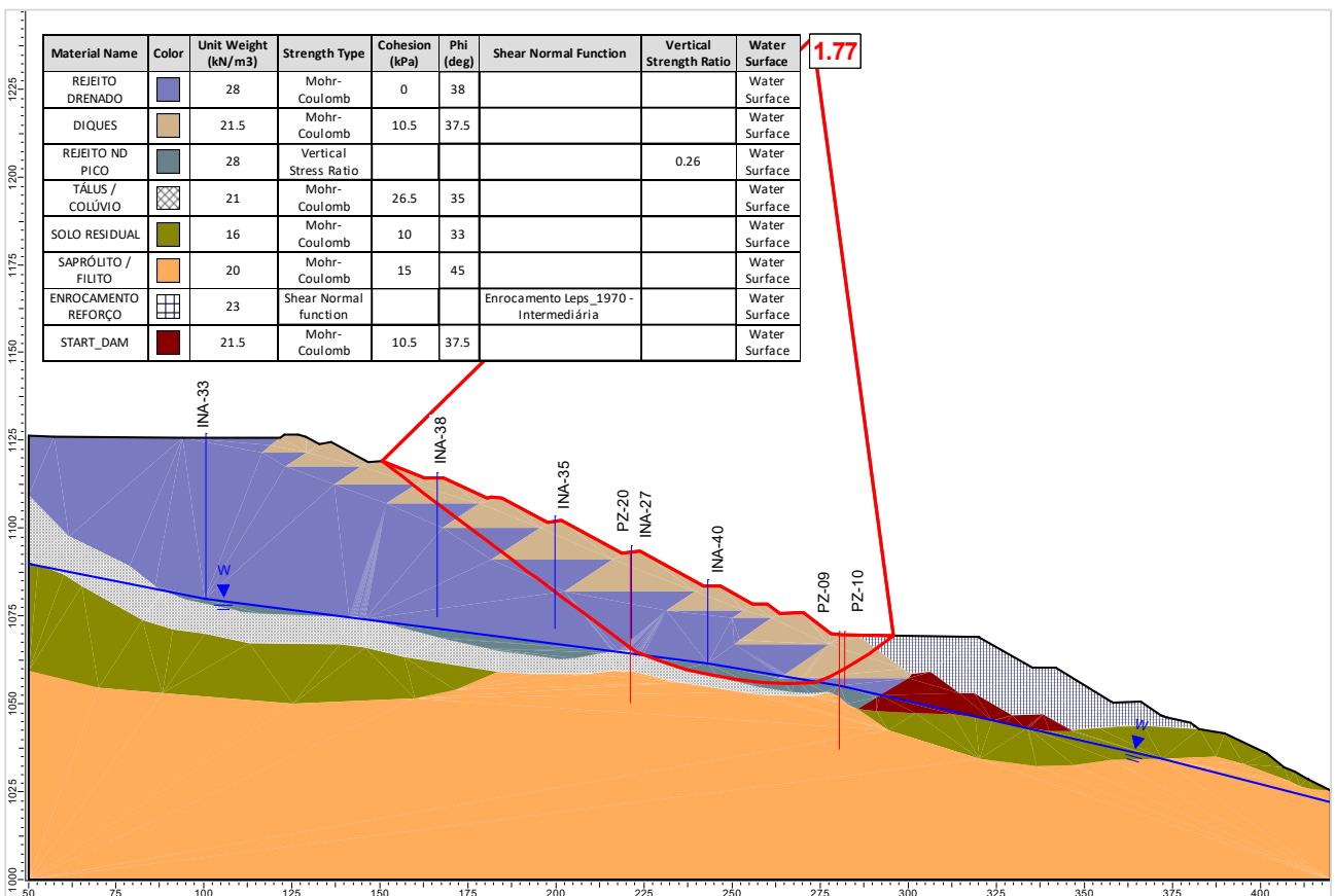
Figura 6.31 – Seção E-E' – Análise Não Drenada – Superfície de ruptura plano-circular otimizada – Freática atual (31/10/2023) – Razão de resistência não drenada de pico.
