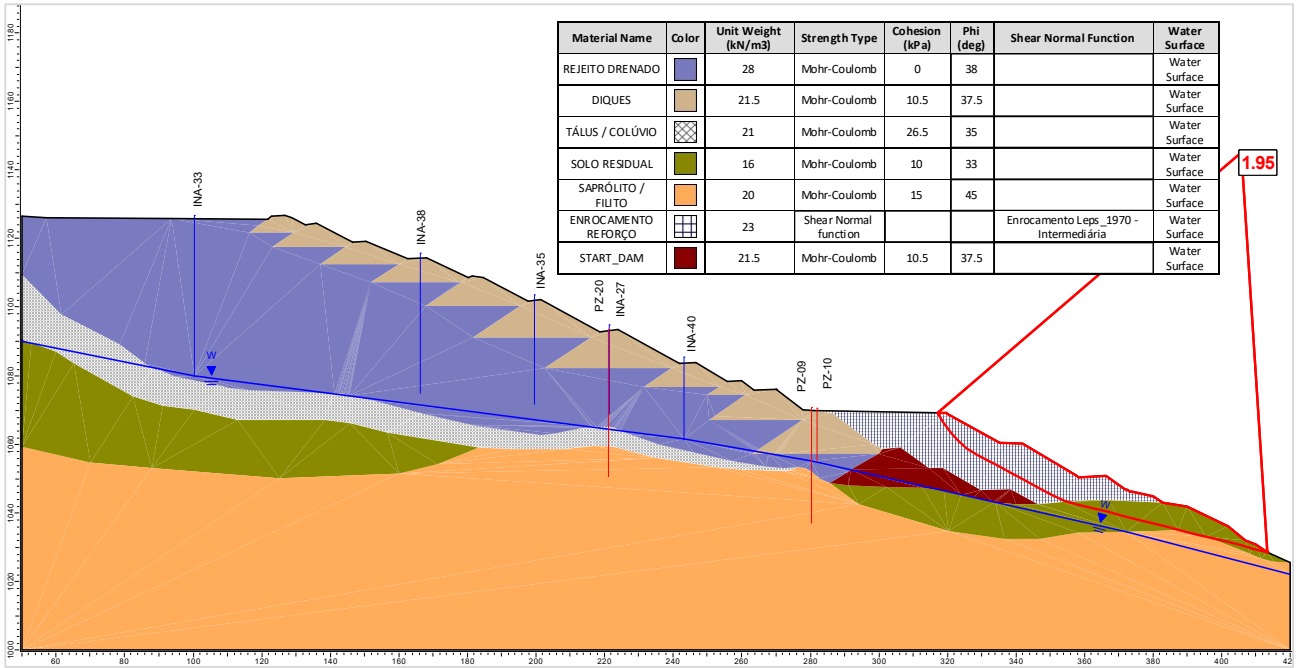
Figura 6.30 – Seção E-E' – Análise Drenada – Superfície de ruptura plano-circular otimizada – Freática atual (31/10/2023).
