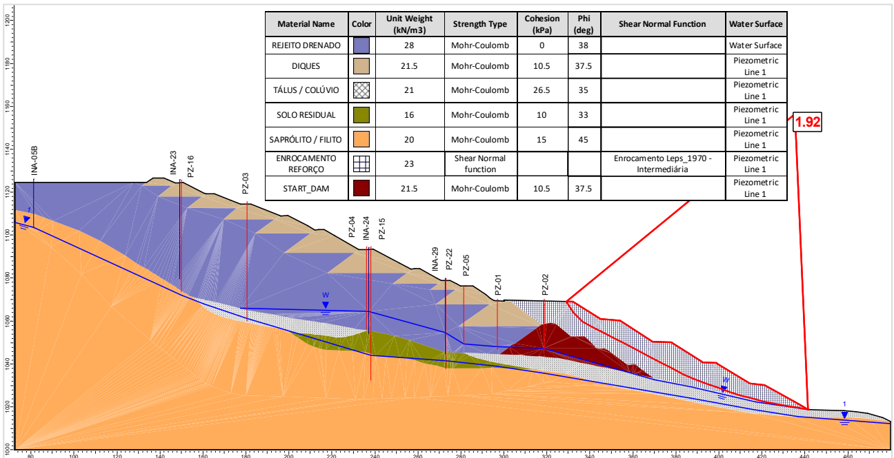
Figura 6.27 – Seção D-D’ – Análise Drenada – Superfície de ruptura plano-circular otimizada – Freática atual (31/10/2023).
