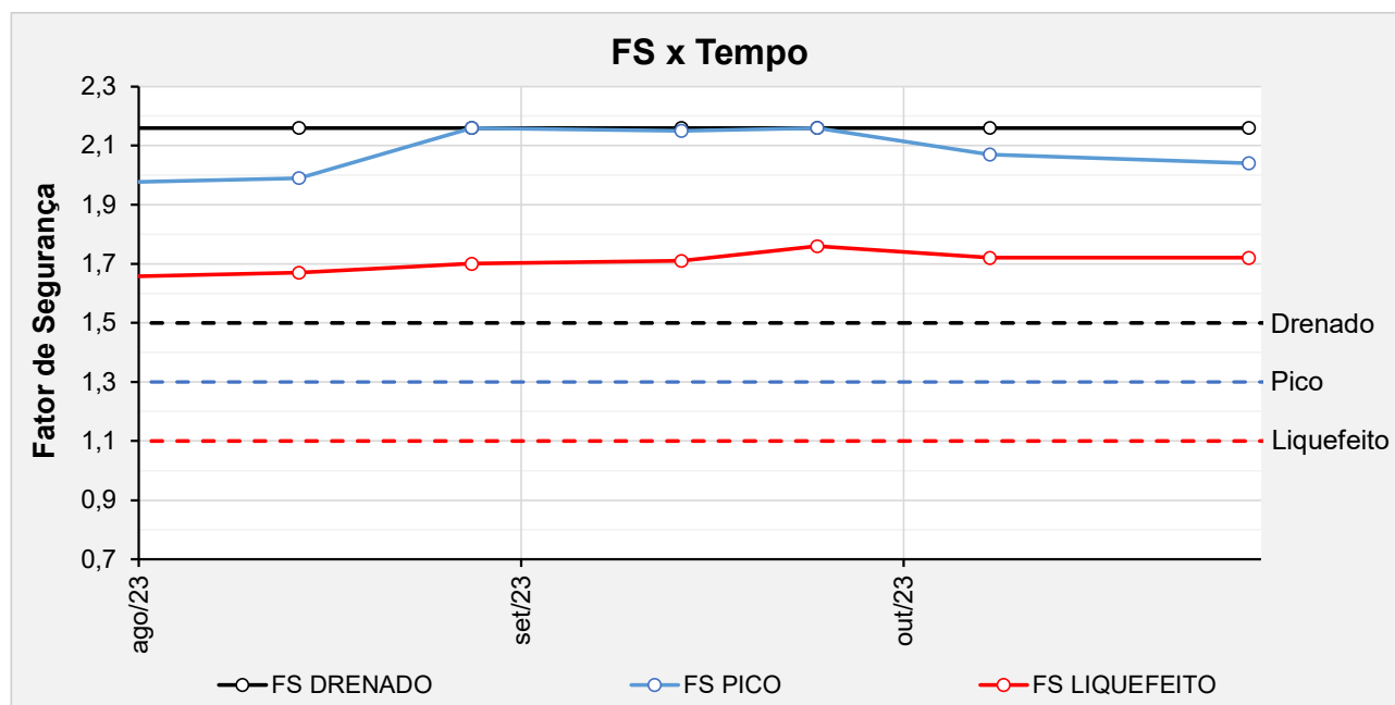
Figura 6.15 – Seção A-A' - Histórico dos F.S. obtidos nas análises de estabilidade no período avaliado.
