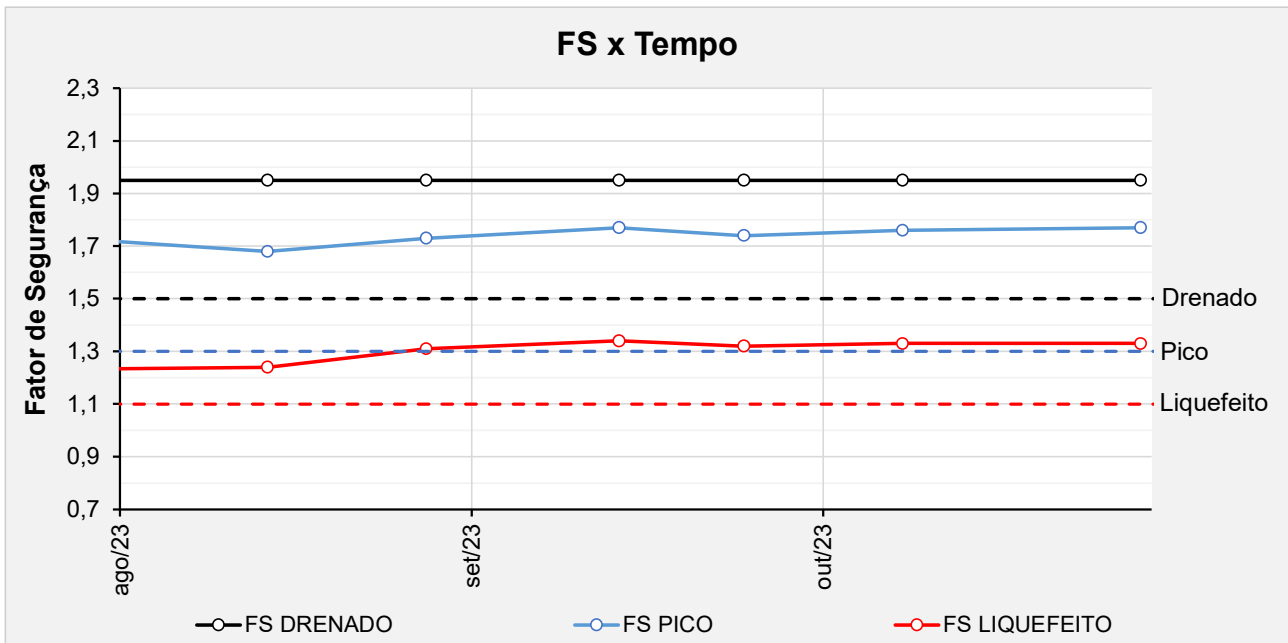
Figura 6.19 – Seção E-E' - Histórico dos F.S. obtidos nas análises de estabilidade no período avaliado.
