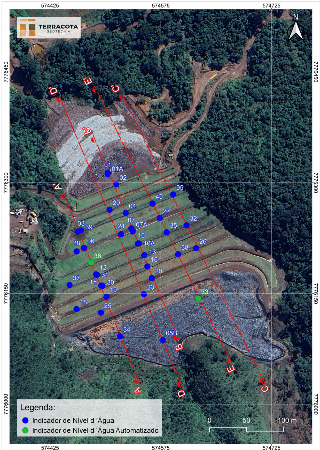
Figura 6.1 – Localização dos Indicadores de Nível d'Água.
