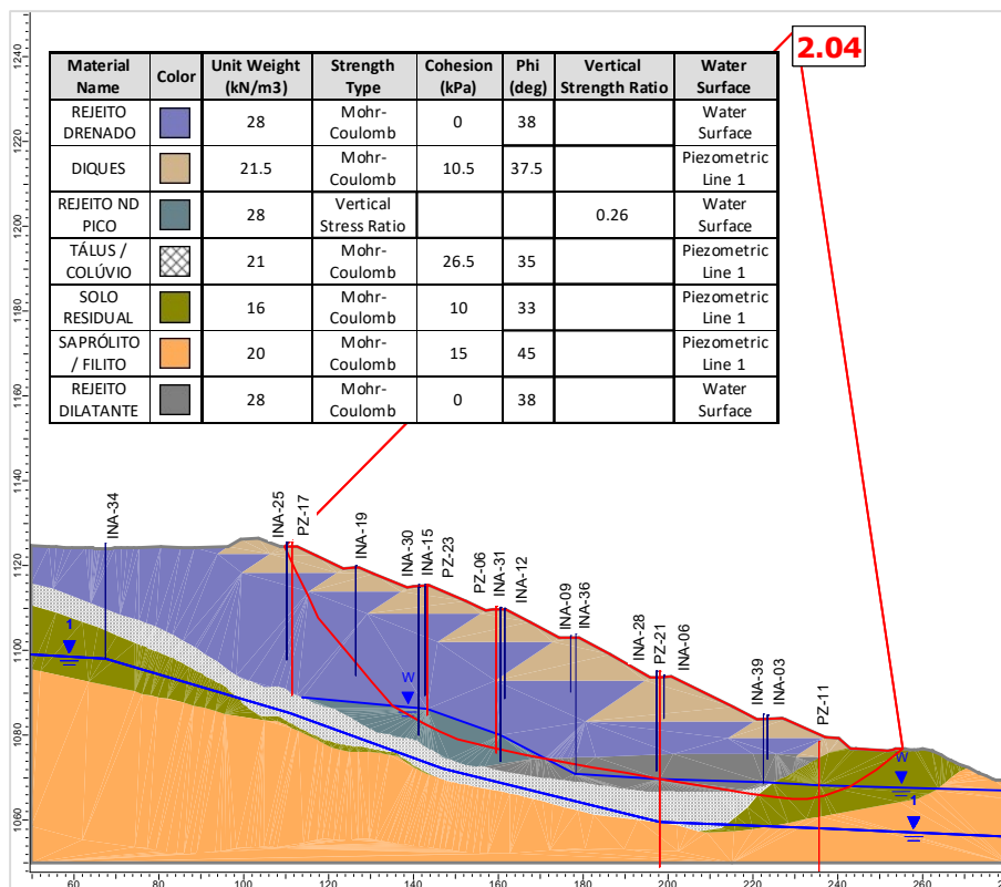
Figura 6.21 – Seção A-A' – Análise Não Drenada – Superfície de ruptura plano-circular otimizada – Freática atual (31/10/2023) – Razão de resistência não drenada de pico.
