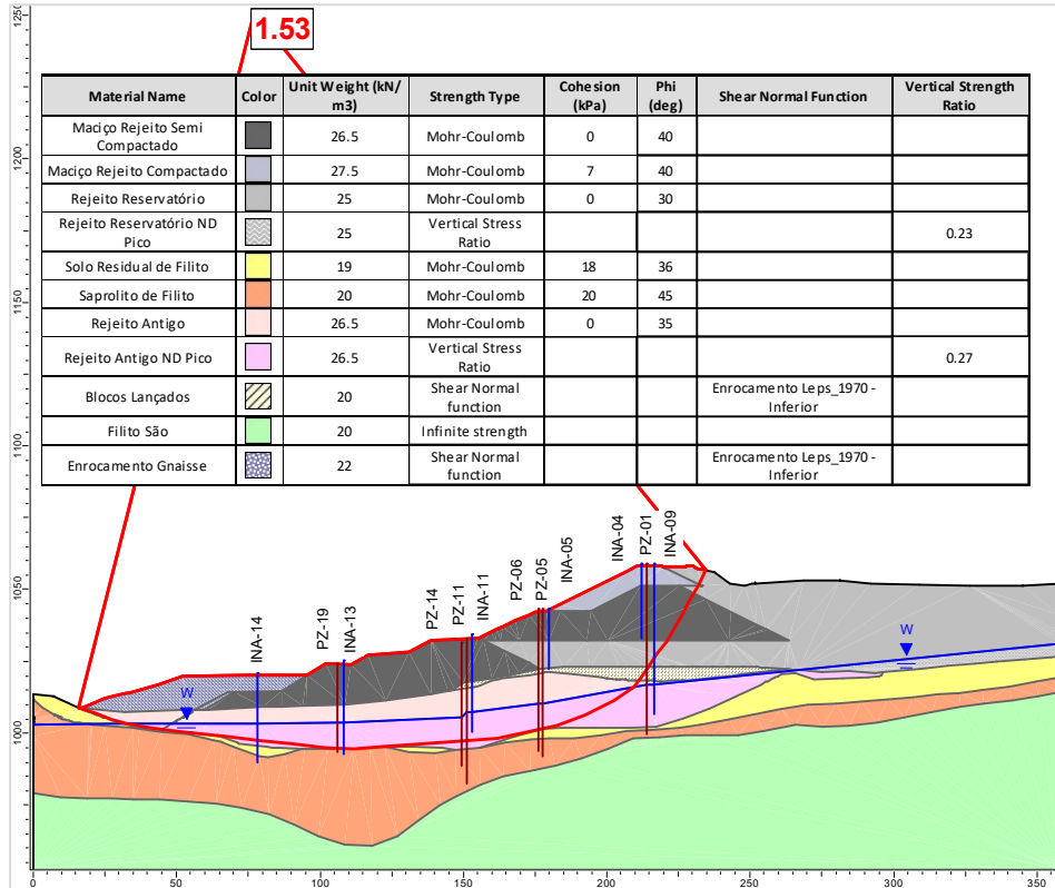
Figura 5.103 – Seção B-B' – Análise Não Drenada – Superfície de ruptura plano-circular otimizada – Freática atual 30/10/2024 – Razão de resistência não drenada de pico.
