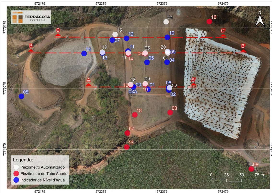
Figura 5.92 – Seções Instrumentadas Barragem B1 – Mina Ipê – Planta.
