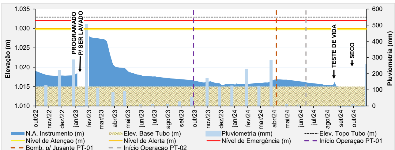
Figura 5.20 - Desempenho do indicador de nível d'água - INA-03A.
