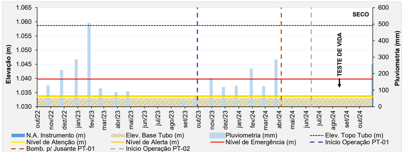
Figura 5.21 - Desempenho do indicador de nível d'água - INA-04.
