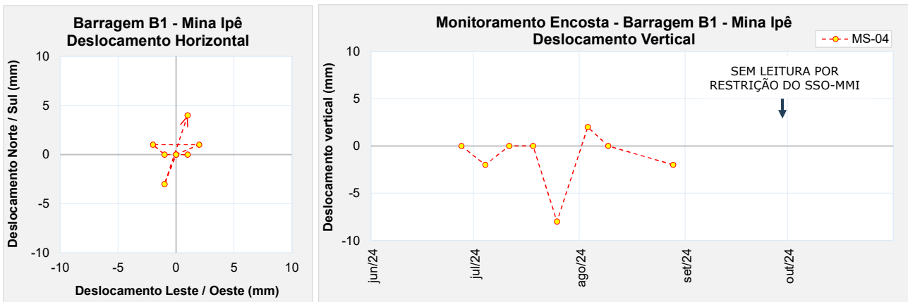
Figura 5.67 – Marco de controle de monitoramento da encosta MS-04.
