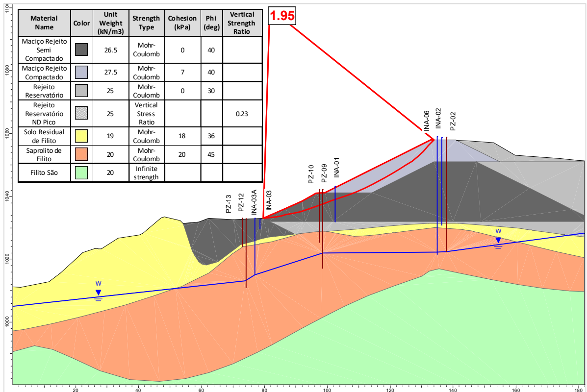
Figura 5.96 – Seção A-A' – Análise Não Drenada – Superfície de ruptura plano-circular otimizada – Freática 30/10/2024 – Razão de resistência não drenada de pico.
