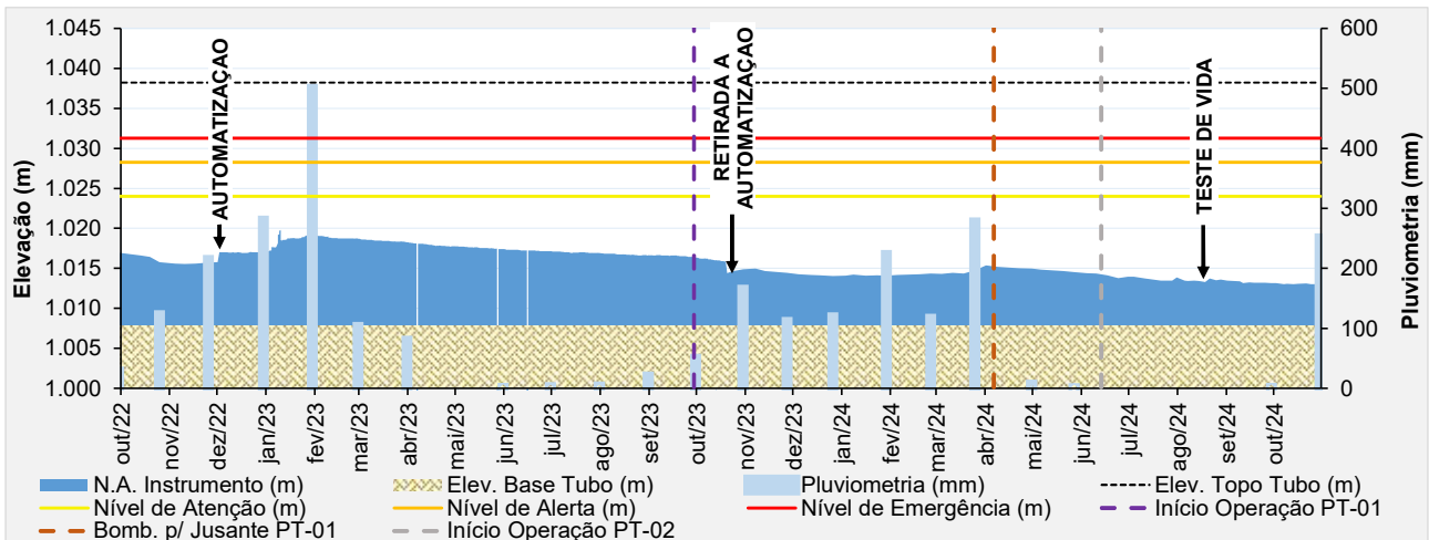
Figura 5.49 - Desempenho do piezômetro de tubo aberto - PZ-18.
