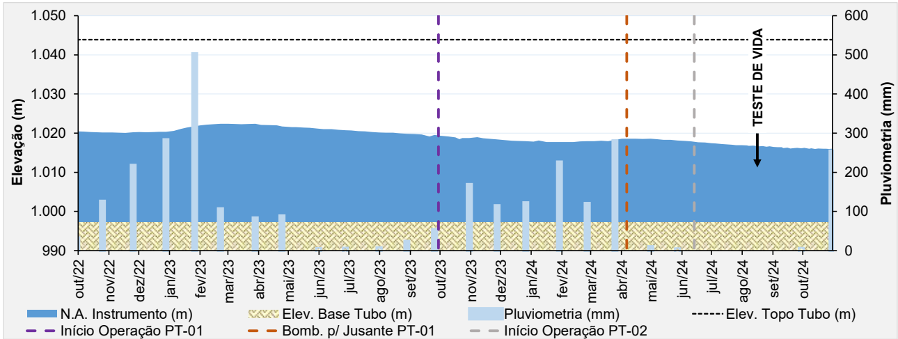
Figura 5.48 - Desempenho do piezômetro de tubo aberto - PZ-17.
