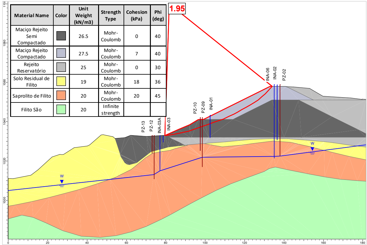
Figura 5.95 – Seção A-A' – Análise Drenada – Superfície de ruptura plano-circular otimizada – Freática 30/10/2024.
