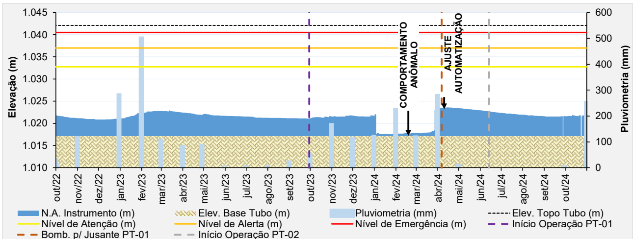
Figura 5.40 - Desempenho do piezômetro automatizado - PZ-09.
