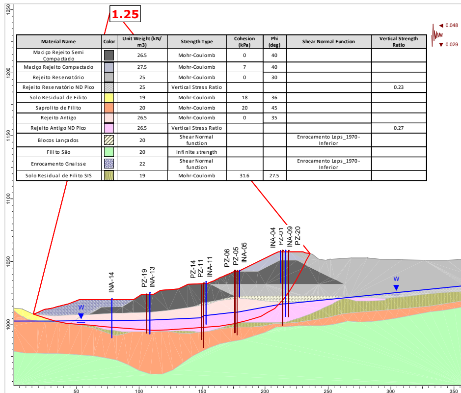
Figura 5.108 – Seção B-B' – Análise Não Drenada – Superfície de ruptura plano-circular otimizada – Freática 30/10/2024 – Razão de resistência não drenada de pico + sismo ↓ (critério vida útil).
