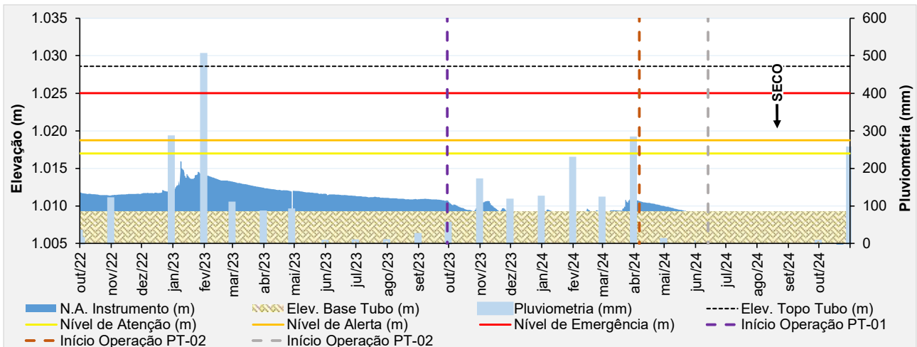
Figura 5.46 – Desempenho do piezômetro automatizado – PZ-15.
