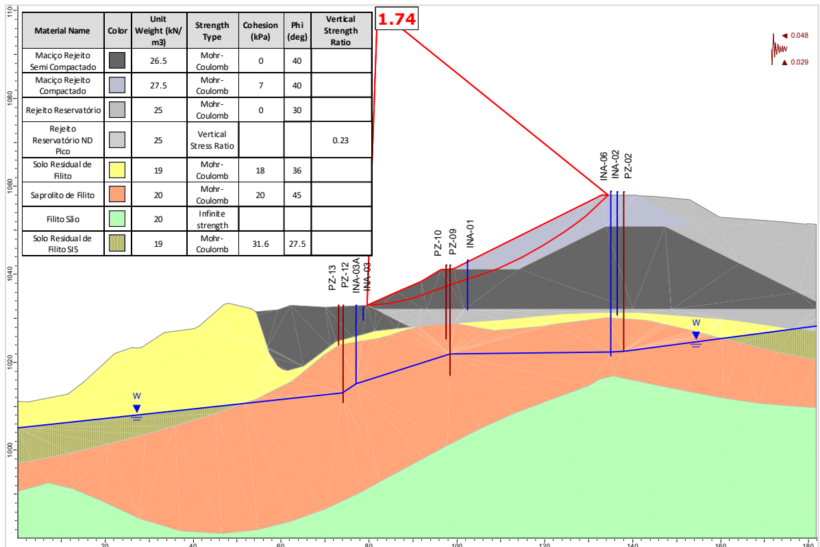
Figura 5.100 – Seção A-A' – Análise Não Drenada – Superfície de ruptura plano-circular otimizada – Freática 30/10/2024 – Razão de resistência não drenada de pico + sismo ↑ (critério vida útil).
