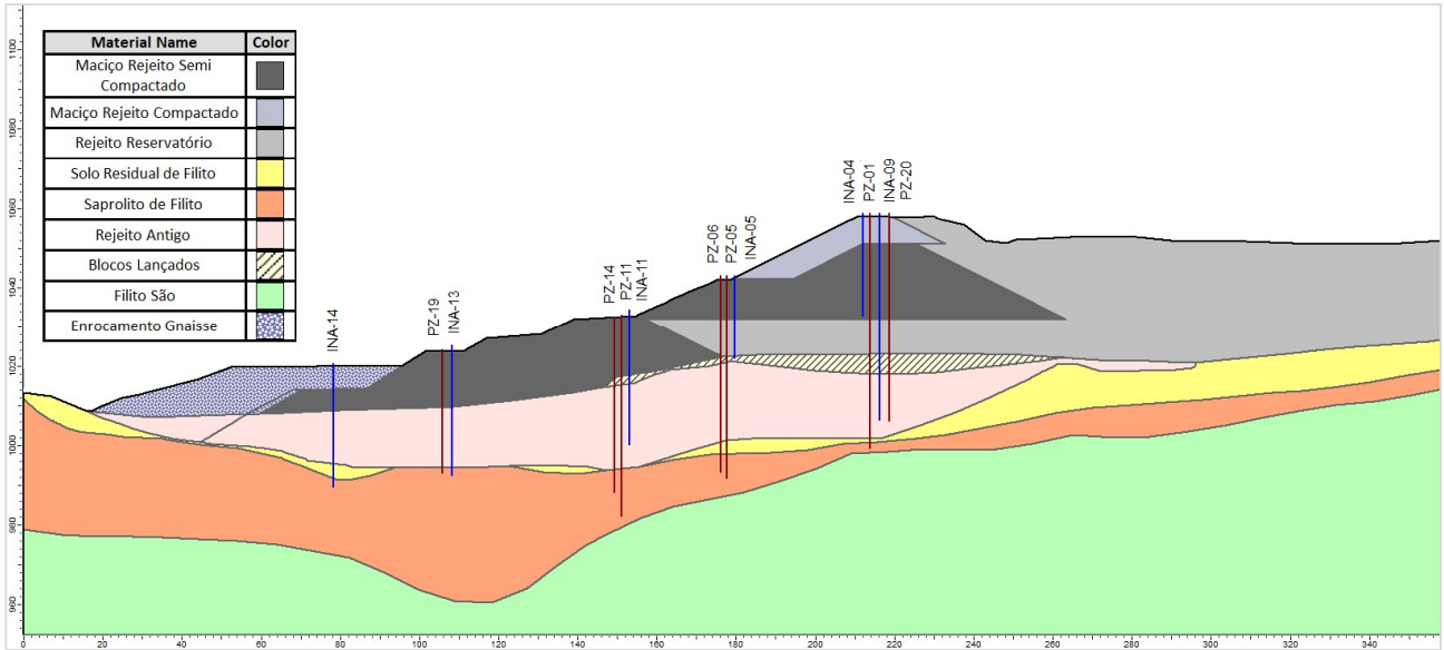
Figura 5.15 – Seção transversal de controle B-B'.
