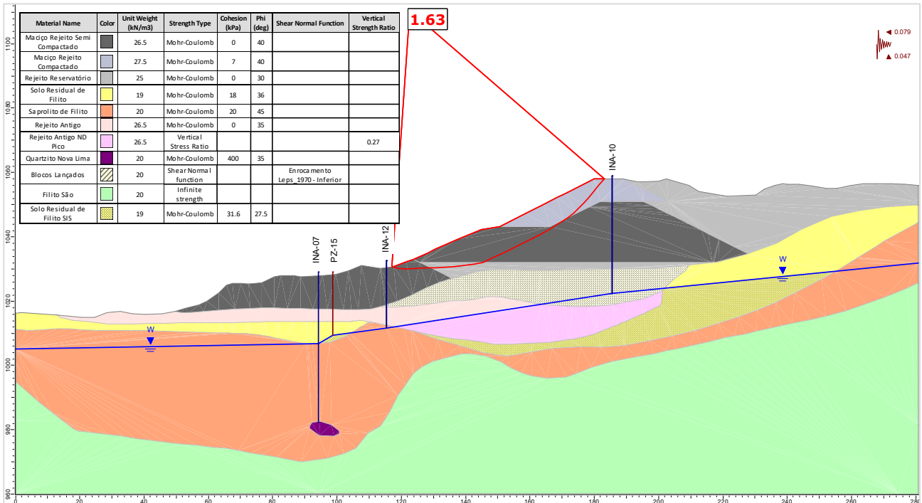
Figura 5.112 – Seção C-C' – Análise Não Drenada – Superfície de ruptura plano-circular otimizada – Freática 30/10/2024 – Razão de resistência não drenada de pico + sismo ↑ (critério CDA).
