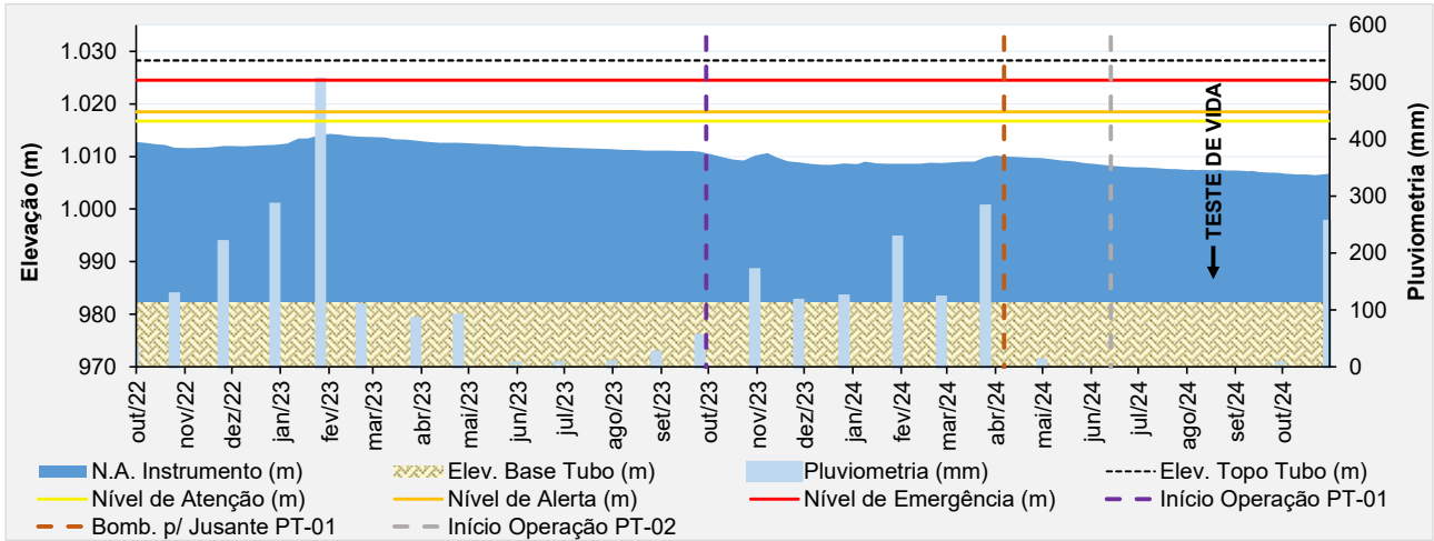
Figura 5.24 – Desempenho do indicador de nível d'água – INA-07.
