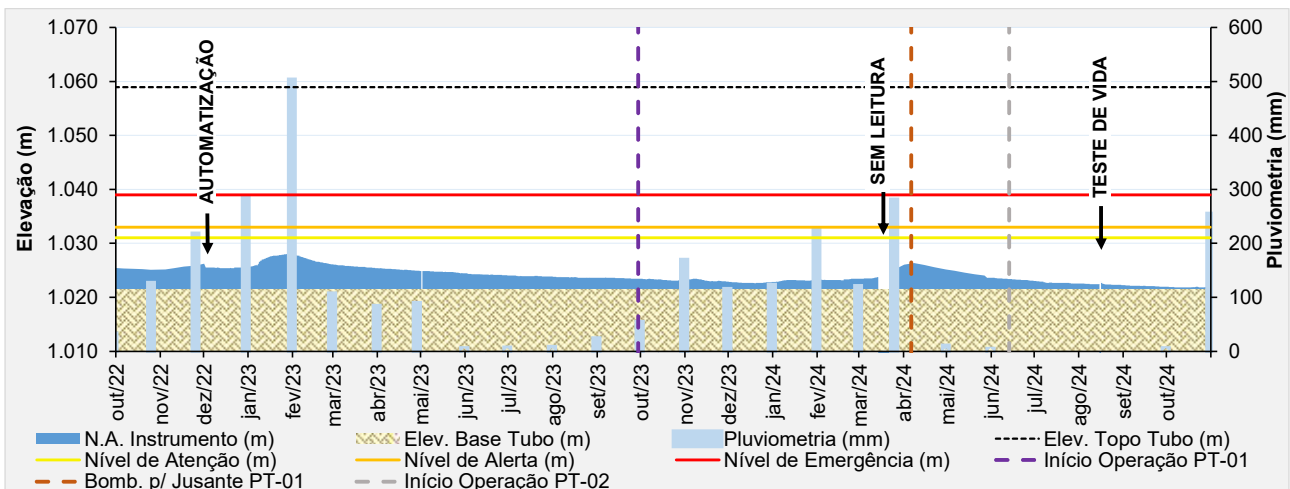
Figura 5.35 - Desempenho do piezômetro automatizado - PZ-04.
