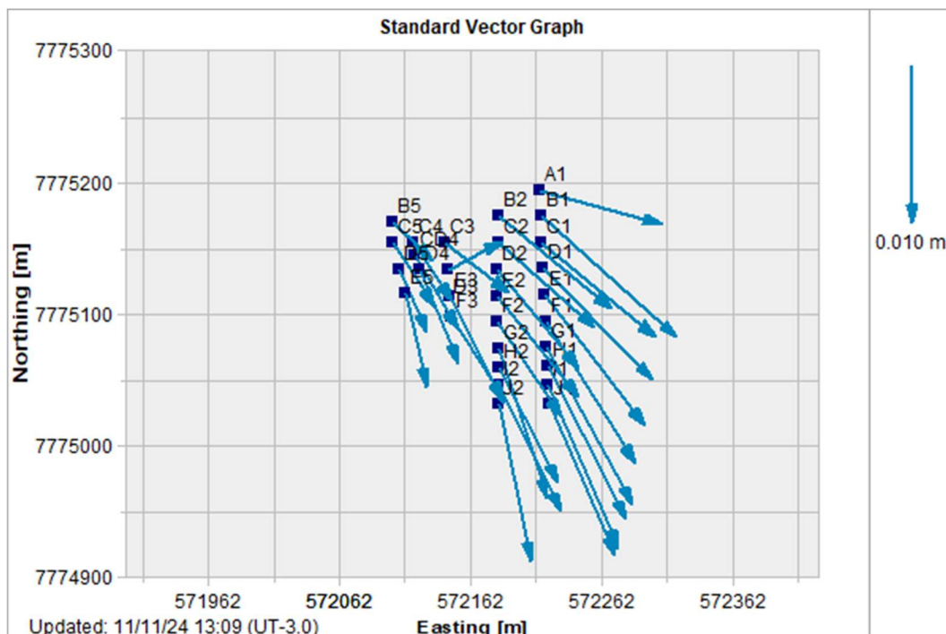
Figura 5.55 – Registros vetores deslocamento dos prismas.
