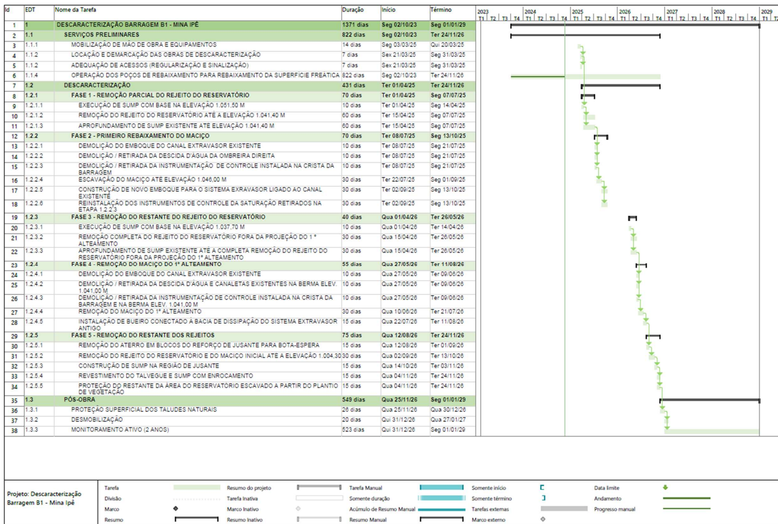
Figura 5.10 – Cronograma preliminar das obras de descaracterização.
