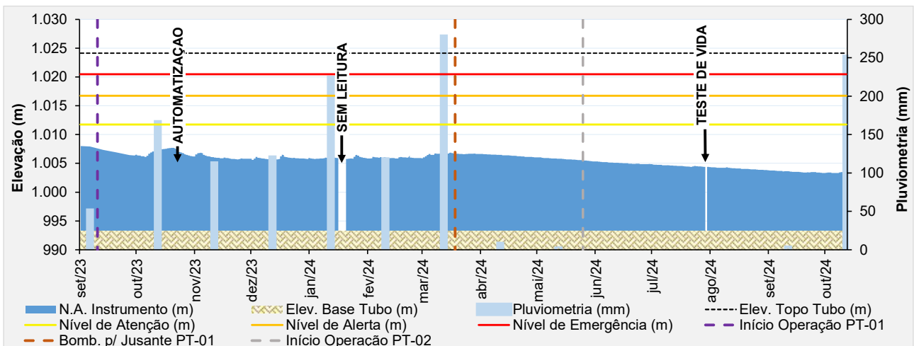
Figura 5.50 - Desempenho do piezômetro automatizado - PZ-19.
