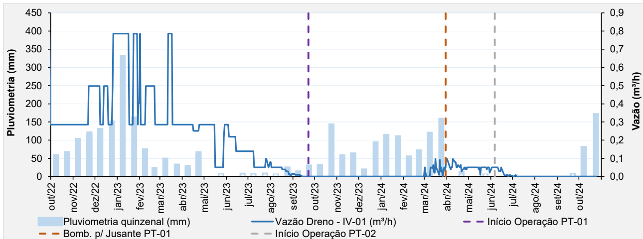
Figura 5.52 – Análise das vazões do IV-01 (Dreno).
