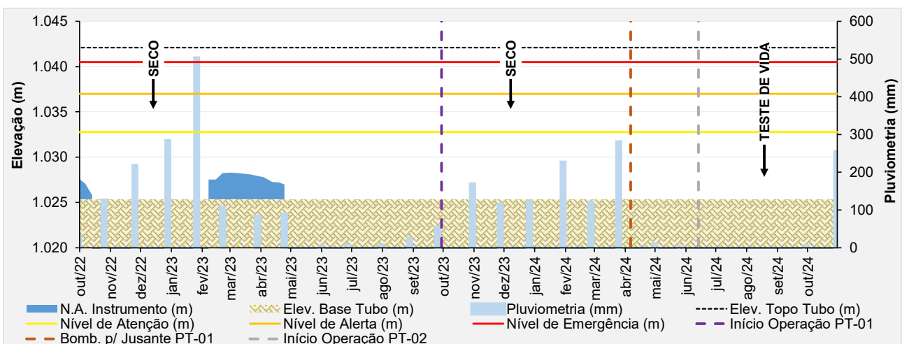
Figura 5.41 - Desempenho do piezômetro de tubo aberto - PZ-10.
