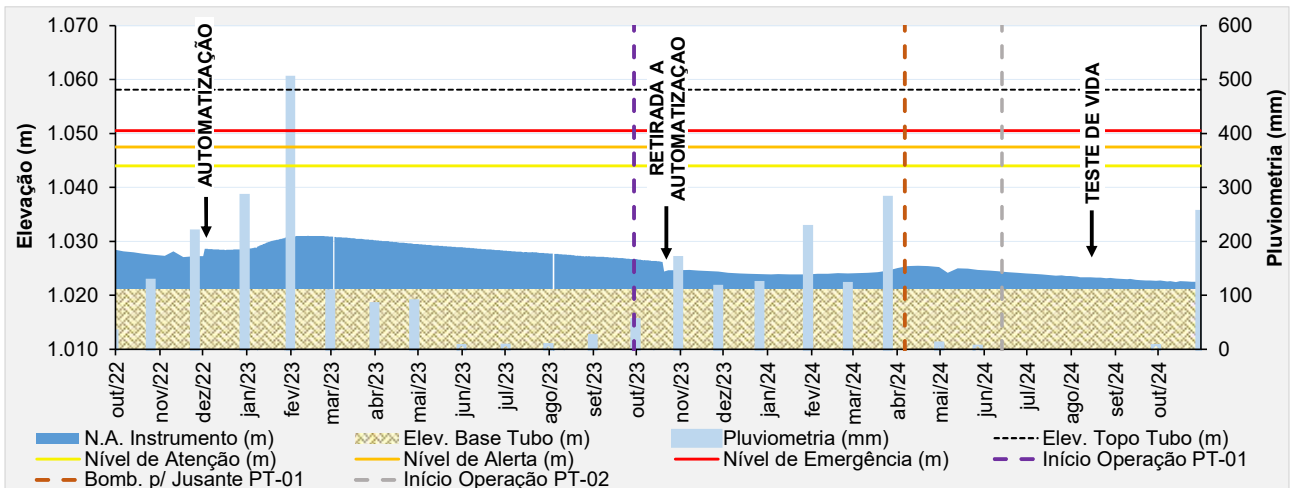
Figura 5.34 - Desempenho do piezômetro de tubo aberto - PZ-03.
