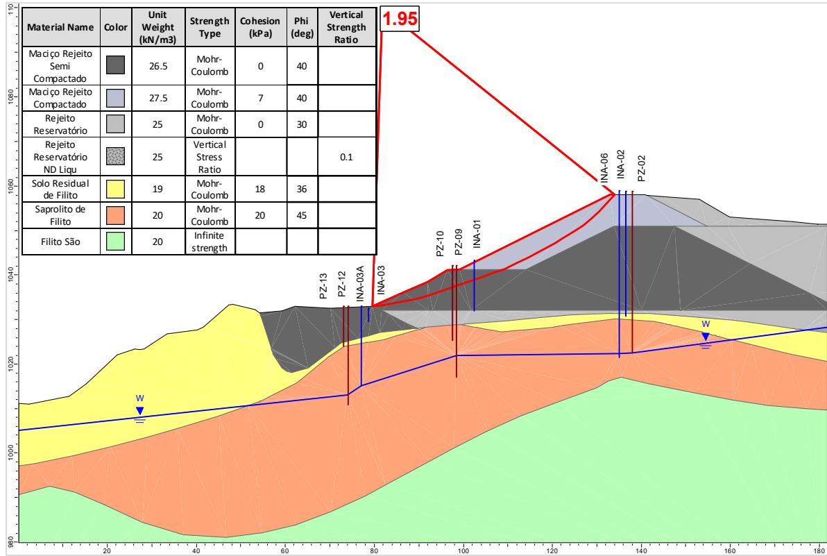
Figura 5.97 – Seção A-A' – Análise Não Drenada – Superfície de ruptura plano-circular otimizada – Freática 30/10/2024 – Razão de resistência não drenada liquefeito.
