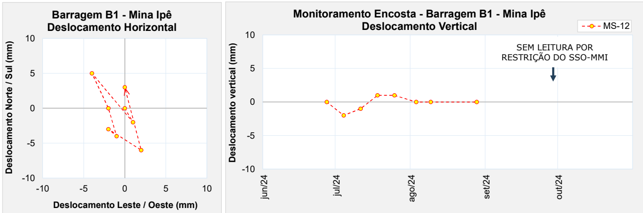
Figura 5.75 – Marco de controle de monitoramento da encosta MS-12.
