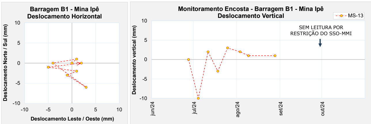
Figura 5.76 – Marco de controle de monitoramento da encosta MS-13.
