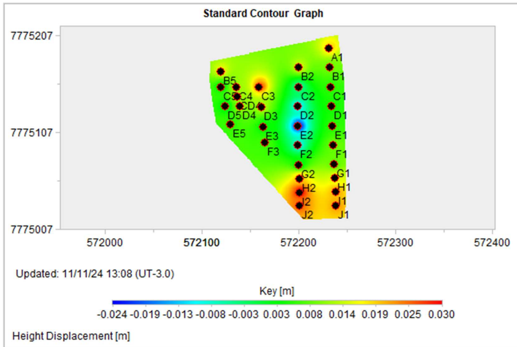
Figura 5.54 – Registros deslocamentos verticais dos prismas.
