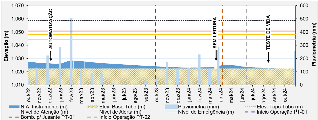
Figura 5.33 - Desempenho do piezômetro automatizado - PZ-02.
