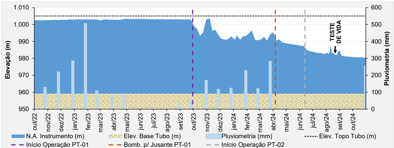
Figura 5.25 – Desempenho do indicador de nível d'água – INA-08.
