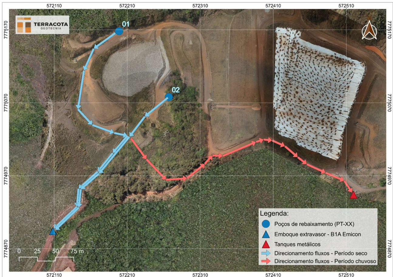
Figura 5.90 – Esquema de direcionamento dos fluxos proveniente dos poços de bombeamento.
