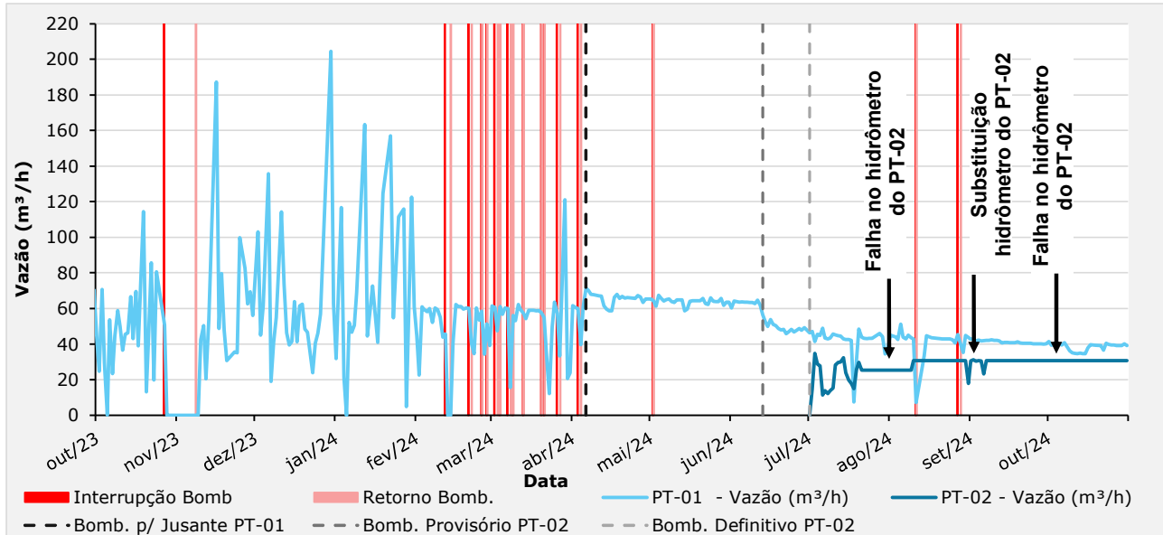
Figura 5.91 – Histórico bombeamento dos poços de rebaixamento.
