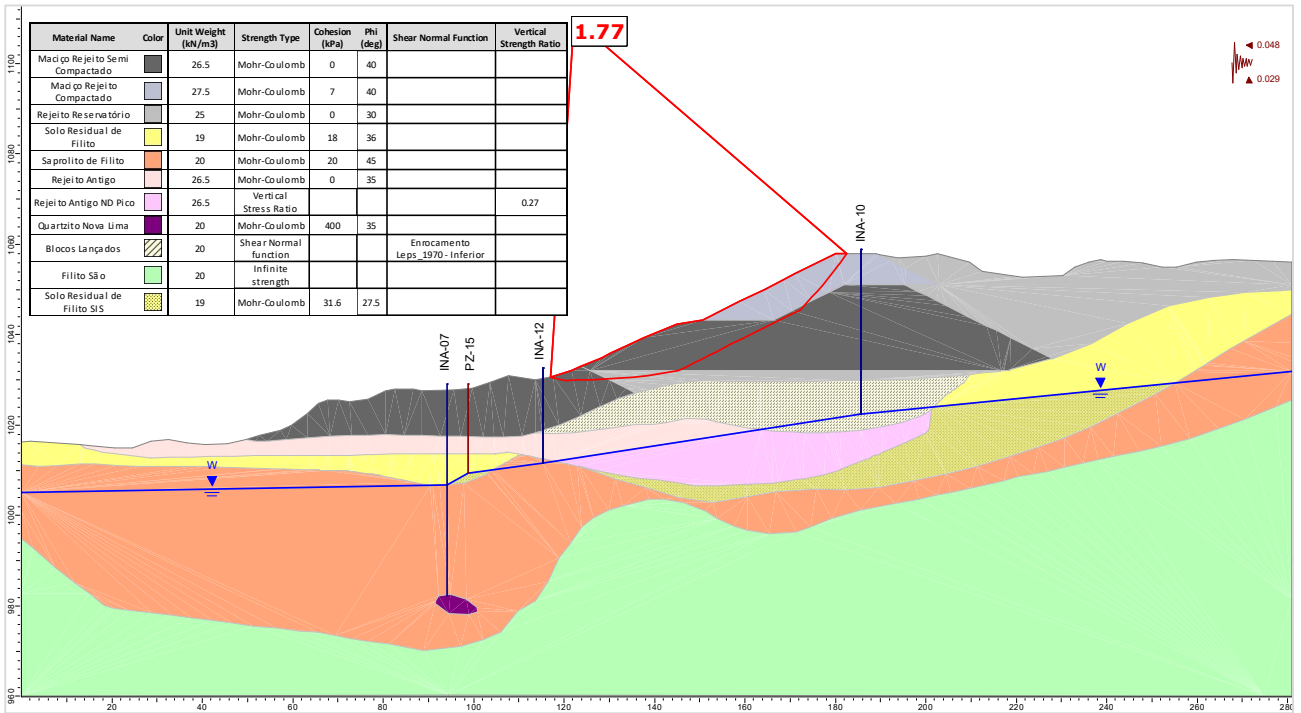
Figura 5.114 – Seção C-C' – Análise Não Drenada – Superfície de ruptura plano-circular otimizada – Freática 30/10/2024 – Razão de resistência não drenada de pico + sismo ↑ (critério vida útil).
