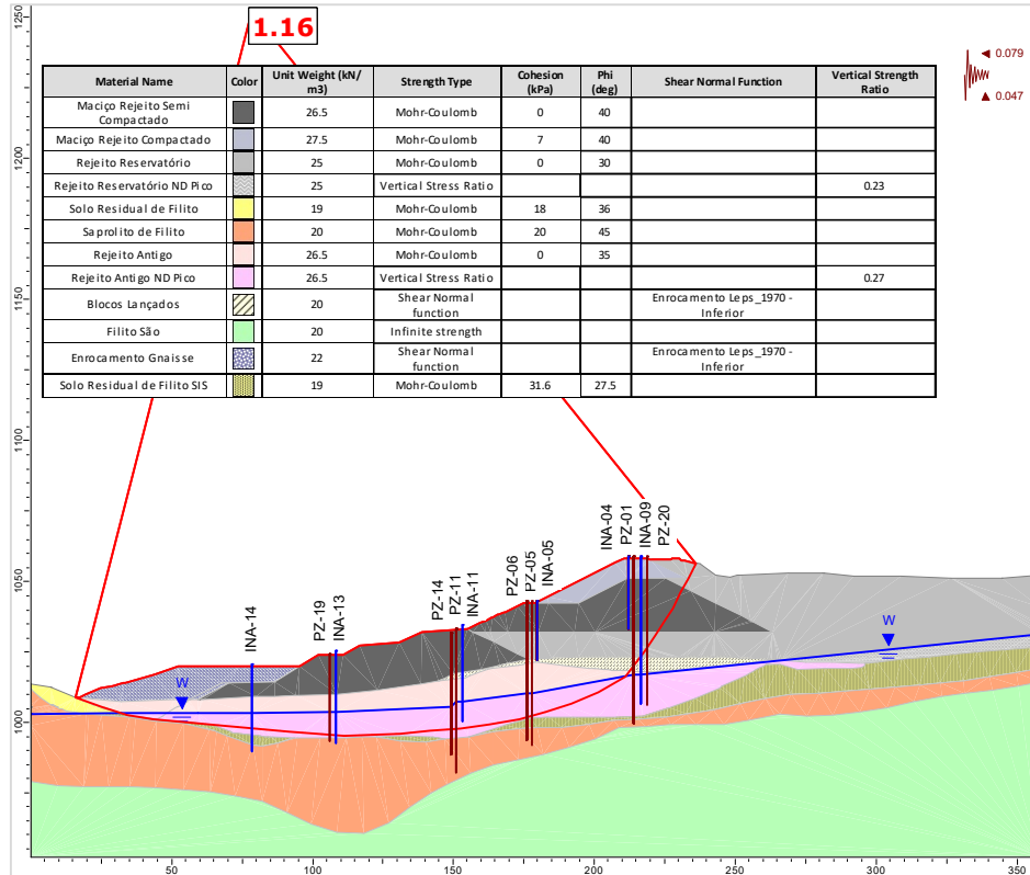
Figura 5.105 – Seção B-B' – Análise Não Drenada – Superfície de ruptura plano-circular otimizada – Freática 30/10/2024 – Razão de resistência não drenada de pico + sismo ↑ (critério CDA).
