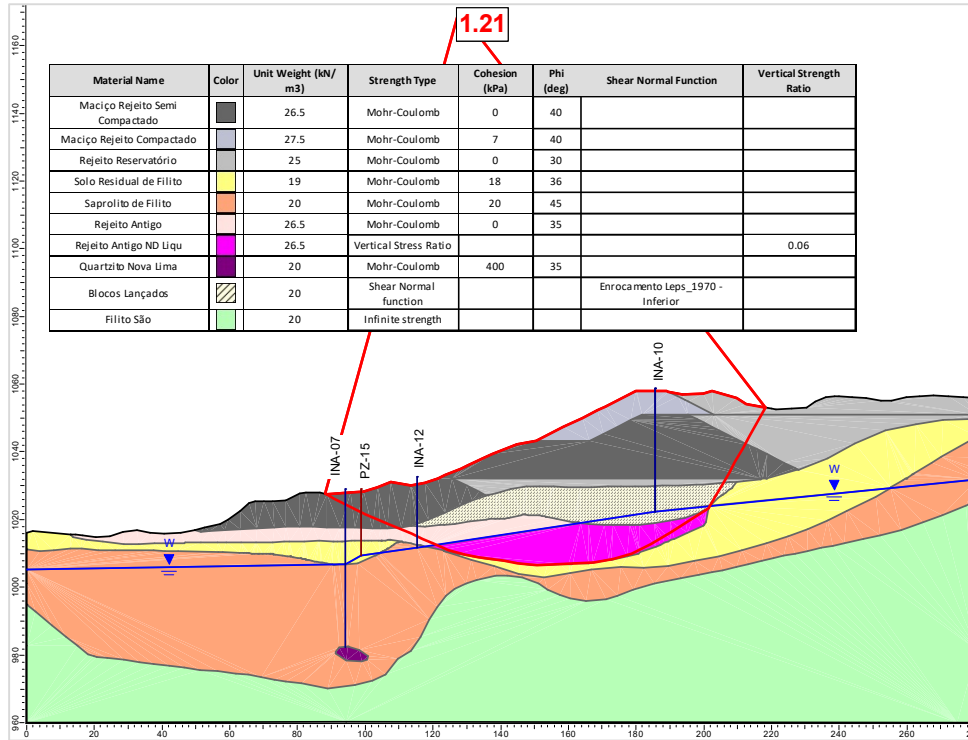
Figura 5.111 – Seção C-C' – Análise Não Drenada – Superfície de ruptura plano-circular otimizada – Freática 30/10/2024 – Razão de resistência não drenada liquefeito.
