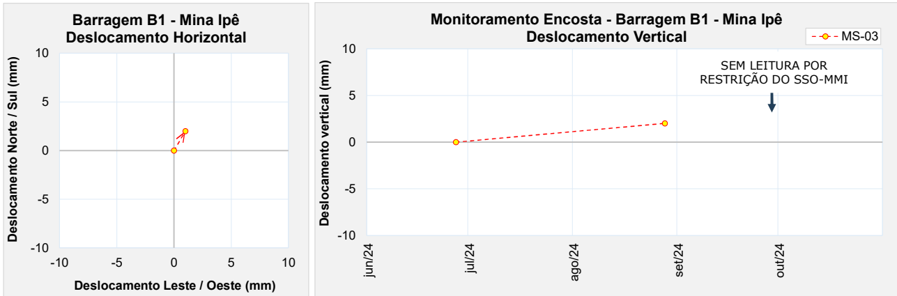
Figura 5.66 – Marco de controle de monitoramento da encosta MS-03.
