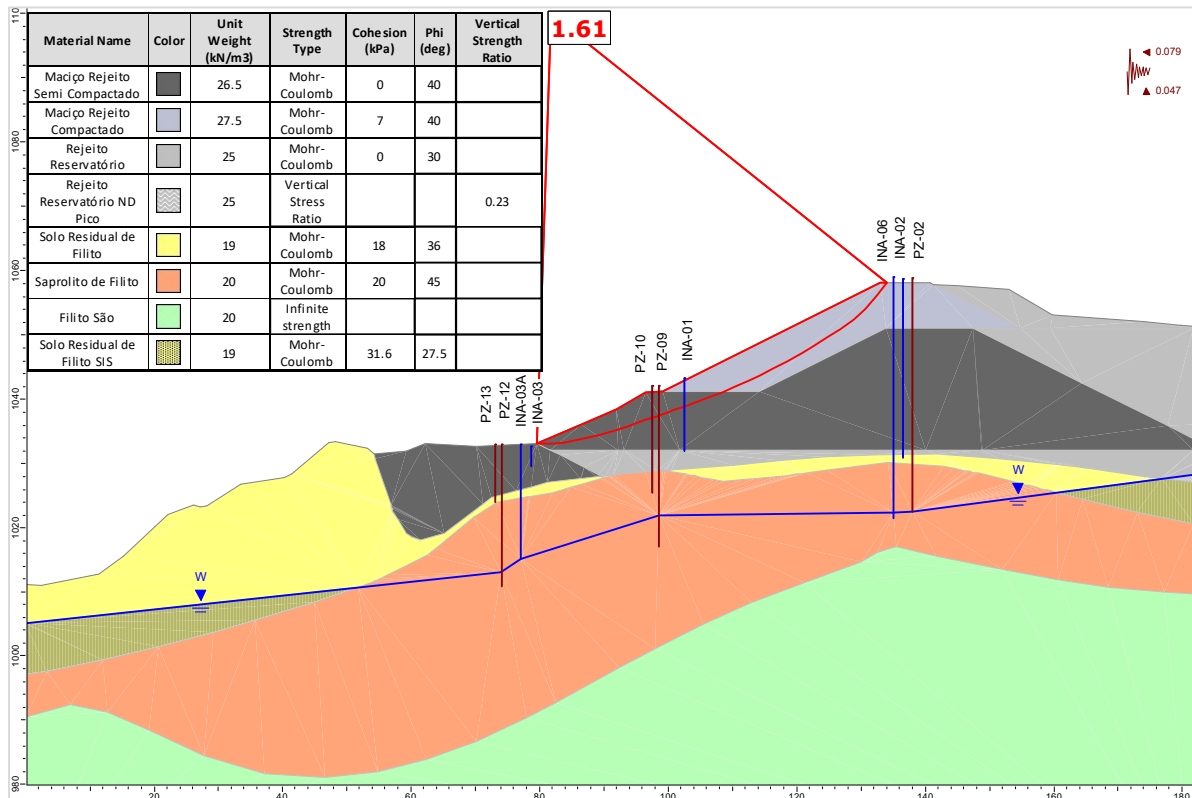
Figura 5.98 – Seção A-A' – Análise Não Drenada – Superfície de ruptura plano-circular otimizada – Freática 30/10/2024 – Razão de resistência não drenada de pico + sismo ↑ (critério CDA).
