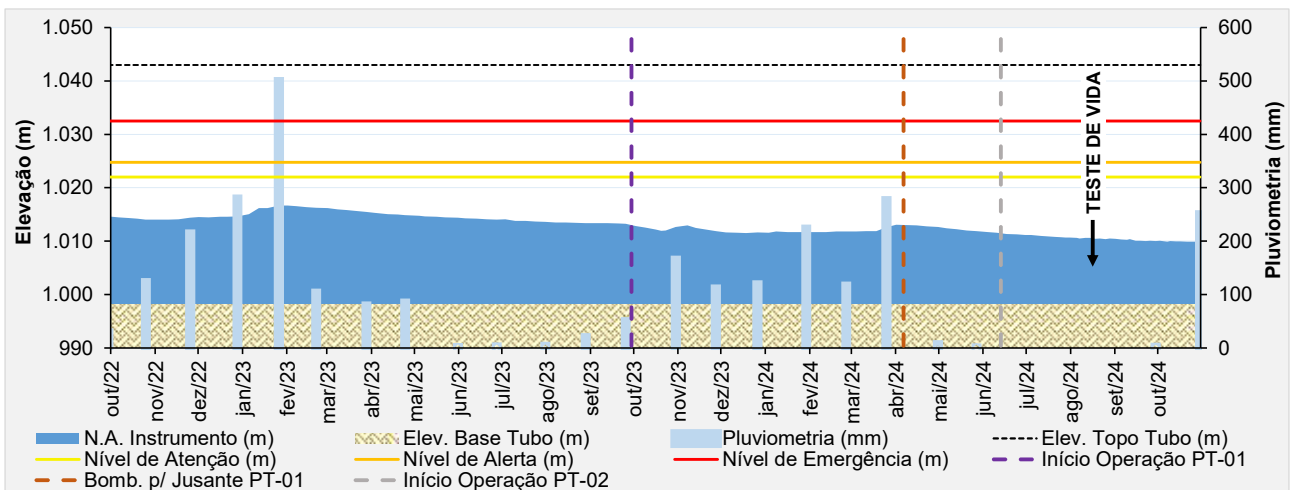
Figura 5.37 – Desempenho do piezômetro de tubo aberto – PZ-06.
