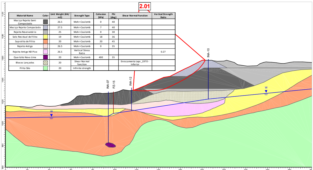
Figura 5.110 – Seção C-C' – Análise Não Drenada – Superfície de ruptura plano-circular otimizada – Freática 30/10/2024 – Razão de resistência não drenada de pico.
