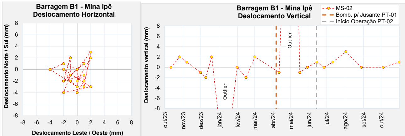
Figura 5.61 – Marco de controle de deformação – MS-02.
