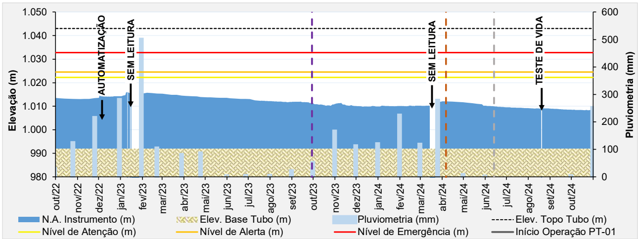
Figura 5.36 – Desempenho do piezômetro automatizado – PZ-05.
