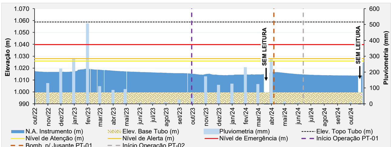
Figura 5.32 – Desempenho do piezômetro automatizado – PZ-01.
