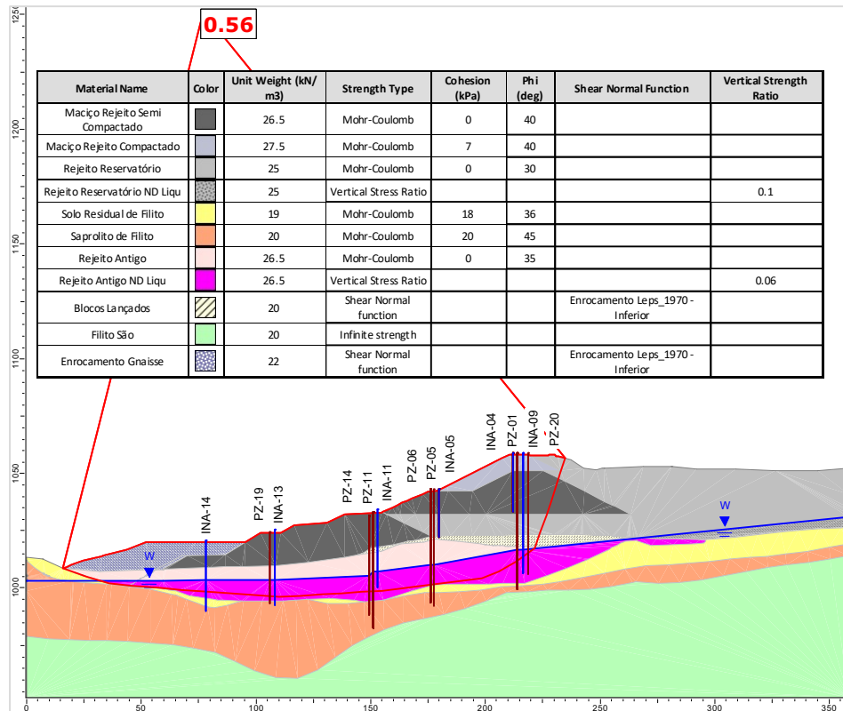
Figura 5.104 – Seção B-B' – Análise Não Drenada – Superfície de ruptura plano-circular otimizada – Freática atual 30/10/2024 – Razão de resistência não drenada liquefeito.
