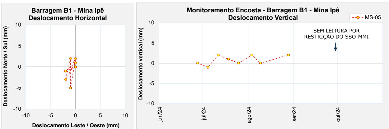
Figura 5.68 – Marco de controle de monitoramento da encosta MS-05.
