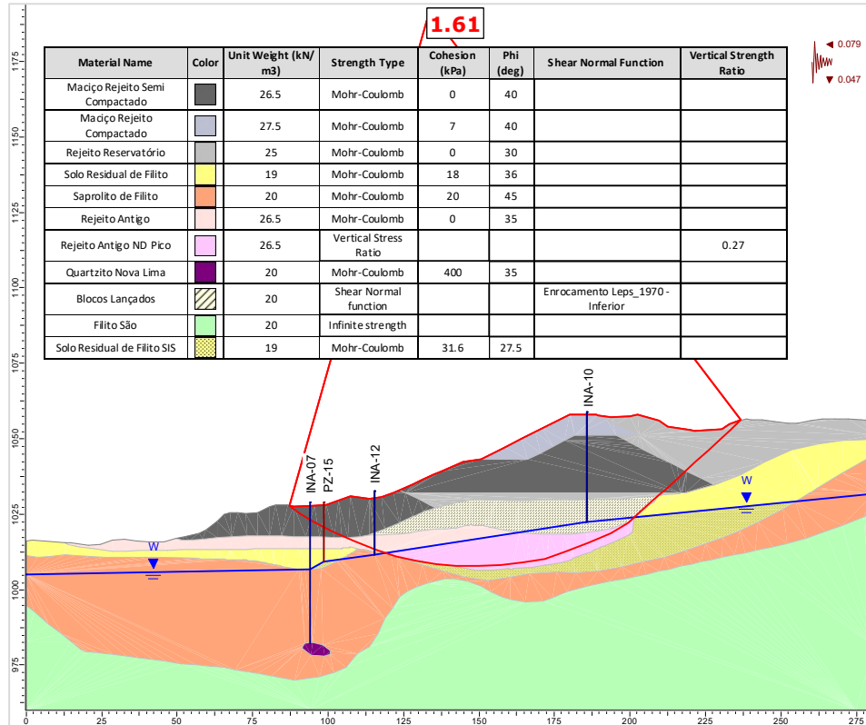
Figura 5.113 – Seção C-C' – Análise Não Drenada – Superfície de ruptura plano-circular otimizada – Freática 30/10/2024 – Razão de resistência não drenada de pico + sismo ↓ (critério CDA).
