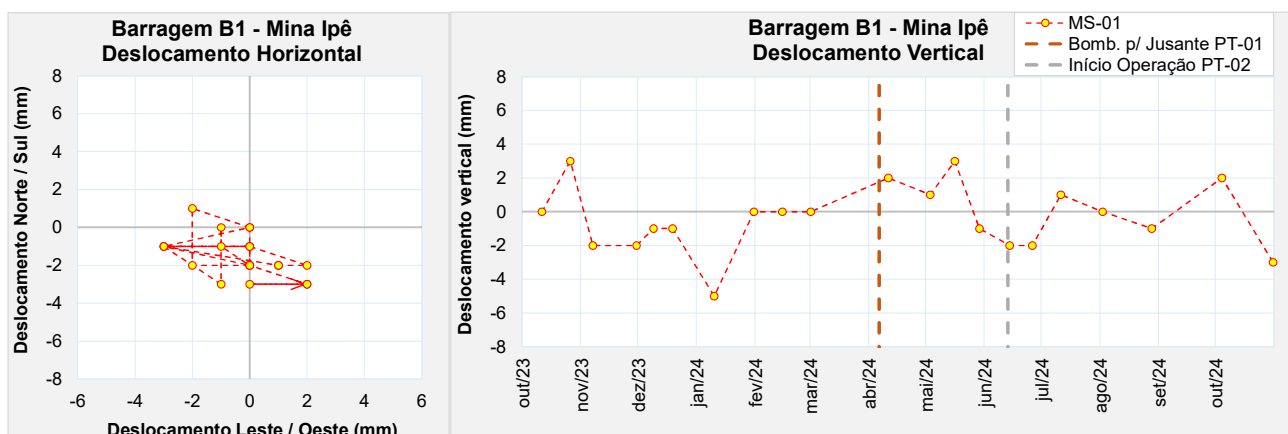
Figura 5.60 – Marco de controle de deformação – MS-01.
