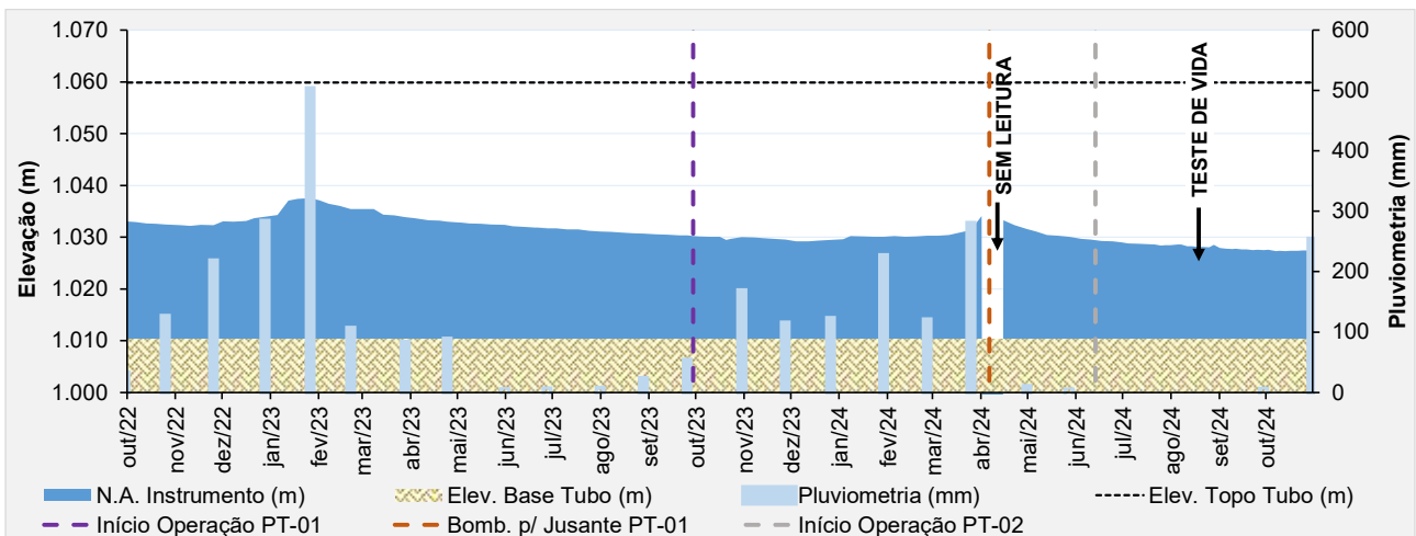
Figura 5.47 – Desempenho do piezômetro de tubo aberto – PZ-16.
