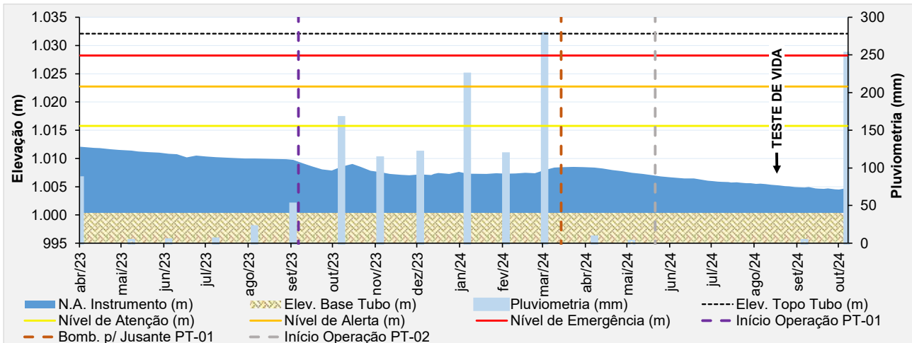
Figura 5.28 – Desempenho do indicador de nível d'água – INA-11.
