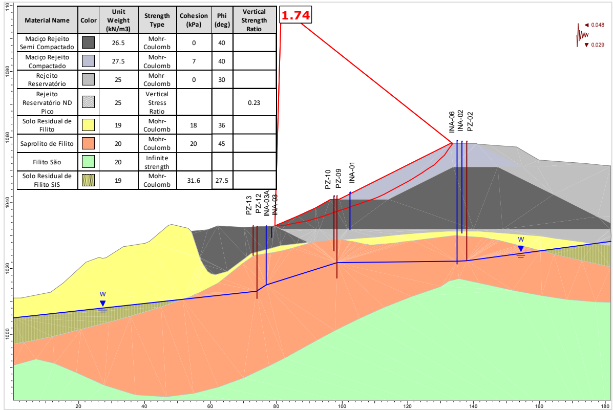
Figura 5.101 – Seção A-A' – Análise Não Drenada – Superfície de ruptura plano-circular otimizada – Freática 30/10/2024 – Razão de resistência não drenada de pico + sismo ↓ (critério vida útil).
