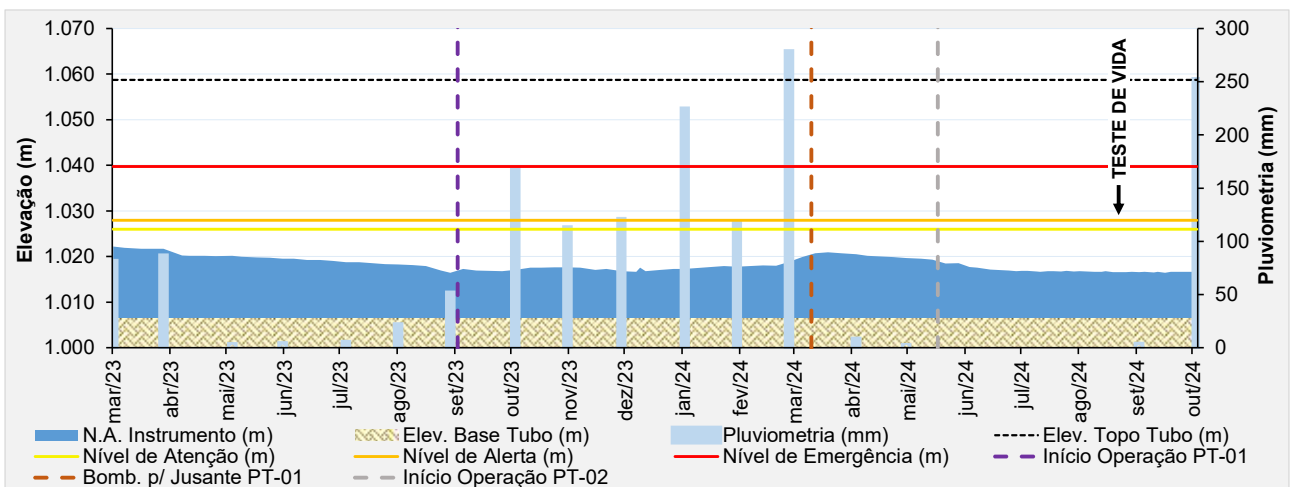
Figura 5.26 – Desempenho do indicador de nível d'água – INA-09.
