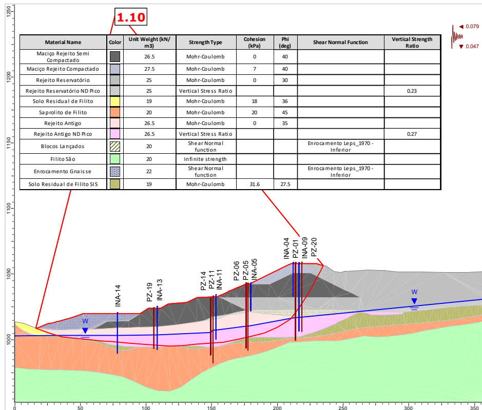
Figura 5.106 – Seção B-B' – Análise Não Drenada – Superfície de ruptura plano-circular otimizada – Freática 30/10/2024 – Razão de resistência não drenada de pico + sismo ↓ (critério CDA).
