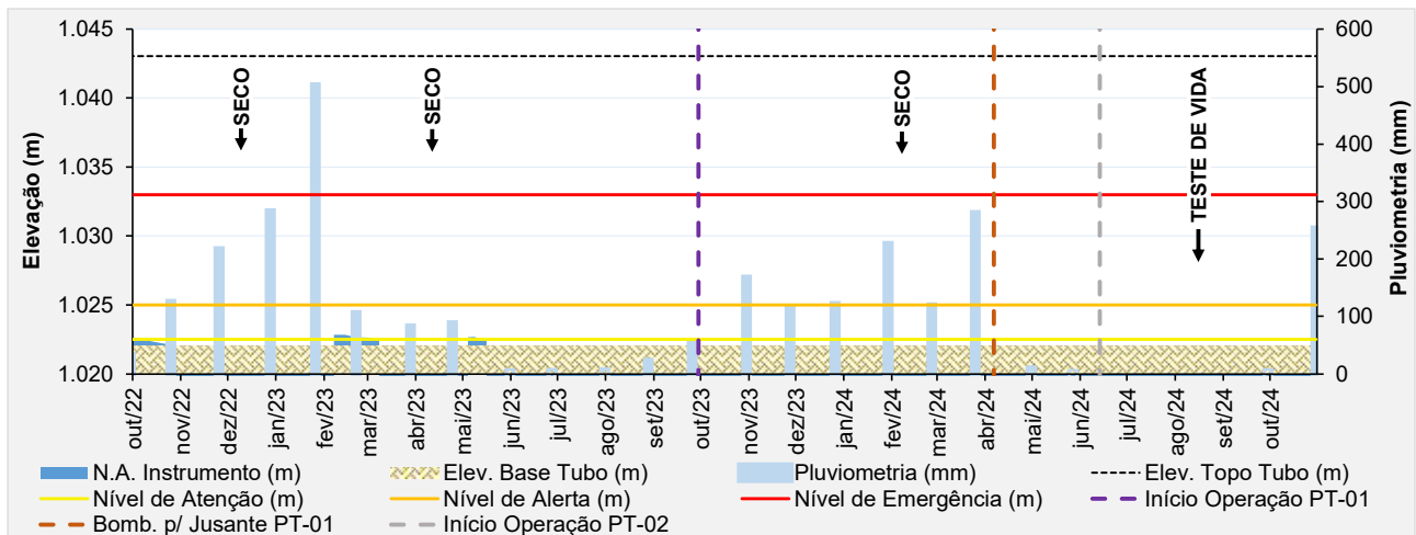
Figura 5.22 - Desempenho do indicador de nível d'água - INA-05.
