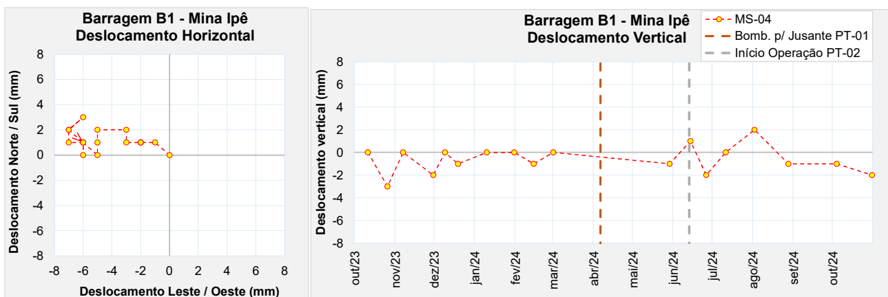
Figura 5.63 – Marco de controle de deformação – MS-04.
