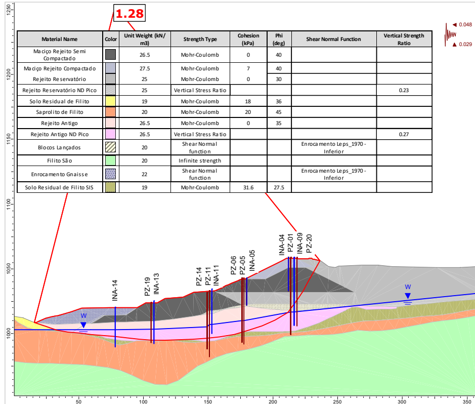
Figura 5.107 – Seção B-B' – Análise Não Drenada – Superfície de ruptura plano-circular otimizada – Freática 30/10/2024 – Razão de resistência não drenada de pico + sismo ↑ (critério vida útil).
