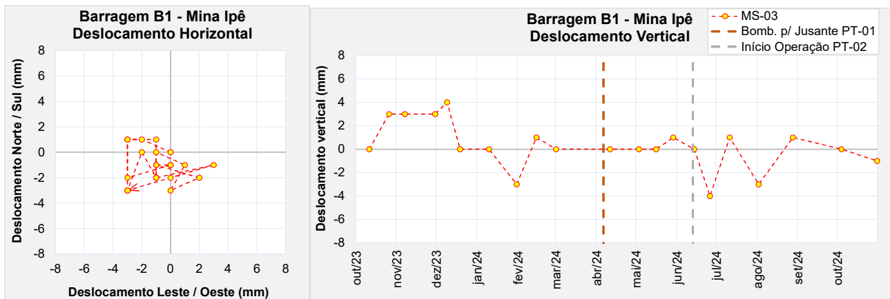
Figura 5.62 – Marco de controle de deformação – MS-03.
