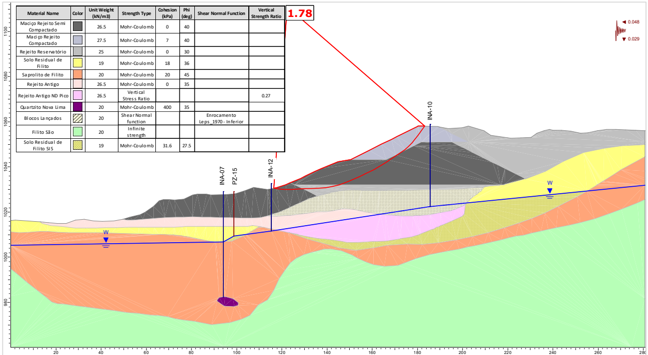
Figura 5.115 – Seção C-C' – Análise Não Drenada – Superfície de ruptura plano-circular otimizada – Freática 30/10/2024 – Razão de resistência não drenada de pico + sismo ↓ (critério vida útil).
