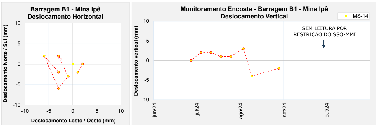
Figura 5.77 – Marco de controle de monitoramento da encosta MS-14.
