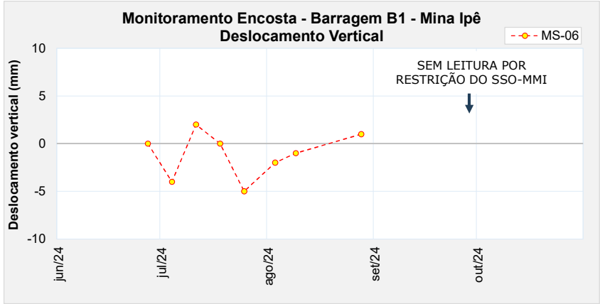
Figura 5.69 – Marco de controle de monitoramento da encosta MS-06.
