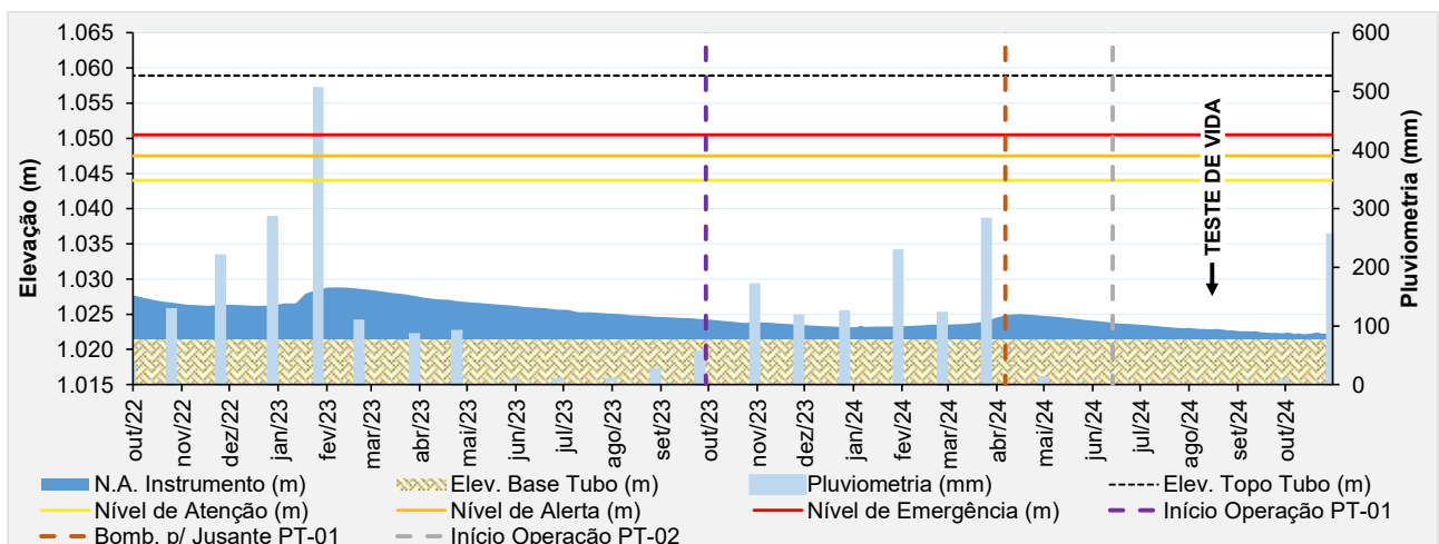
Figura 5.23 - Desempenho do indicador de nível d'água - INA-06.
