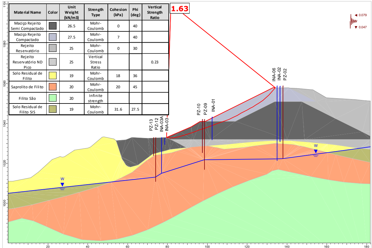
Figura 5.99 – Seção A-A' – Análise Não Drenada – Superfície de ruptura plano-circular otimizada – Freática 30/10/2024 – Razão de resistência não drenada de pico + sismo ↓ (critério CDA).
