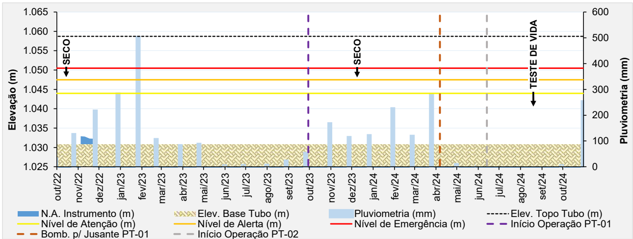
Figura 5.18 - Desempenho do indicador de nível d'água - INA-02.
