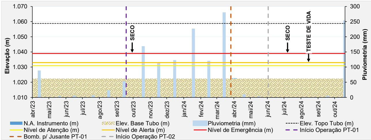
Figura 5.27 – Desempenho do indicador de nível d'água – INA-10.
