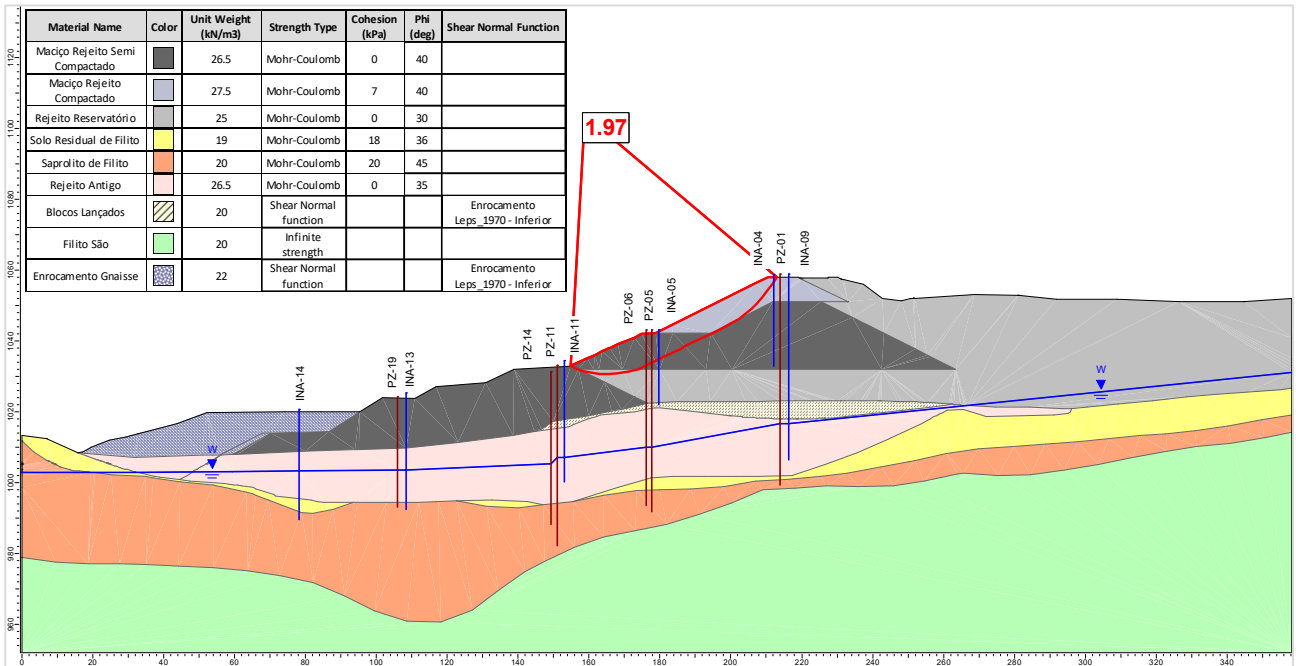
Figura 5.102 – Seção B-B' – Análise Drenada – Superfície de ruptura plano-circular otimizada – Freática 30/10/2024.
