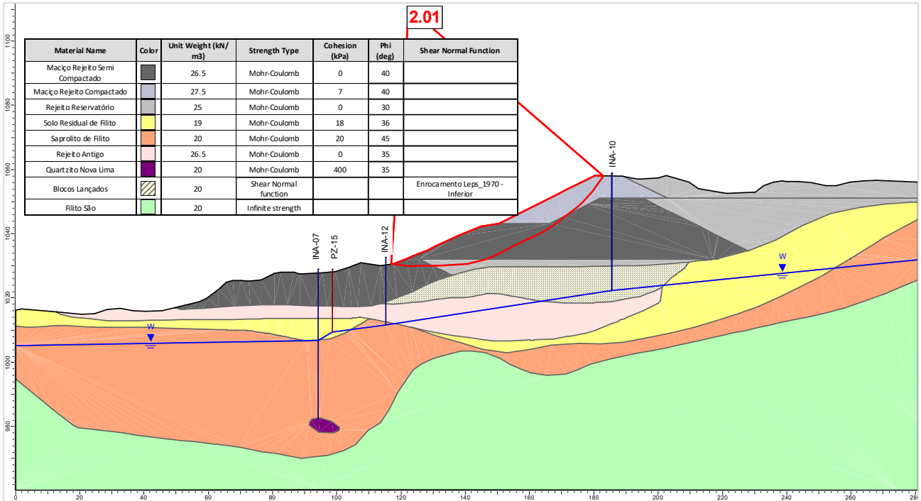
Figura 5.109 – Seção C-C' – Análise Drenada – Superfície de ruptura plano-circular otimizada – Freática 30/10/2024.
