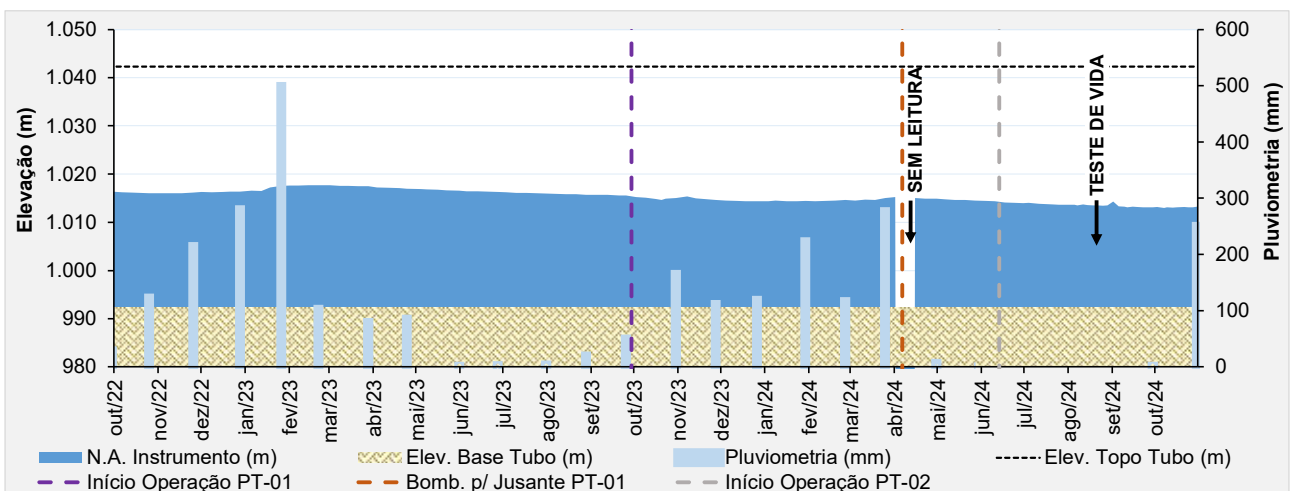
Figura 5.38 – Desempenho do piezômetro de tubo aberto – PZ-07.
