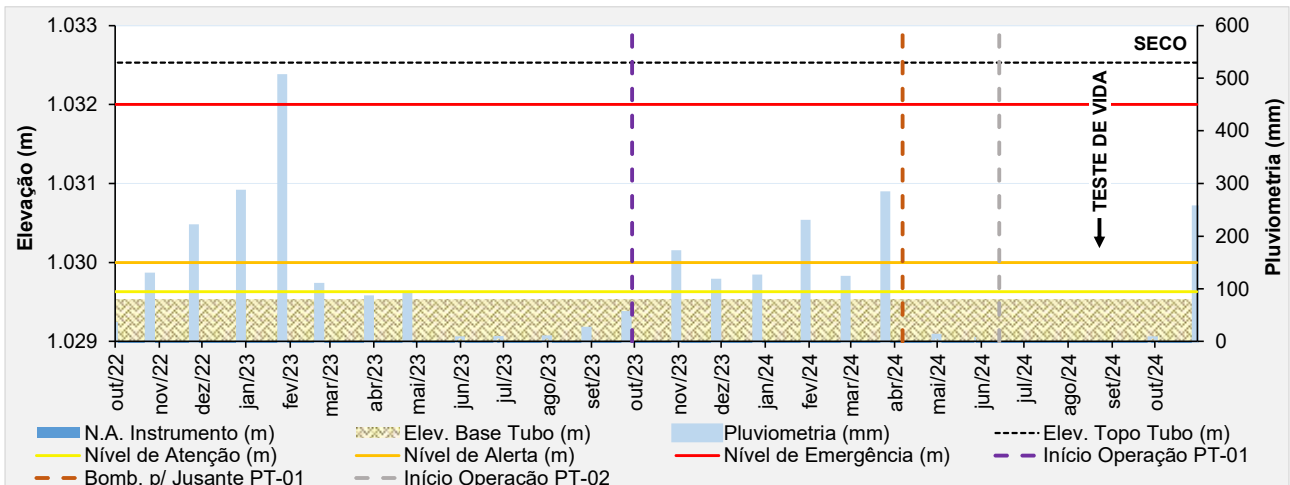
Figura 5.19 - Desempenho do indicador de nível d'água - INA-03.
