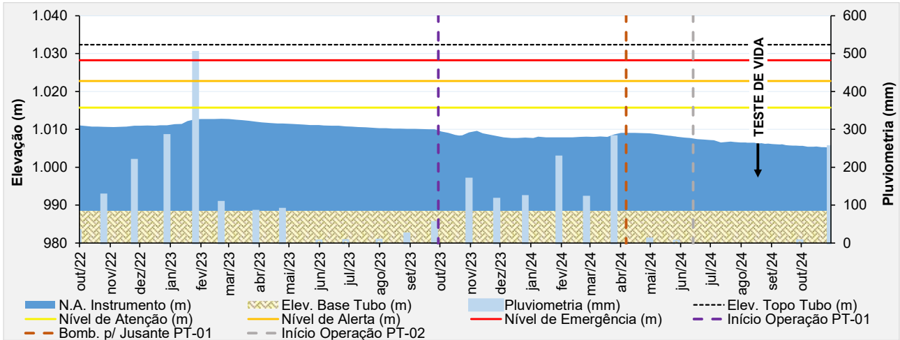
Figura 5.45 – Desempenho do piezômetro de tubo aberto – PZ-14.
