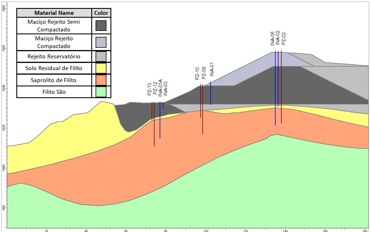
Figura 5.14 – Seção transversal de controle A-A'.
