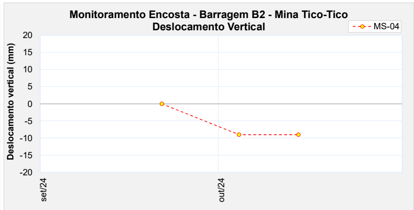
Figura 5.24 - Marco de controle de monitoramento da encosta - MS-04.
