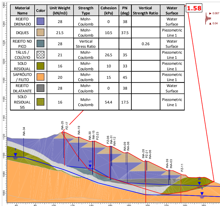
Figura 6.101 – Seção A-A' – Análise Não Drenada – Superfície de ruptura plano-circular otimizada – Freática 30/10/2024 – Razão de resistência não drenada de pico + sismo ↑ (critério vida útil).
