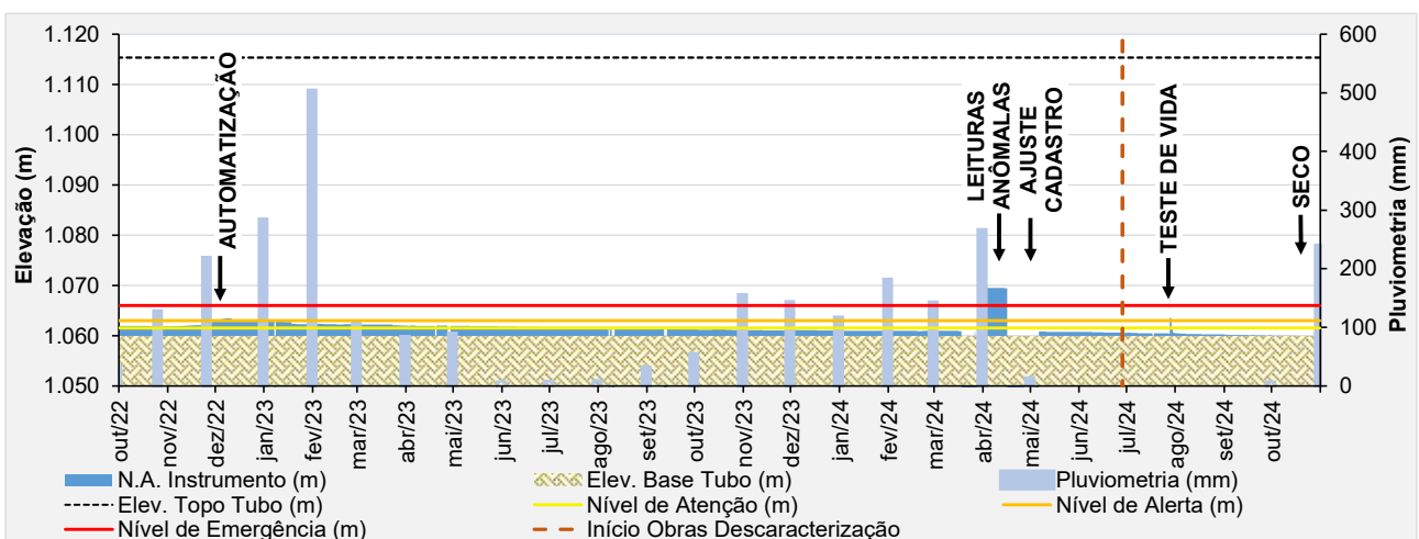
Figura 6.64 – Desempenho do piezômetro automatizado – PZ-03.
