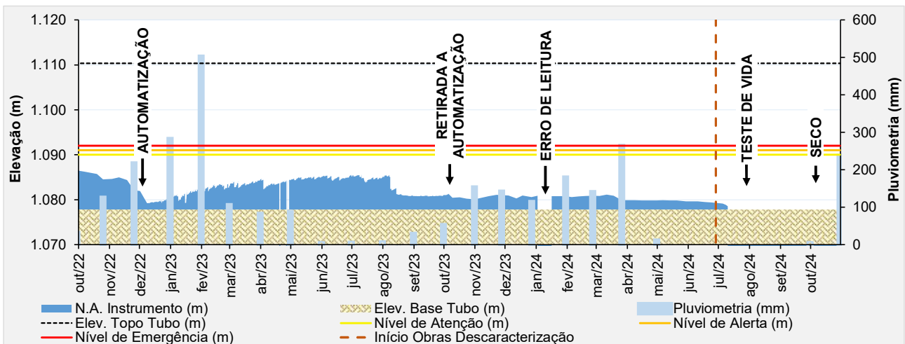
Figura 6.52 – Desempenho do indicador de nível d'água – INA-31.
