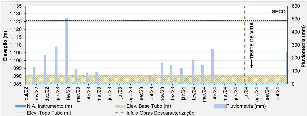
Figura 6.78 – Desempenho do piezômetro de tubo aberto – PZ-17.
