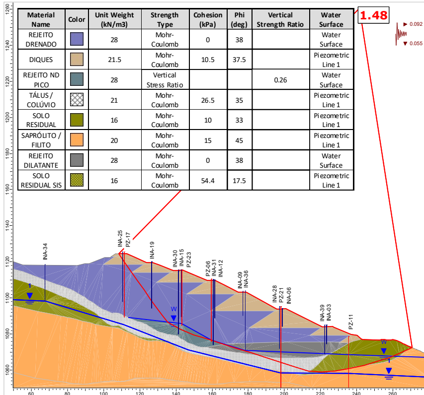
Figura 6.100 – Seção A-A' – Análise Não Drenada – Superfície de ruptura plano-circular otimizada – Freática 30/10/2024 – Razão de resistência não drenada de pico + sismo ↓ (critério CDA).
