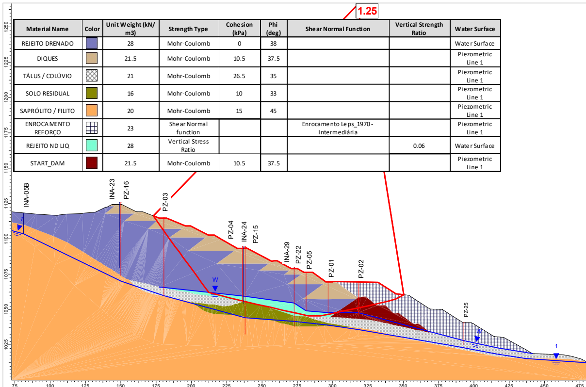
Figura 6.117 – Seção D-D' – Análise Não Drenada – Superfície de ruptura plano-circular otimizada – Freática 30/10/2024 – Razão de resistência não drenada liquefeita.
