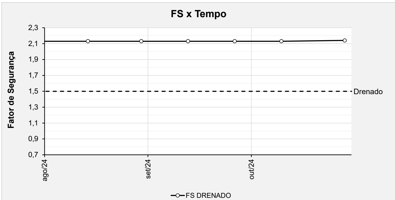
Figura 6.131 – Seção C-C' - Histórico dos F.S. obtidos nas análises de estabilidade no período avaliado.
