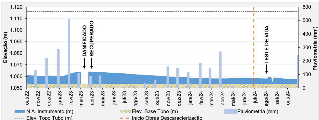
Figura 6.69 – Desempenho do piezômetro de tubo aberto – PZ-08.
