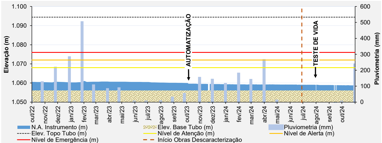
Figura 6.65 – Desempenho do piezômetro automatizado – PZ-04.
