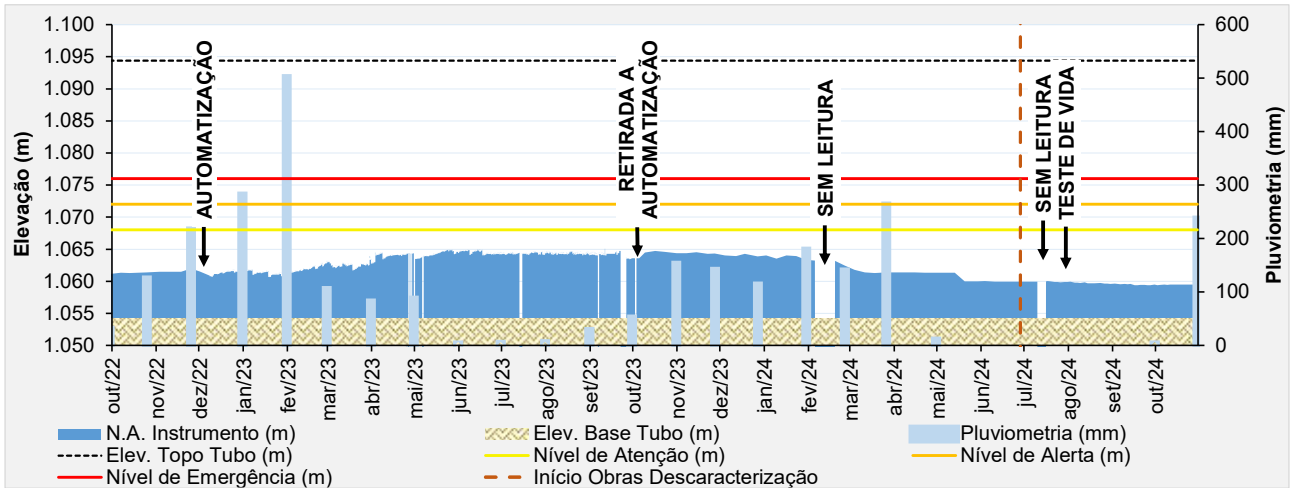
Figura 6.45 – Desempenho do indicador de nível d'água – INA-24.
