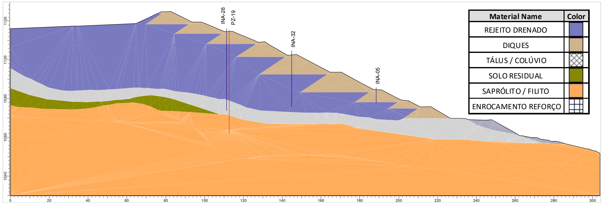
Figura 6.22 – Seção transversal de controle C-C' (Condição em 31/10/2024).
