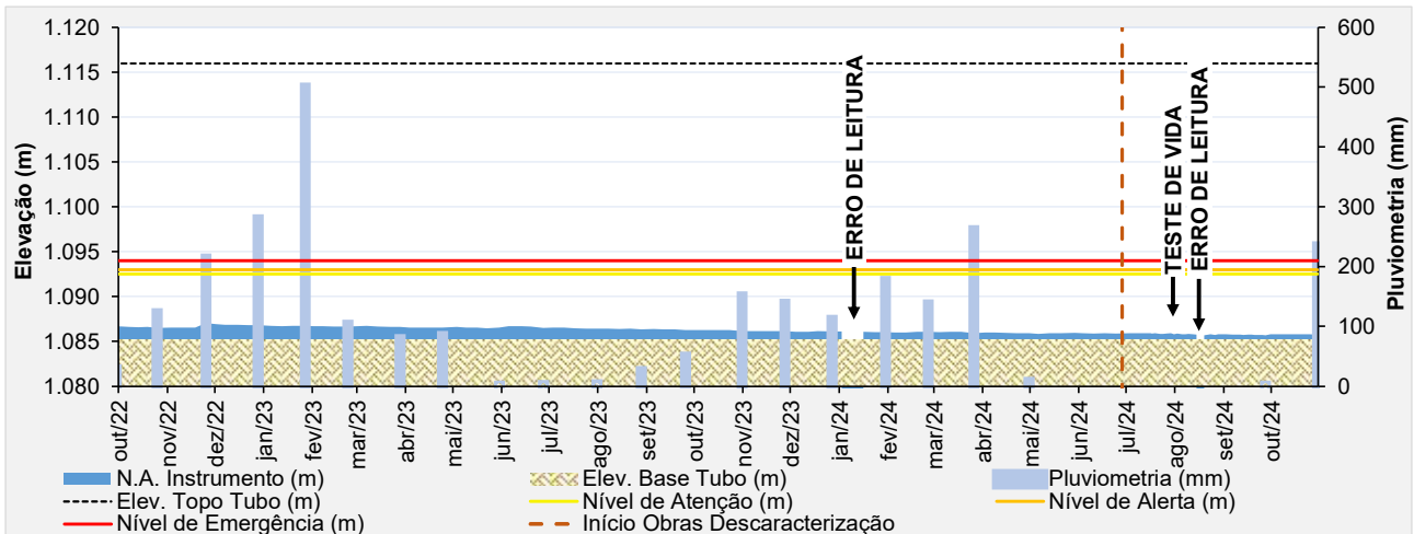
Figura 6.84 – Desempenho do piezômetro de tubo aberto – PZ-23.
