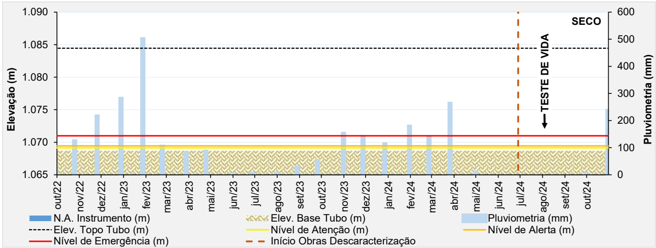
Figura 6.29 – Desempenho do indicador de nível d'água – INA-04.
