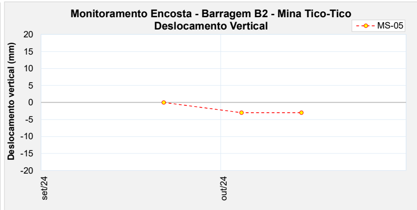
Figura 5.25 – Marco de controle de monitoramento da encosta – MS-05.
