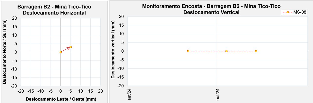
Figura 5.28 – Marco de controle de monitoramento da encosta – MS-08.
