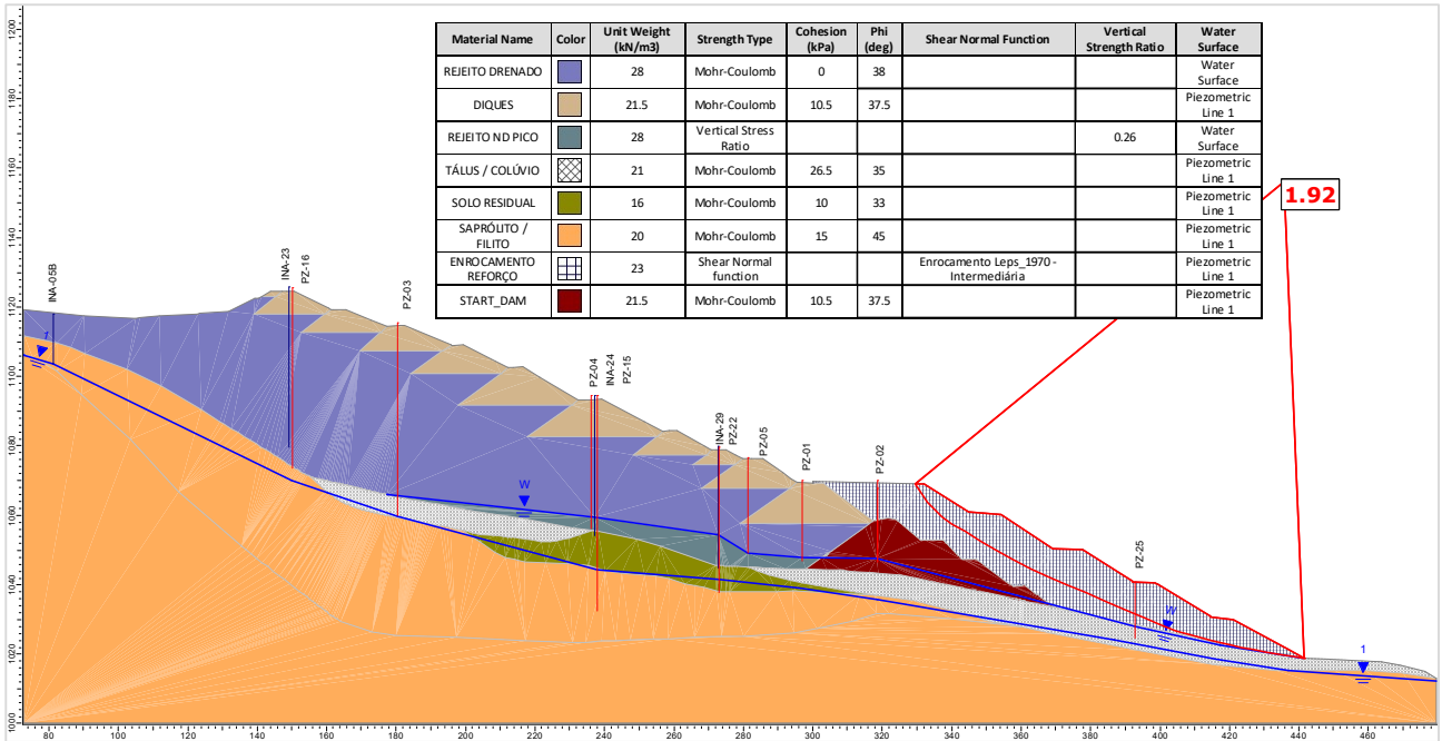
Figura 6.116 – Seção D-D' – Análise Não Drenada – Superfície de ruptura plano-circular otimizada – Freática 30/10/2024 – Razão de resistência não drenada de pico.
