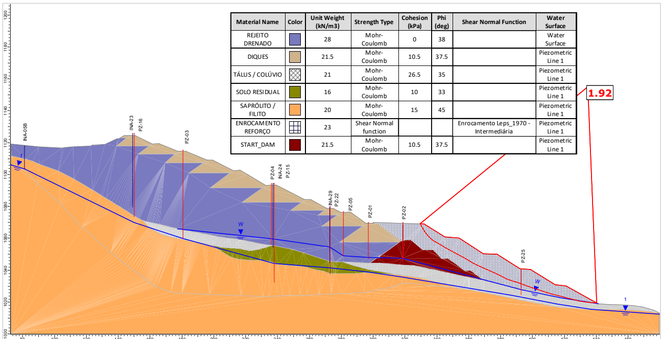
Figura 6.115 – Seção D-D' – Análise Drenada – Superfície de ruptura plano-circular otimizada – Freática 30/10/2024.
