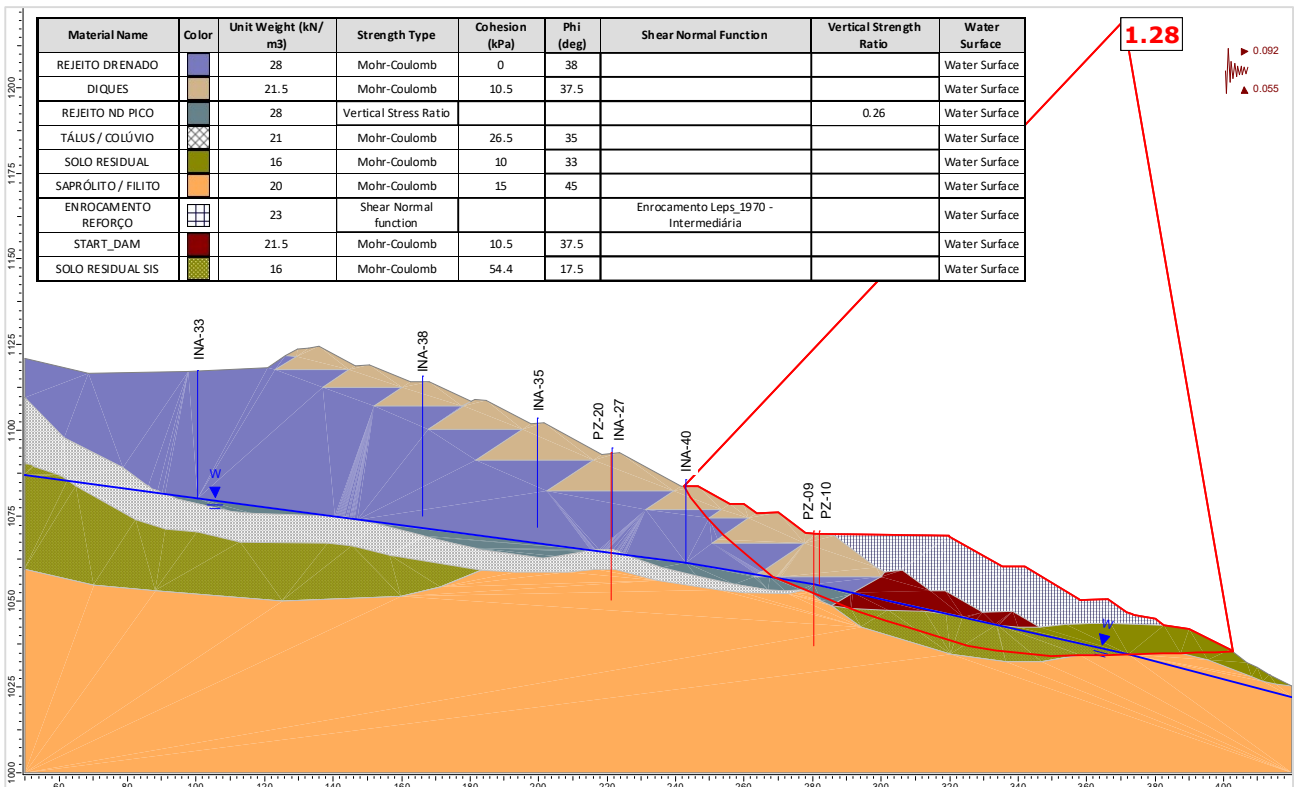
Figura 6.125 – Seção E-E' – Análise Não Drenada – Superfície de ruptura plano-circular otimizada – Freática 30/10/2024 – Razão de resistência não drenada de pico + sismo ↑ (critério CDA).
