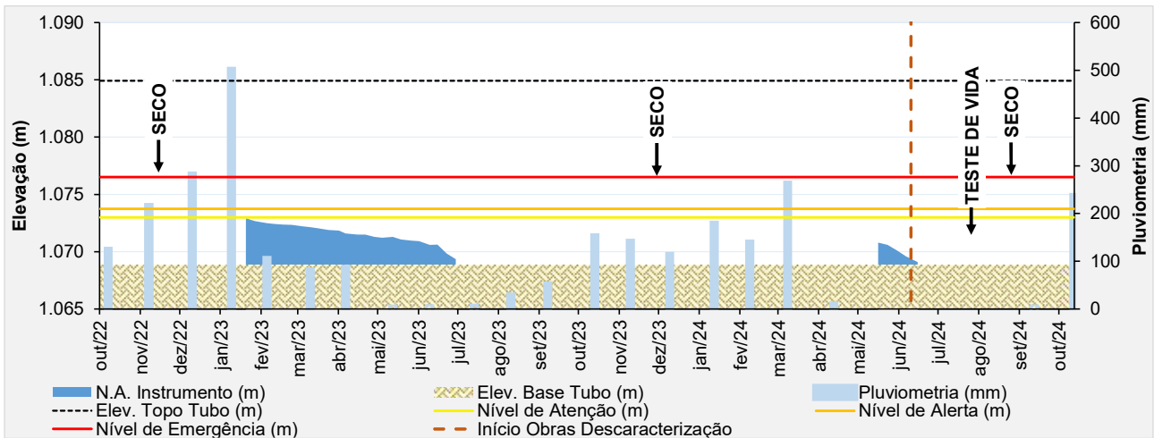
Figura 6.60 – Desempenho do indicador de nível d'água – INA-39.
