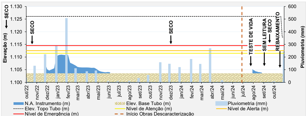
Figura 6.31 – Desempenho do indicador de nível d'água – INA-05B.
