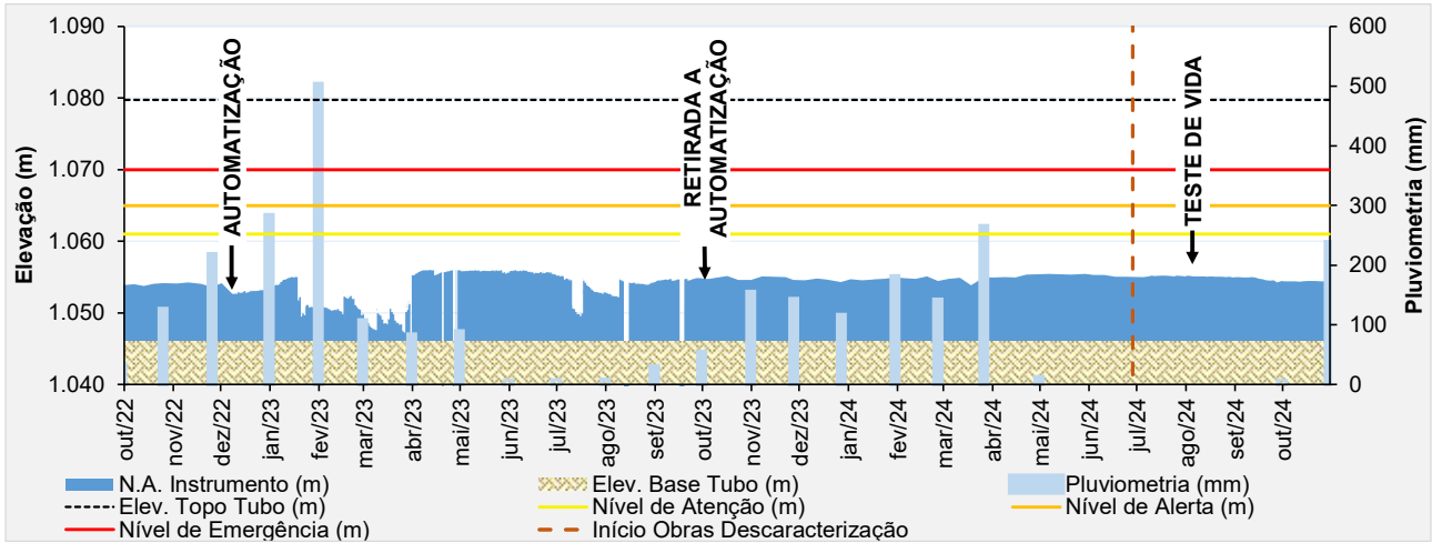
Figura 6.50 – Desempenho do indicador de nível d'água – INA-29.
