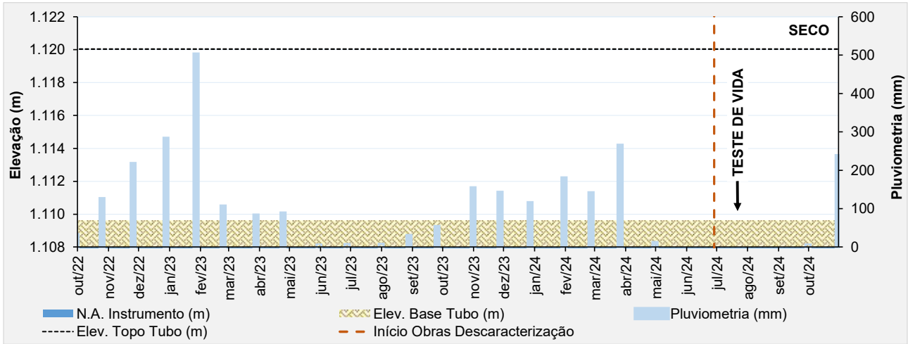
Figura 6.41 - Desempenho do indicador de nível d'água - INA-18.
