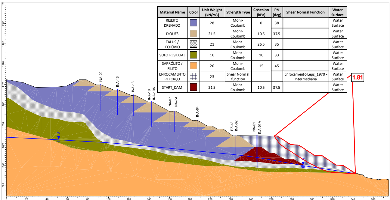
Figura 6.103 – Seção B-B' – Análise Drenada – Superfície de ruptura plano-circular otimizada – Freática 30/10/2024.
