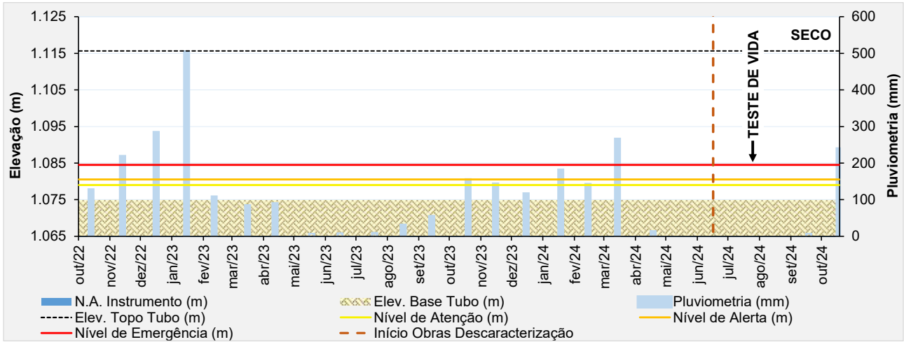
Figura 6.59 – Desempenho do indicador de nível d'água – INA-38.
