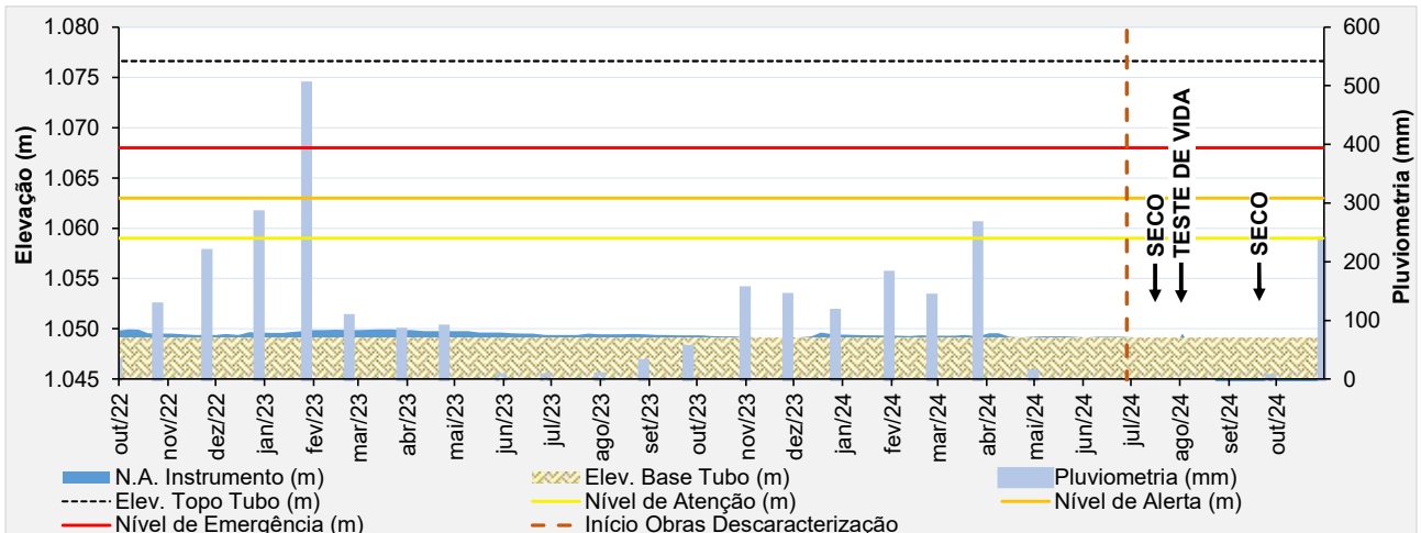
Figura 6.66 – Desempenho do piezômetro de tubo aberto – PZ-05.
