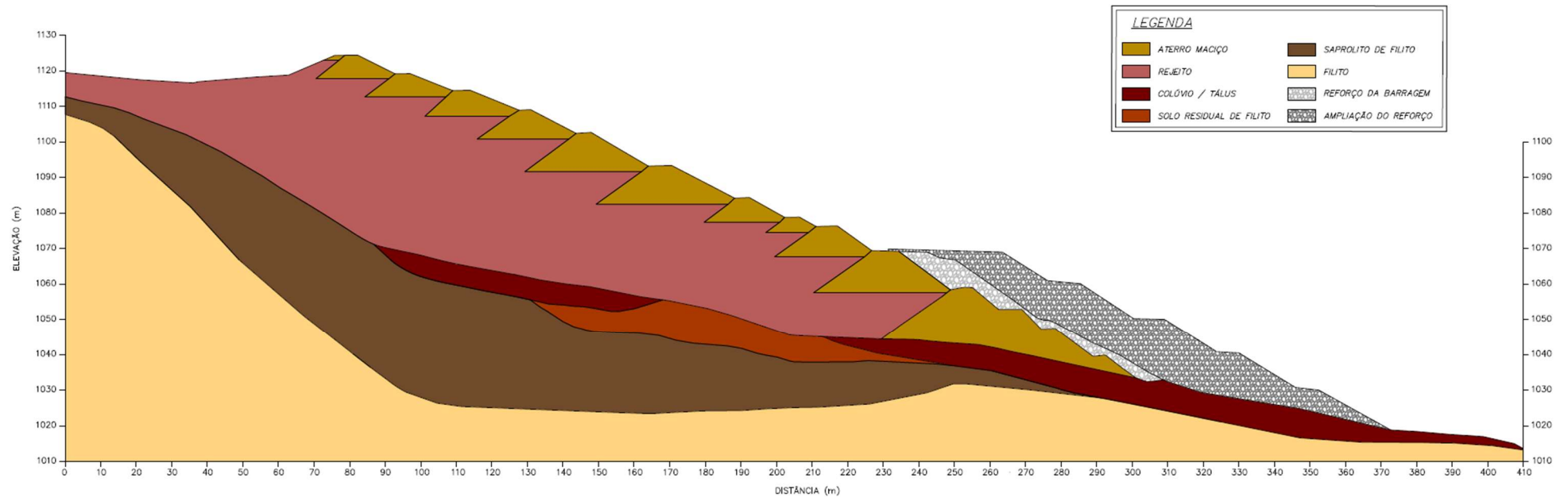
Figura 4.3 – Seção de maior altura (D-D') da Barragem B2 – Mina Tico-Tico (Condição em 31/10/2024).
