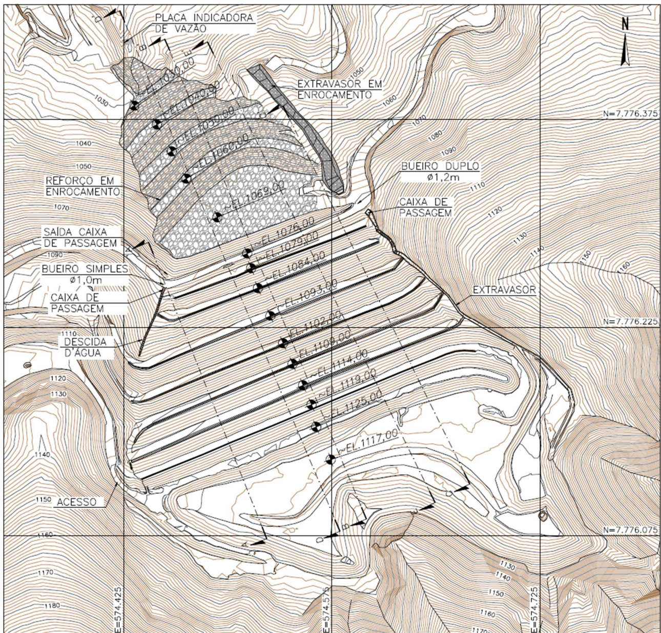
Figura 6.7 – Levantamento topográfico 31/10/24 – Obras Executadas - Planta.
