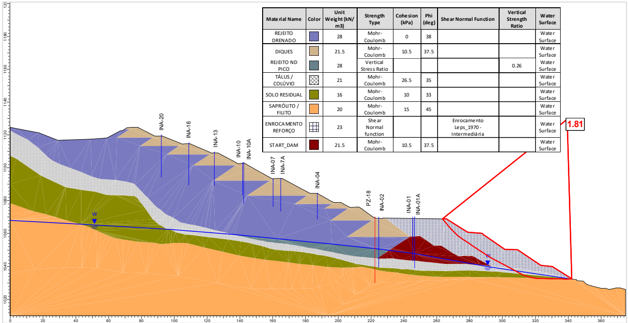
Figura 6.104 – Seção B-B' – Análise Não Drenada – Superfície de ruptura plano-circular otimizada – Freática 30/10/2024 – Razão de resistência não drenada de pico.
