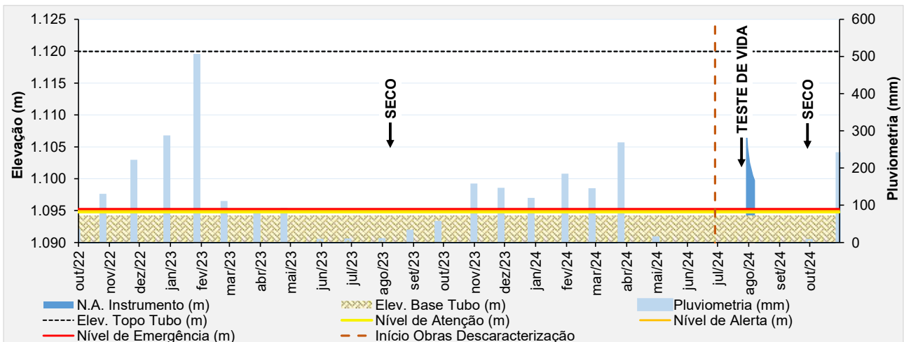
Figura 6.43 - Desempenho do indicador de nível d'água - INA-20.
