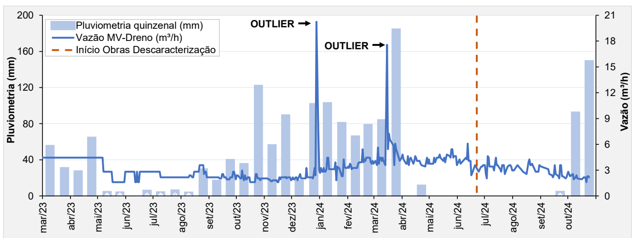
Figura 6.87 – Vazão – MV-Dreno – Barragem B2 – Mina Tico-Tico.
