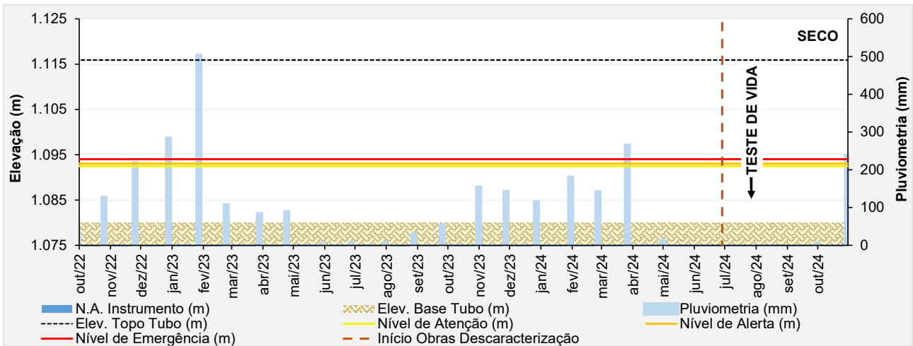
Figura 6.51 – Desempenho do indicador de nível d'água – INA-30.
