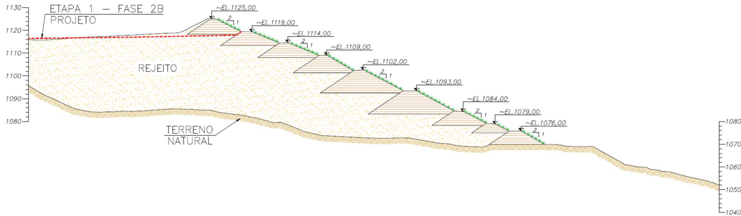
Figura 6.13 – Comparativo Projeto (Etapa 1 - Fase 2B) x Executado – Seção C-C’.
