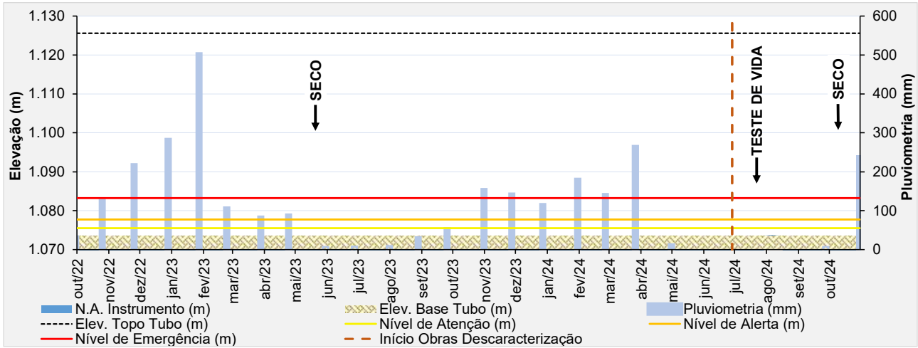
Figura 6.77 – Desempenho do piezômetro de tubo aberto – PZ-16.
