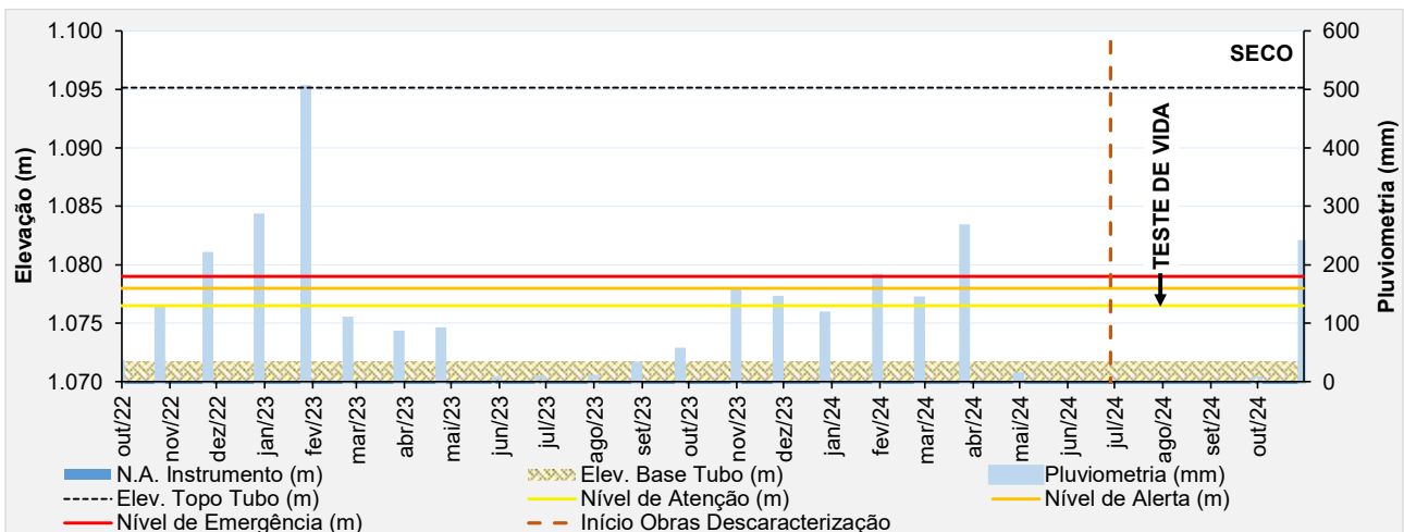
Figura 6.49 – Desempenho do indicador de nível d'água – INA-28.
