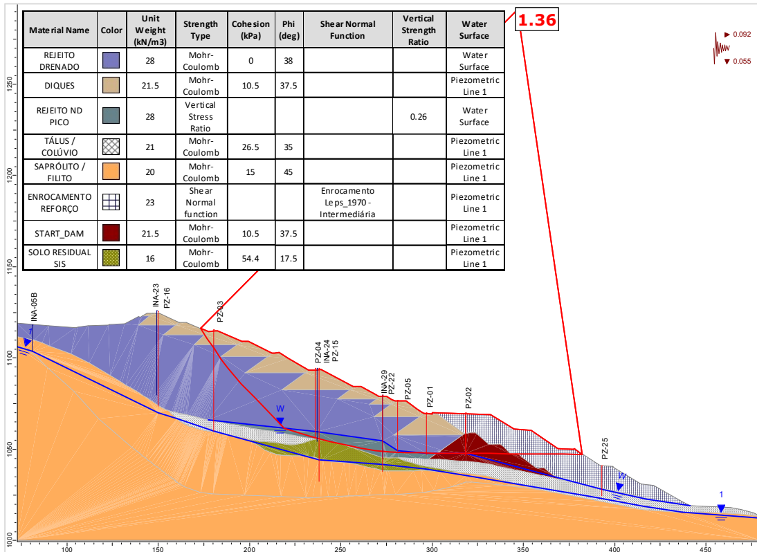
Figura 6.119 – Seção D-D' – Análise Não Drenada – Superfície de ruptura plano-circular otimizada – Freática 30/10/2024 – Razão de resistência não drenada de pico + sismo ↓ (critério CDA).
