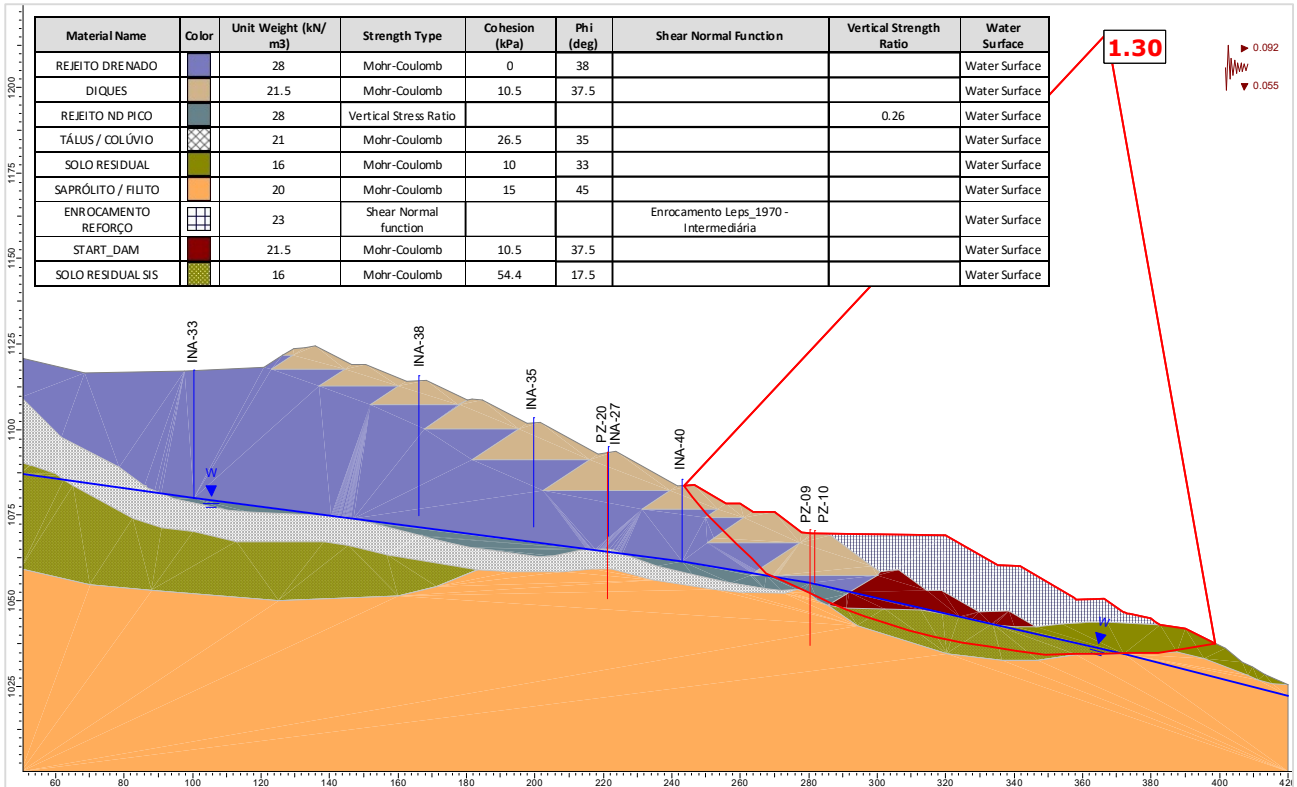
Figura 6.126 – Seção E-E' – Análise Não Drenada – Superfície de ruptura plano-circular otimizada – Freática 30/10/2024 – Razão de resistência não drenada de pico + sismo ↓ (critério CDA).
