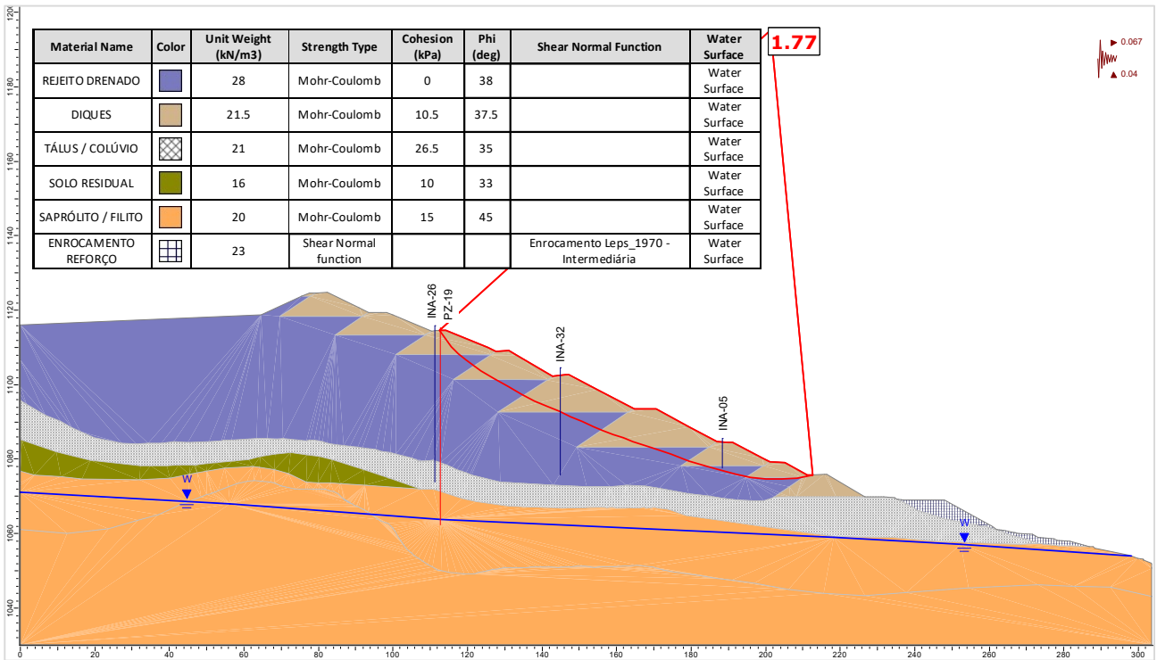
Figura 6.113 – Seção C-C' – Análise Drenada – Superfície de ruptura plano-circular otimizada – Freática 30/10/2024 – Carregamento sísmico ↑ (critério vida útil).
