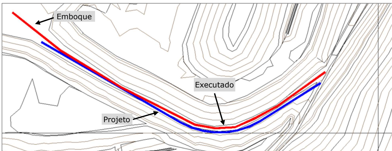
Figura 6.2 – Comparação entre o alinhamento do eixo do canal executado e de projeto – Planta. (Fonte: IPE.OP.DE.8000.GT.20.1055).
