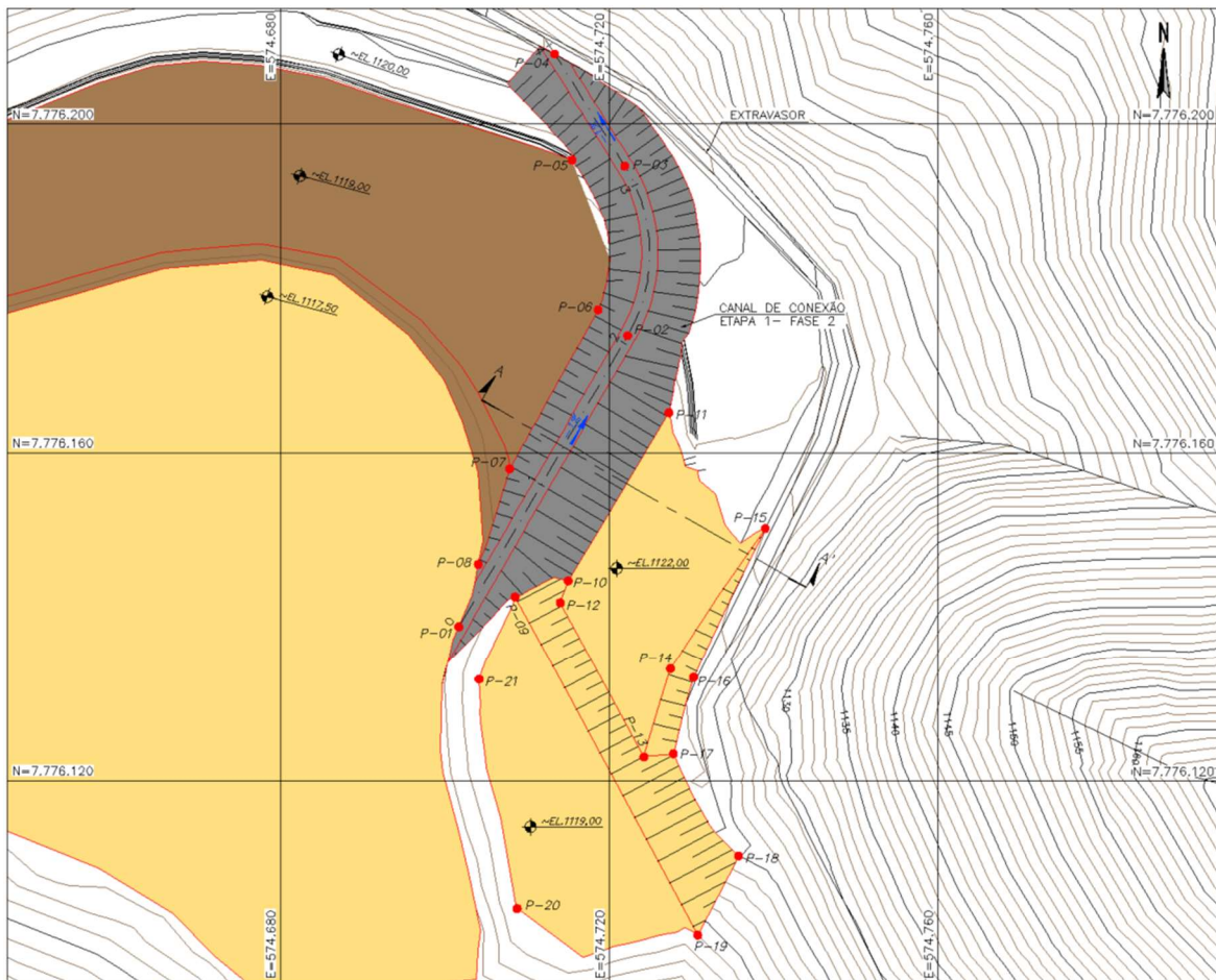
Figura 5.12 - Canal de conexão com extravasor de emergência (Etapa 1 - Fase 2) - Planta (Fonte: IPE.OP.DE.8000.GT.20.1013).
