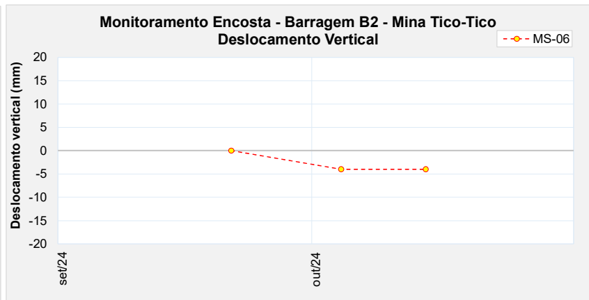
Figura 5.26 – Marco de controle de monitoramento da encosta – MS-06.
