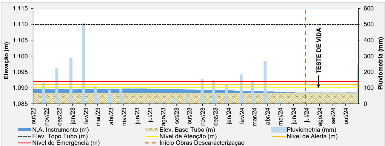
Figura 6.37 – Desempenho do indicador de nível d'água – INA-12.
