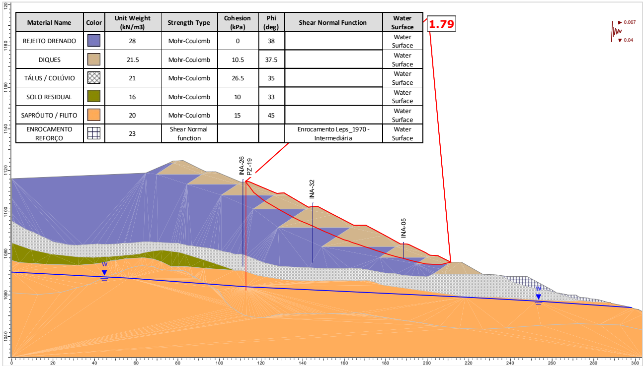
Figura 6.114 – Seção C-C' – Análise Drenada – Superfície de ruptura plano-circular otimizada – Freática 30/10/2024 – Carregamento sísmico ↓ (critério vida útil).
