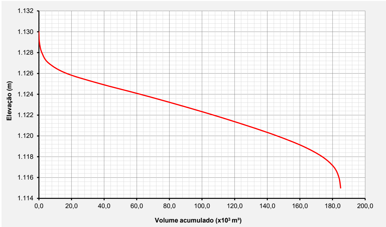
Figura 6.9 – Curva elevação x volume – Remoção Executada.
