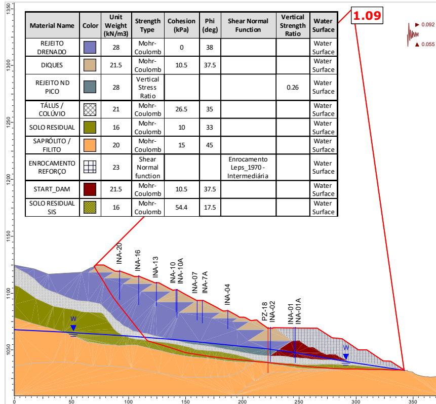
Figura 6.106 – Seção B-B' – Análise Não Drenada – Superfície de ruptura plano-circular otimizada – Freática 30/10/2024 – Razão de resistência não drenada de pico + sismo ↑ (critério CDA).
