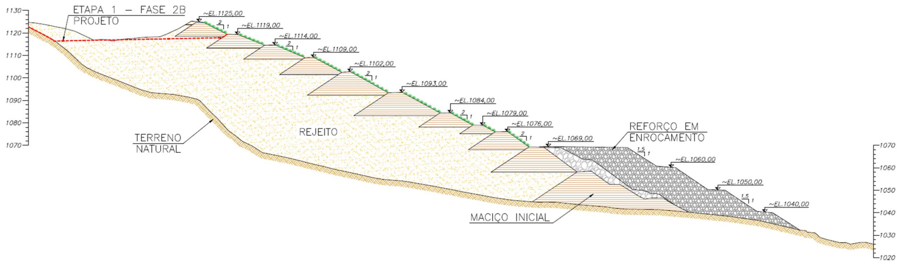
Figura 6.12 – Comparativo Projeto (Etapa 1 - Fase 2B) x Executado – Seção B-B’.
