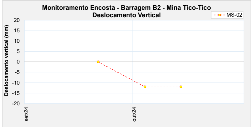
Figura 5.22 - Marco de controle de monitoramento da encosta - MS-02.
