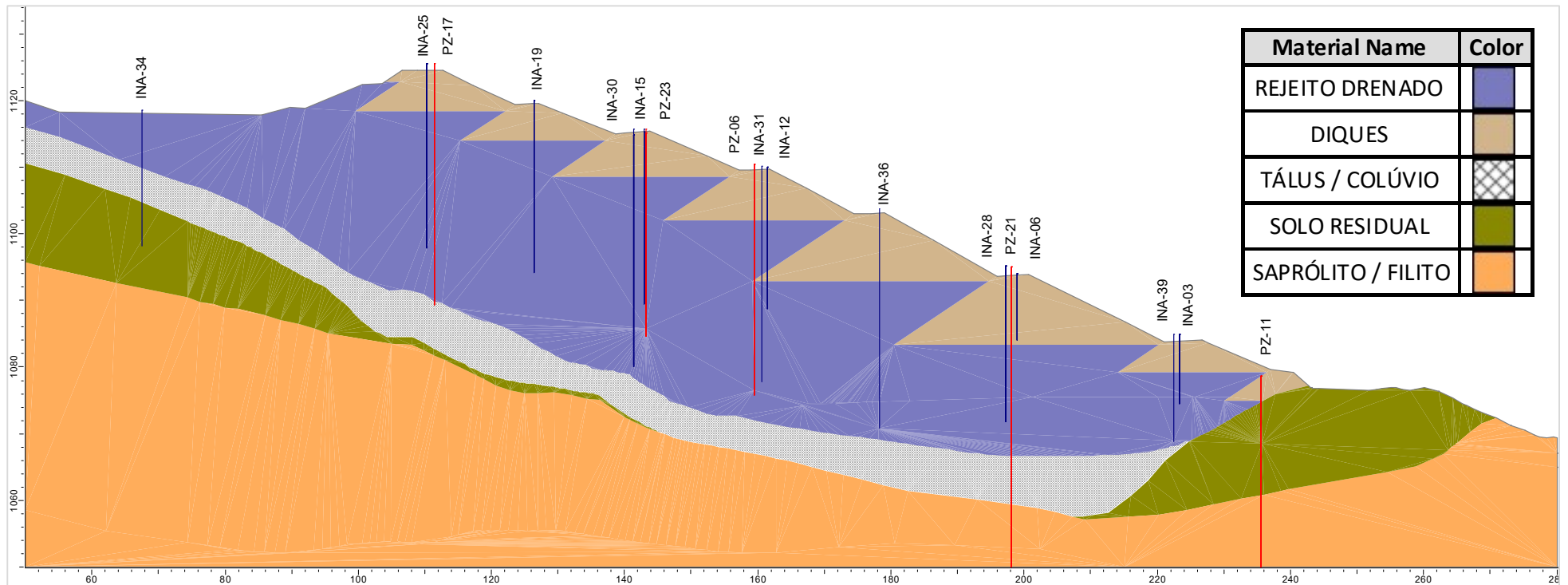
Figura 6.20 – Seção transversal de controle A-A' (Condição em 31/10/2024).
