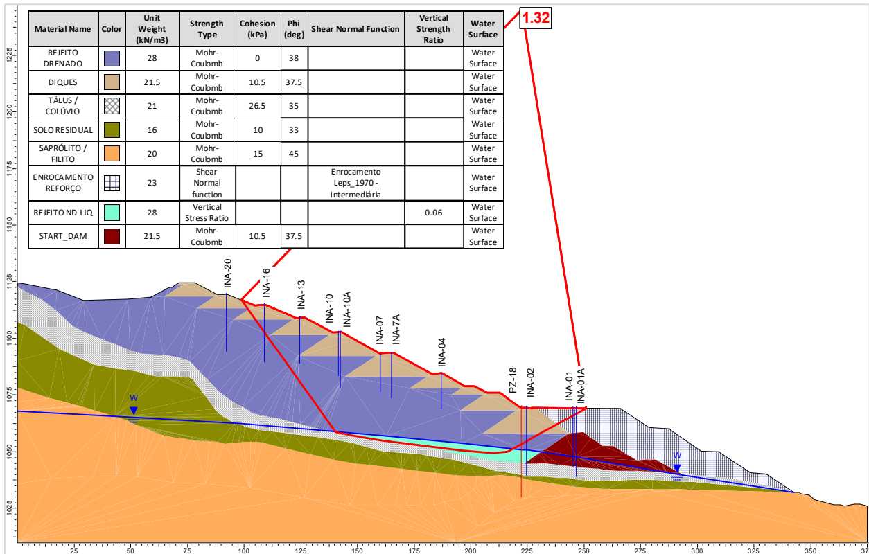
Figura 6.105 – Seção B-B' – Análise Não Drenada – Superfície de ruptura plano-circular otimizada – Freática 30/10/2024 – Razão de resistência não drenada liquefeita.
