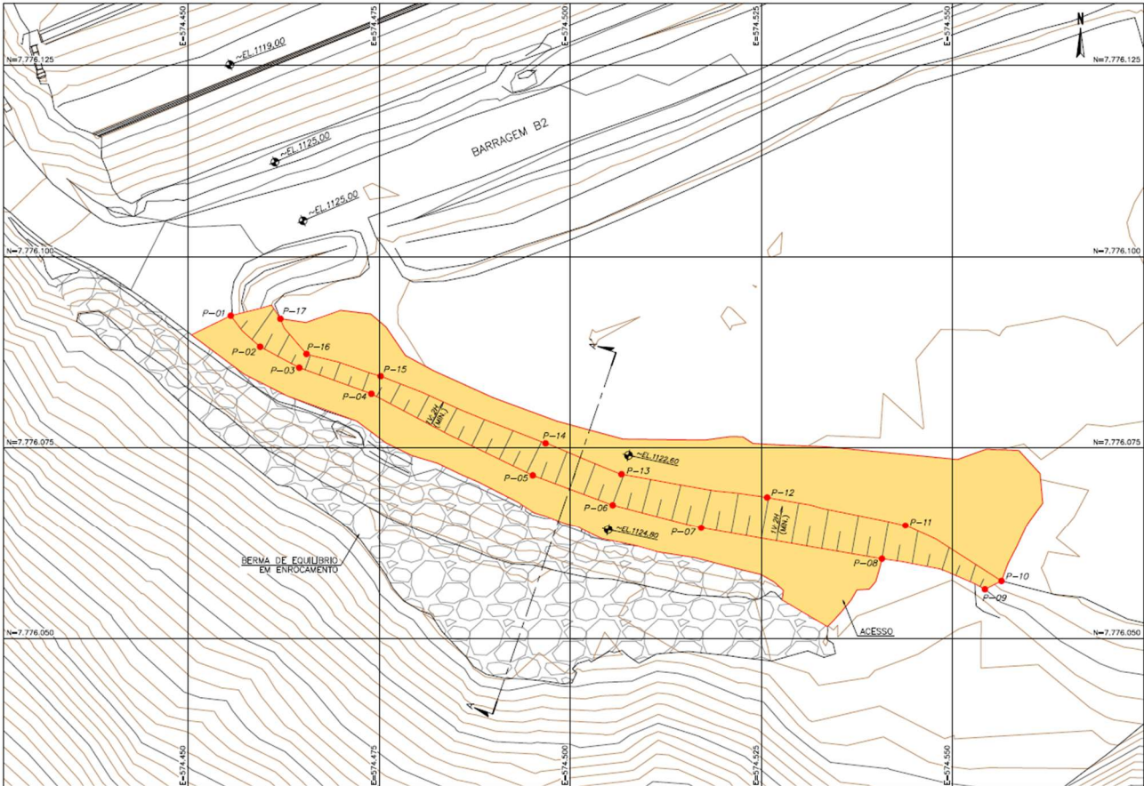
Figura 5.10 – Limites escavação próximo à berma de equilíbrio - Planta (Fonte: IPE.OP.DE.8000.GT.20.1012).
