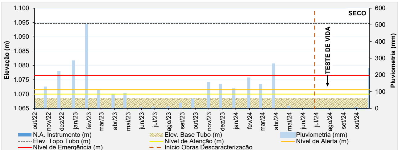
Figura 6.48 – Desempenho do indicador de nível d'água – INA-27.
