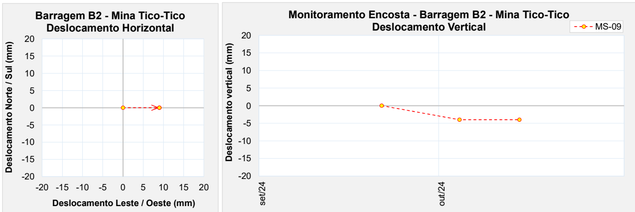
Figura 5.29 – Marco de controle de monitoramento da encosta – MS-09.
