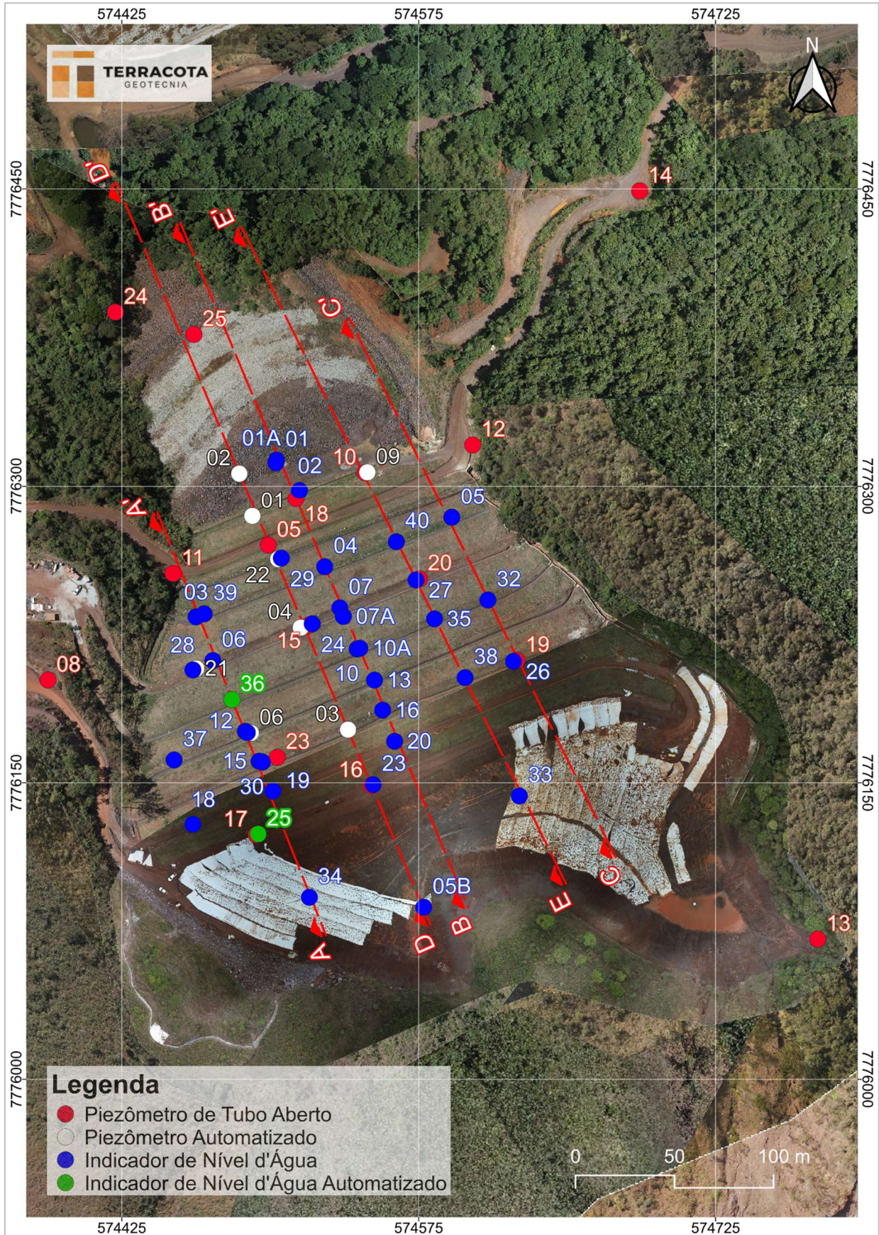
Figura 6.93 – Seções Instrumentadas Barragem B2 – Mina Tico-Tico – Planta.
