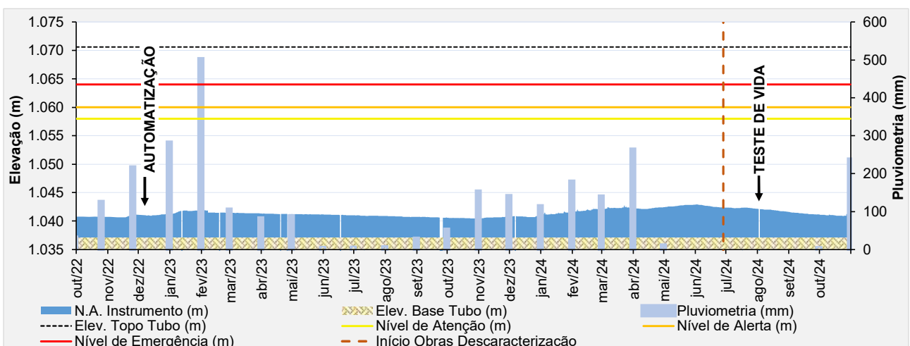
Figura 6.70 – Desempenho do piezômetro automatizado – PZ-09.
