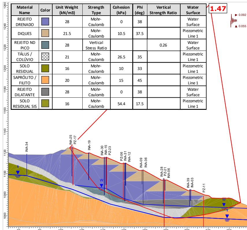
Figura 6.99 – Seção A-A' – Análise Não Drenada – Superfície de ruptura plano-circular otimizada – Freática 30/10/2024 – Razão de resistência não drenada de pico + sismo ↑ (critério CDA).
