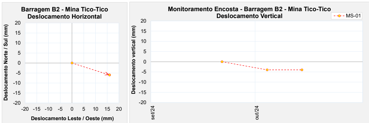
Figura 5.21 – Marco de controle de monitoramento da encosta – MS-01.
