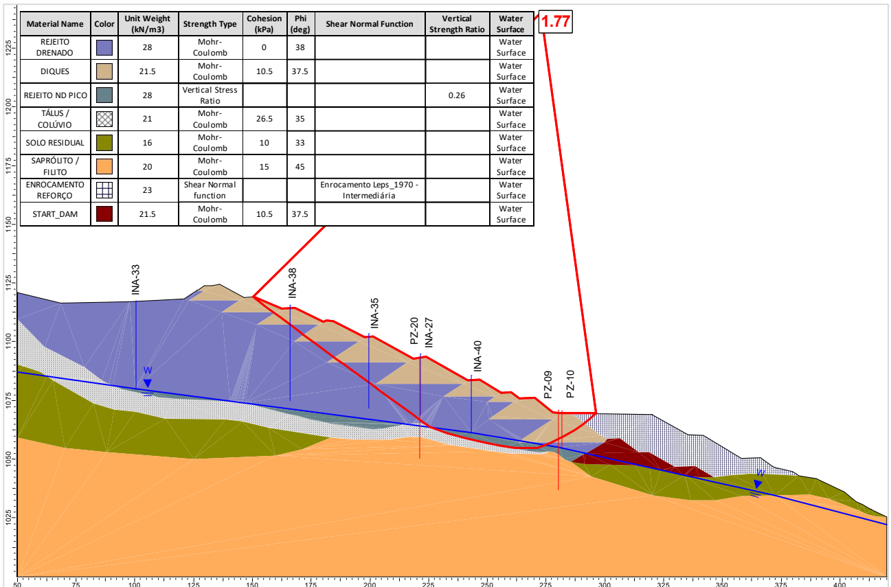
Figura 6.123 – Seção E-E' – Análise Não Drenada – Superfície de ruptura plano-circular otimizada – Freática 30/10/2024 – Razão de resistência não drenada de pico.
