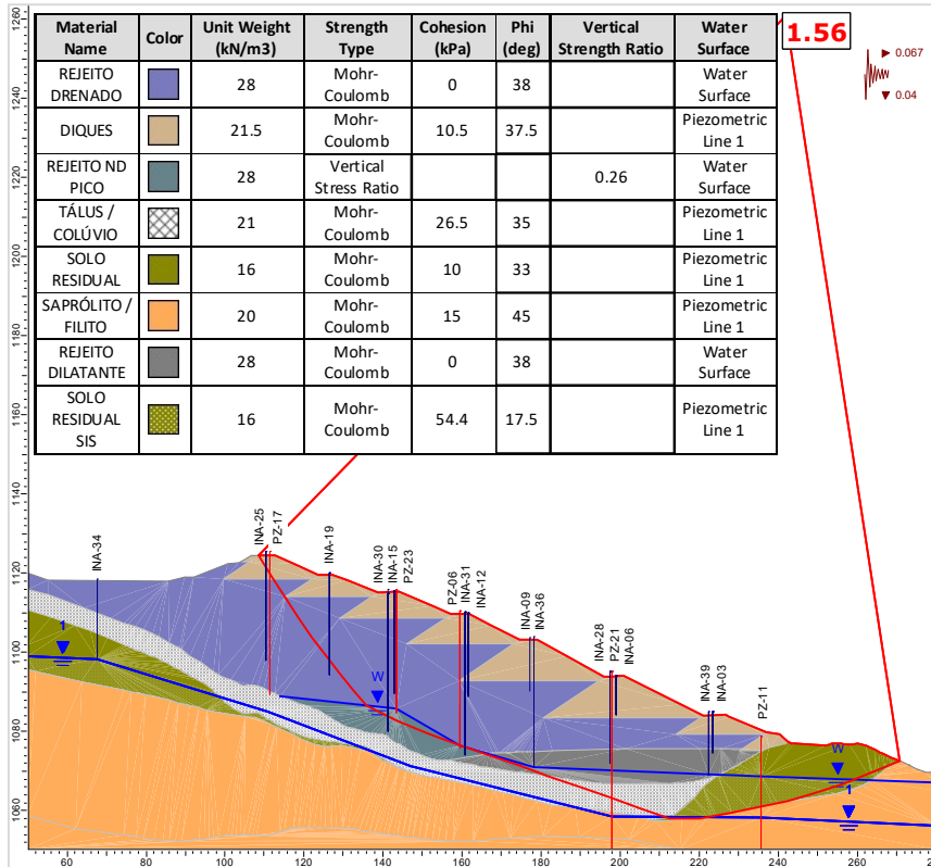
Figura 6.102 – Seção A-A' – Análise Não Drenada – Superfície de ruptura plano-circular otimizada – Freática 30/10/2024 – Razão de resistência não drenada de pico + sismo ↓ (critério vida útil).
