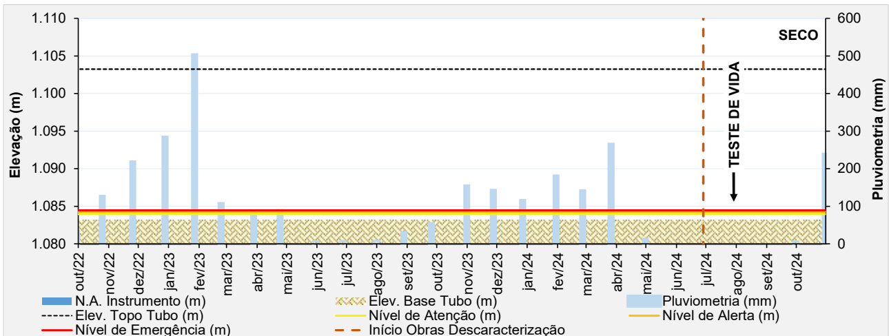
Figura 6.36 – Desempenho do indicador de nível d'água – INA-10A.
