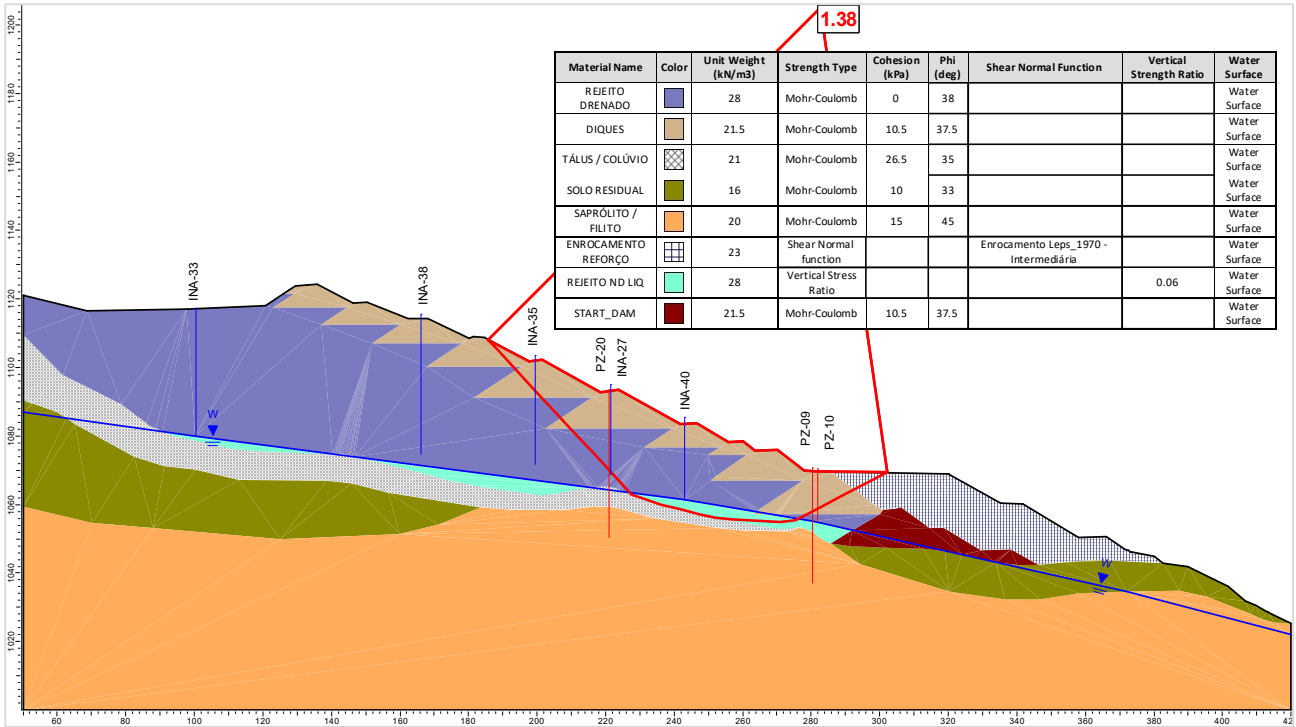
Figura 6.124 – Seção E-E' – Análise Não Drenada – Superfície de ruptura plano-circular otimizada – Freática 30/10/2024 – Razão de resistência não drenada liquefeita.
