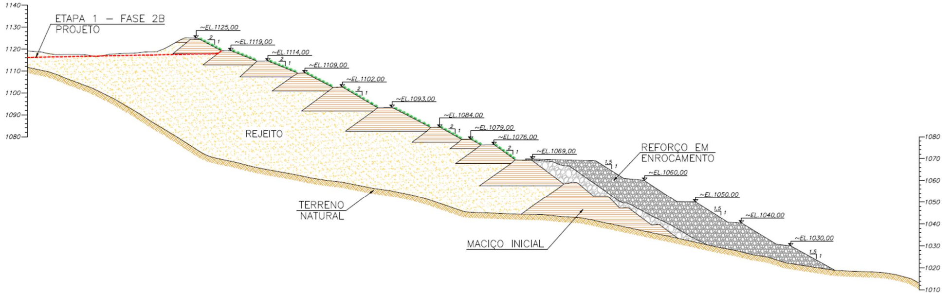
Figura 6.14 – Comparativo Projeto (Etapa 1 - Fase 2B) x Executado – Seção D-D’.
