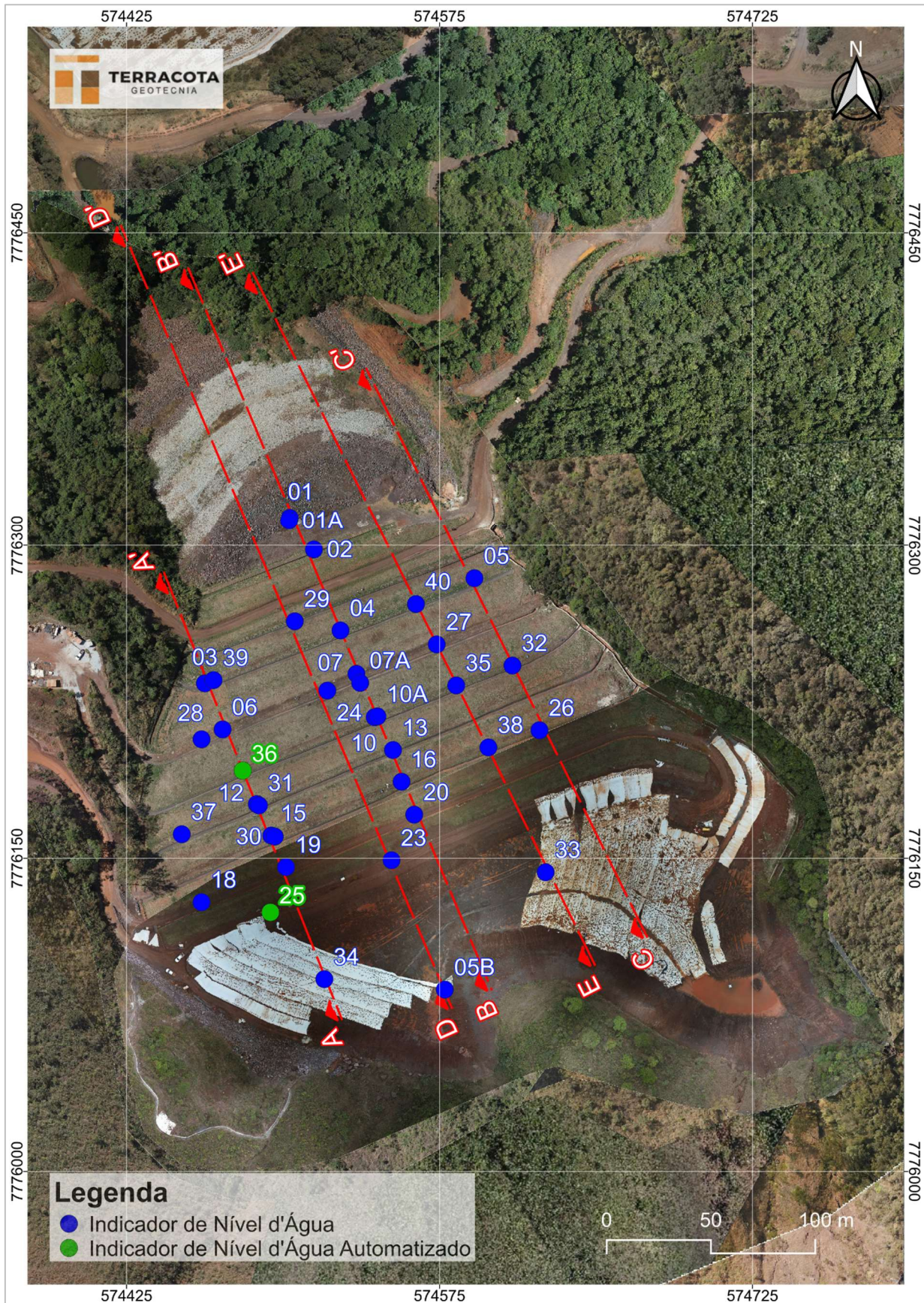
Figura 6.17 – Localização dos indicadores de nível d'água.
