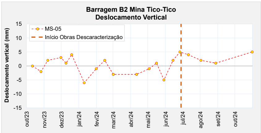
Figura 6.92 – Marco de controle de deformação – MS-05.
