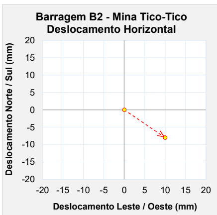
Figura 5.26 – Marco de controle de monitoramento da encosta – MS-06.
