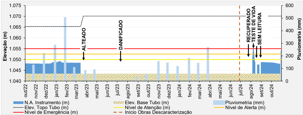
Figura 6.26 – Desempenho do indicador de nível d'água - INA-01A.
