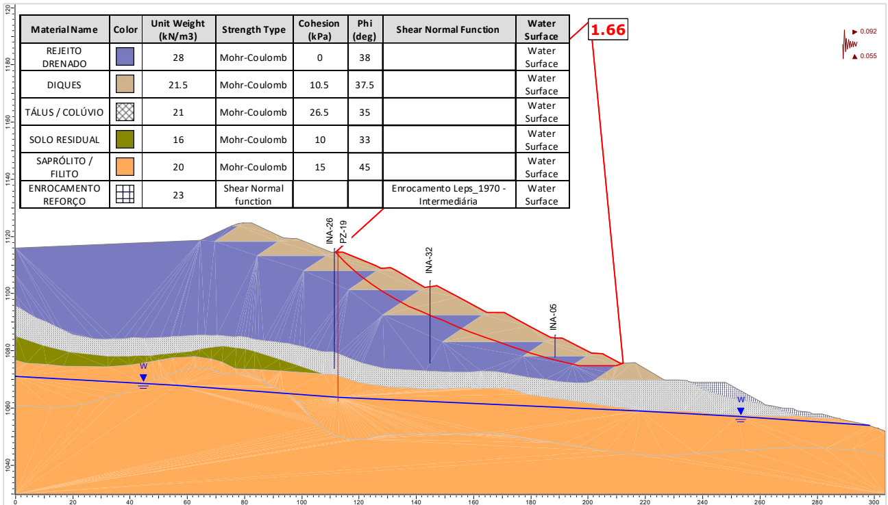
Figura 6.111 – Seção C-C' – Análise Drenada – Superfície de ruptura plano-circular otimizada – Freática 30/10/2024 – Carregamento sísmico ↑ (critério CDA).
