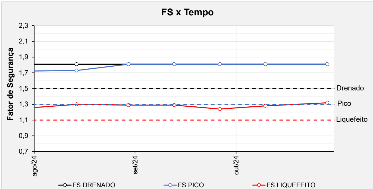
Figura 6.130 – Seção B-B' - Histórico dos F.S. obtidos nas análises de estabilidade no período avaliado.
