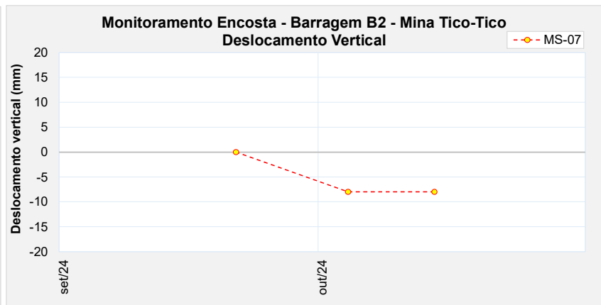
Figura 5.27 – Marco de controle de monitoramento da encosta – MS-07.
