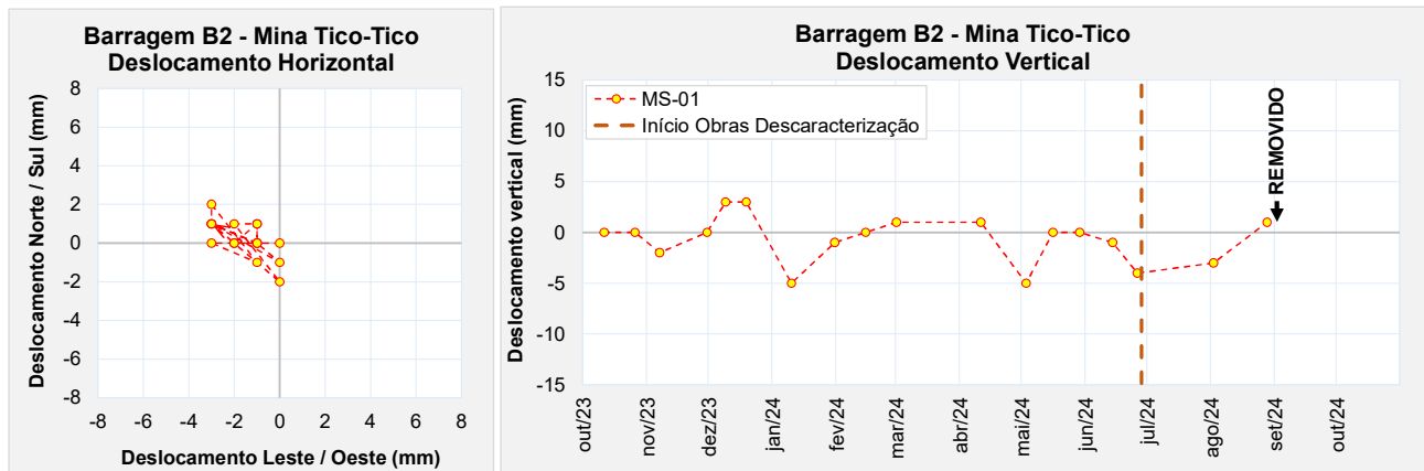
Figura 6.88 – Marco de controle de deformação – MS-01.
