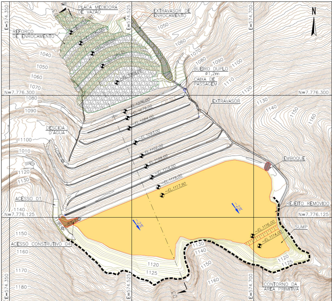
Figura 6.5 – Sequência Construtiva – Planta – Etapa 1-Fase 2B (IPE.OP.DE.8000.GT.20.746).
