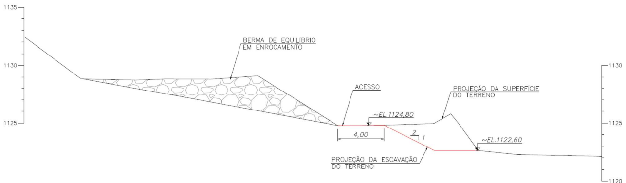
Figura 5.11 – Limites escavação próximo à berma de equilíbrio - Seção Transversal (Fonte: IPE.OP.DE.8000.GT.20.1011).
