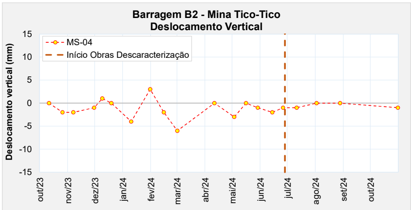
Figura 6.91 – Marco de controle de deformação – MS-04.
