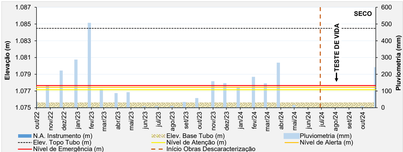
Figura 6.30 – Desempenho do indicador de nível d'água – INA-05.
