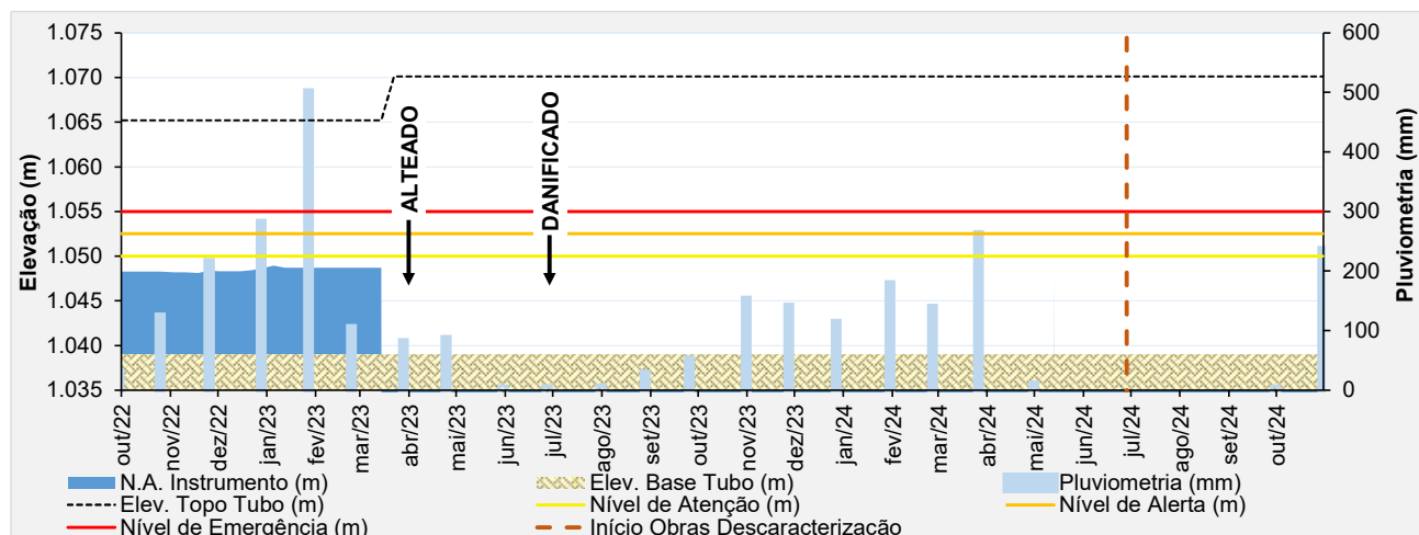
Figura 6.25 – Desempenho do indicador de nível d'água – INA-01 (Danificado).
