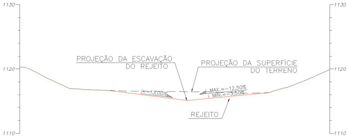
Figura 5.16 – Canal central do reservatório – Seção Transversal (Fonte: IPE.OP.DE.8000.GT.20.1026).
