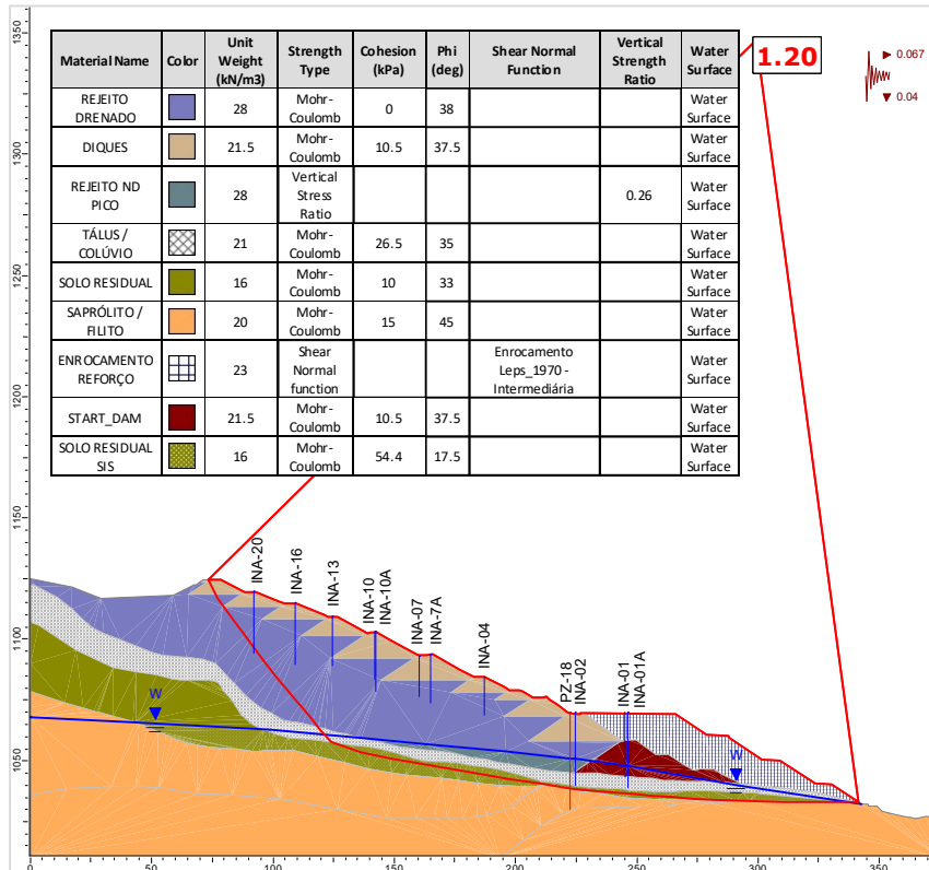
Figura 6.109 – Seção B-B' – Análise Não Drenada – Superfície de ruptura plano-circular otimizada – Freática 30/10/2024 – Razão de resistência não drenada de pico + sismo ↓ (critério vida útil).
