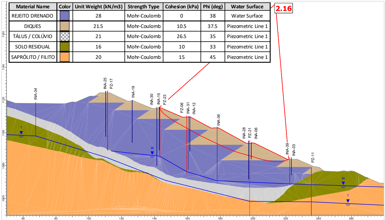
Figura 6.96 – Seção A-A' – Análise Drenada – Superfície de ruptura plano-circular otimizada – Freática 30/10/2024.
