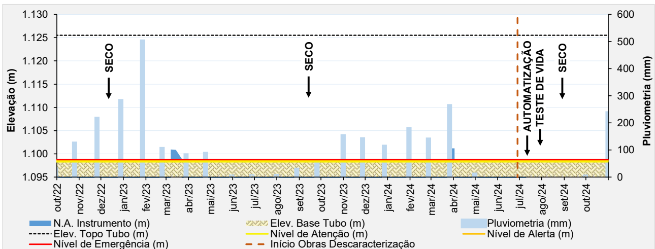
Figura 6.46 – Desempenho do indicador de nível d'água automatizado – INA-25.
