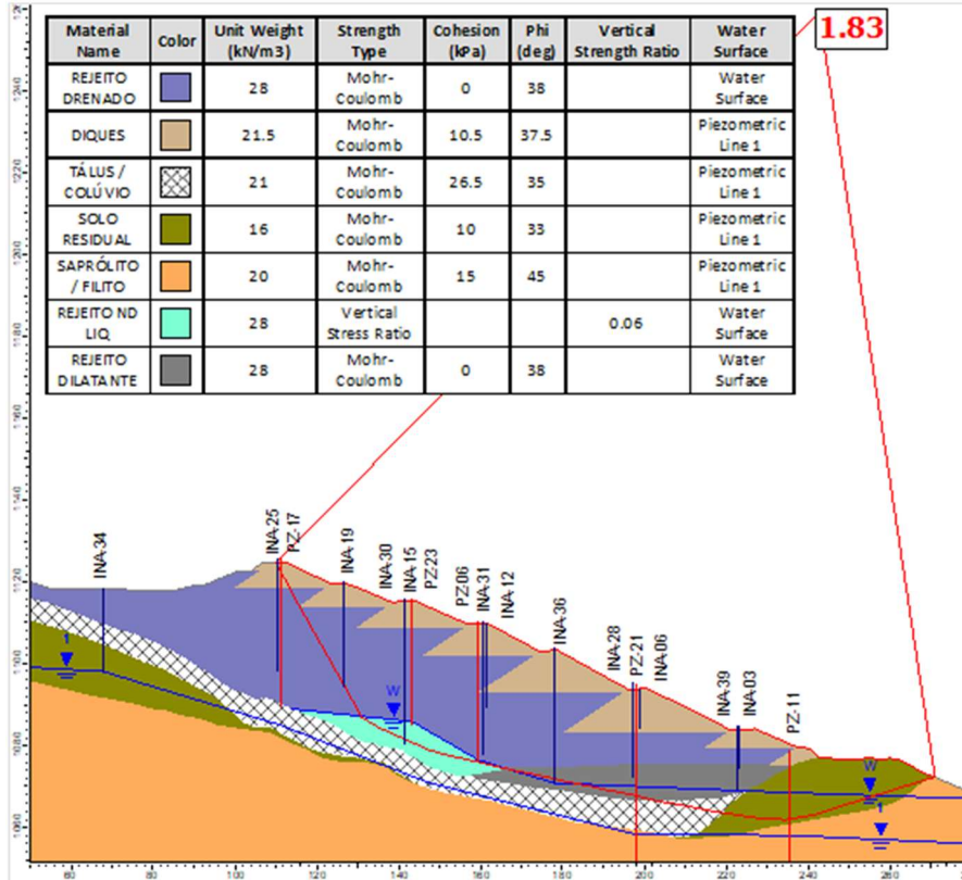
Figura 6.98 – Seção A-A' – Análise Não Drenada – Superfície de ruptura plano-circular otimizada – Freática 30/10/2024 – Razão de resistência não drenada liquefeita.
