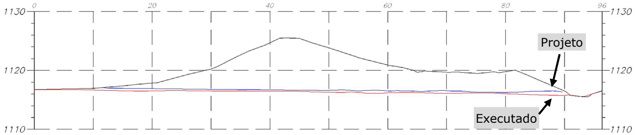
Figura 6.3 – Comparação entre a declividade do eixo do canal executado e de projeto – Seção Longitudinal. (Fonte: IPE.OP.DE.8000.GT.20.1055).
