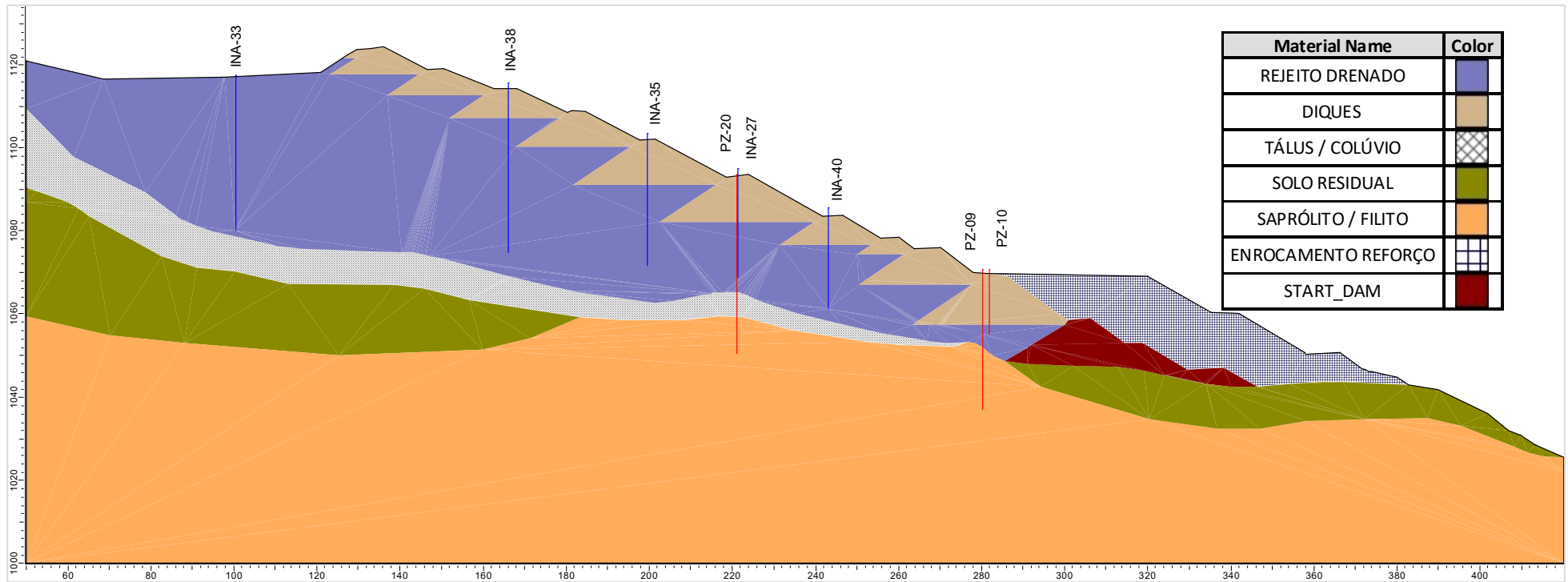
Figura 6.24 – Seção transversal de controle E-E' (Condição em 31/10/2024).
