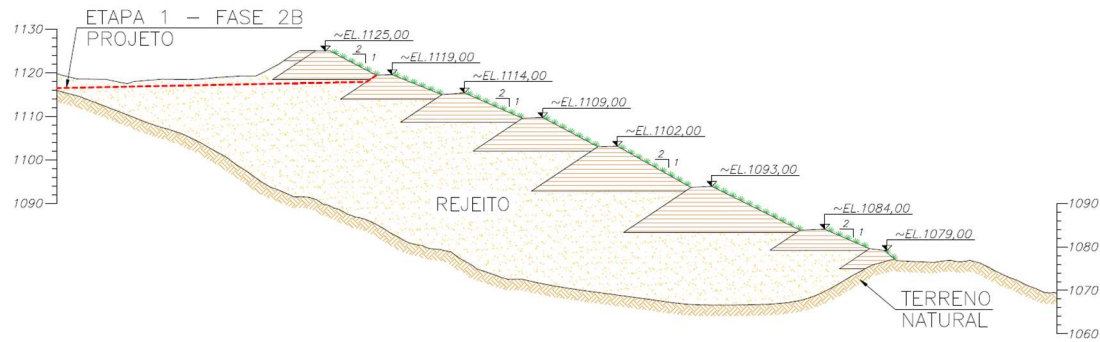
Figura 6.11 – Comparativo Projeto (Etapa 1 - Fase 2B) x Executado – Seção A-A’.
