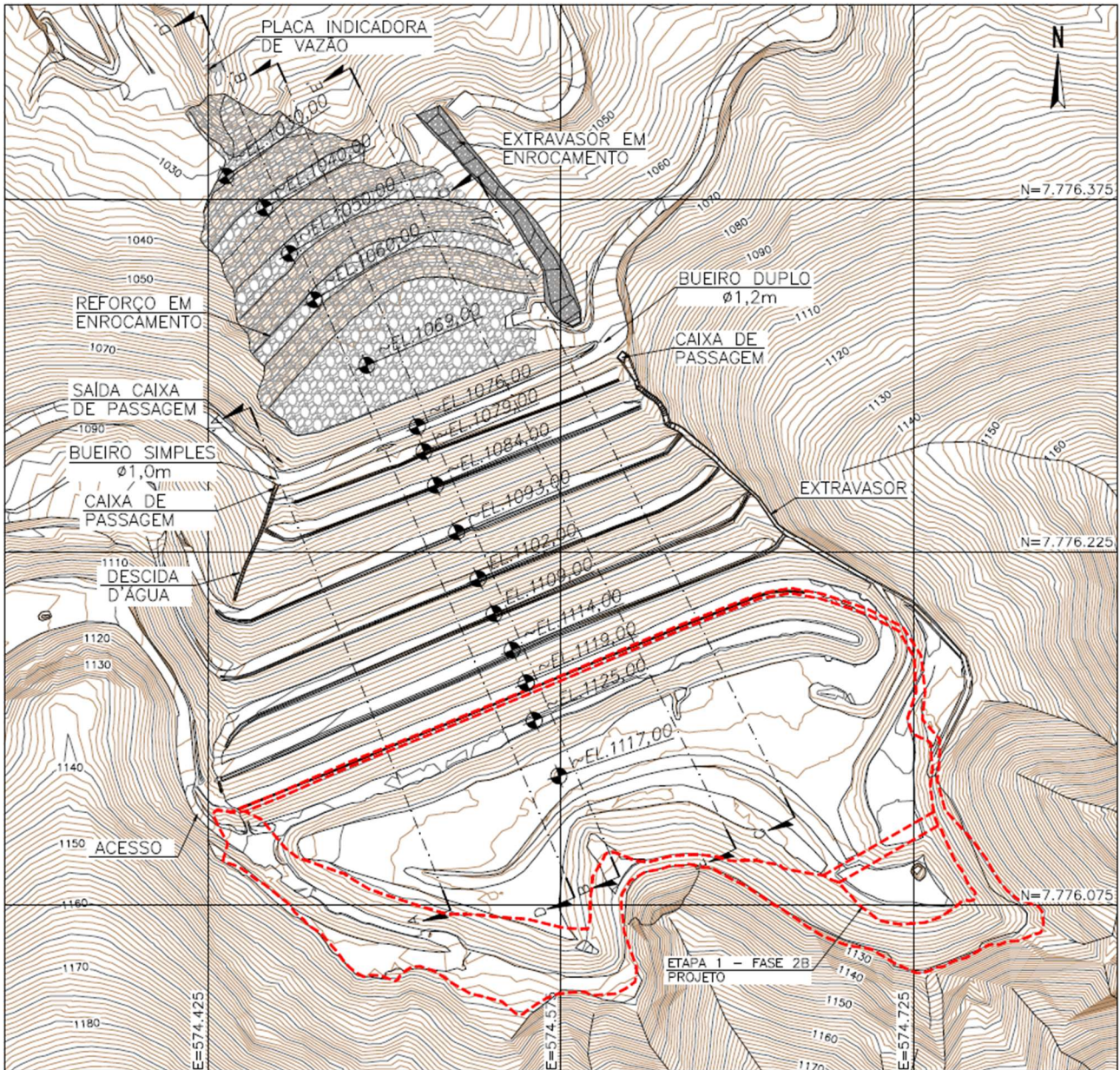
Figura 6.10 – Comparativo Projeto (Etapa 1 - Fase 2B) x Executado – Planta.
