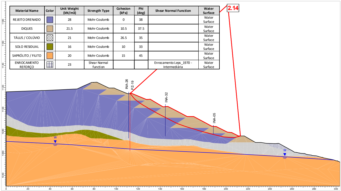
Figura 6.110 – Seção C-C' – Análise Drenada – Superfície de ruptura plano-circular otimizada – Freática 30/10/2024.
