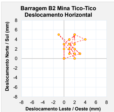
Figura 6.92 – Marco de controle de deformação – MS-05.
