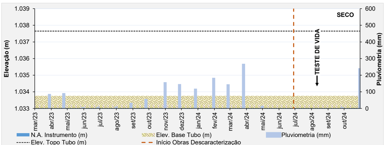
Figura 6.85 – Desempenho do piezômetro de tubo aberto – PZ-24.
