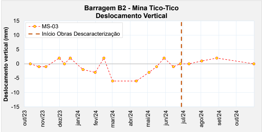
Figura 6.90 – Marco de controle de deformação – MS-03.
