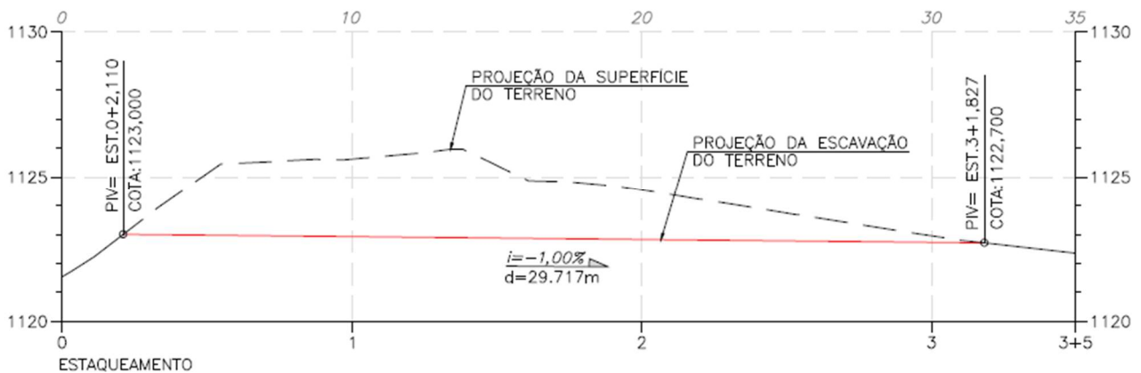
Figura 5.8 – Canal de conexão com extravasor de emergência (Etapa 1 – Fase 1) – Seção Longitudinal (Fonte: IPE.OP.DE.8000.GT.20.1011).
