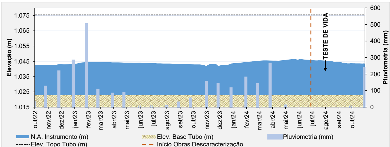
Figura 6.73 – Desempenho do piezômetro de tubo aberto – PZ-12.
