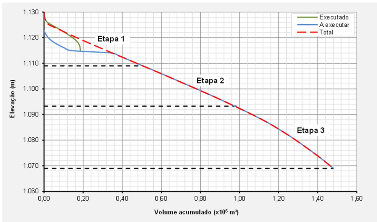
Figura 6.16 – Curva elevação-volume – Comparativo andamento das obras.
