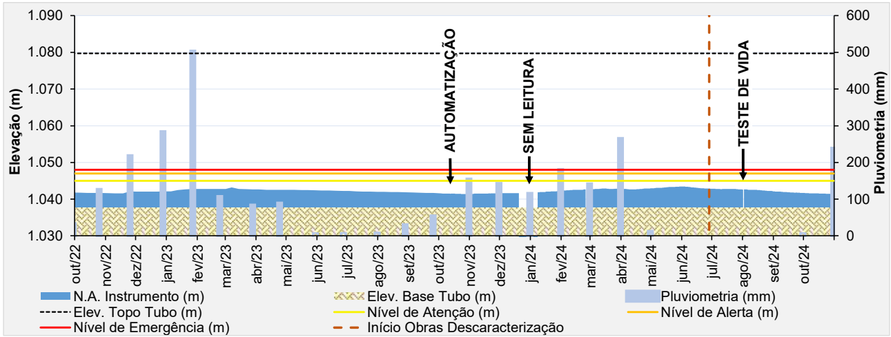
Figura 6.83 – Desempenho do piezômetro automatizado – PZ-22.
