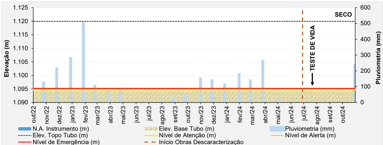
Figura 6.42 - Desempenho do indicador de nível d'água - INA-19.
