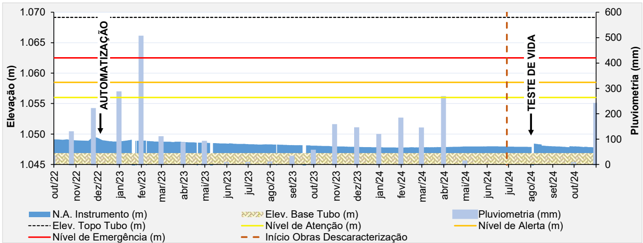
Figura 6.62 – Desempenho do piezômetro automatizado – PZ-01.
