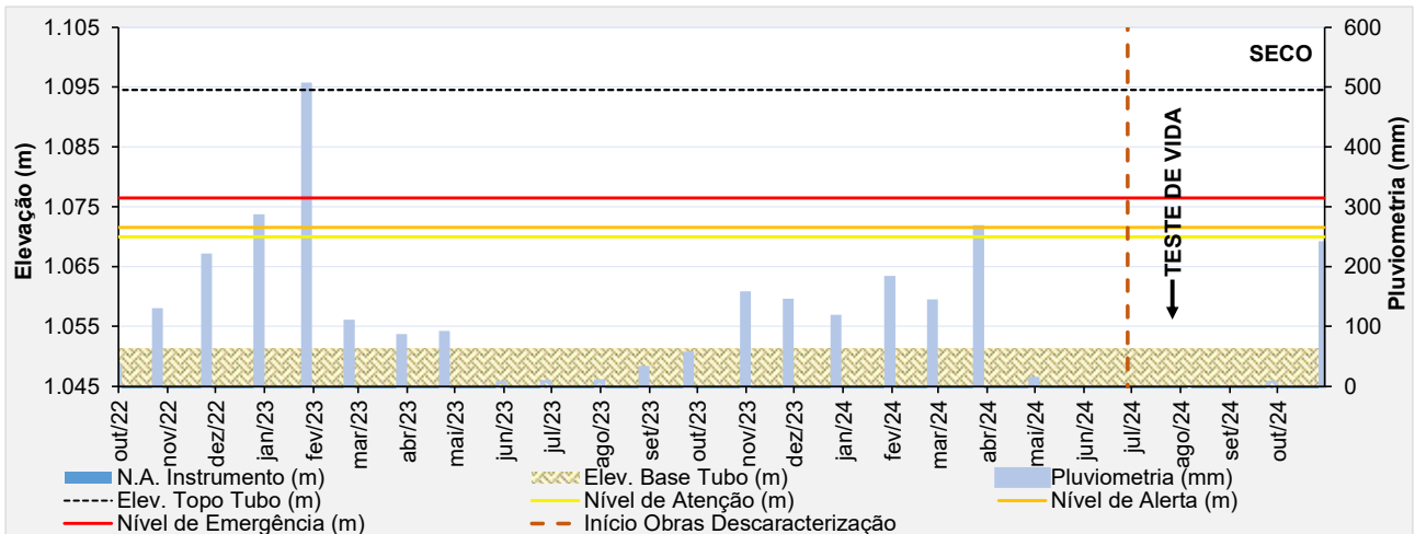
Figura 6.81 – Desempenho do piezômetro de tubo aberto – PZ-20.
