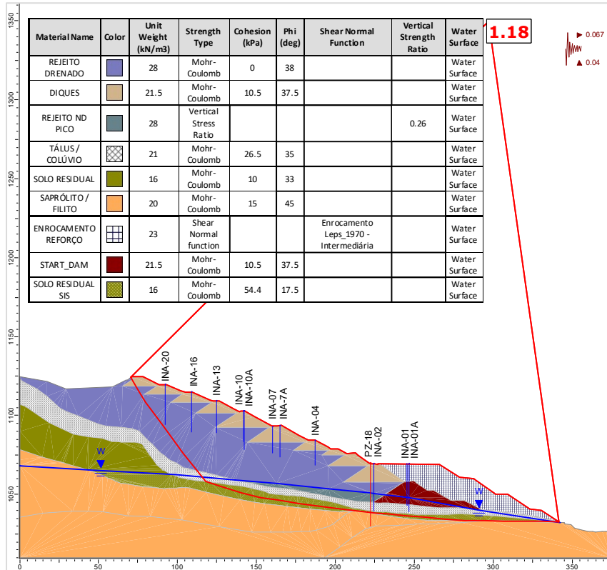
Figura 6.108 – Seção B-B' – Análise Não Drenada – Superfície de ruptura plano-circular otimizada – Freática 30/10/2024 – Razão de resistência não drenada de pico + sismo ↑ (critério vida útil).
