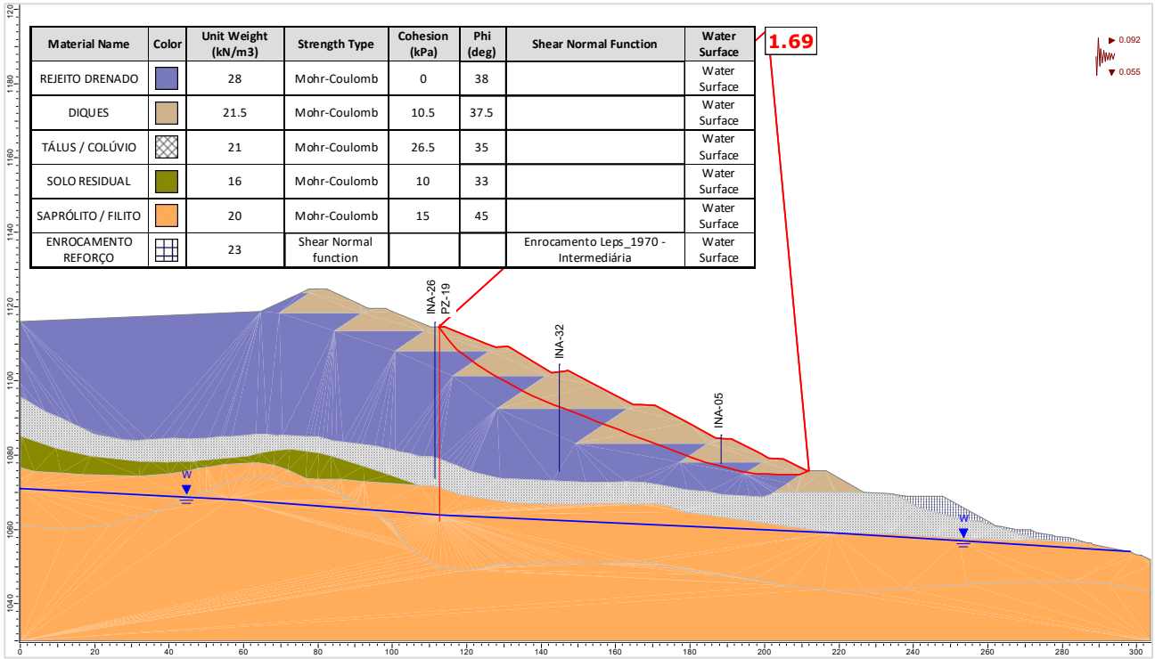
Figura 6.112 – Seção C-C' – Análise Drenada – Superfície de ruptura plano-circular otimizada – Freática 30/10/2024 – Carregamento sísmico ↓ (critério CDA).
