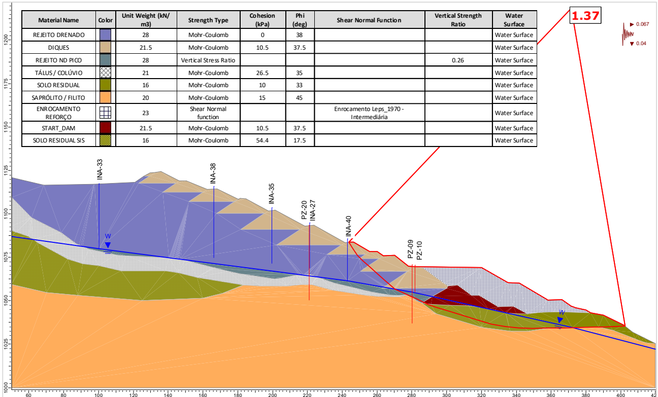
Figura 6.128 – Seção E-E' – Análise Não Drenada – Superfície de ruptura plano-circular otimizada – Freática 30/10/2024 – Razão de resistência não drenada de pico + sismo ↓ (critério vida útil).
