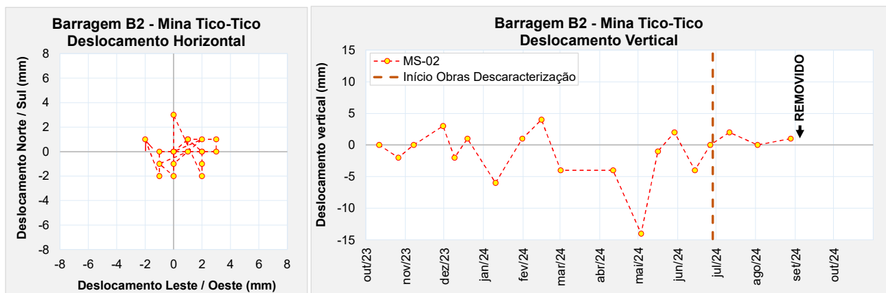
Figura 6.89 – Marco de controle de deformação – MS-02.
