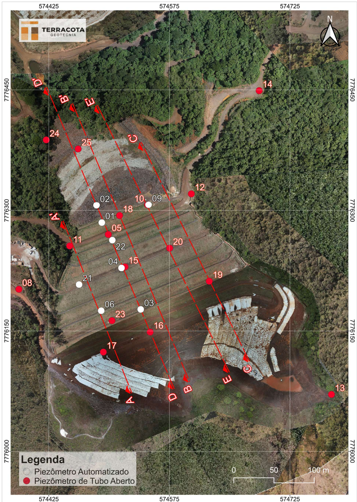
Figura 6.18 - Localização dos piezômetros.
