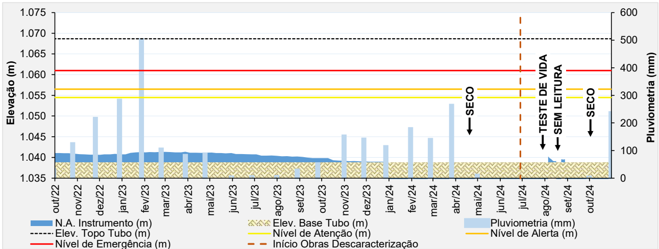
Figura 6.27 – Desempenho do indicador de nível d'água - INA-02.
