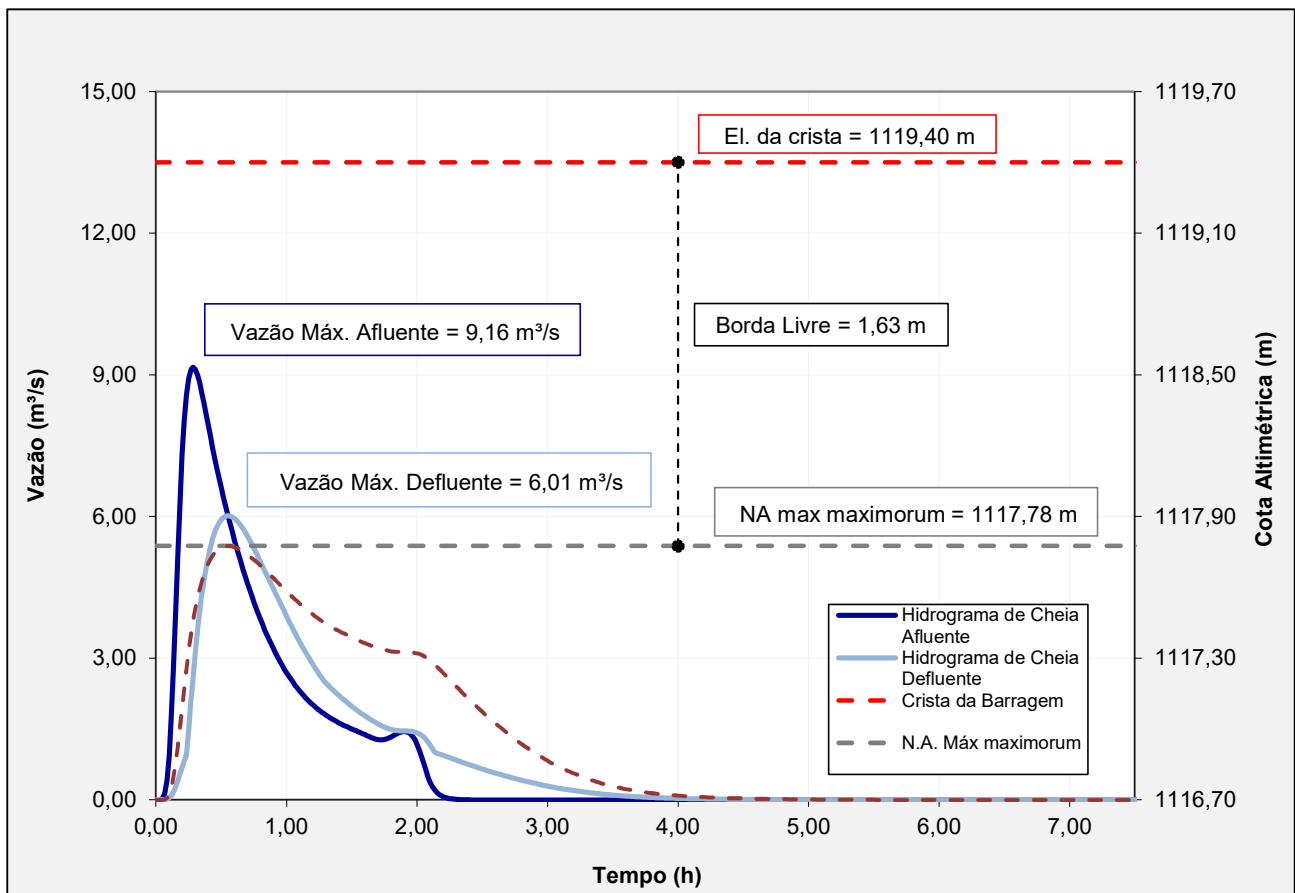
Figura 6.4 – Hidrograma do trânsito de cheias para PMP – 2h.
