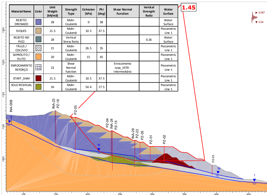
Figura 6.121 – Seção D-D' – Análise Não Drenada – Superfície de ruptura plano-circular otimizada – Freática 30/10/2024 – Razão de resistência não drenada de pico + sismo ↓ (critério vida útil).
