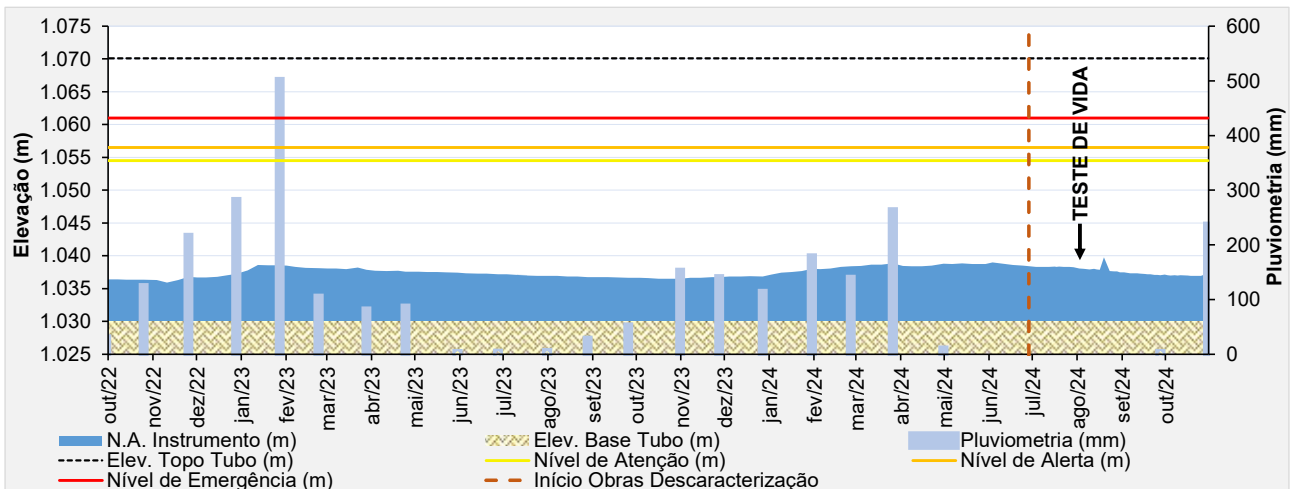
Figura 6.79 – Desempenho do piezômetro de tubo aberto – PZ-18.
