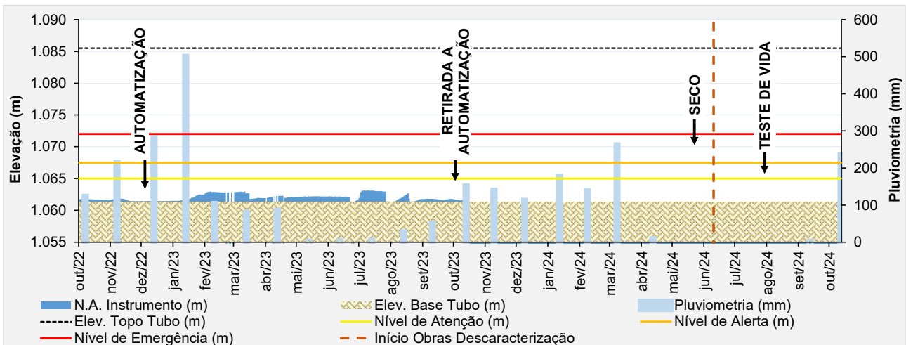
Figura 6.61 – Desempenho do indicador de nível d'água – INA-40.
