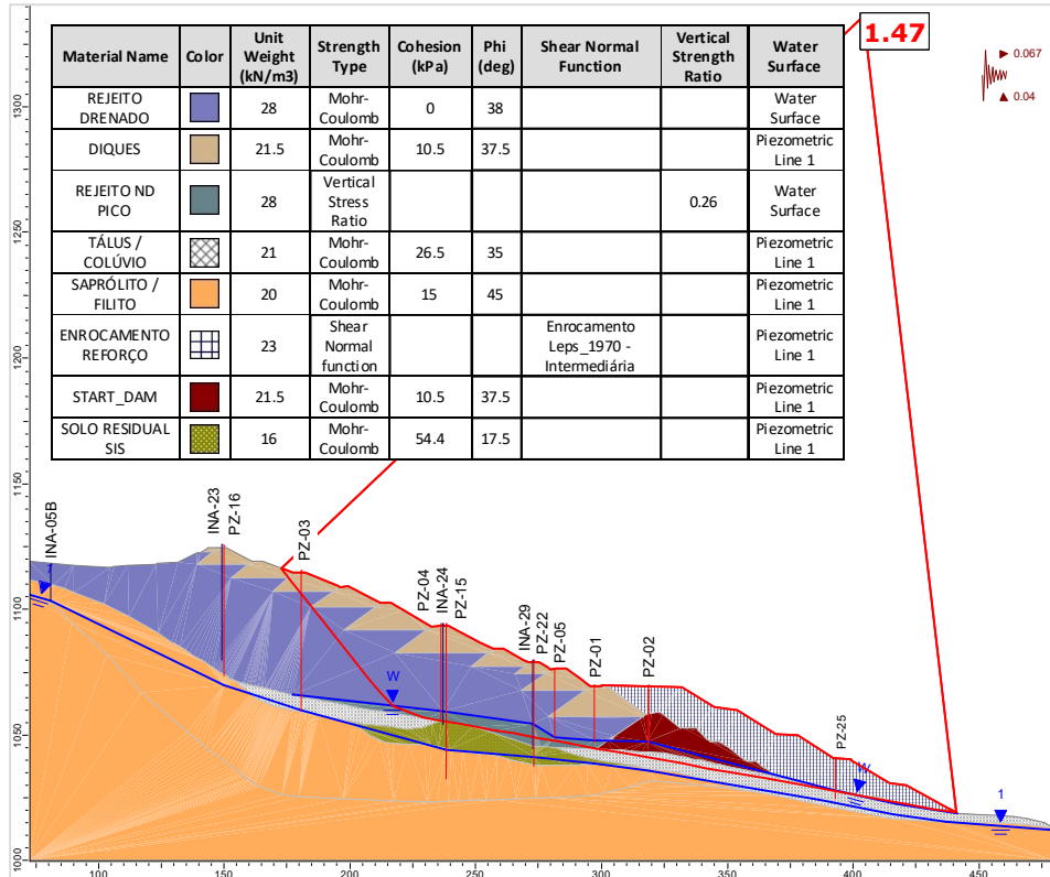
Figura 6.120 – Seção D-D' – Análise Não Drenada – Superfície de ruptura plano-circular otimizada – Freática 30/10/2024 – Razão de resistência não drenada de pico + sismo ↑ (critério vida útil).
