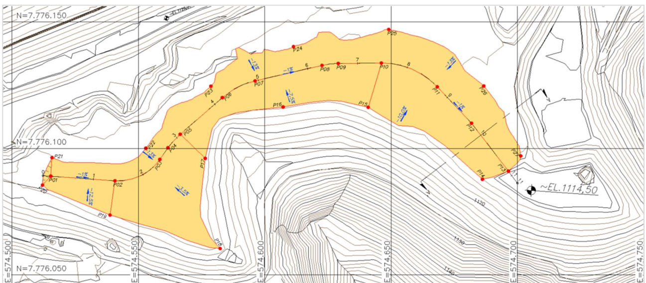
Figura 5.15 – Canal central do reservatório - Planta (Fonte: IPE.OP.DE.8000.GT.20.1026).
