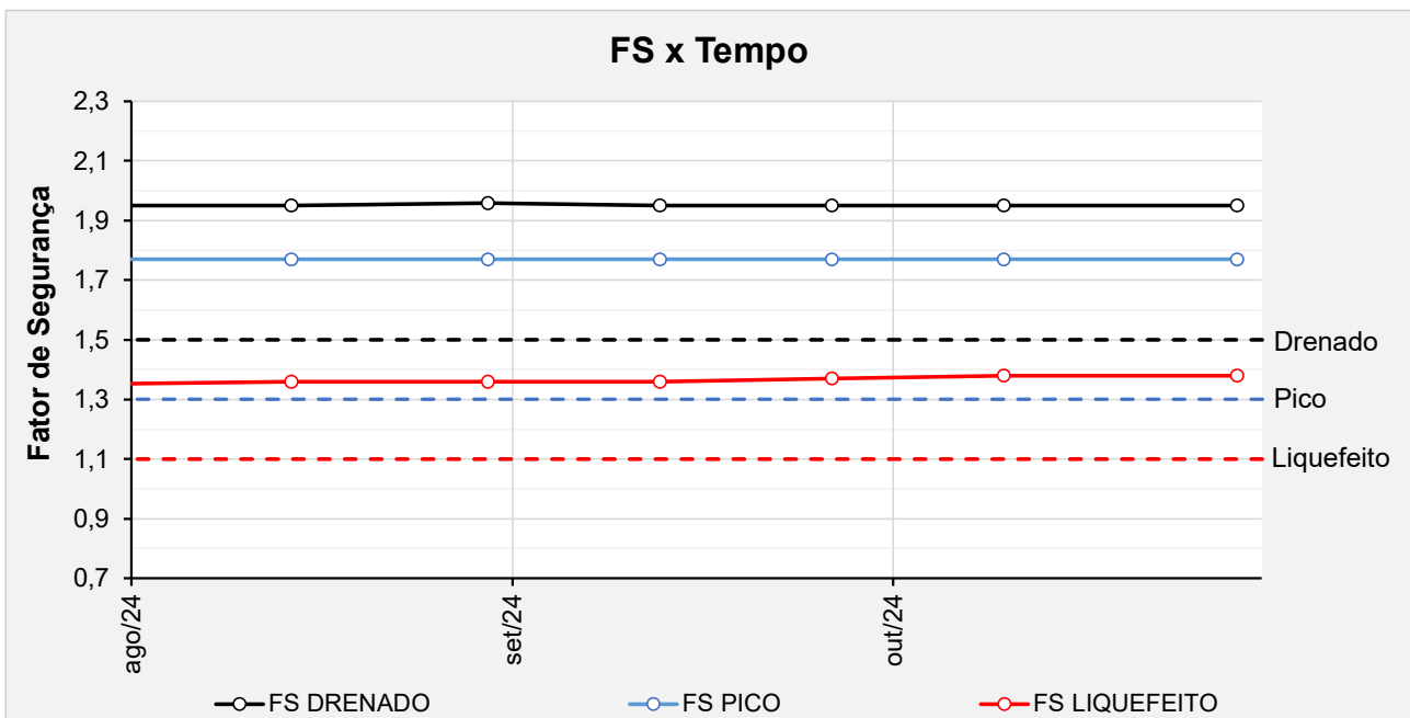
Figura 6.133 – Seção E-E' - Histórico dos F.S. obtidos nas análises de estabilidade no período avaliado.
