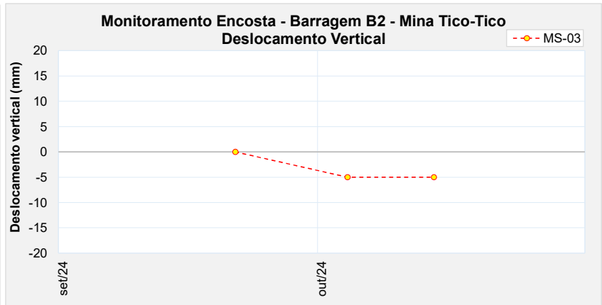
Figura 5.23 - Marco de controle de monitoramento da encosta - MS-03.
