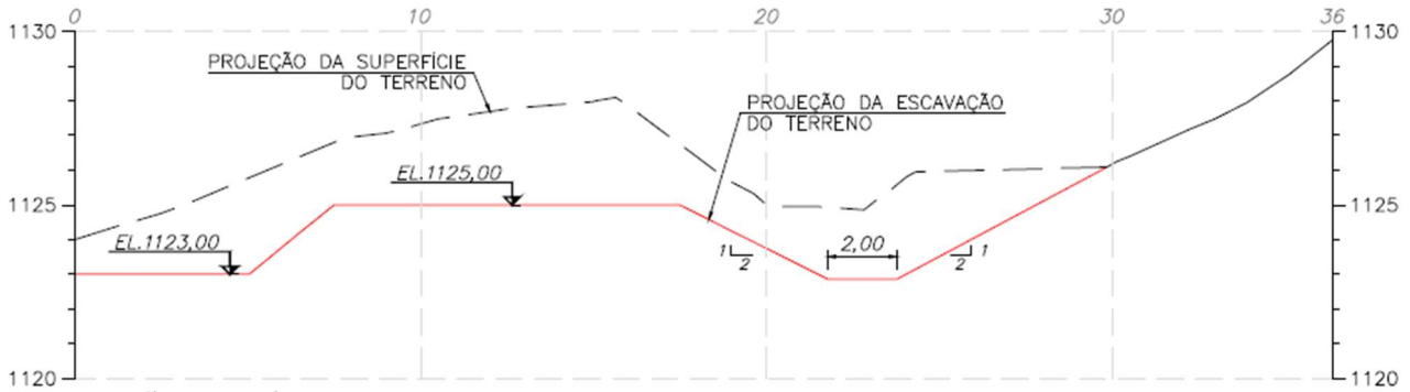
Figura 5.9 - Canal de conexão com extravasor de emergência (Etapa 1 - Fase 1) - Seção Transversal (Fonte: IPE.OP.DE.8000.GT.20.1011).
