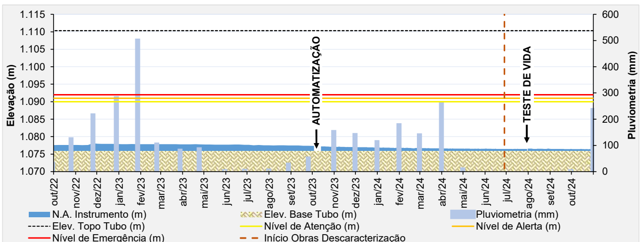
Figura 6.67 – Desempenho do piezômetro automatizado – PZ-06.
