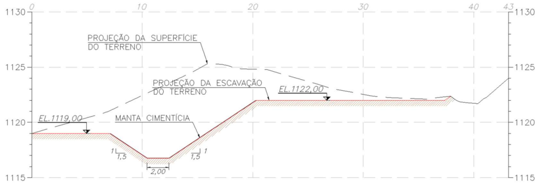
Figura 5.14 – Canal de conexão com extravasor de emergência (Etapa 1 – Fase 2) – Seção Transversal (Fonte: IPE.OP.DE.8000.GT.20.1013).
