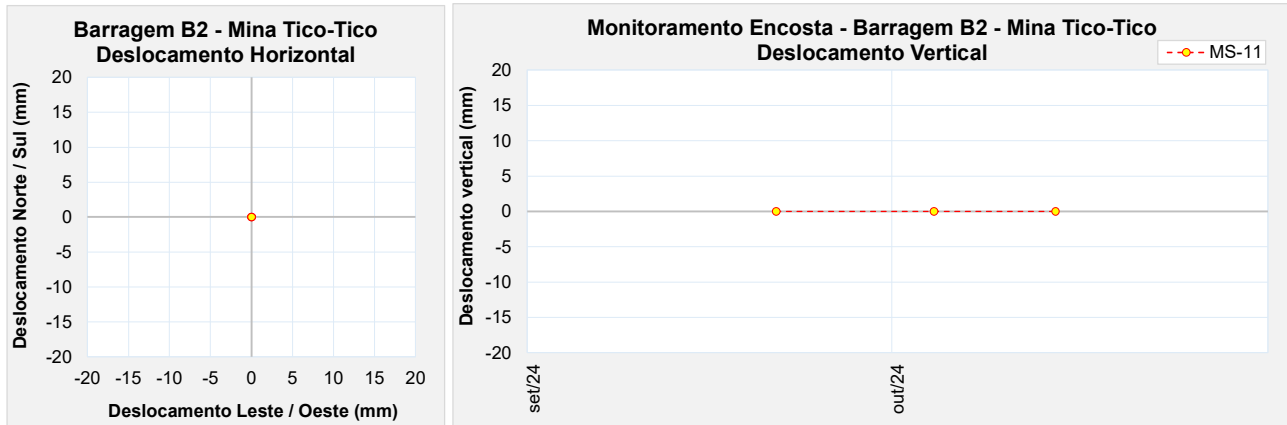
Figura 5.31 – Marco de controle de monitoramento da encosta – MS-11.
