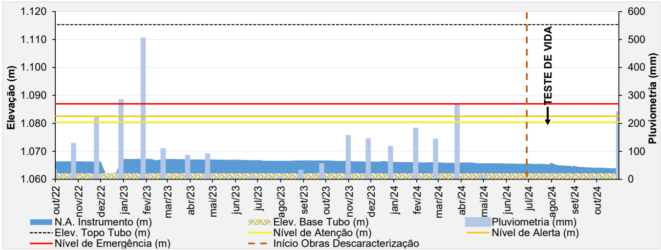
Figura 6.80 – Desempenho do piezômetro de tubo aberto – PZ-19.
