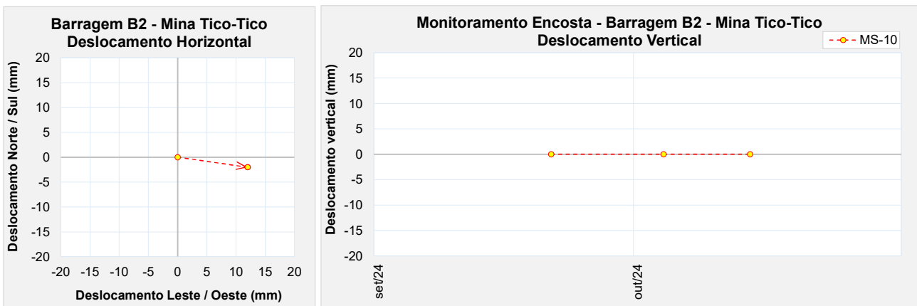
Figura 5.30 – Marco de controle de monitoramento da encosta – MS-10.
