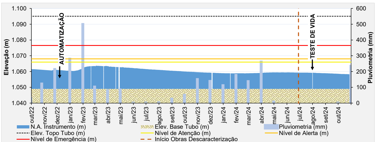
Figura 6.82 – Desempenho do piezômetro automatizado – PZ-21.
