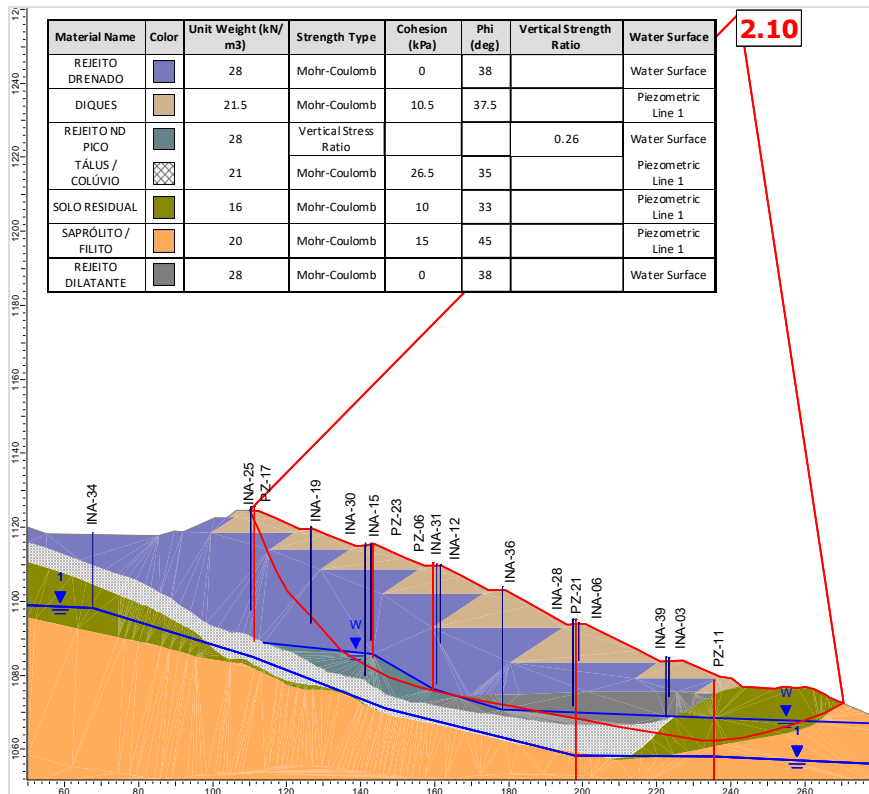
Figura 6.97 – Seção A-A' – Análise Não Drenada – Superfície de ruptura plano-circular otimizada – Freática 30/10/2024 – Razão de resistência não drenada de pico.
