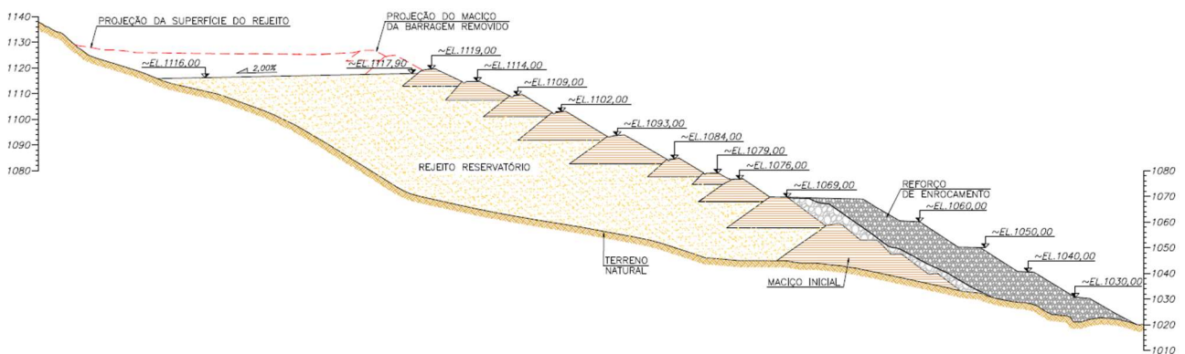
Figura 6.6 – Sequência Construtiva – Seção D-D' – Etapa 1 - Fase 2B.
