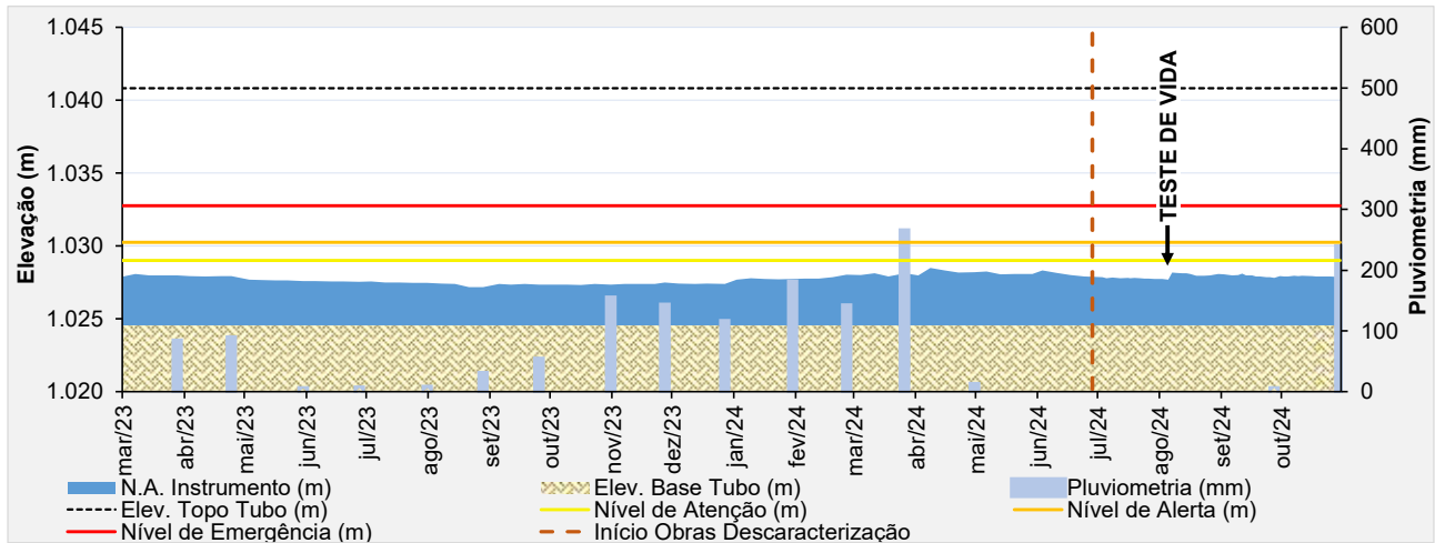
Figura 6.86 – Desempenho do piezômetro de tubo aberto – PZ-25.
