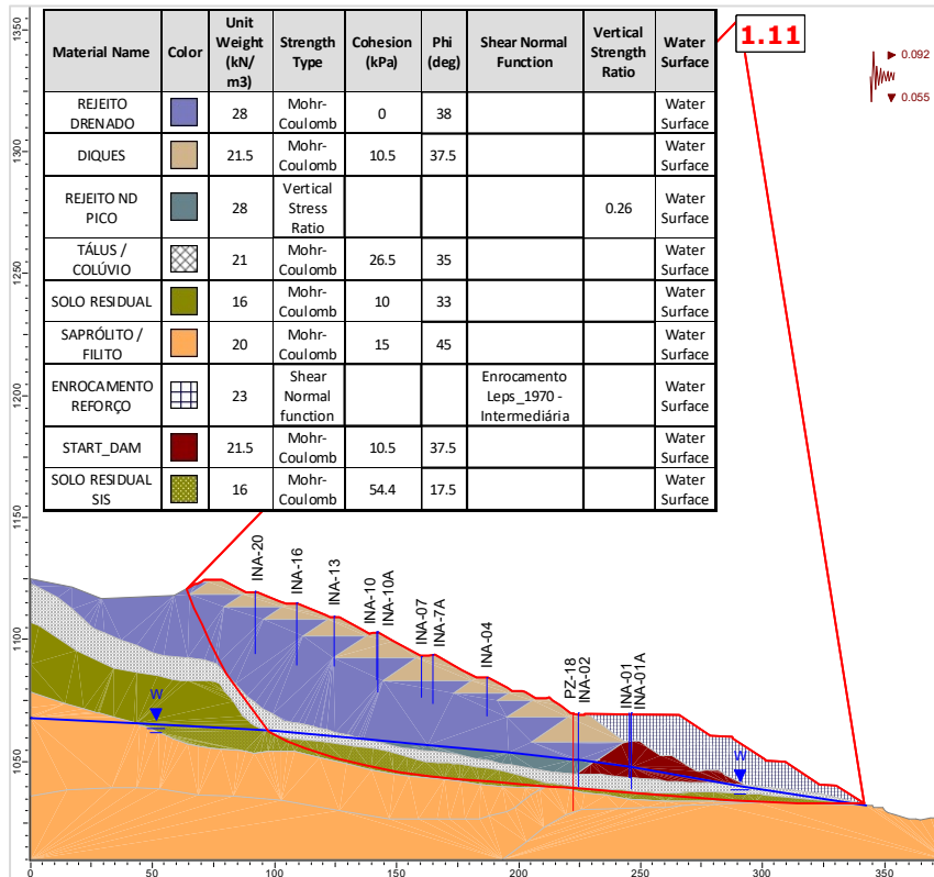
Figura 6.107 – Seção B-B' – Análise Não Drenada – Superfície de ruptura plano-circular otimizada – Freática 30/10/2024 – Razão de resistência não drenada de pico + sismo ↓ (critério CDA).
