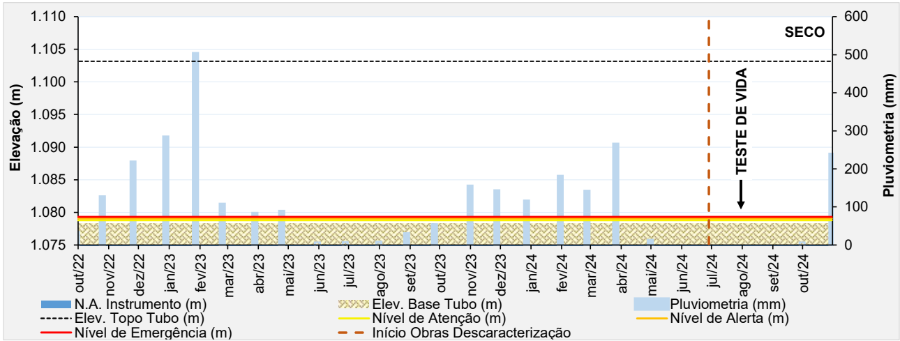
Figura 6.35 – Desempenho do indicador de nível d'água – INA-10.
