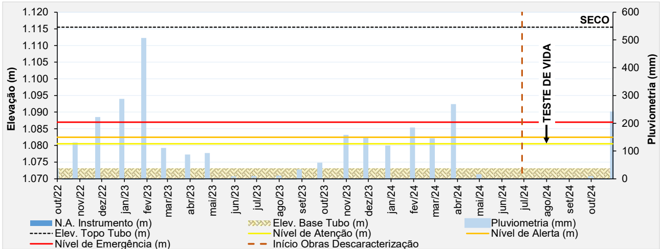
Figura 6.47 – Desempenho do indicador de nível d'água – INA-26.
