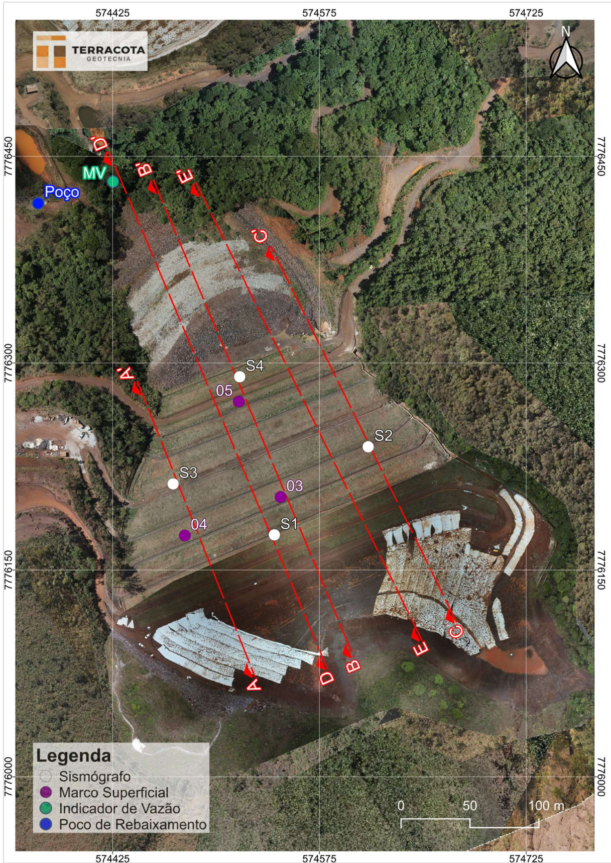
Figura 6.19 – Localização dos marcos superficiais, sismógrafos, indicador de vazão e poço de rebaixamento.
