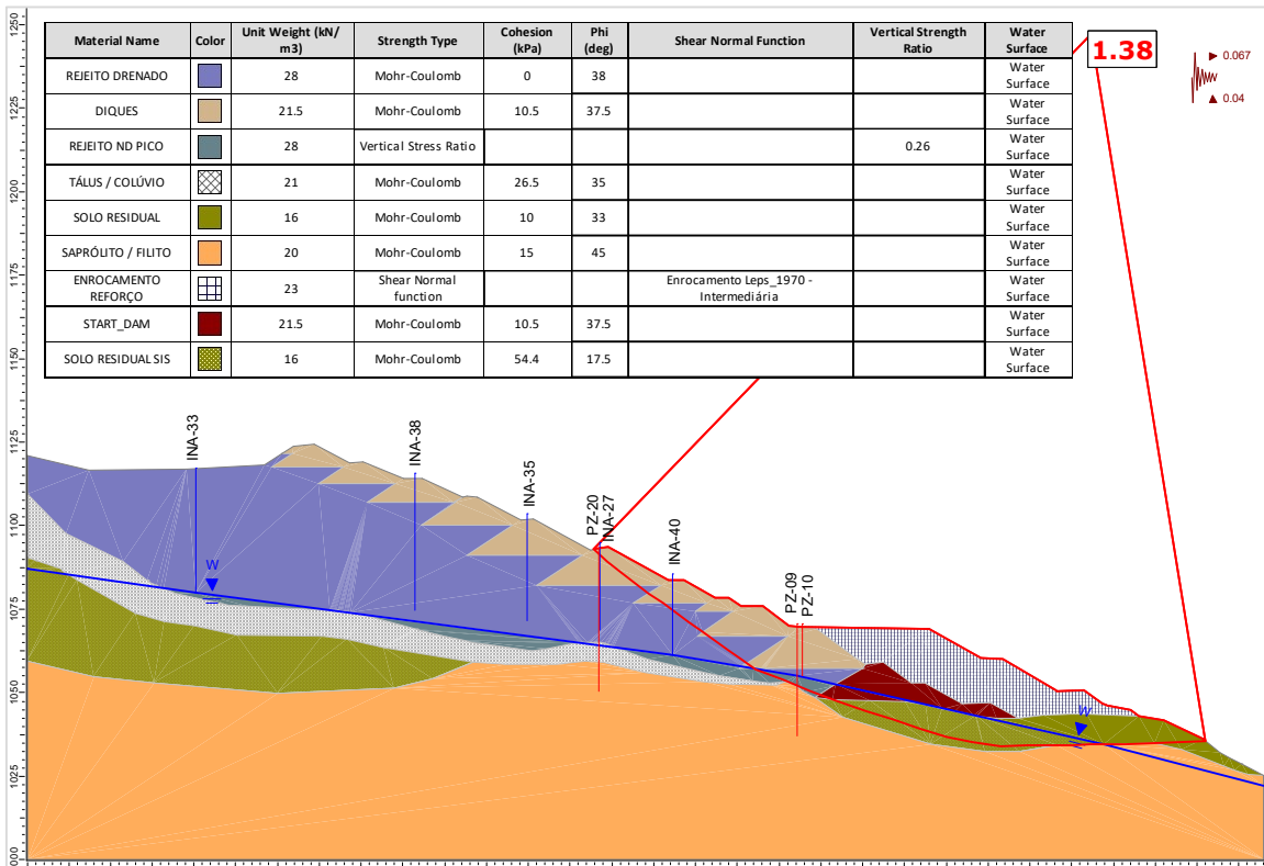
Figura 6.127 – Seção E-E' – Análise Não Drenada – Superfície de ruptura plano-circular otimizada – Freática 30/10/2024 – Razão de resistência não drenada de pico + sismo ↑ (critério vida útil).
