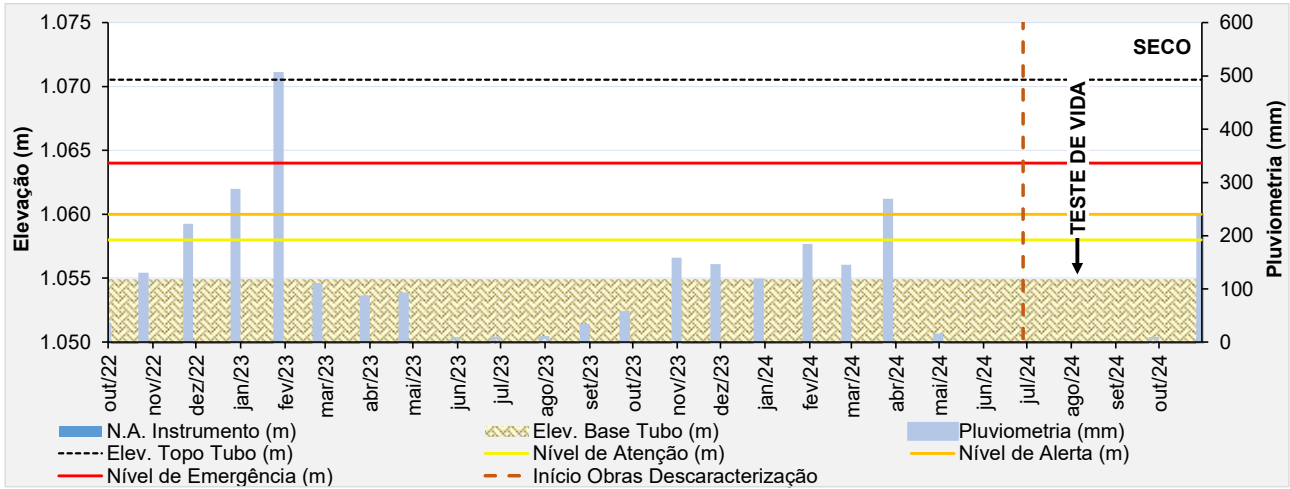
Figura 6.71 – Desempenho do piezômetro de tubo aberto – PZ-10.
