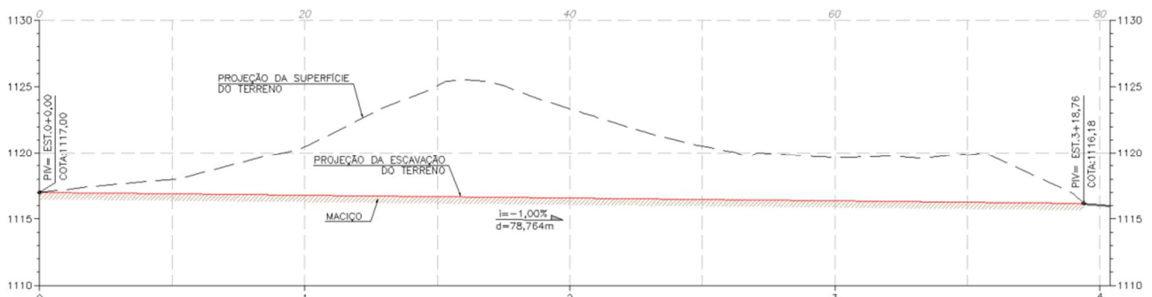
Figura 5.13 - Canal de conexão com extravasor de emergência (Etapa 1 - Fase 2) - Seção Longitudinal (Fonte: IPE.OP.DE.8000.GT.20.1013).
