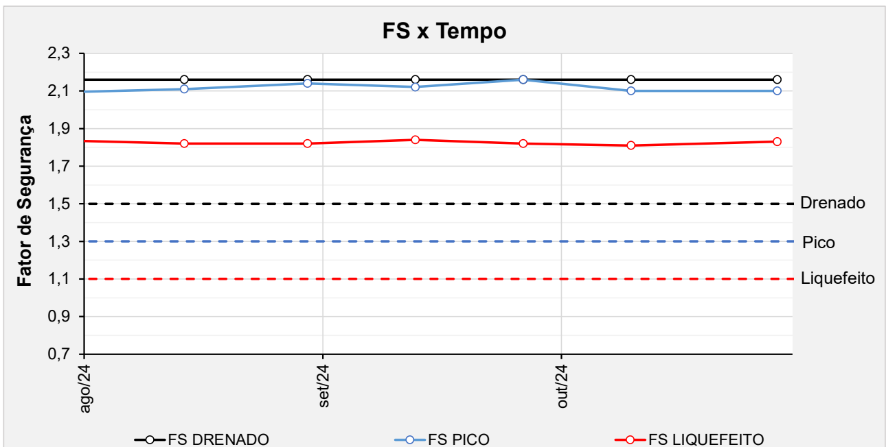
Figura 6.129 – Seção A-A' - Histórico dos F.S. obtidos nas análises de estabilidade no período avaliado.
