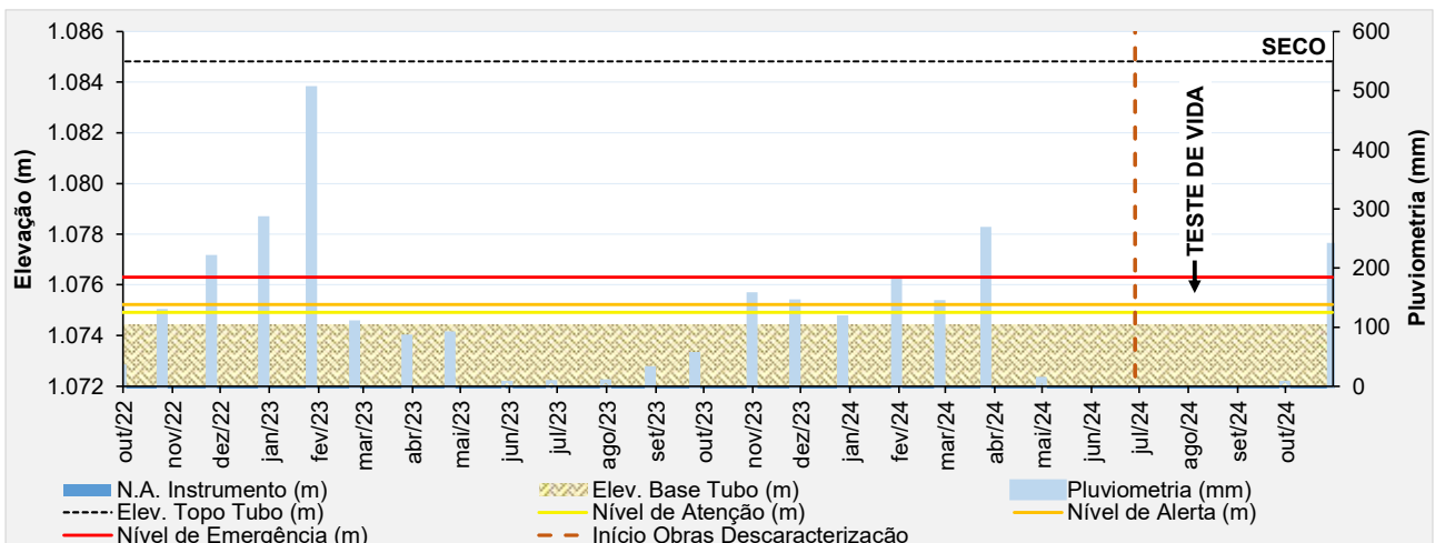
Figura 6.28 – Desempenho do indicador de nível d'água - INA-03.
