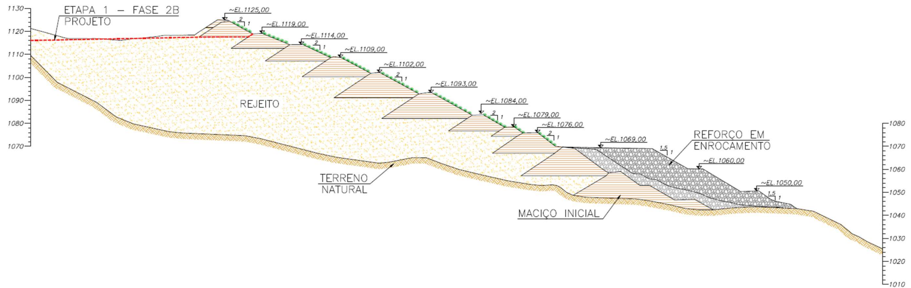
Figura 6.15 – Comparativo Projeto (Etapa 1 - Fase 2B) x Executado – Seção E-E’.
