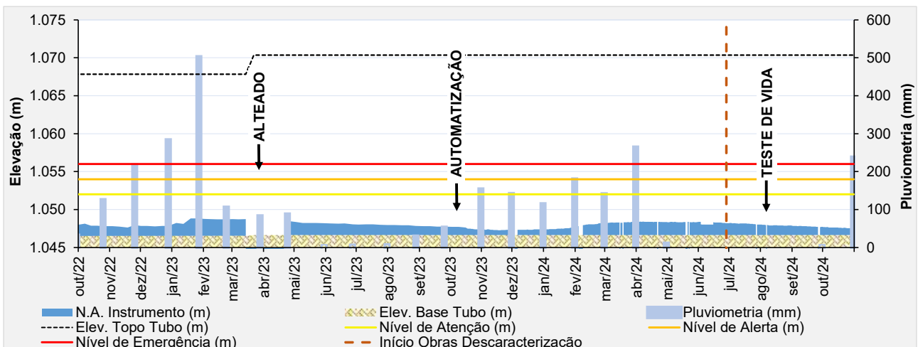
Figura 6.63 – Desempenho do piezômetro automatizado – PZ-02.
