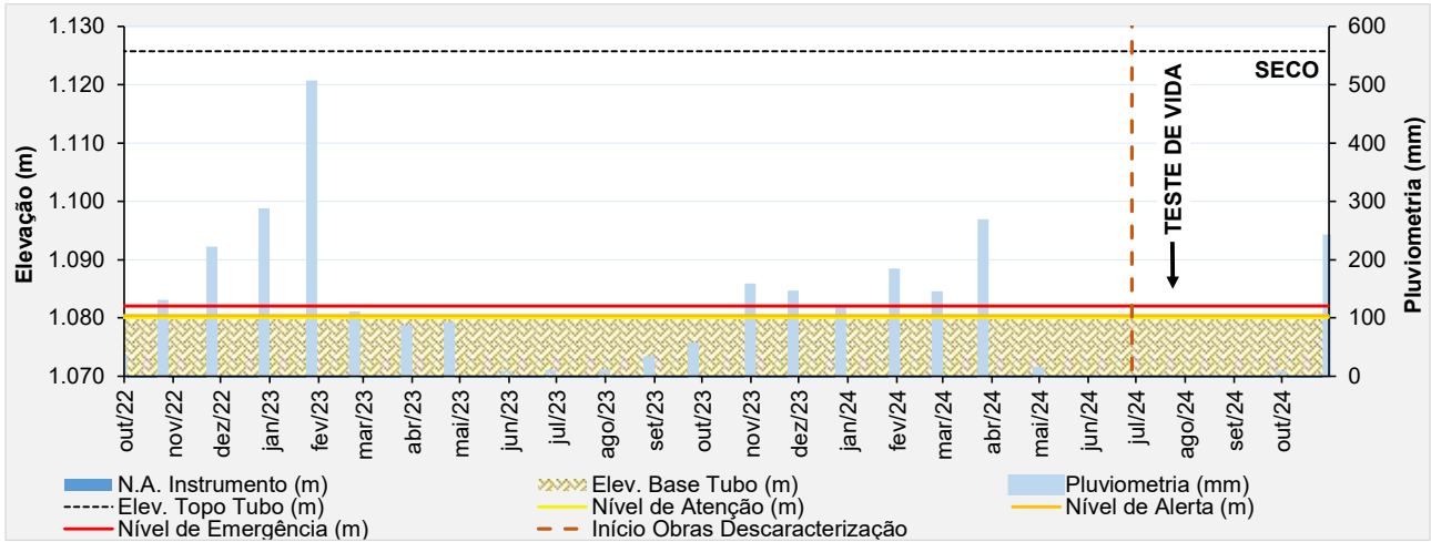
Figura 6.44 – Desempenho do indicador de nível d'água – INA-23.
