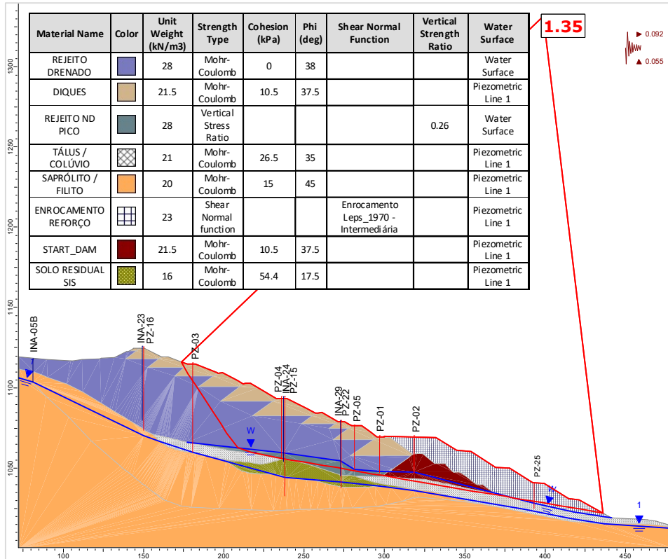
Figura 6.118 – Seção D-D' – Análise Não Drenada – Superfície de ruptura plano-circular otimizada – Freática 30/10/2024 – Razão de resistência não drenada de pico + sismo ↑ (critério CDA).
