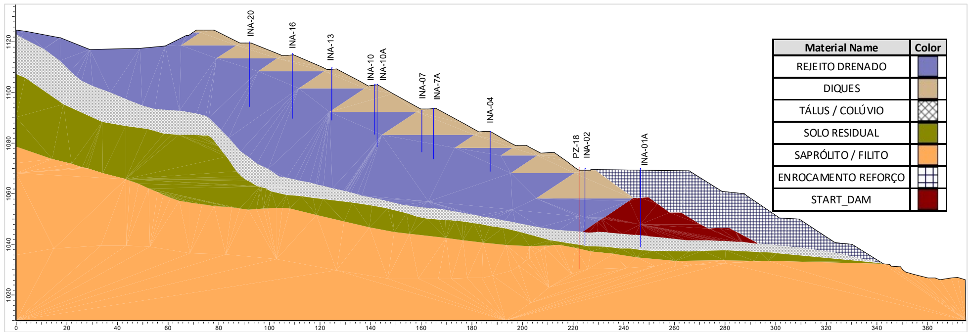
Figura 6.21 – Seção transversal de controle B-B' (Condição em 31/10/2024).
