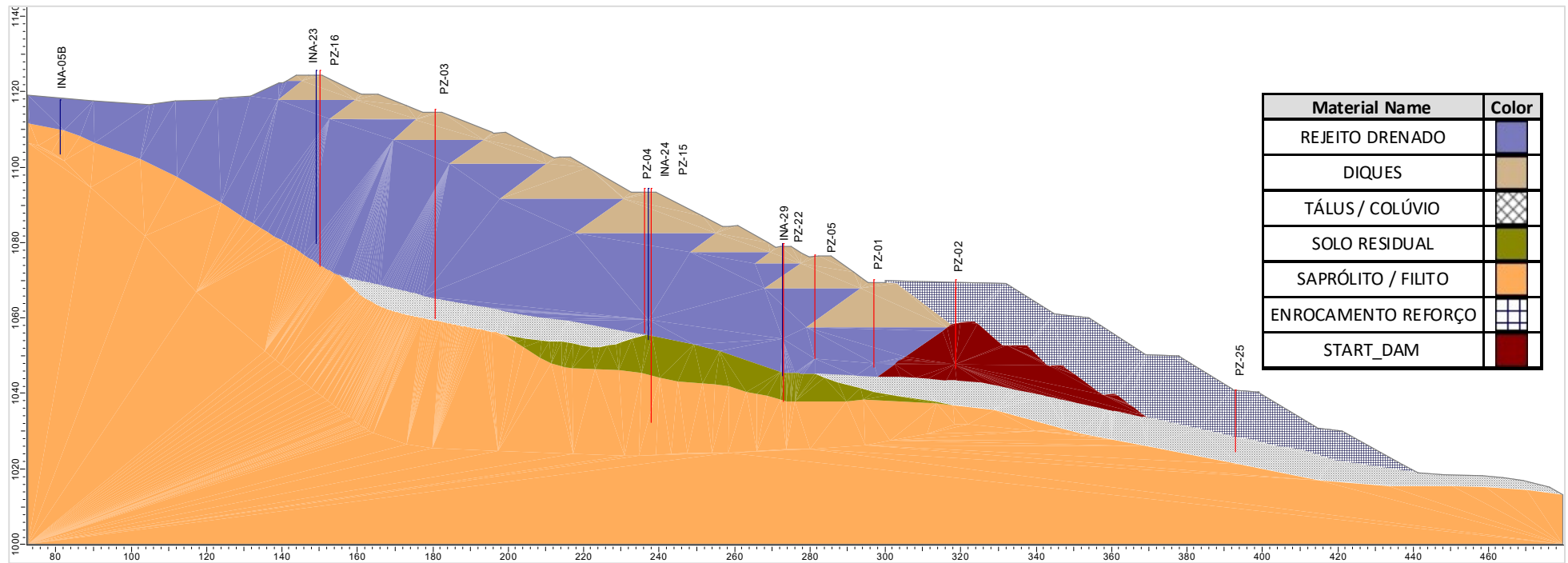
Figura 6.23 – Seção transversal de controle D-D' (Condição em 31/10/2024).
