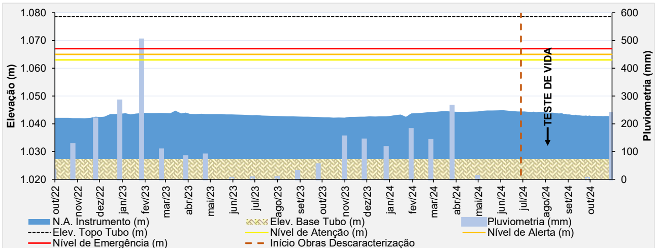
Figura 6.72 – Desempenho do piezômetro de tubo aberto – PZ-11.
