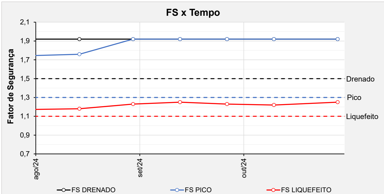
Figura 6.132 – Seção D-D' - Histórico dos F.S. obtidos nas análises de estabilidade no período avaliado.
