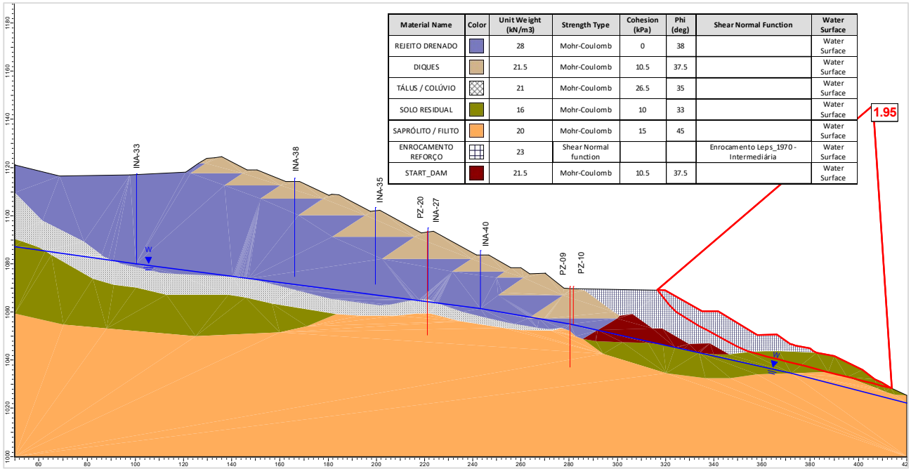
Figura 6.122 – Seção E-E' – Análise Drenada – Superfície de ruptura plano-circular otimizada – Freática 30/10/2024.
