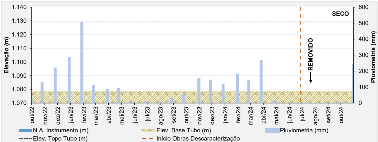
Figura 6.68 – Desempenho do piezômetro de tubo aberto – PZ-07 (removido).
