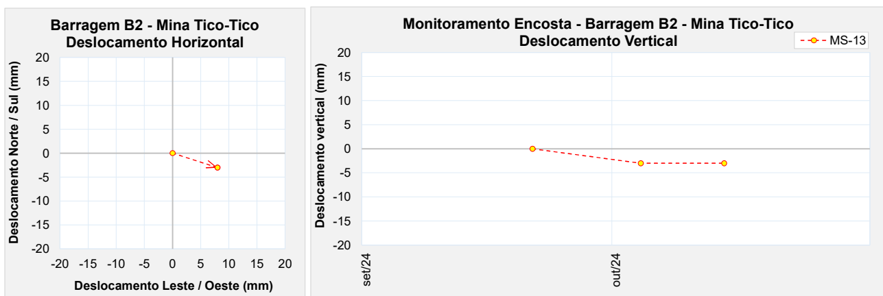
Figura 5.32 – Marco de controle de monitoramento da encosta – MS-13.
