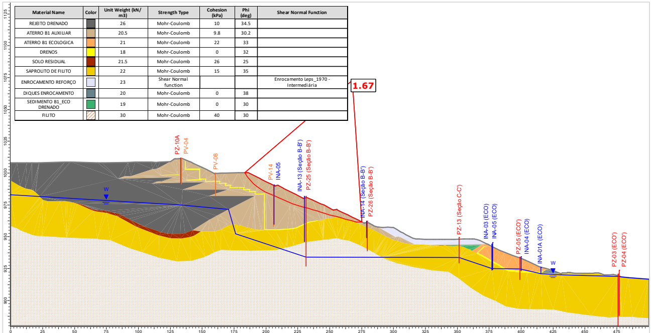
Figura 5.108 – Seção A-A' – Análise Drenada – Superfície de ruptura plano-circular otimizada – Freática 28/10/2024.
