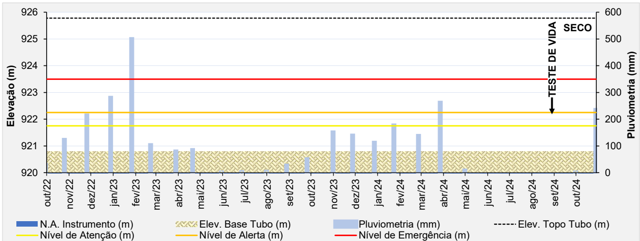
Figura 5.78 – Desempenho do indicador de nível d'água - INA-01A ECO.
