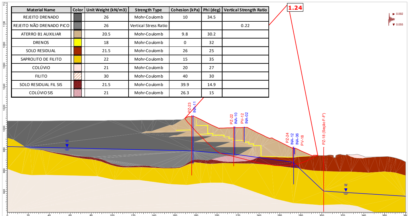
Figura 5.140 – Seção E-E' – Análise Não Drenada – Superfície de ruptura plano-circular otimizada – Freática 28/10/2024 – Razão de resistência não drenada de pico + sismo ↓ (critério CDA).
