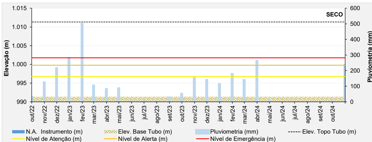
Figura 5.23 – Desempenho do piezômetro elétrico - PV-07.
