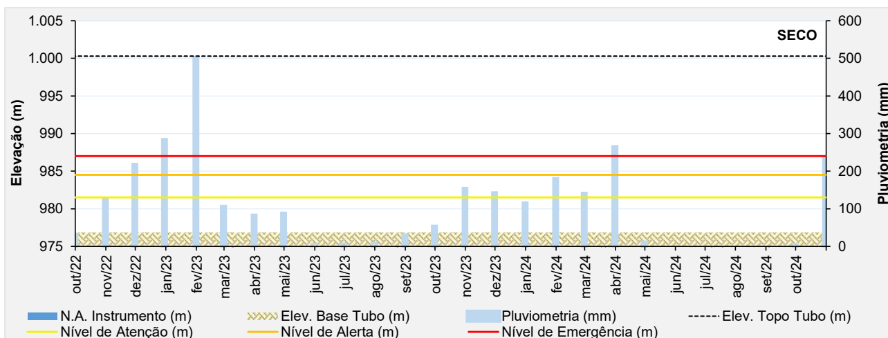
Figura 5.25 – Desempenho do piezômetro elétrico - PV-09.
