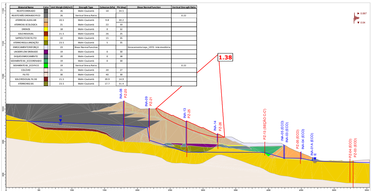
Figura 5.121 – Seção B-B' – Análise Não Drenada – Superfície de ruptura plano-circular otimizada – Freática 28/10/2024 – Razão de resistência não drenada de pico + sismo ↓ (critério vida útil).
