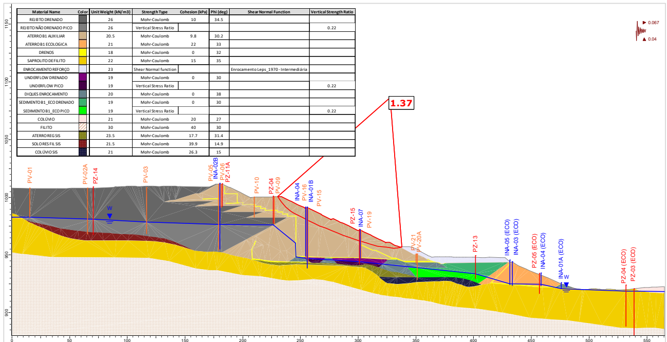
Figura 5.127 – Seção C-C' – Análise Não Drenada – Superfície de ruptura plano-circular otimizada – Freática 28/10/2024 – Razão de resistência não drenada de pico + sismo ↑ (critério vida útil).
