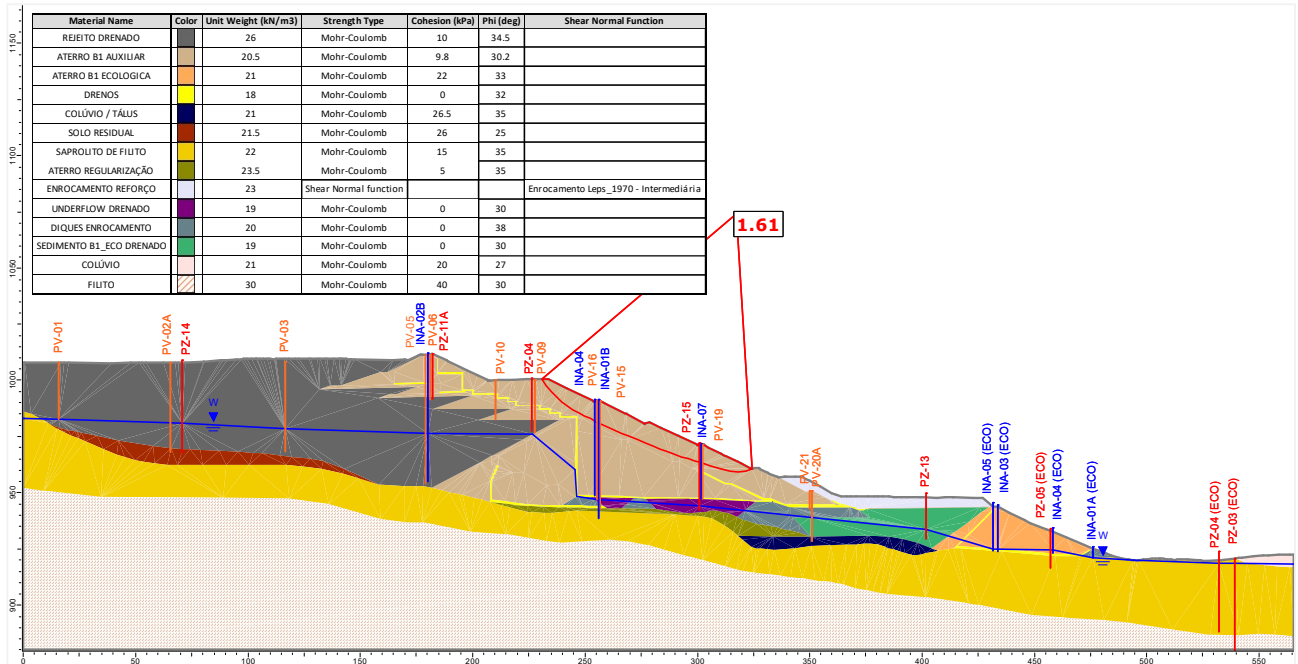
Figura 5.122 – Seção C-C’ – Análise Drenada – Superfície de ruptura plano-circular otimizada – Freática 28/10/2024.
