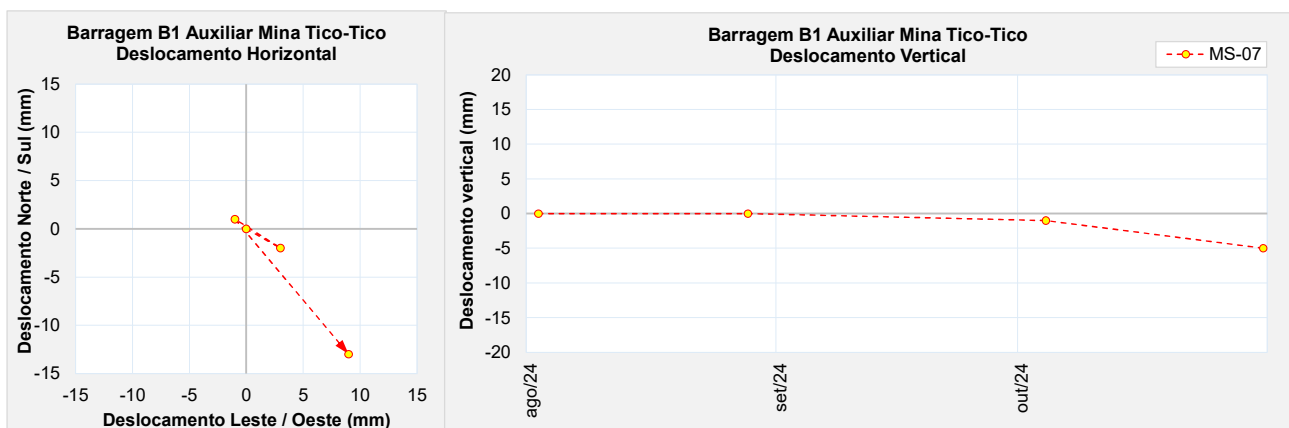
Figura 5.99 – Marco de controle de deformação – MS-07.
