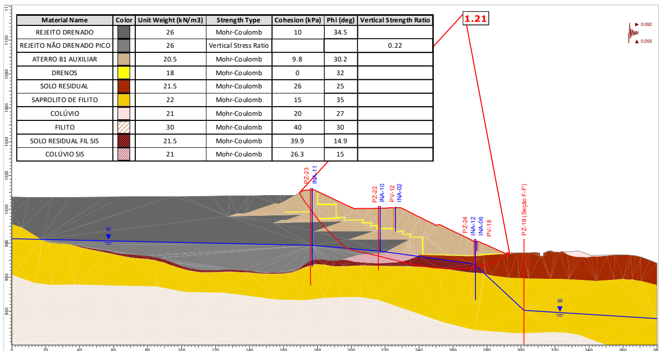
Figura 5.139 – Seção E-E' – Análise Não Drenada – Superfície de ruptura plano-circular otimizada – Freática 28/10/2024 – Razão de resistência não drenada de pico + sismo ↑ (critério CDA).
