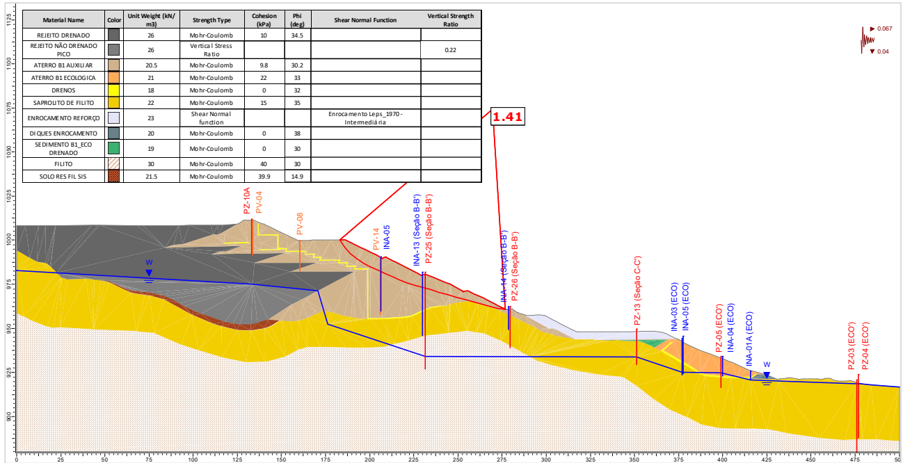
Figura 5.114 – Seção A-A’ – Análise Não Drenada – Superfície de ruptura plano-circular otimizada – Freática 28/10/2024 – Razão de resistência não drenada de pico + sismo ↓ (critério vida útil).
