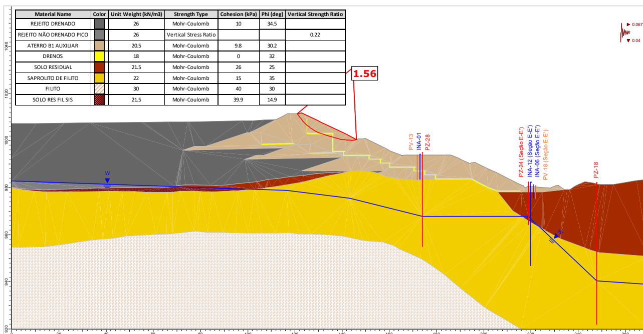
Figura 5.149 – Seção F-F’ – Análise Não Drenada – Superfície de ruptura plano-circular otimizada – Freática 28/10/2024 – Razão de resistência não drenada de pico + sismo ↓ (critério vida útil).
