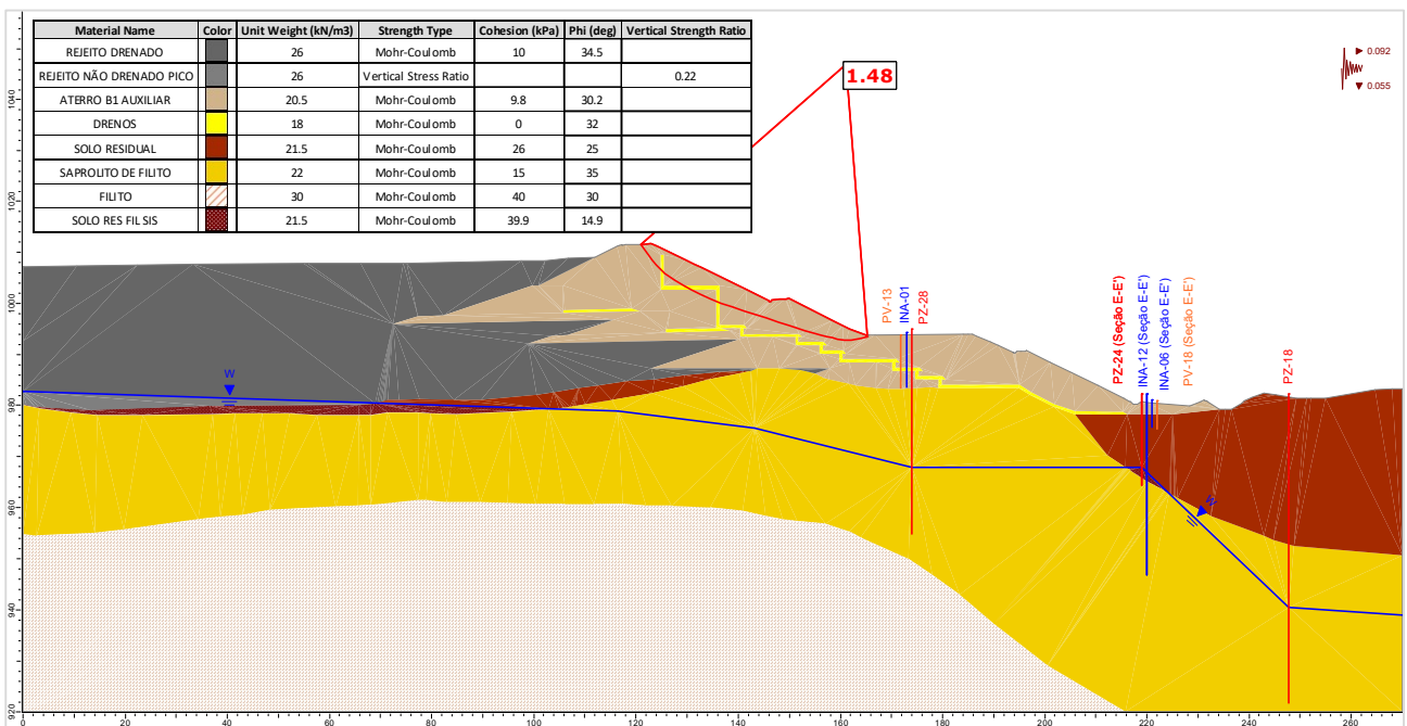
Figura 5.147 – Seção F-F' – Análise Não Drenada – Superfície de ruptura plano-circular otimizada – Freática 28/10/2024 – Razão de resistência não drenada de pico + sismo ↓ (critério CDA).
