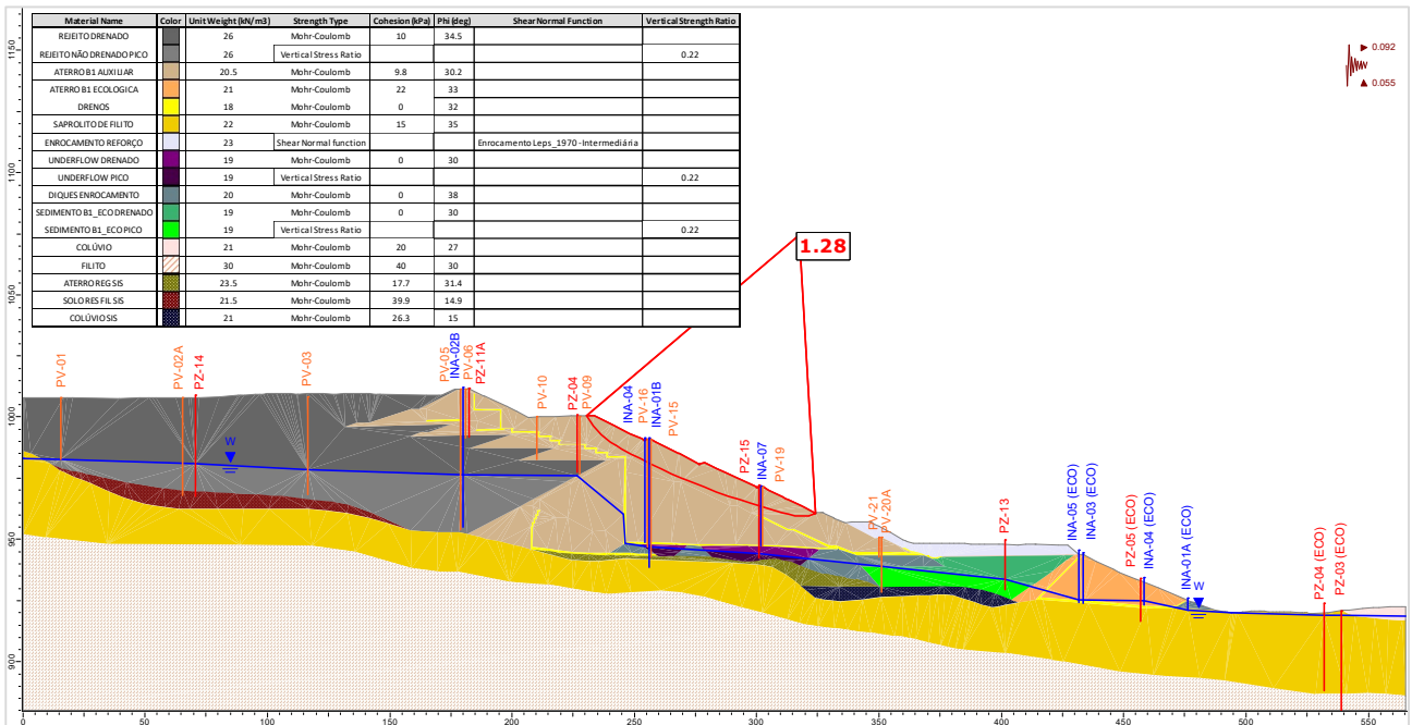
Figura 5.125 – Seção C-C' – Análise Não Drenada – Superfície de ruptura plano-circular otimizada – Freática 28/10/2024 – Razão de resistência não drenada de pico + sismo ↑ (critério CDA).
