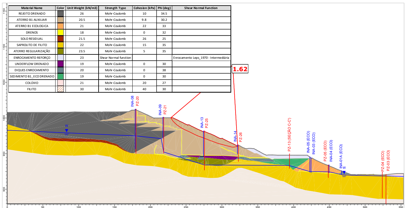
Figura 5.115 – Seção B-B’ – Análise Drenada – Superfície de ruptura plano-circular otimizada – Freática 28/10/2024.
