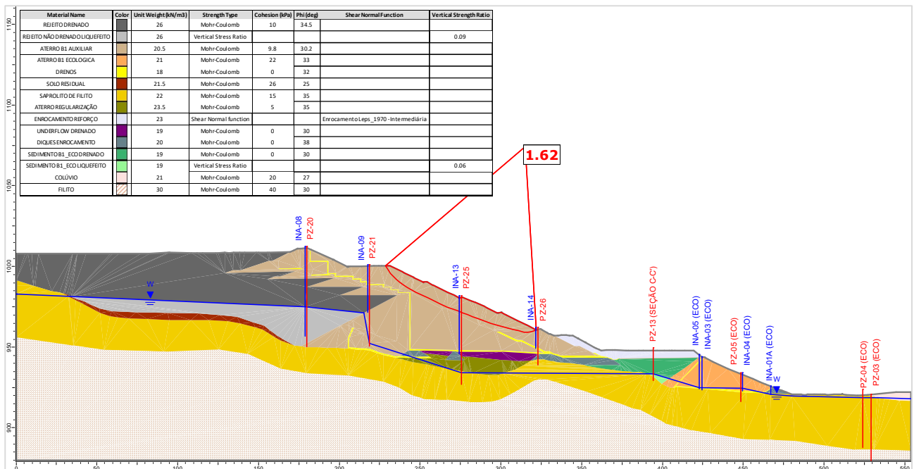
Figura 5.117 – Seção B-B' – Análise Não Drenada – Superfície de ruptura plano-circular otimizada – Freática 28/10/2024 – Razão de resistência não drenada liquefeita.
