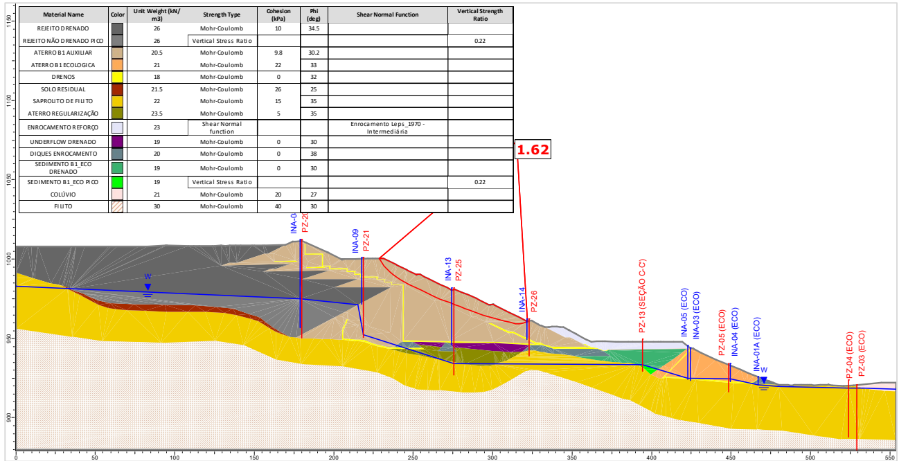
Figura 5.116 – Seção B-B' – Análise Não Drenada – Superfície de ruptura plano-circular otimizada – Freática 28/10/2024 – Razão de resistência não drenada de pico.
