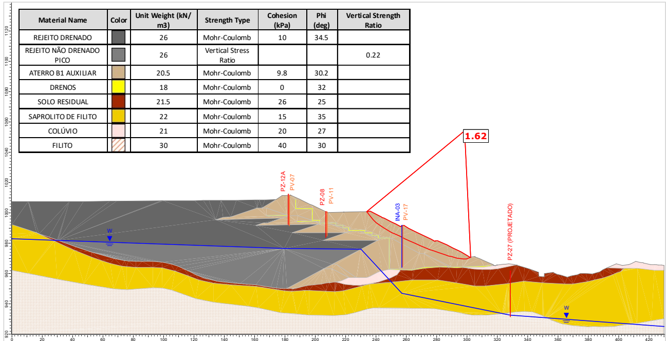
Figura 5.130 – Seção D-D' – Análise Não Drenada – Superfície de ruptura plano-circular otimizada – Freática 28/10/2024 – Razão de resistência não drenada de pico.
