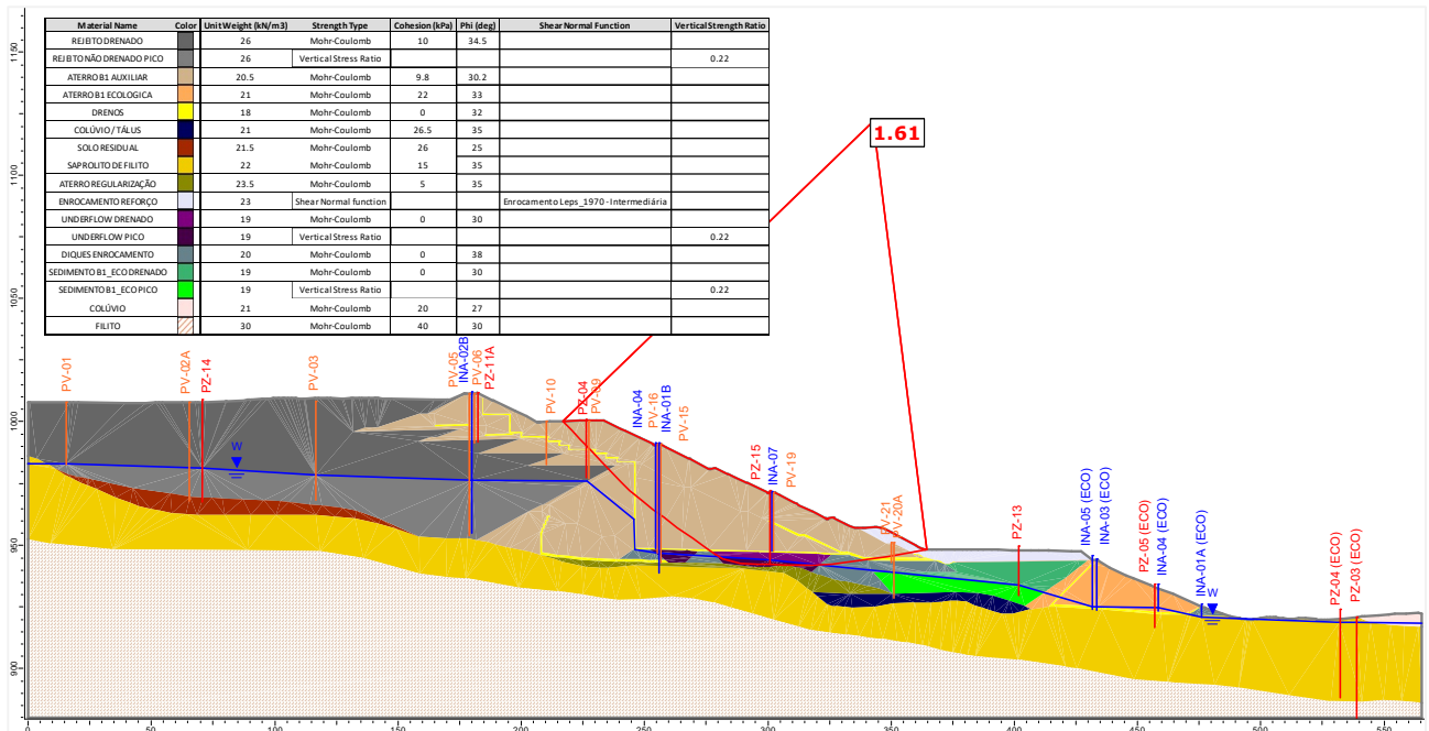
Figura 5.123 – Seção C-C’ – Análise Não Drenada – Superfície de ruptura plano-circular otimizada – Freática 28/10/2024 – Razão de resistência não drenada de pico.
