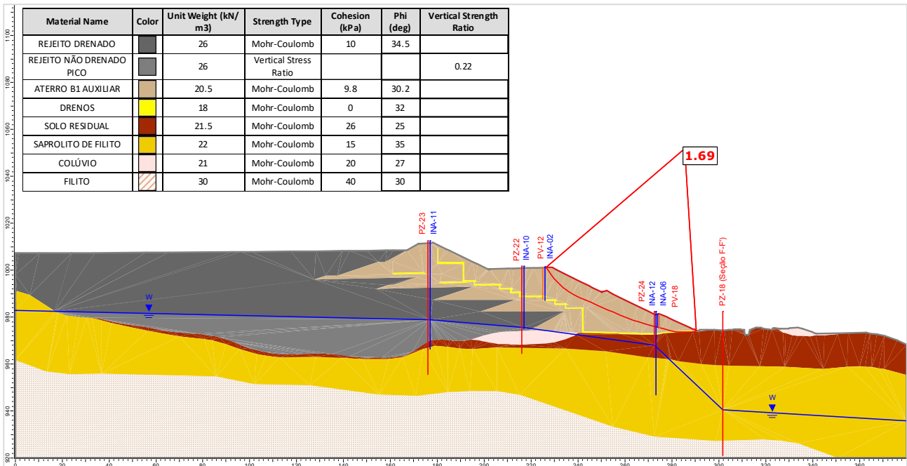
Figura 5.137 – Seção E-E' – Análise Não Drenada – Superfície de ruptura plano-circular otimizada – Freática 28/10/2024 – Razão de resistência não drenada de pico.
