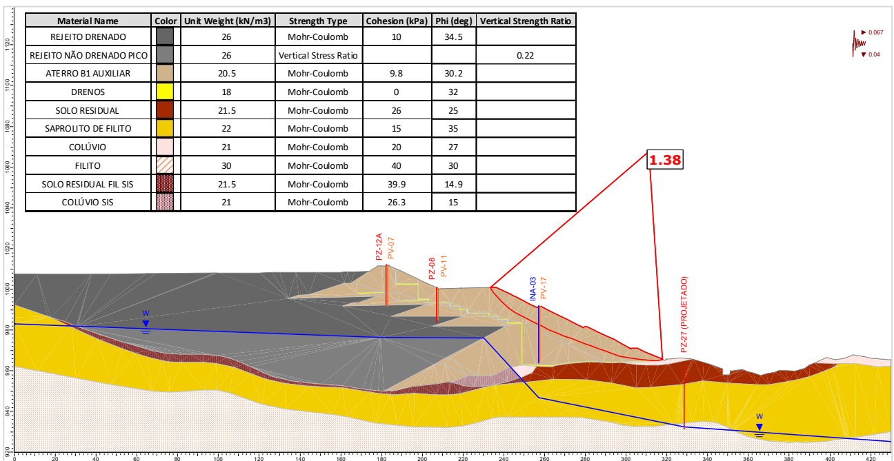
Figura 5.135 – Seção D-D' – Análise Não Drenada – Superfície de ruptura plano-circular otimizada – Freática 28/10/2024 – Razão de resistência não drenada de pico + sismo ↓ (critério vida útil).
