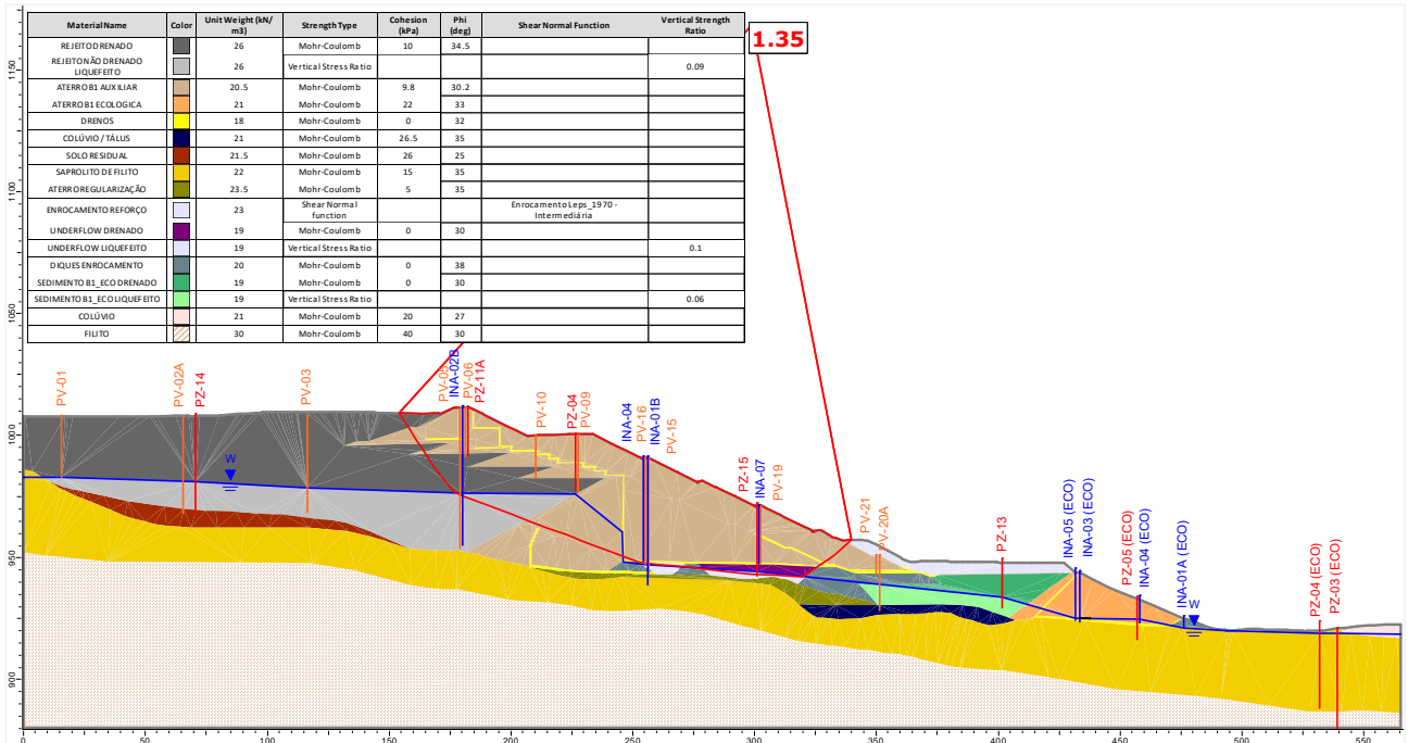
Figura 5.124 – Seção C-C' – Análise Não Drenada – Superfície de ruptura plano-circular otimizada – Freática 28/10/2024 – Razão de resistência não drenada liquefeita.
