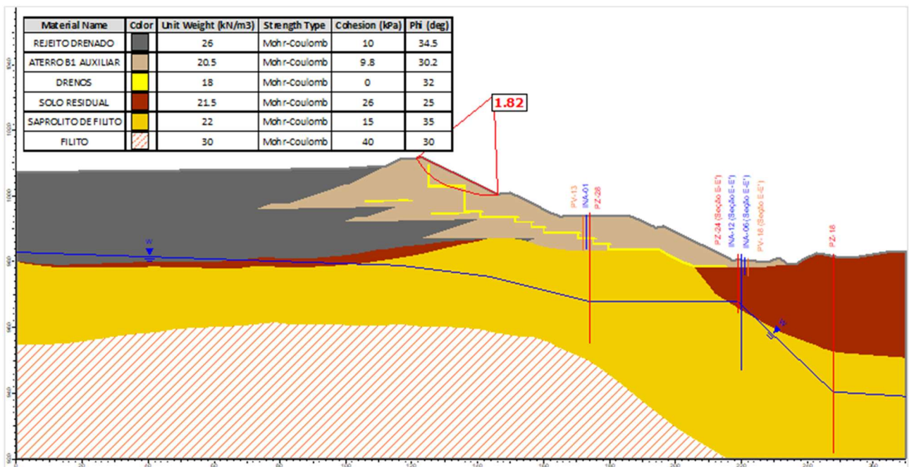
Figura 5.143 – Seção F-F' – Análise Drenada – Superfície de ruptura plano-circular otimizada – Freática 28/10/2024.
