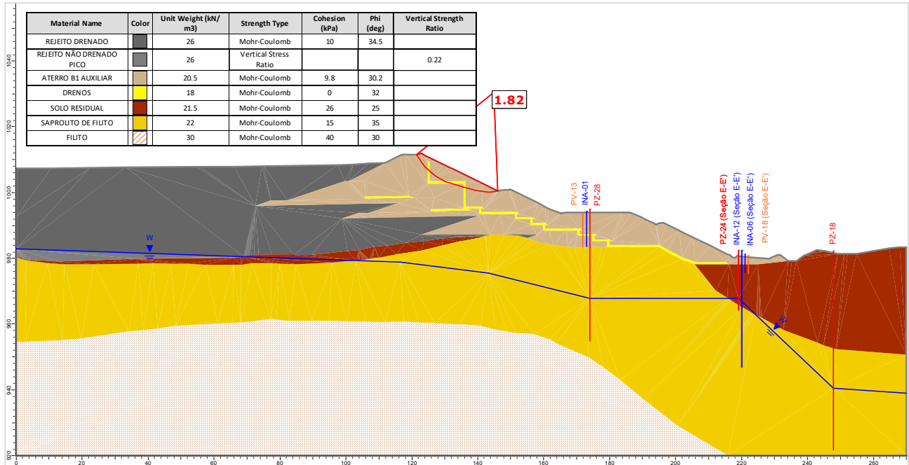
Figura 5.144 – Seção F-F' – Análise Não Drenada – Superfície de ruptura plano-circular otimizada – Freática 28/10/2024 – Razão de resistência não drenada de pico.
