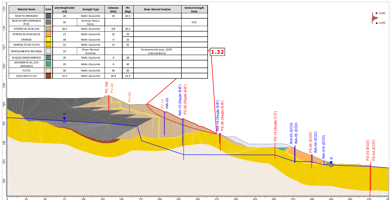
Figura 5.111 – Seção A-A' – Análise Não Drenada – Superfície de ruptura plano-circular otimizada – Freática 28/10/2024 – Razão de resistência não drenada de pico + sismo ↑ (critério CDA).
