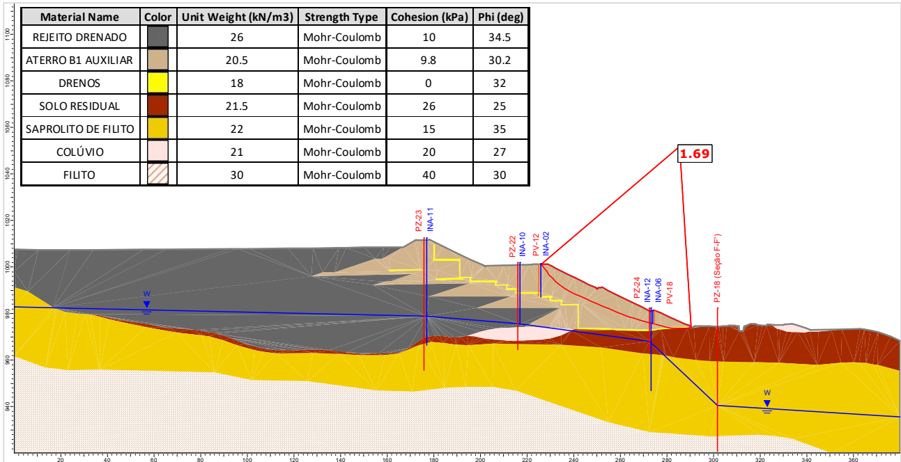
Figura 5.136 – Seção E-E' – Análise Drenada – Superfície de ruptura plano-circular otimizada – Freática 28/10/2024.
