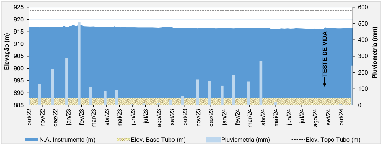
Figura 5.60 – Desempenho do piezômetro de tubo aberto - PZ-04 ECO.
