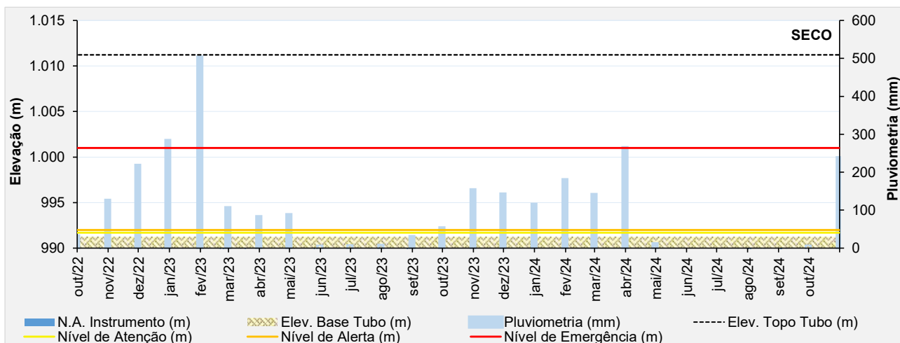
Figura 5.22 – Desempenho do piezômetro elétrico - PV-06.
