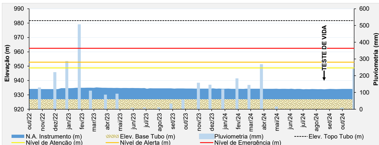
Figura 5.55 – Desempenho do piezômetro de tubo aberto - PZ-25.
