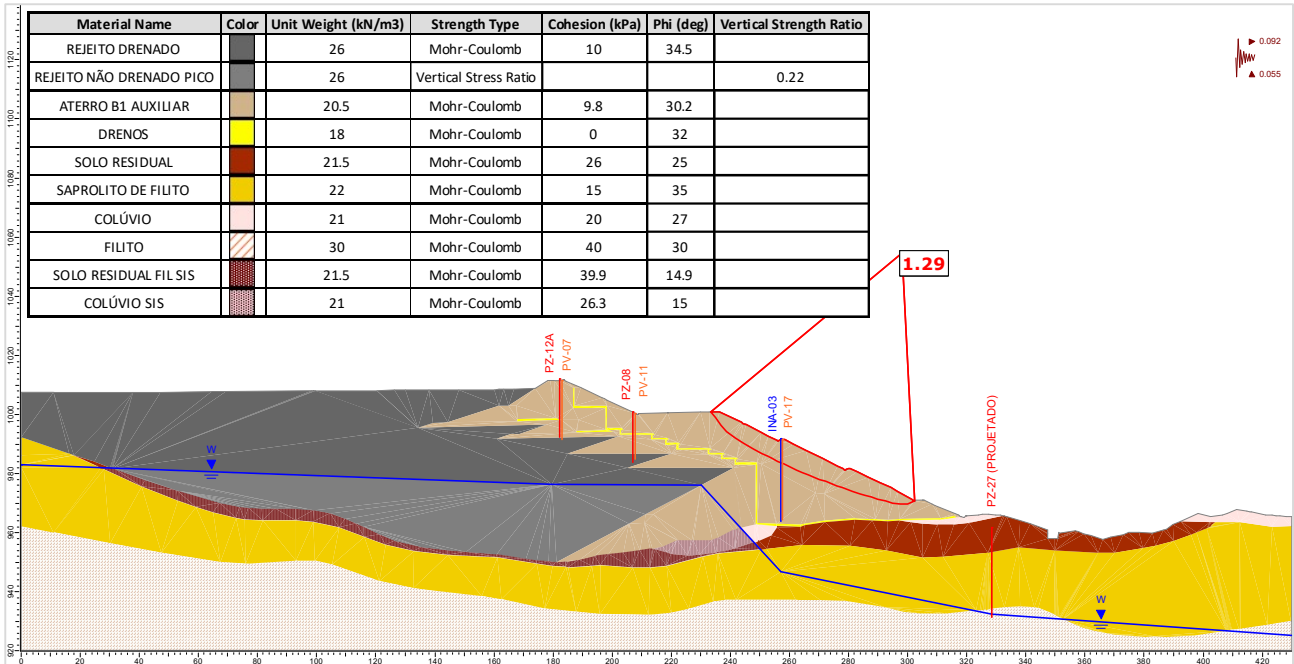
Figura 5.132 – Seção D-D' – Análise Não Drenada – Superfície de ruptura plano-circular otimizada – Freática 28/10/2024 – Razão de resistência não drenada de pico + sismo ↑ (critério CDA).
