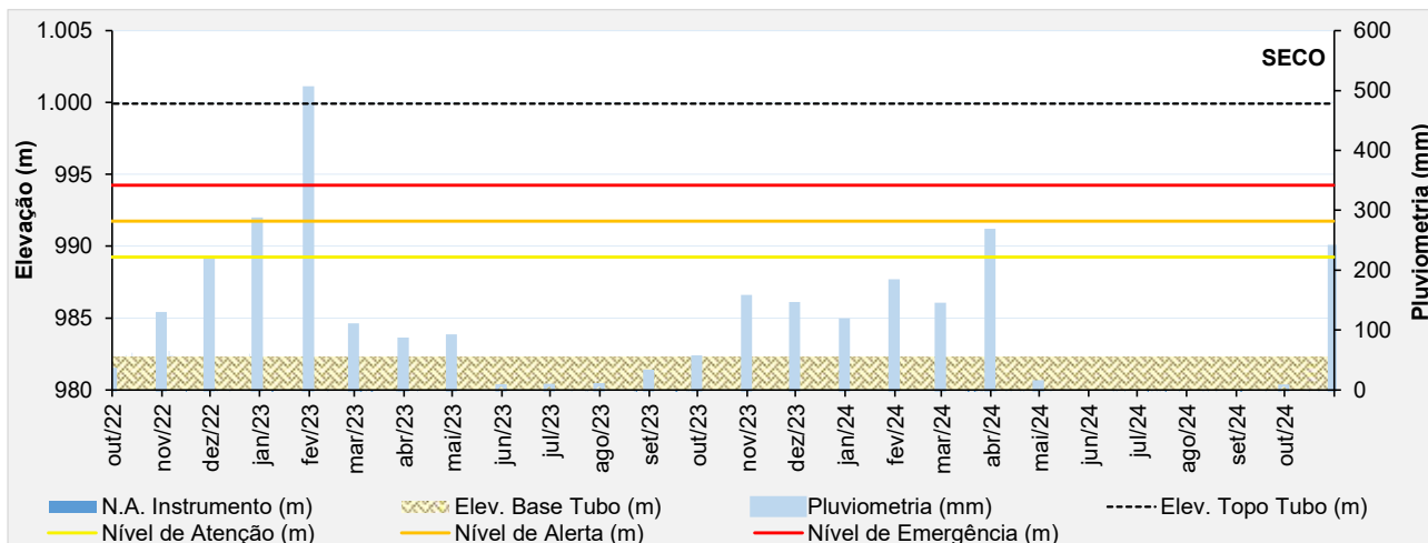
Figura 5.24 – Desempenho do piezômetro elétrico - PV-08.
