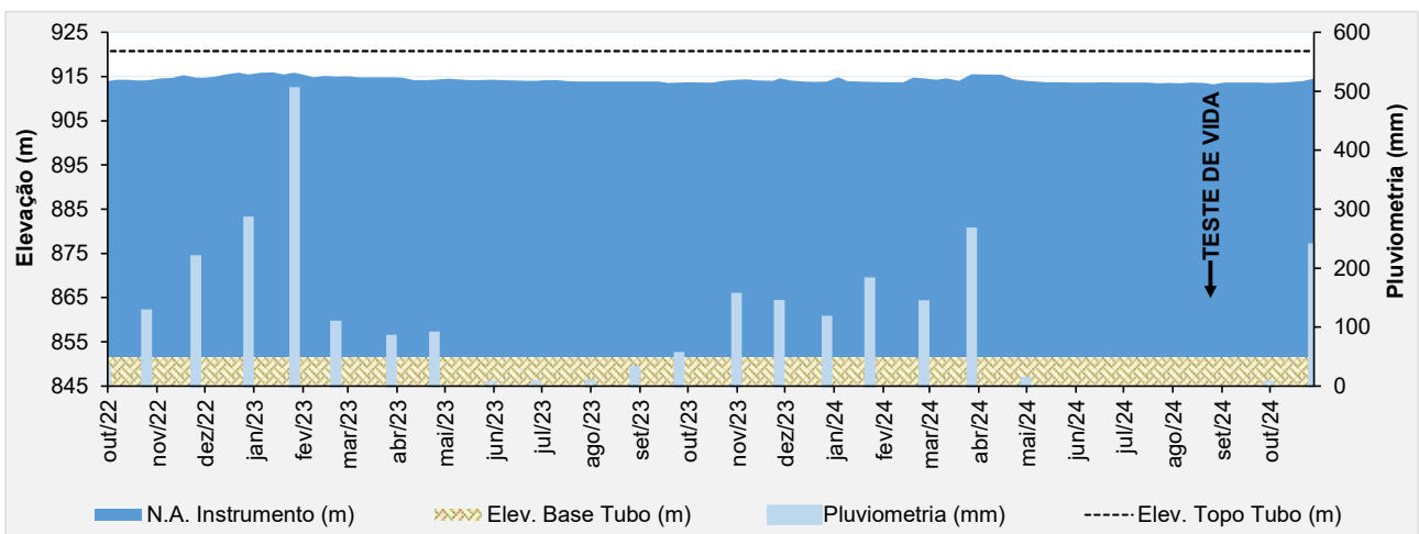
Figura 5.59 – Desempenho do piezômetro de tubo aberto - PZ-03 ECO.
