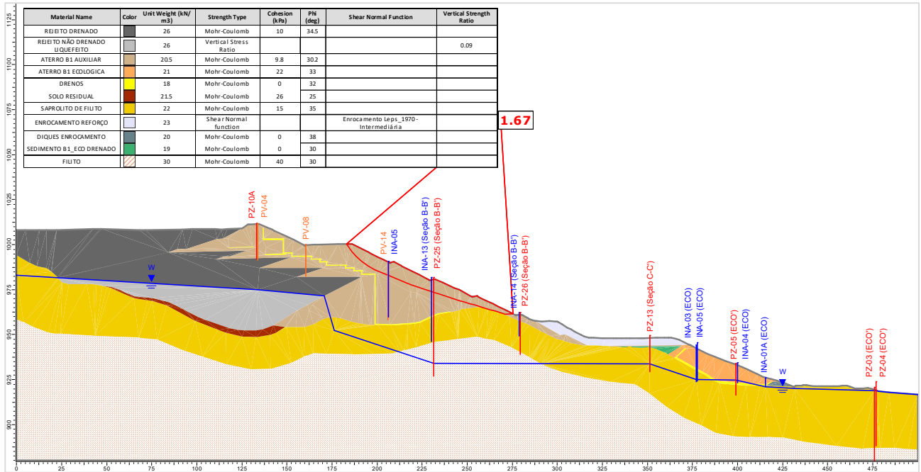
Figura 5.110 – Seção A-A' – Análise Não Drenada – Superfície de ruptura plano-circular otimizada – Freática 28/10/2024 – Razão de resistência não drenada liquefeita.
