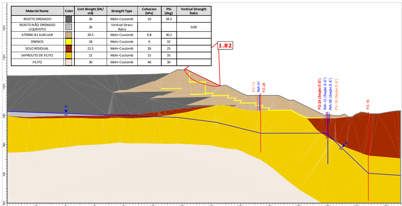
Figura 5.145 – Seção F-F' – Análise Não Drenada – Superfície de ruptura plano-circular otimizada – Freática 28/10/2024 – Razão de resistência não drenada liquefeita.
