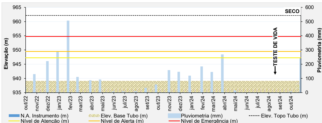
Figura 5.56 – Desempenho do piezômetro de tubo aberto - PZ-26.
