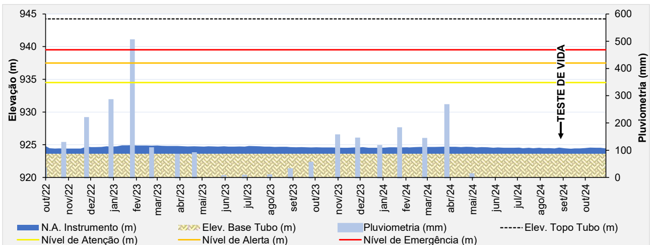
Figura 5.79 – Desempenho do indicador de nível d'água - INA-03 ECO.
