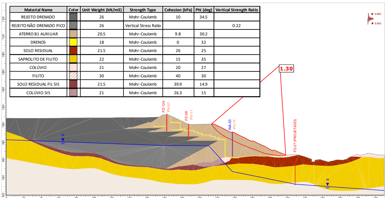
Figura 5.133 – Seção D-D' – Análise Não Drenada – Superfície de ruptura plano-circular otimizada – Freática 28/10/2024 – Razão de resistência não drenada de pico + sismo ↓ (critério CDA).
