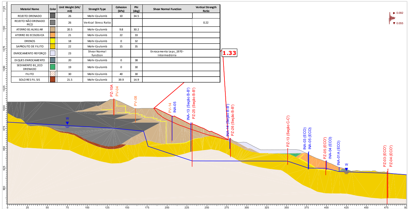
Figura 5.112 – Seção A-A' – Análise Não Drenada – Superfície de ruptura plano-circular otimizada – Freática 28/10/2024 – Razão de resistência não drenada de pico + sismo ↓ (critério CDA).
