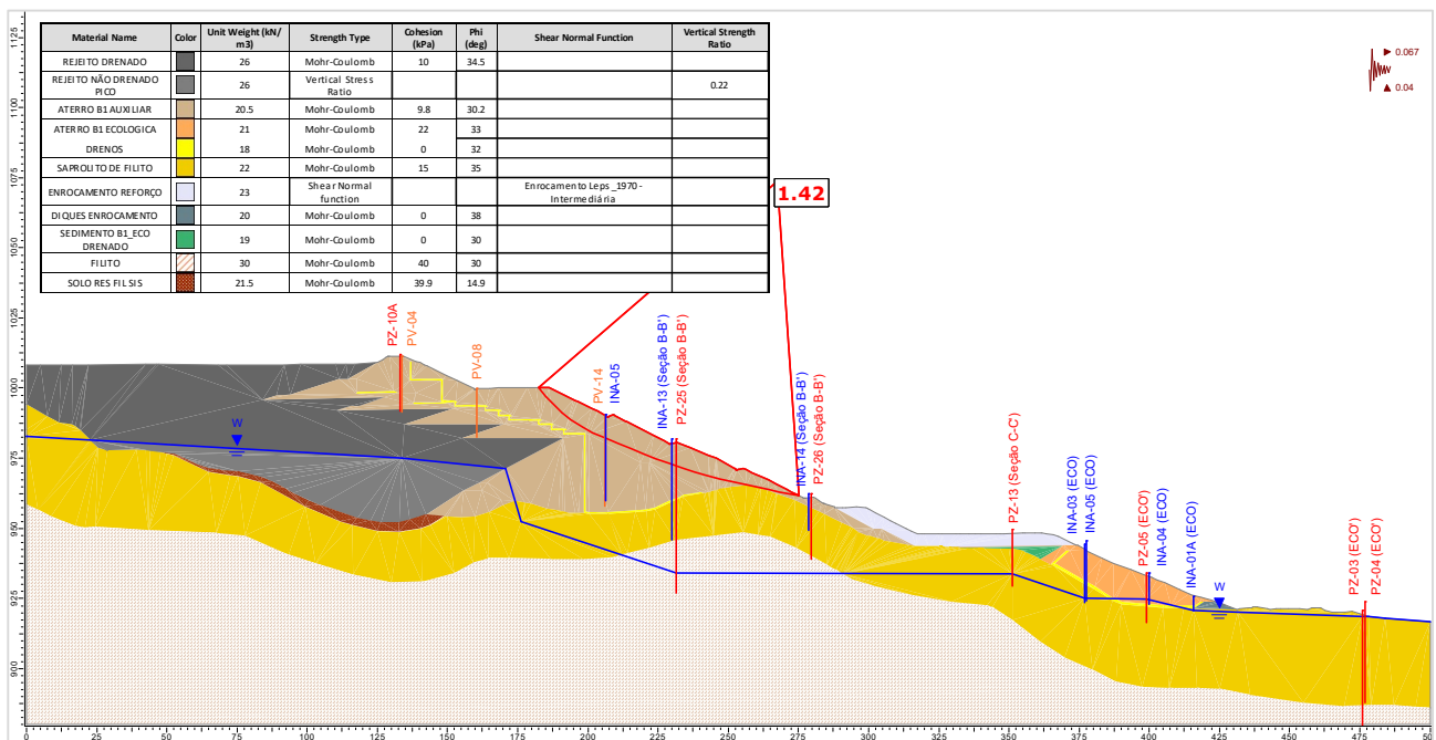
Figura 5.113 – Seção A-A' – Análise Não Drenada – Superfície de ruptura plano-circular otimizada – Freática 28/10/2024 – Razão de resistência não drenada de pico + sismo ↑ (critério vida útil).
