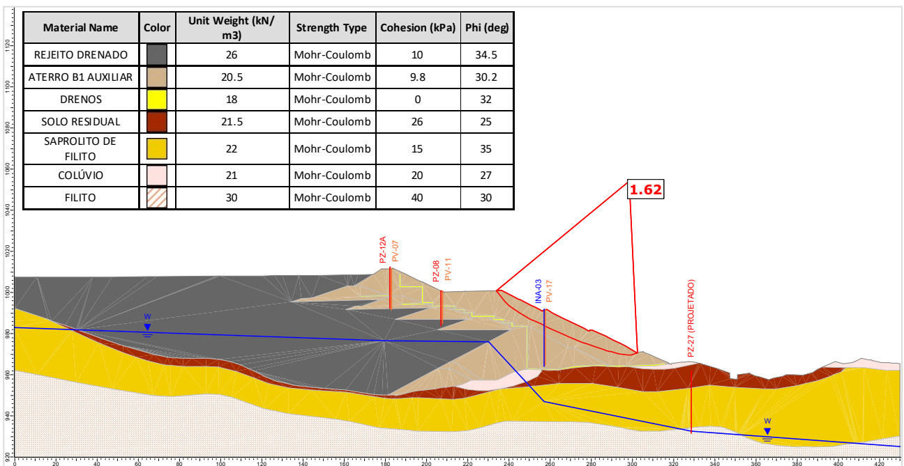
Figura 5.129 – Seção D-D’ – Análise Drenada – Superfície de ruptura plano-circular otimizada – Freática 28/10/2024.
