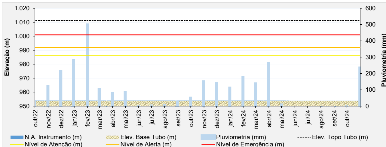
Figura 5.21 – Desempenho do piezômetro elétrico - PV-05.
