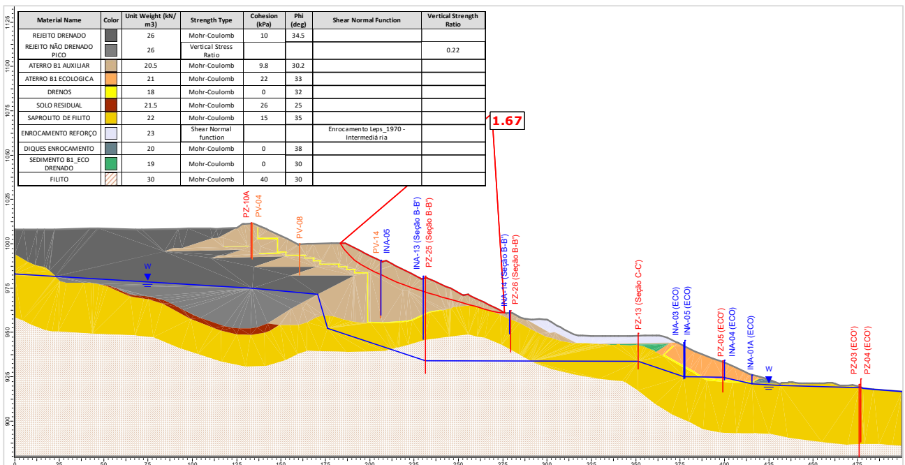
Figura 5.109 – Seção A-A' – Análise Não Drenada – Superfície de ruptura plano-circular otimizada – Freática 28/10/2024 – Razão de resistência não drenada de pico.
