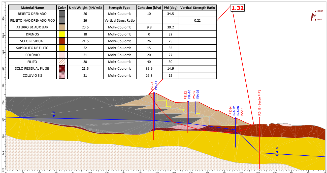
Figura 5.142 – Seção E-E' – Análise Não Drenada – Superfície de ruptura plano-circular otimizada – Freática 28/10/2024 – Razão de resistência não drenada de pico + sismo ↓ (critério vida útil).
