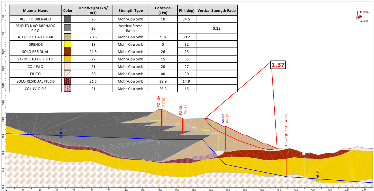
Figura 5.134 – Seção D-D' – Análise Não Drenada – Superfície de ruptura plano-circular otimizada – Freática 28/10/2024 – Razão de resistência não drenada de pico + sismo ↑ (critério vida útil).
