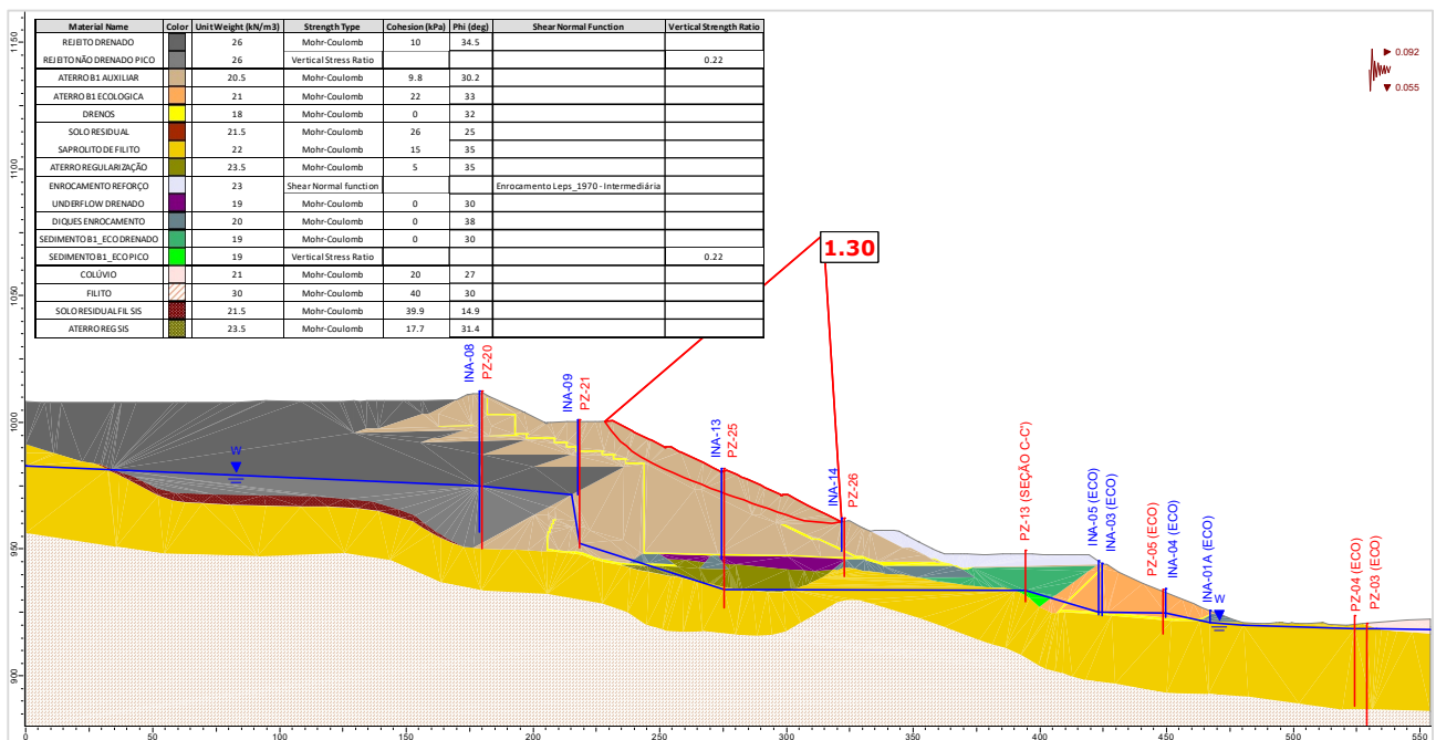
Figura 5.119 – Seção B-B' – Análise Não Drenada – Superfície de ruptura plano-circular otimizada – Freática 28/10/2024 – Razão de resistência não drenada de pico + sismo ↓ (critério CDA).
