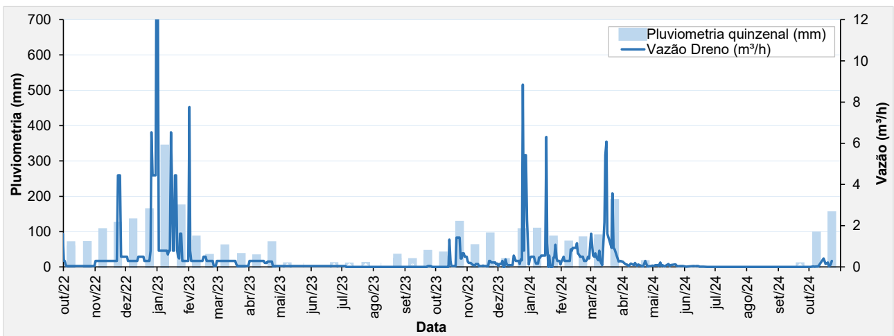
Figura 5.82 – Histórico de leituras da placa indicadora de vazões.
