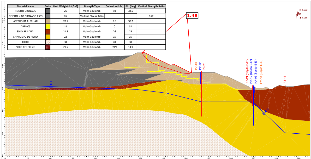
Figura 5.146 – Seção F-F' – Análise Não Drenada – Superfície de ruptura plano-circular otimizada – Freática 28/10/2024 – Razão de resistência não drenada de pico + sismo ↑ (critério CDA).
