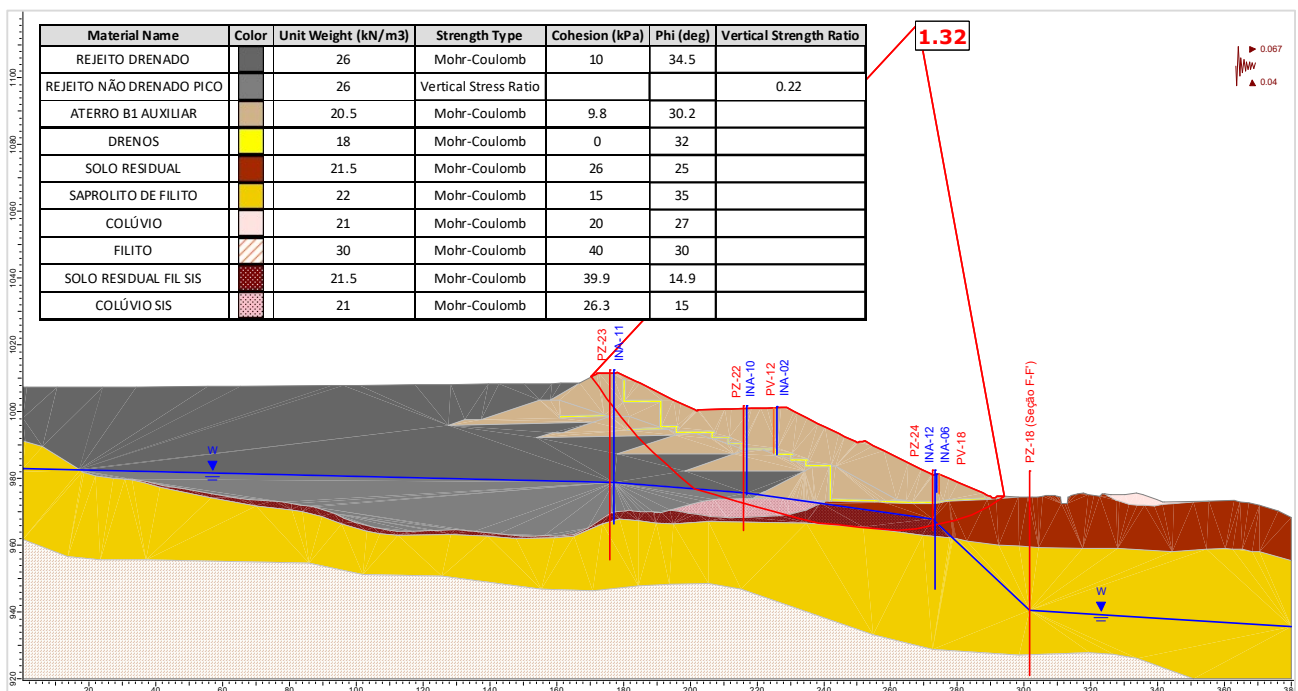
Figura 5.141 – Seção E-E' – Análise Não Drenada – Superfície de ruptura plano-circular otimizada – Freática 28/10/2024 – Razão de resistência não drenada de pico + sismo ↑ (critério vida útil).
