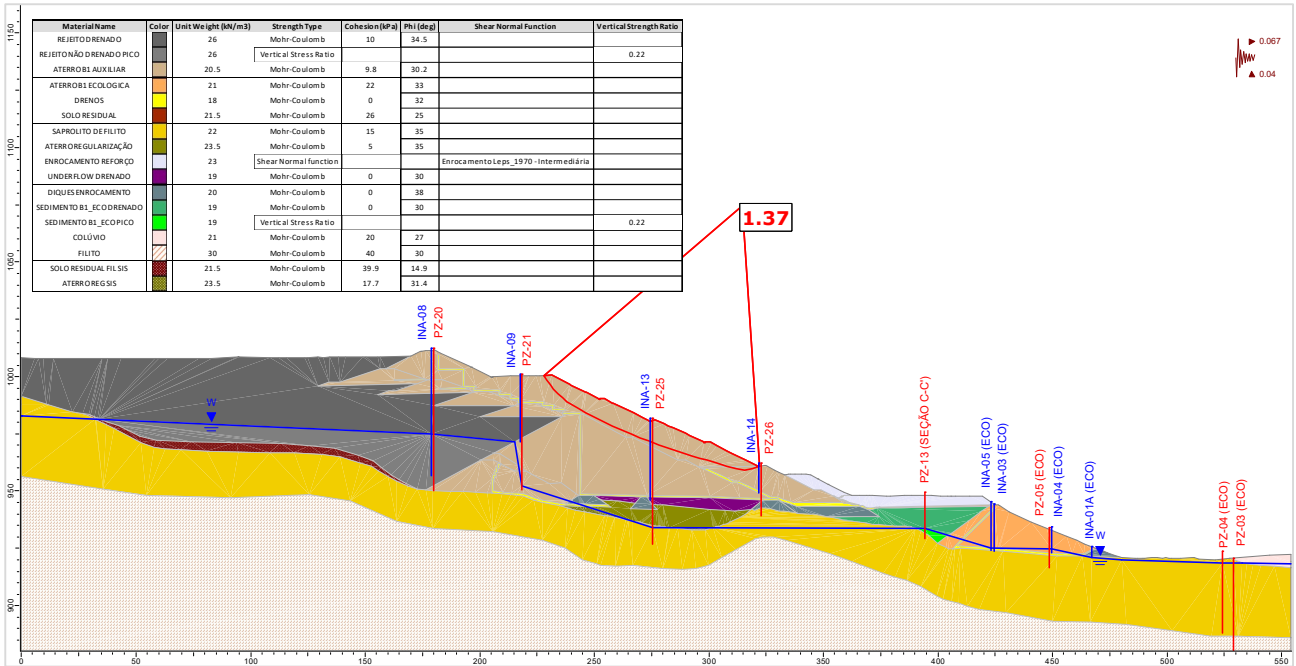
Figura 5.120 – Seção B-B' – Análise Não Drenada – Superfície de ruptura plano-circular otimizada – Freática 28/10/2024 – Razão de resistência não drenada de pico + sismo ↑ (critério vida útil).
