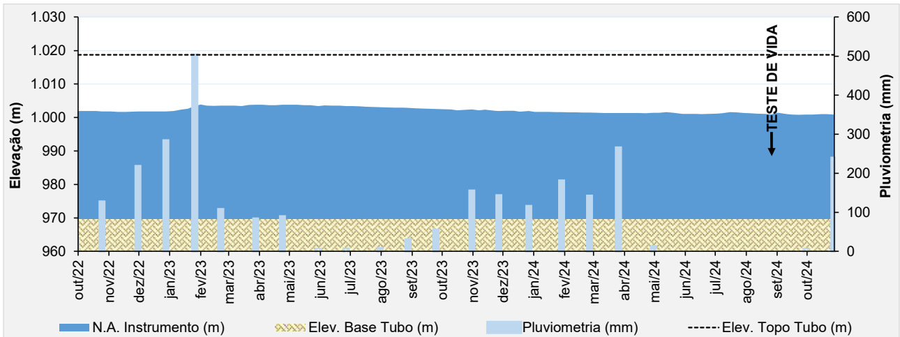
Figura 5.49 – Desempenho do piezômetro de tubo aberto - PZ-19.
