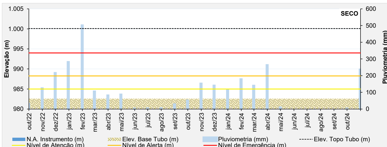
Figura 5.26 – Desempenho do piezômetro elétrico - PV-10.
