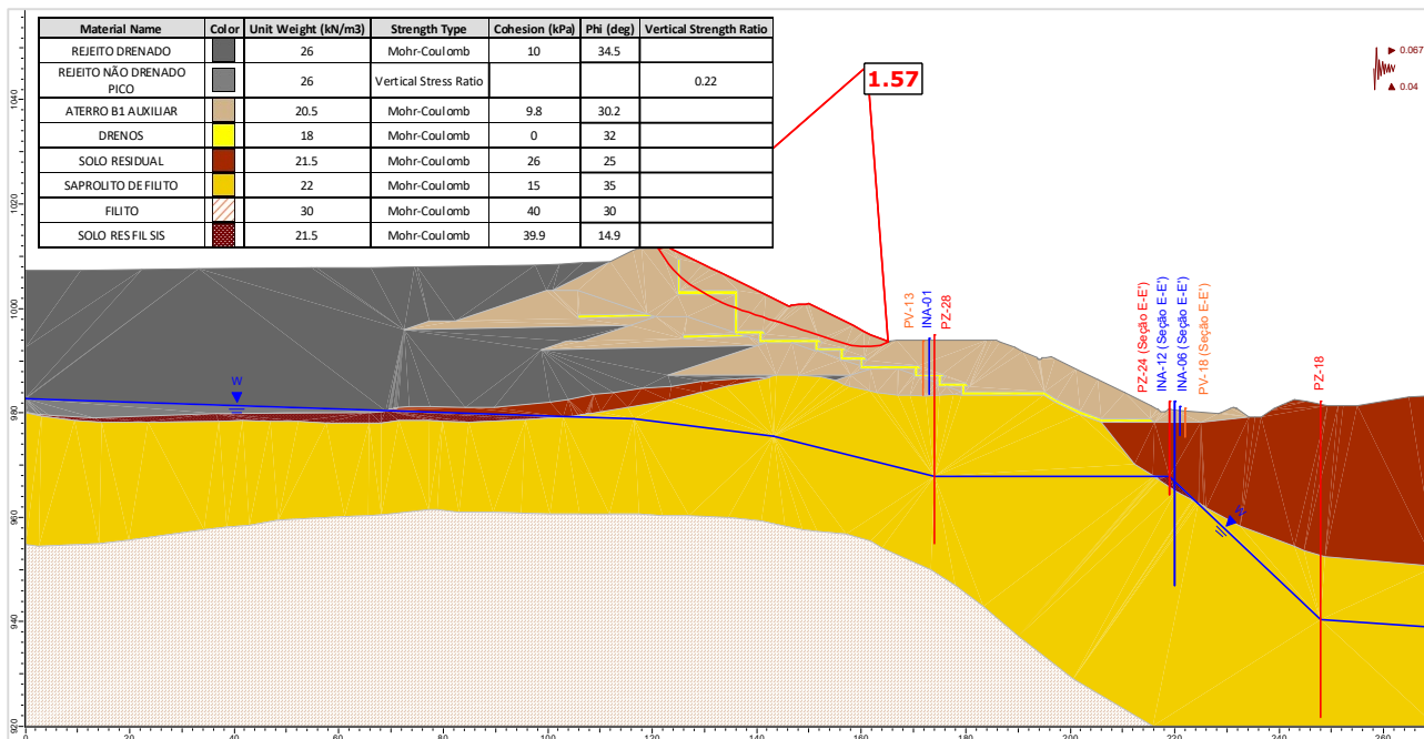
Figura 5.148 – Seção F-F’ – Análise Não Drenada – Superfície de ruptura plano-circular otimizada – Freática 28/10/2024 – Razão de resistência não drenada de pico + sismo ↑ (critério vida útil).
