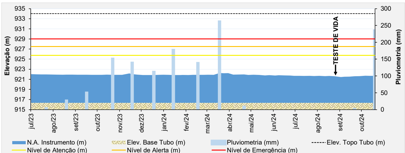
Figura 5.61 – Desempenho do piezômetro de tubo aberto - PZ-05 ECO.
