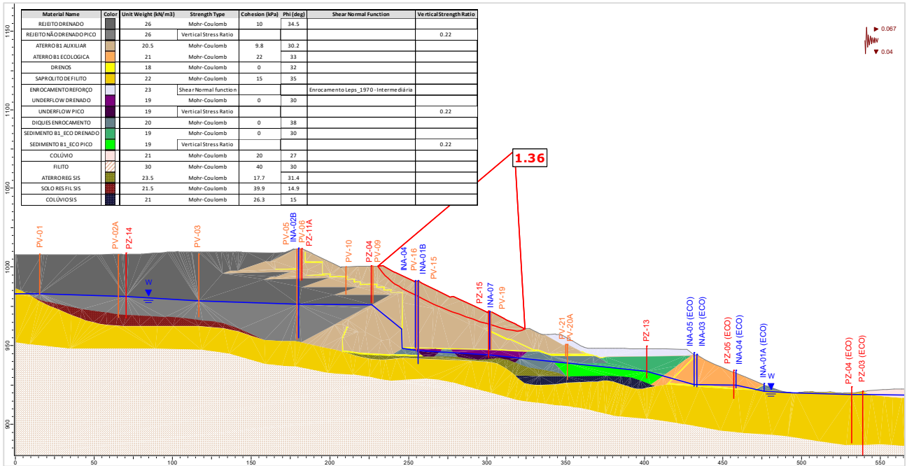
Figura 5.128 – Seção C-C’ – Análise Não Drenada – Superfície de ruptura plano-circular otimizada – Freática 28/10/2024 – Razão de resistência não drenada de pico + sismo ↓ (critério vida útil).
