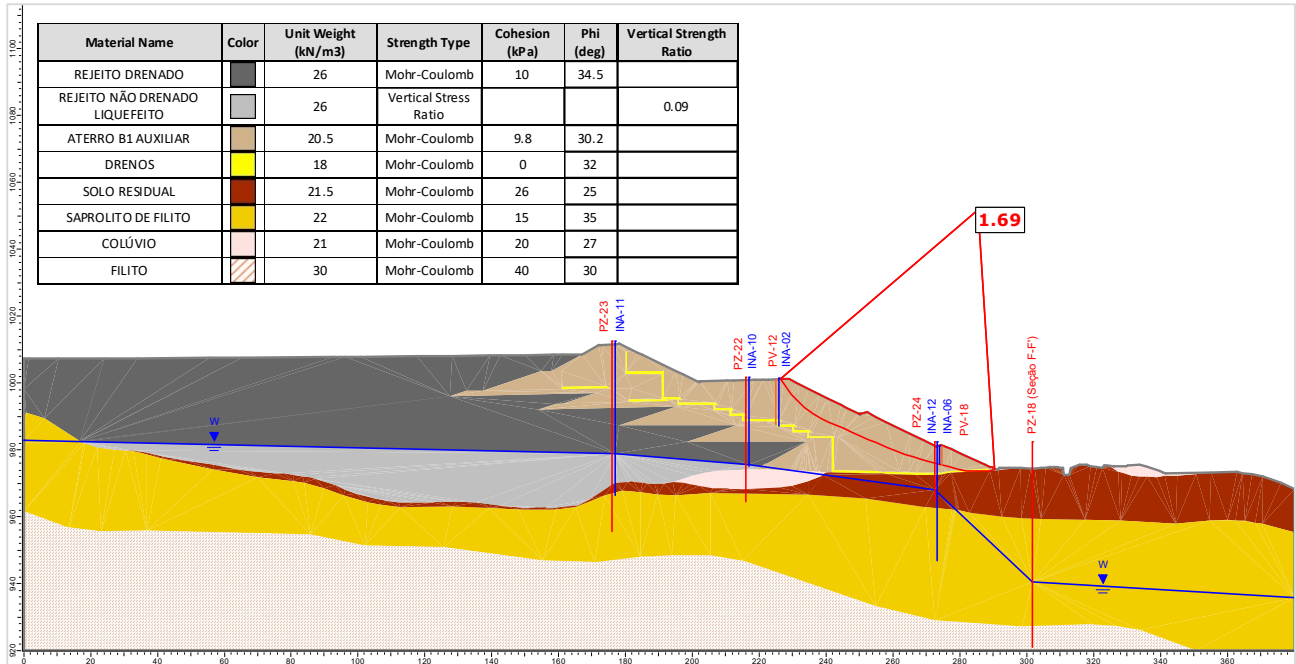
Figura 5.138 – Seção E-E' – Análise Não Drenada – Superfície de ruptura plano-circular otimizada – Freática 28/10/2024 – Razão de resistência não drenada liquefeita.
