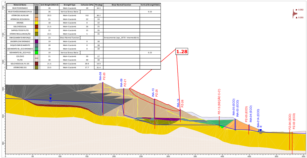
Figura 5.118 – Seção B-B' – Análise Não Drenada – Superfície de ruptura plano-circular otimizada – Freática 28/10/2024 – Razão de resistência não drenada de pico + sismo ↑ (critério CDA).
