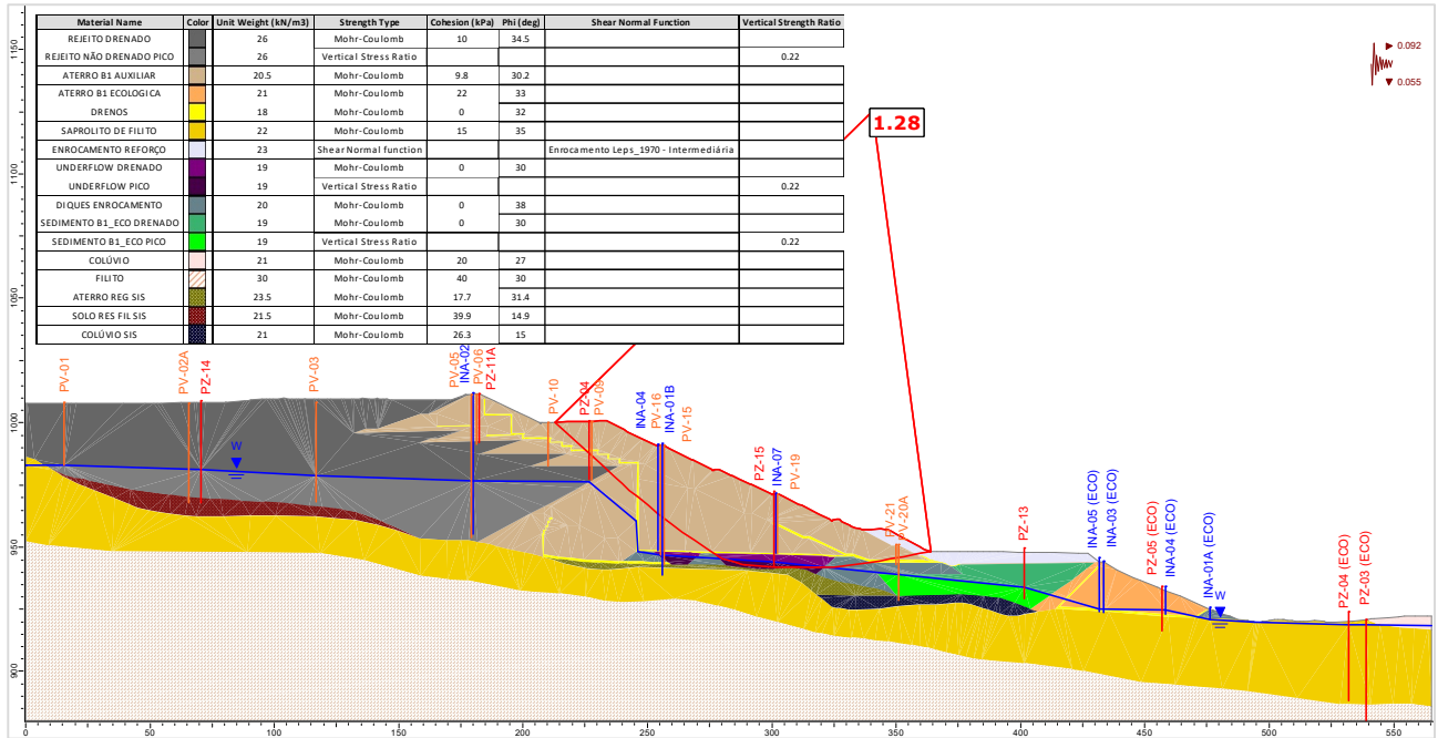
Figura 5.126 – Seção C-C' – Análise Não Drenada – Superfície de ruptura plano-circular otimizada – Freática 28/10/2024 – Razão de resistência não drenada de pico + sismo ↓ (critério CDA).
