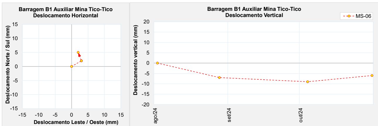
Figura 5.98 – Marco de controle de deformação – MS-06.
