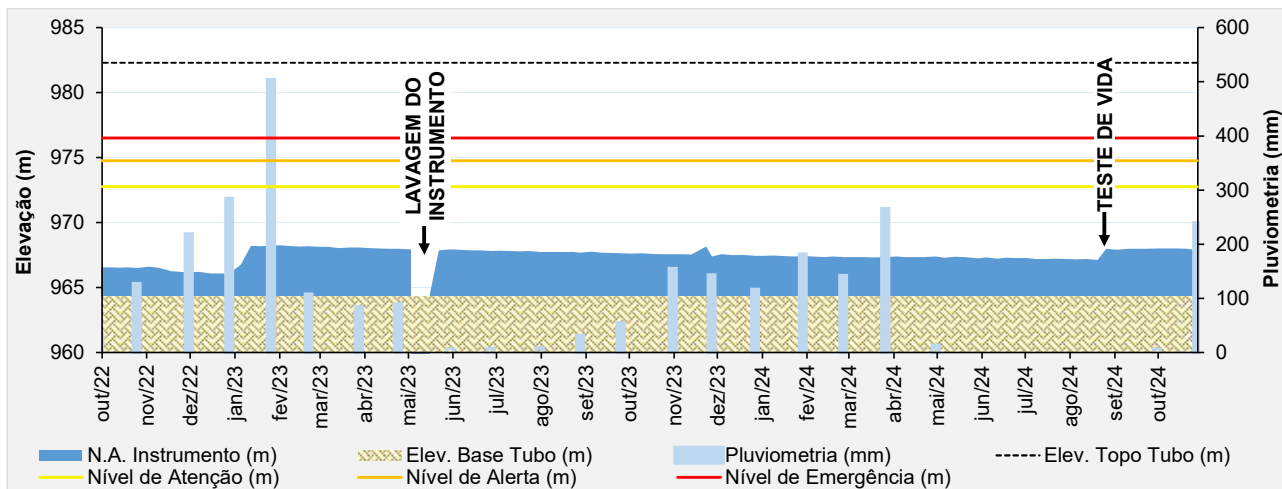
Figura 5.54 – Desempenho do piezômetro de tubo aberto - PZ-24.
