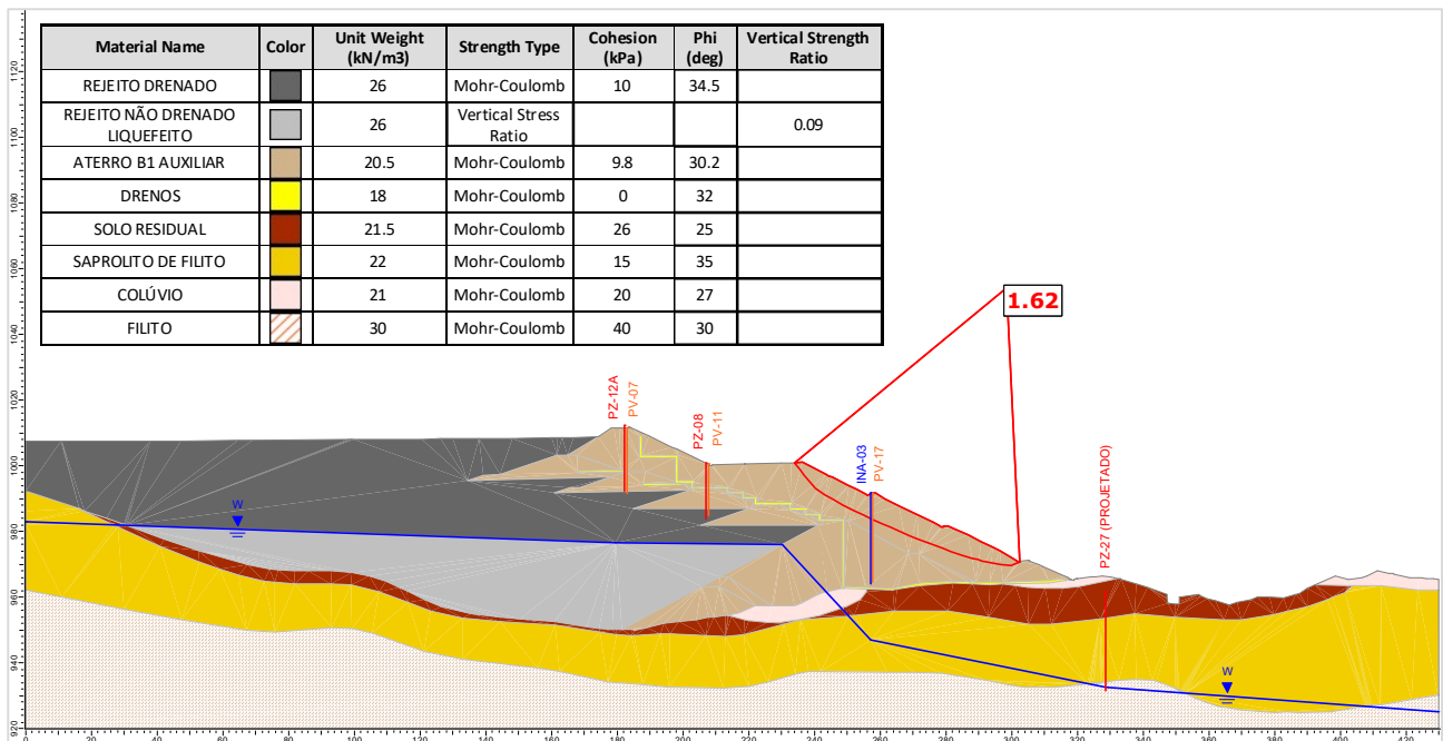
Figura 5.131 – Seção D-D' – Análise Não Drenada – Superfície de ruptura plano-circular otimizada – Freática 28/10/2024 – Razão de resistência não drenada liquefeita.
