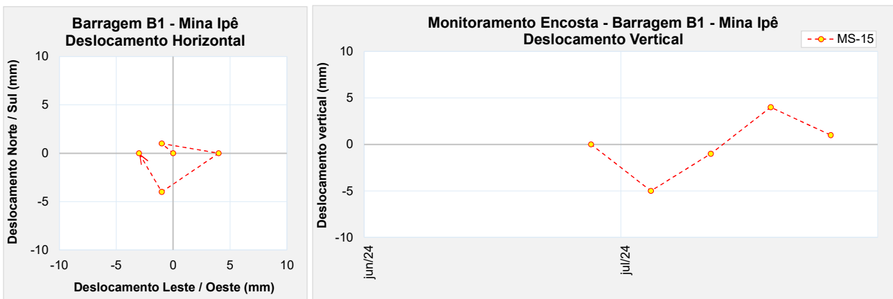
Figura 5.75 – Marco de controle de monitoramento da encosta MS-15.
