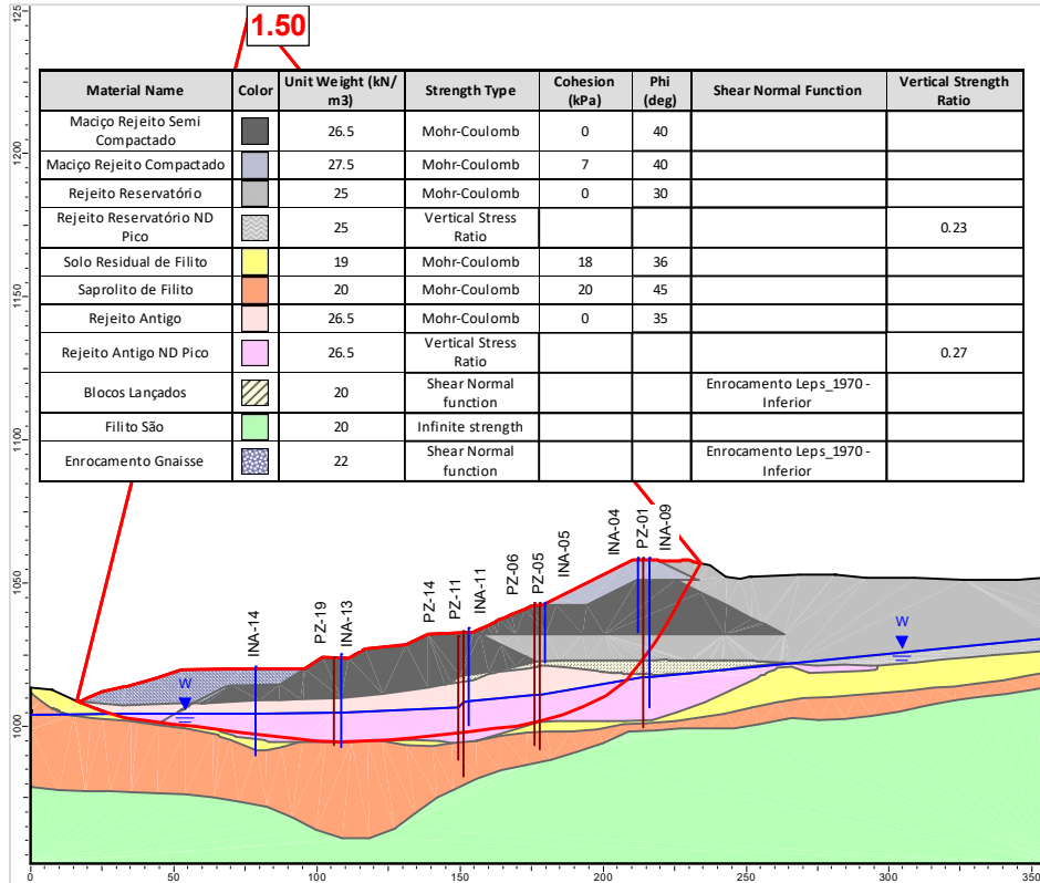
Figura 5.100 – Seção B-B' – Análise Não Drenada – Superfície de ruptura plano-circular otimizada – Freática atual 31/07/2024 – Razão de resistência não drenada de pico.
