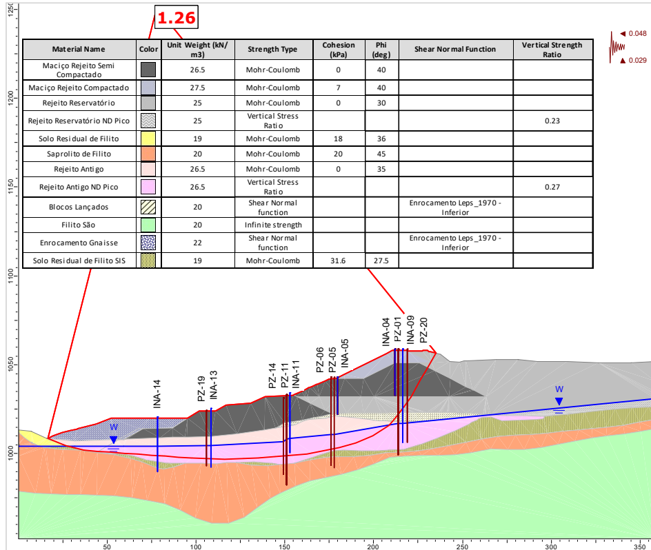
Figura 5.104 – Seção B-B' – Análise Não Drenada – Superfície de ruptura plano-circular otimizada – Freática 31/07/2024 – Razão de resistência não drenada de pico + sismo ↑ (critério vida útil).
