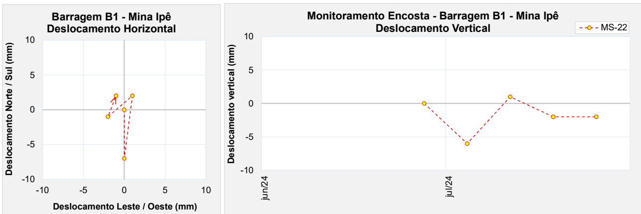
Figura 5.82 – Marco de controle de monitoramento da encosta MS-22.
