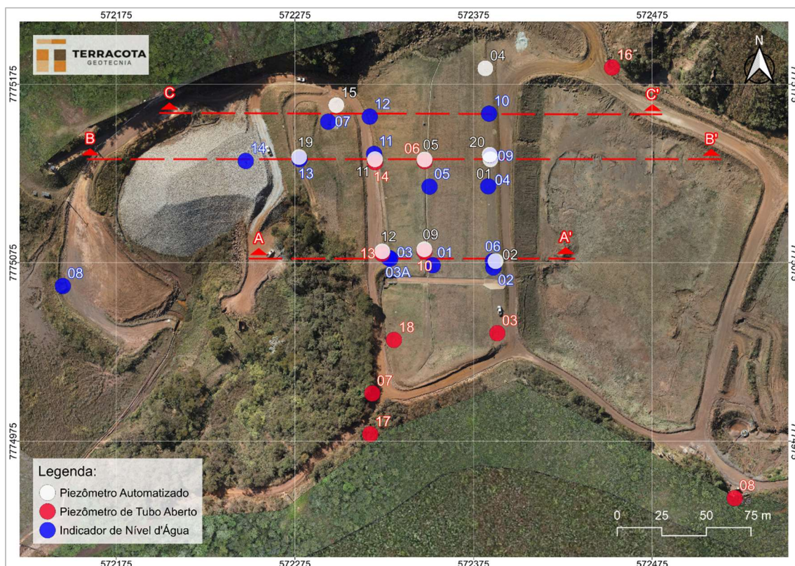
Figura 5.89 – Seções Instrumentadas Barragem B1 – Mina Ipê – Planta.
