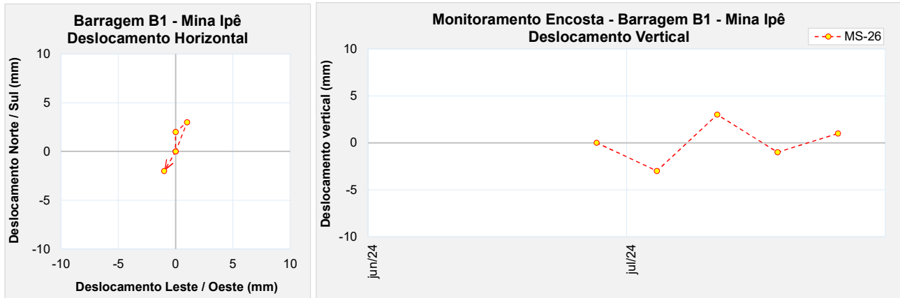
Figura 5.86 – Marco de controle de monitoramento da encosta MS-26.
