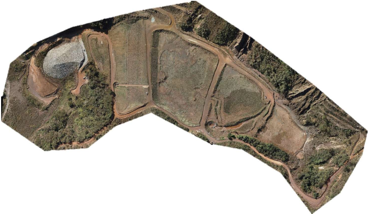
Figura 4.2 – Imagem da Barragem B1 – Mina Ipê. (Fonte: Ortofoto MMI – Julho/2024).
