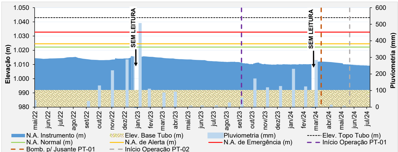
Figura 5.35 - Desempenho do piezômetro automatizado - PZ-05.
