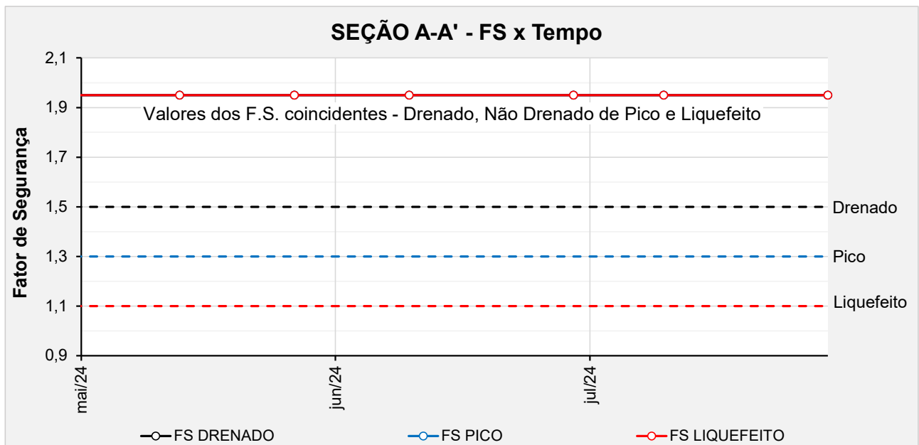
Figura 5.113 – Seção A-A' - Histórico dos F.S. obtidos nas análises de estabilidade no período avaliado.
