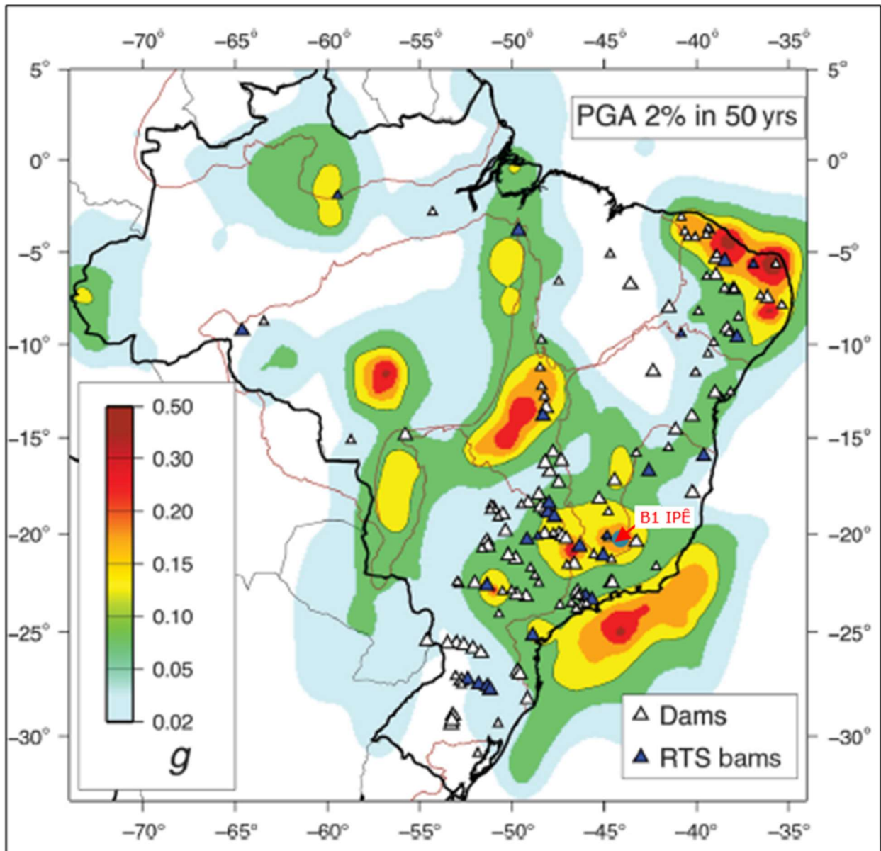
Figura 5.91 – Mapa de Ameaça Sísmica Brasileiro com probabilidade de excedência de 2% durante 50 anos (Assumpção Et al., 2018).
