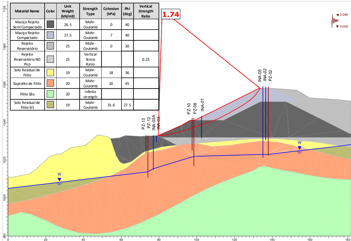
Figura 5.98 – Seção A-A' – Análise Não Drenada – Superfície de ruptura plano-circular otimizada – Freática 31/07/2024 – Razão de resistência não drenada de pico + sismo ↓ (critério vida útil).
