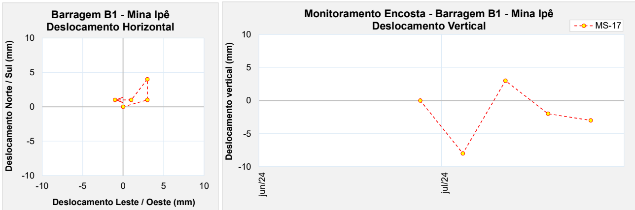
Figura 5.77 – Marco de controle de monitoramento da encosta MS-17.
