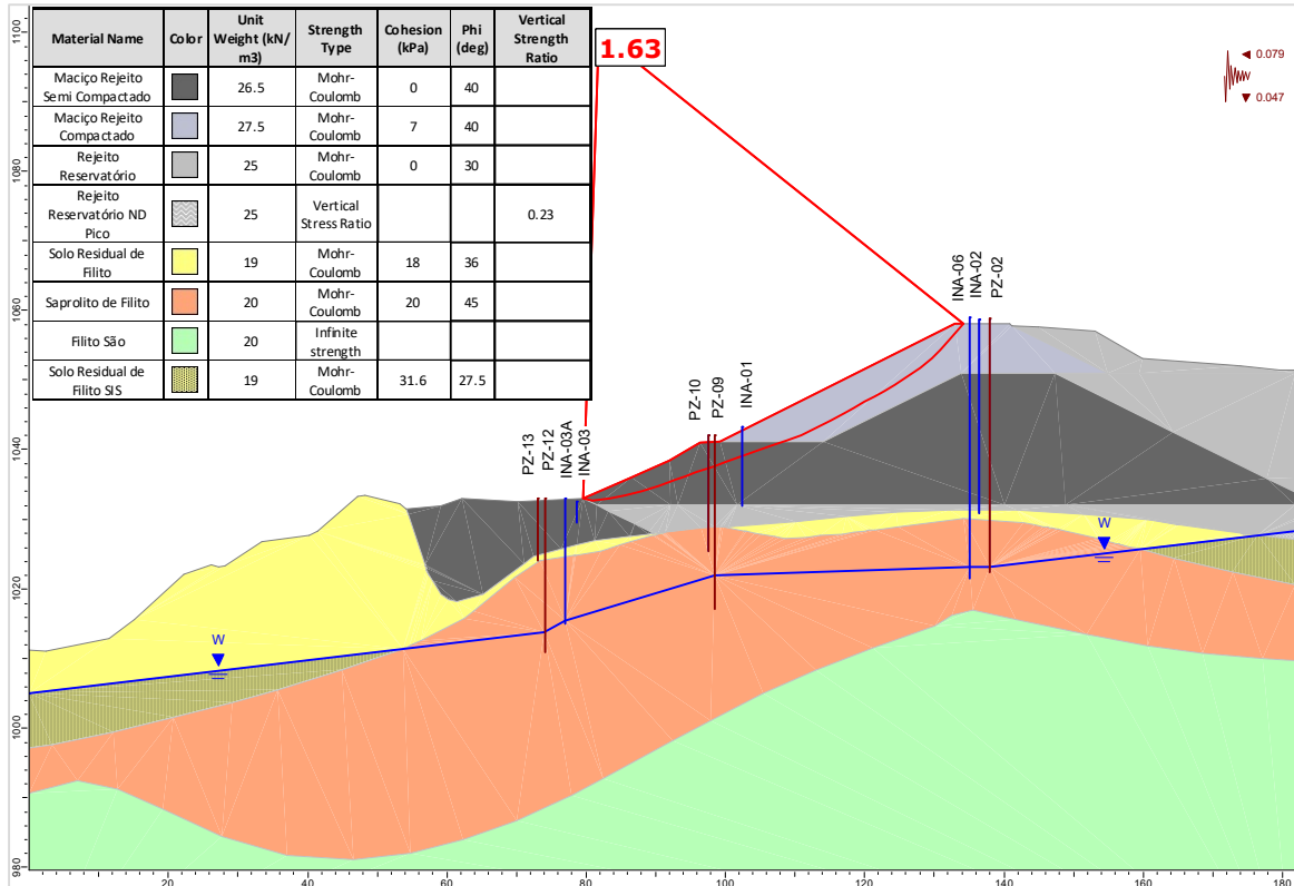
Figura 5.96 – Seção A-A' – Análise Não Drenada – Superfície de ruptura plano-circular otimizada – Freática 31/07/2024 – Razão de resistência não drenada de pico + sismo ↓ (critério CDA).
