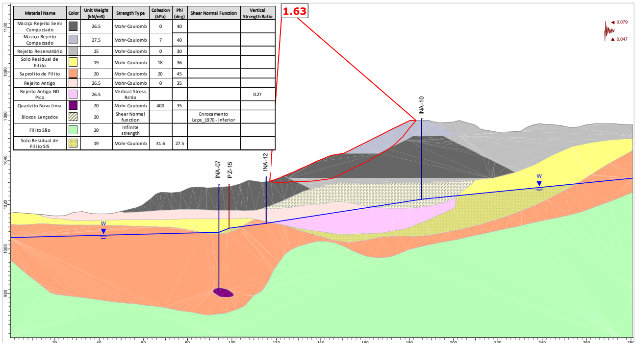
Figura 5.109 – Seção C-C' – Análise Não Drenada – Superfície de ruptura plano-circular otimizada – Freática 31/07/2024 – Razão de resistência não drenada de pico + sismo ↑ (critério CDA).
