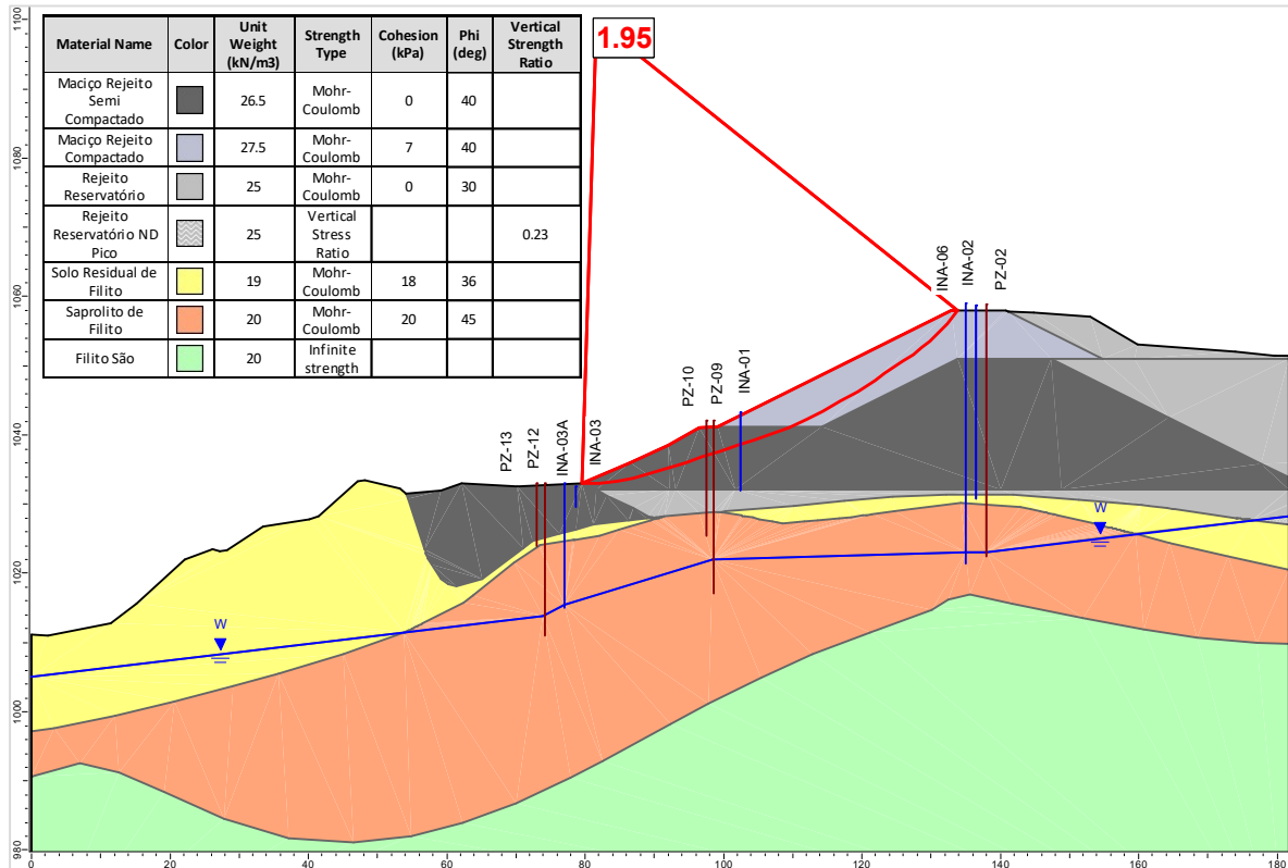
Figura 5.93 – Seção A-A' – Análise Não Drenada – Superfície de ruptura plano-circular otimizada – Freática 31/07/2024 – Razão de resistência não drenada de pico.
