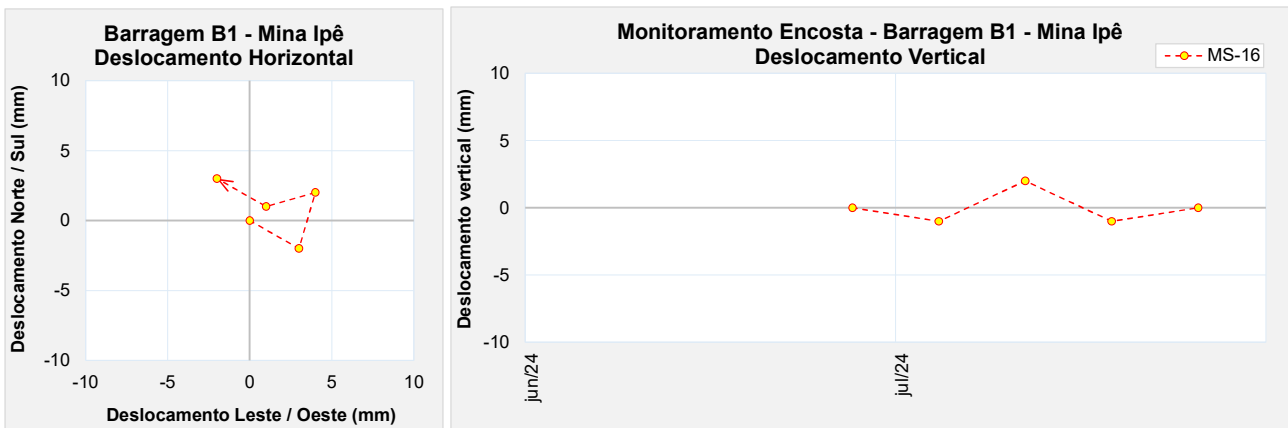
Figura 5.76 – Marco de controle de monitoramento da encosta MS-16.
