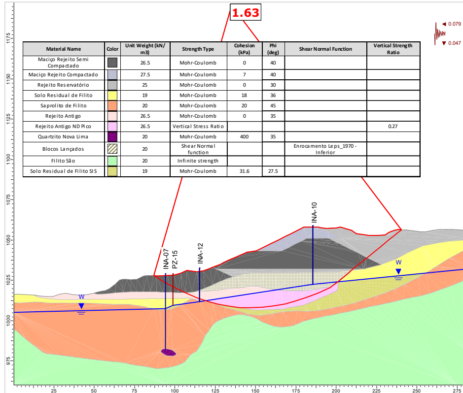
Figura 5.110 – Seção C-C' – Análise Não Drenada – Superfície de ruptura plano-circular otimizada – Freática 31/07/2024 – Razão de resistência não drenada de pico + sismo ↓ (critério CDA).
