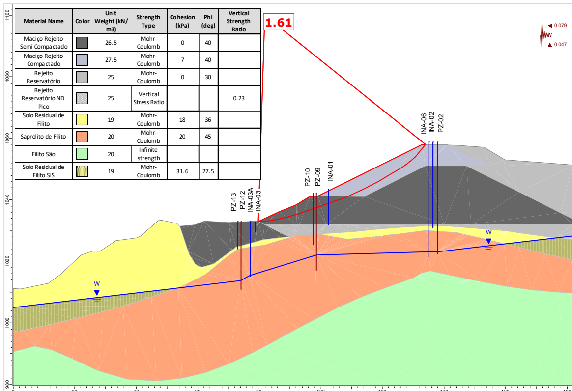
Figura 5.95 – Seção A-A' – Análise Não Drenada – Superfície de ruptura plano-circular otimizada – Freática 31/07/2024 – Razão de resistência não drenada de pico + sismo ↑ (critério CDA).
