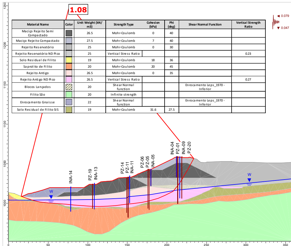
Figura 5.103 – Seção B-B' – Análise Não Drenada – Superfície de ruptura plano-circular otimizada – Freática 31/07/2024 – Razão de resistência não drenada de pico + sismo ↓ (critério CDA).
