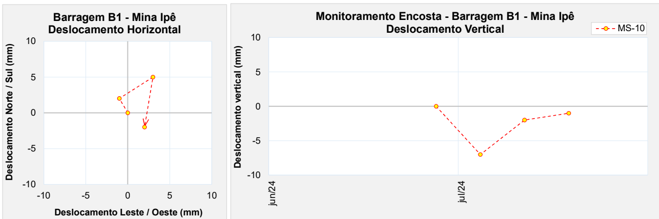
Figura 5.70 – Marco de controle de monitoramento da encosta MS-10.
