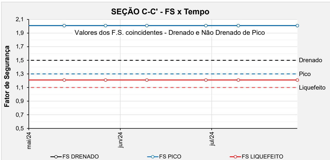
Figura 5.115 – Seção C-C' - Histórico dos F.S. obtidos nas análises de estabilidade no período avaliado.
