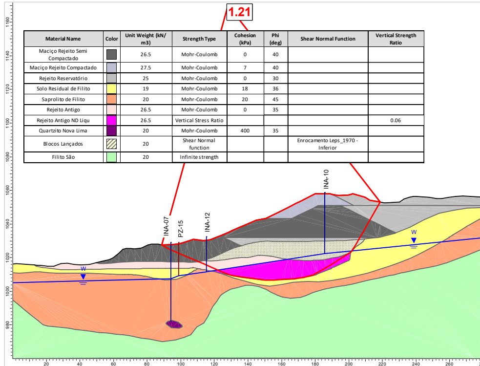
Figura 5.108 – Seção C-C' – Análise Não Drenada – Superfície de ruptura plano-circular otimizada – Freática 31/07/2024 – Razão de resistência não drenada liquefeito.
