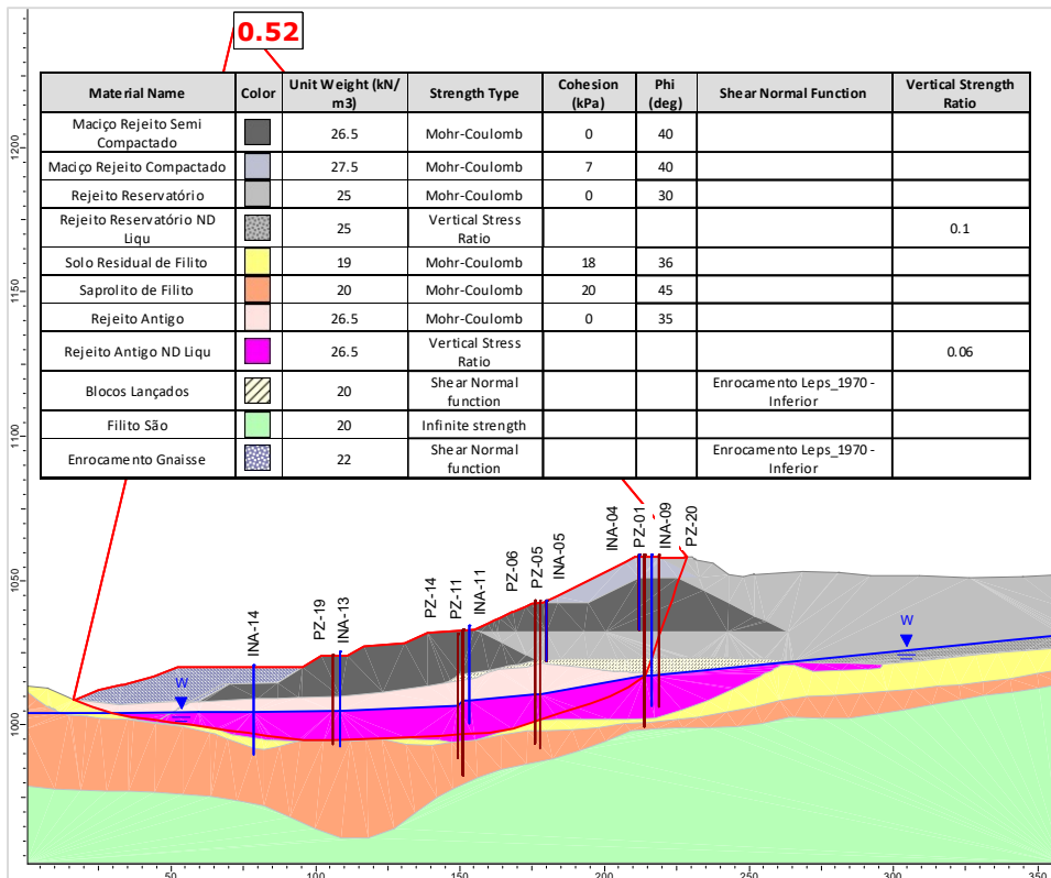
Figura 5.101 – Seção B-B' – Análise Não Drenada – Superfície de ruptura plano-circular otimizada – Freática atual 31/07/2024 – Razão de resistência não drenada liquefeito.
