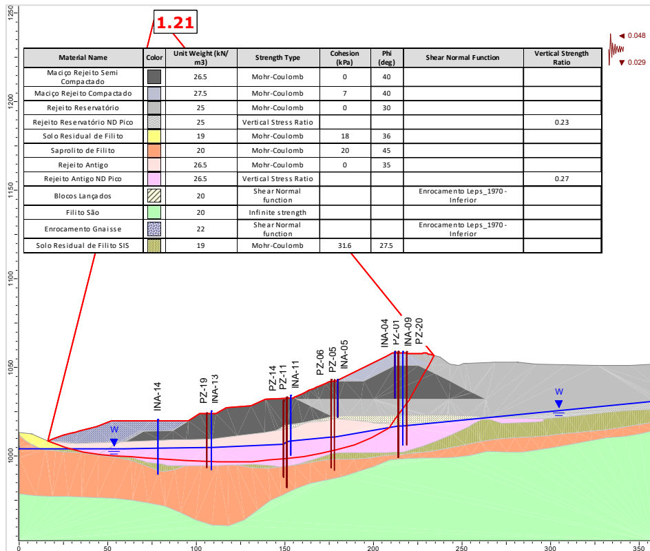
Figura 5.105 – Seção B-B' – Análise Não Drenada – Superfície de ruptura plano-circular otimizada – Freática 31/07/2024 – Razão de resistência não drenada de pico + sismo ↓ (critério vida útil).
