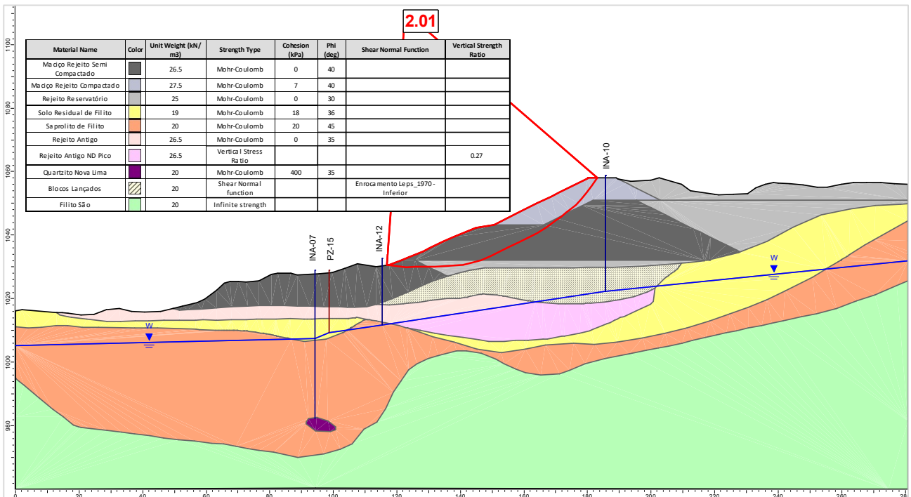
Figura 5.107 – Seção C-C' – Análise Não Drenada – Superfície de ruptura plano-circular otimizada – Freática 31/07/2024 – Razão de resistência não drenada de pico.
