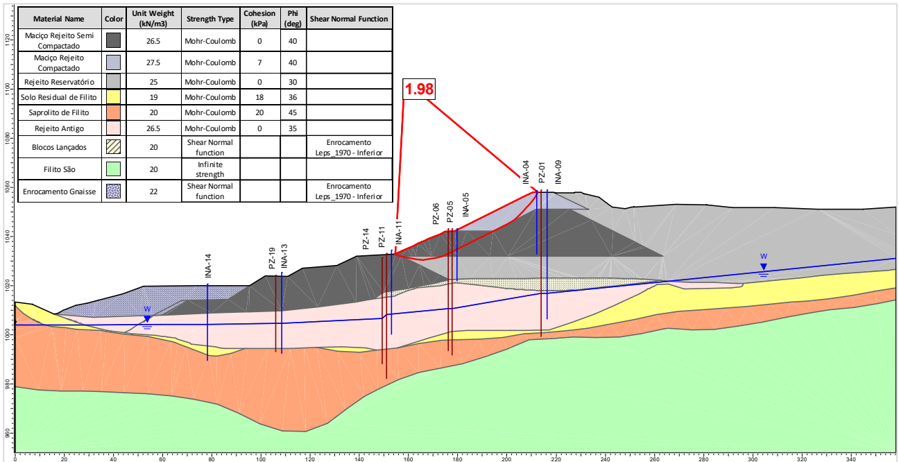
Figura 5.99 – Seção B-B' – Análise Drenada – Superfície de ruptura plano-circular otimizada – Freática 31/07/2024.
