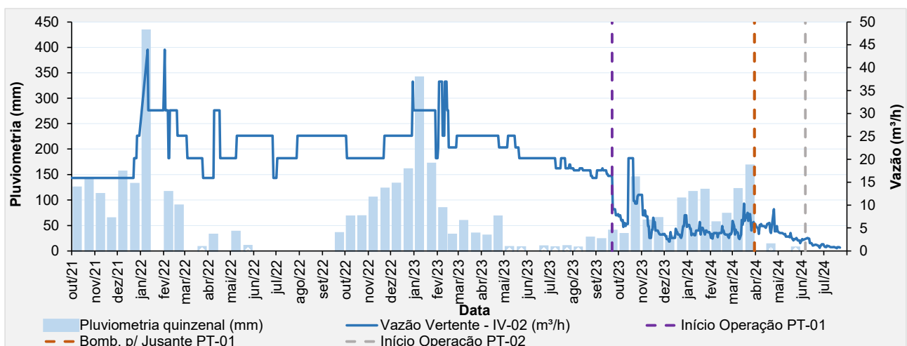
Figura 5.52 – Análise das vazões do IV-02 (Vertente).
