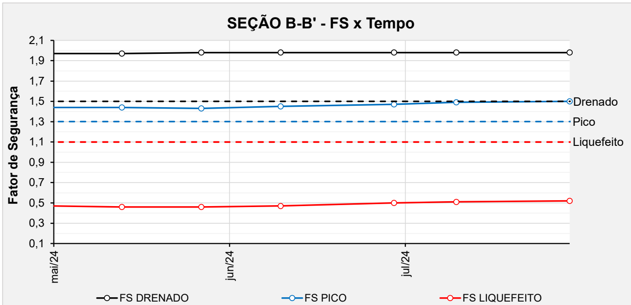
Figura 5.114 – Seção B-B' - Histórico dos F.S. obtidos nas análises de estabilidade no período avaliado.
