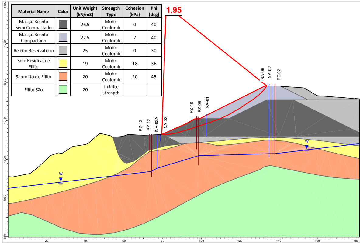
Figura 5.92 – Seção A-A' – Análise Drenada – Superfície de ruptura plano-circular otimizada – Freática 31/07/2024.
