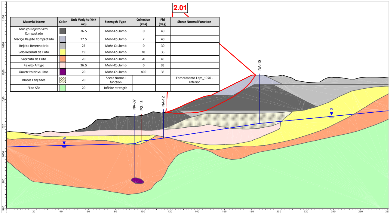
Figura 5.106 – Seção C-C' – Análise Drenada – Superfície de ruptura plano-circular otimizada – Freática 31/07/2024.
