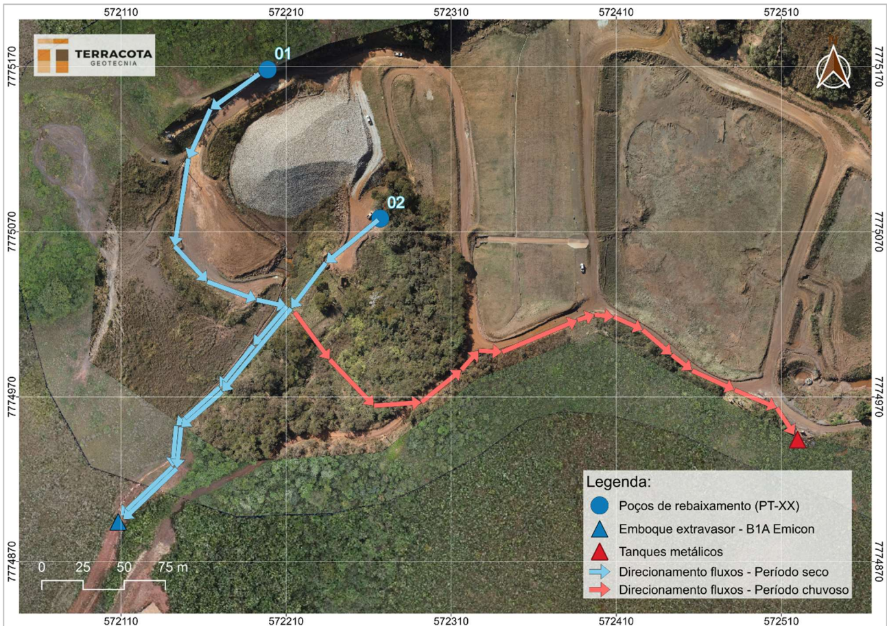
Figura 5.87 – Esquema de direcionamento dos fluxos proveniente dos poços de bombeamento.
