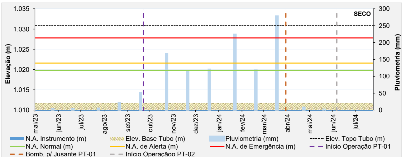
Figura 5.28 – Desempenho do indicador de nível d'água – INA-12.
