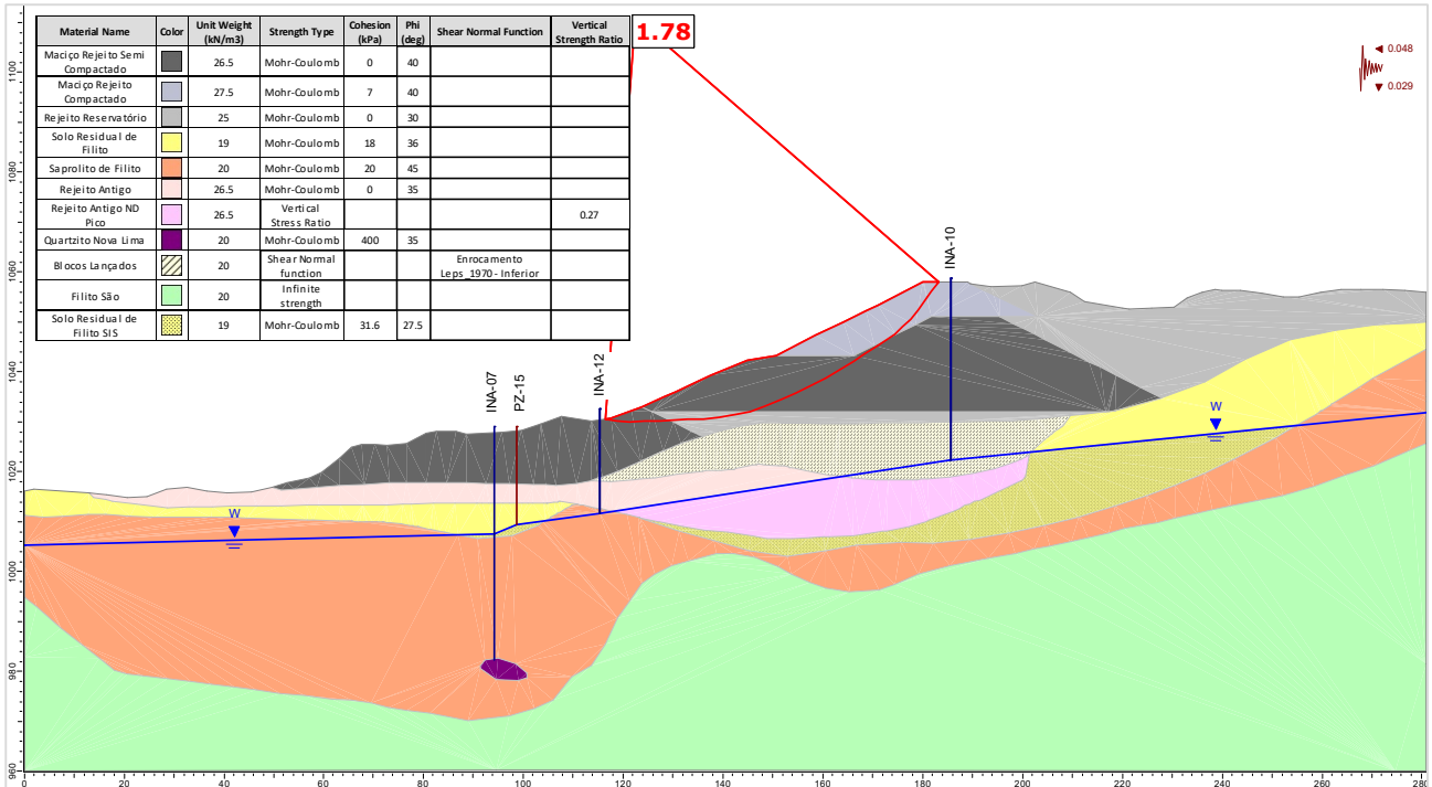
Figura 5.112 – Seção C-C' – Análise Não Drenada – Superfície de ruptura plano-circular otimizada – Freática 31/07/2024 – Razão de resistência não drenada de pico + sismo ↓ (critério vida útil).
