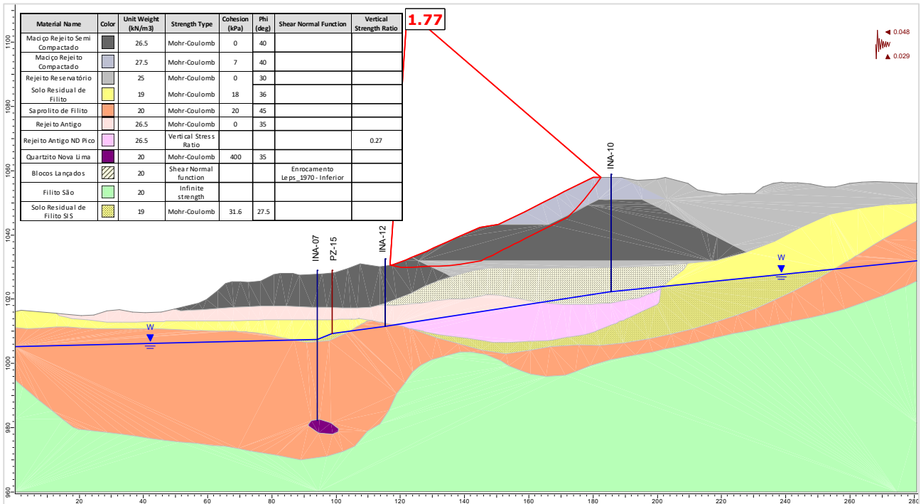
Figura 5.111 – Seção C-C' – Análise Não Drenada – Superfície de ruptura plano-circular otimizada – Freática 31/07/2024 – Razão de resistência não drenada de pico + sismo ↑ (critério vida útil).
