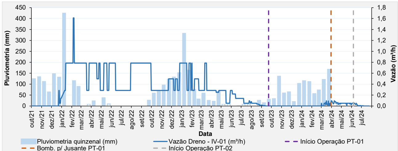
Figura 5.51 – Análise das vazões do IV-01 (Dreno).
