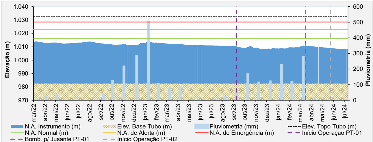
Figura 5.41 - Desempenho do piezômetro automatizado - PZ-11.
