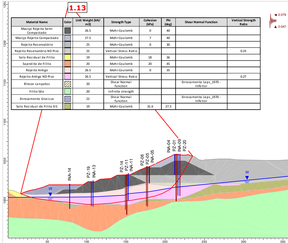
Figura 5.102 – Seção B-B' – Análise Não Drenada – Superfície de ruptura plano-circular otimizada – Freática 31/07/2024 – Razão de resistência não drenada de pico + sismo ↑ (critério CDA).
