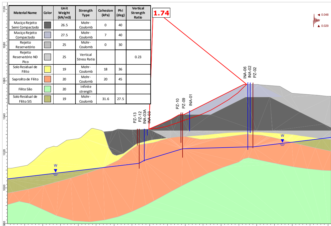
Figura 5.97 – Seção A-A' – Análise Não Drenada – Superfície de ruptura plano-circular otimizada – Freática 31/07/2024 – Razão de resistência não drenada de pico + sismo ↑ (critério vida útil).
