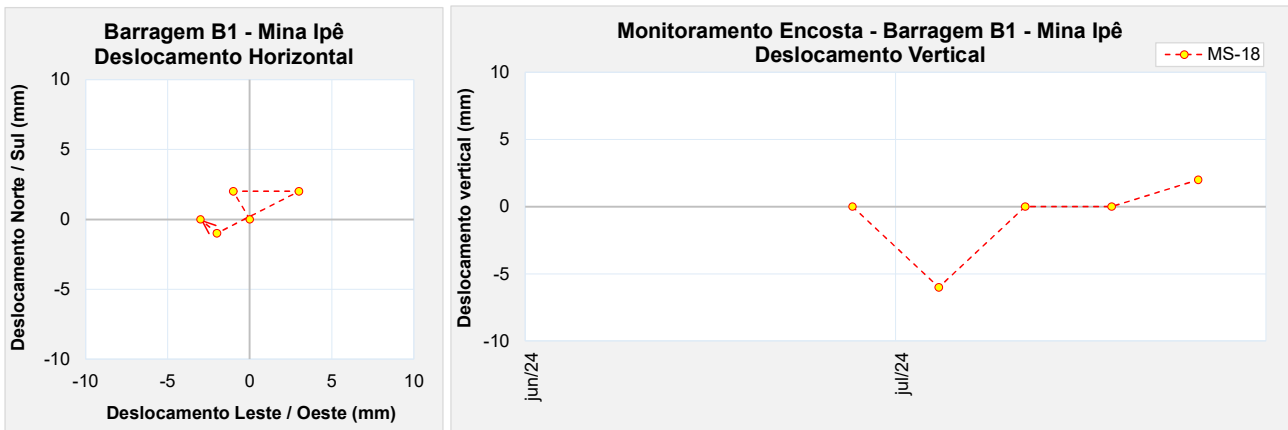
Figura 5.78 – Marco de controle de monitoramento da encosta MS-18.
