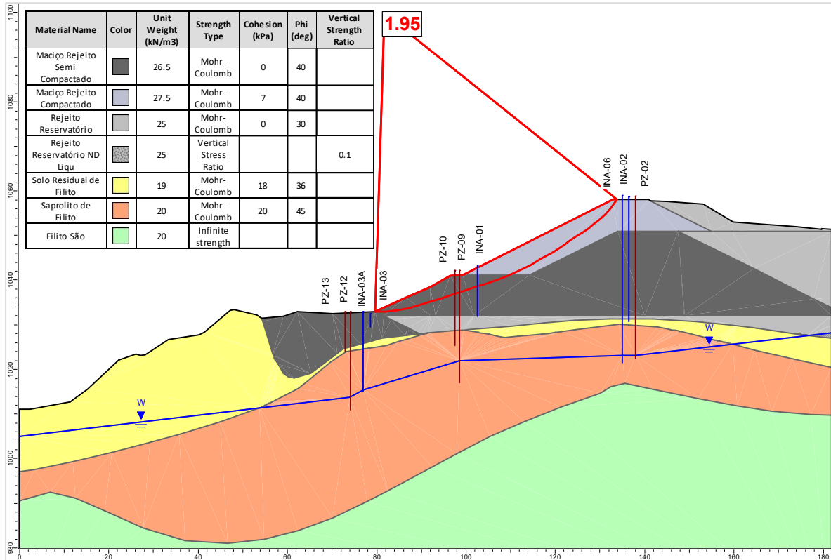
Figura 5.94 – Seção A-A' – Análise Não Drenada – Superfície de ruptura plano-circular otimizada – Freática 31/07/2024 – Razão de resistência não drenada liquefeito.
