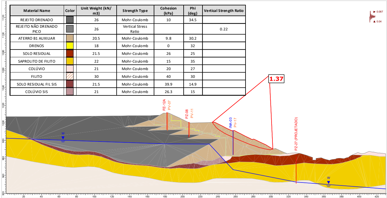
Figura 5.134 – Seção D-D' – Análise Não Drenada – Superfície de ruptura plano-circular otimizada – Freática 30/07/2024 – Razão de resistência não drenada de pico + sismo ↑ (critério vida útil).
