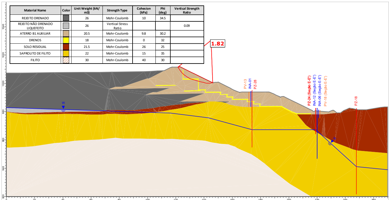
Figura 5.145 – Seção F-F' – Análise Não Drenada – Superfície de ruptura plano-circular otimizada – Freática 30/07/2024 – Razão de resistência não drenada liquefeita.
