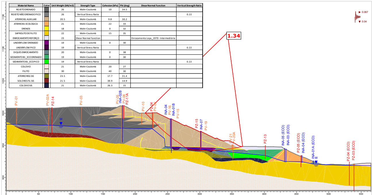
Figura 5.128 – Seção C-C' – Análise Não Drenada – Superfície de ruptura plano-circular otimizada – Freática 30/07/2024 – Razão de resistência não drenada de pico + sismo ↓ (critério vida útil).
