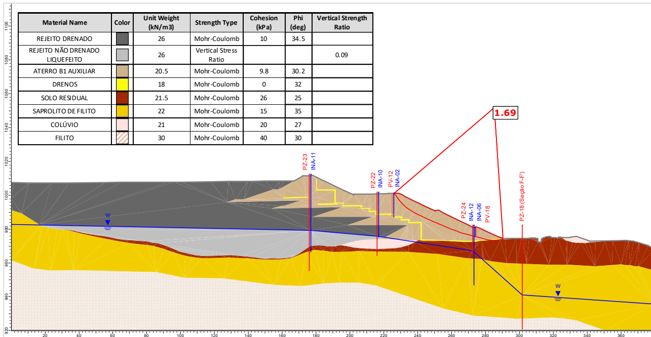
Figura 5.138 – Seção E-E' – Análise Não Drenada – Superfície de ruptura plano-circular otimizada – Freática 30/07/2024 – Razão de resistência não drenada liquefeita.
