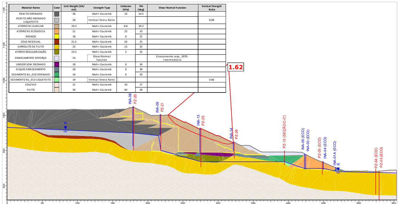
Figura 5.117 – Seção B-B' – Análise Não Drenada – Superfície de ruptura plano-circular otimizada – Freática 30/07/2024 – Razão de resistência não drenada liquefeita.
