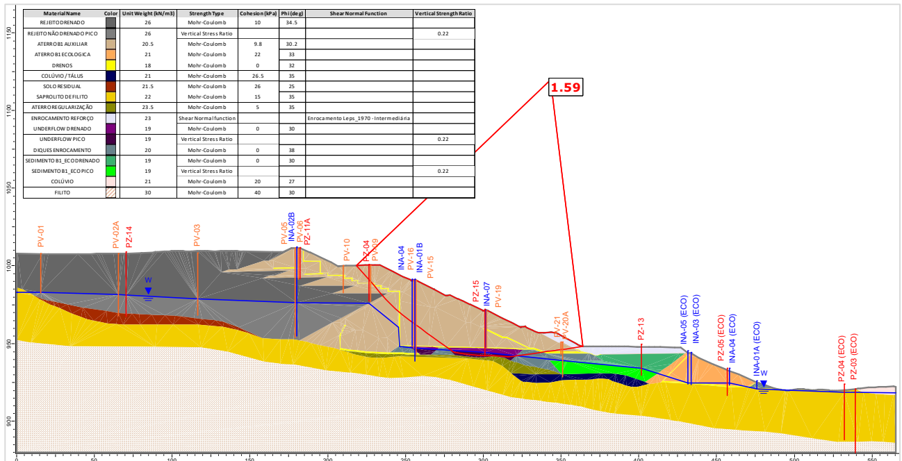
Figura 5.123 – Seção C-C' – Análise Não Drenada – Superfície de ruptura plano-circular otimizada – Freática 30/07/2024 – Razão de resistência não drenada de pico.
