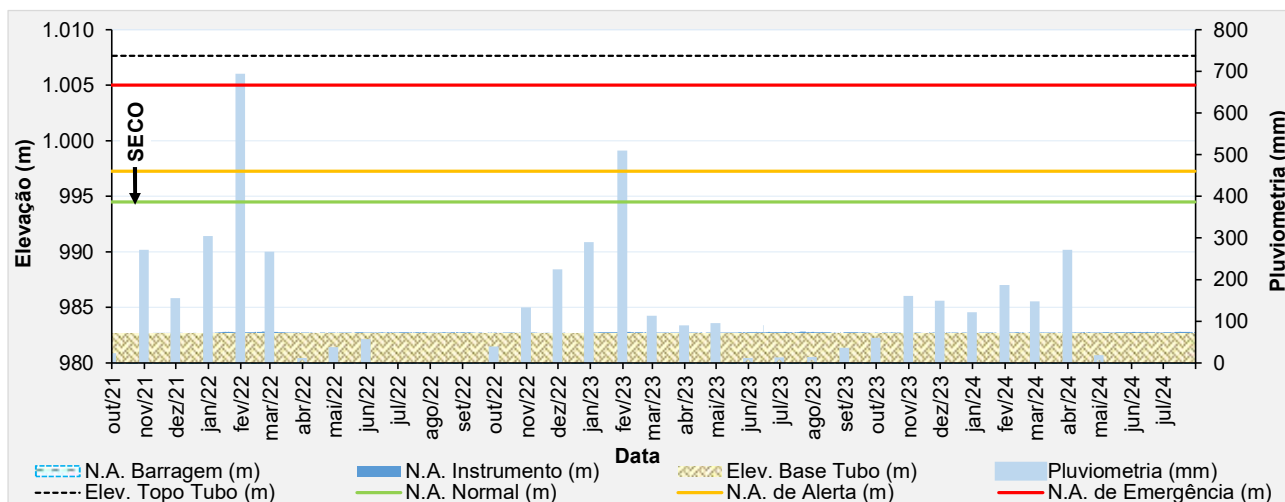
Figura 5.17 – Desempenho do piezômetro elétrico - PV-01.
