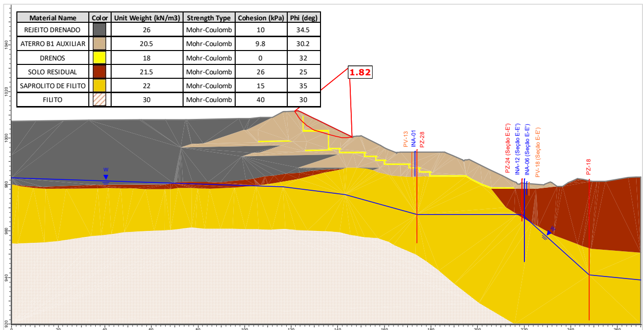
Figura 5.143 – Seção F-F' – Análise Drenada – Superfície de ruptura plano-circular otimizada – Freática 30/07/2024.
