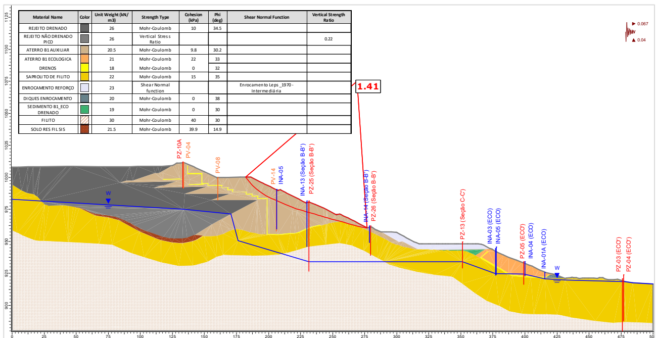
Figura 5.113 – Seção A-A' – Análise Não Drenada – Superfície de ruptura plano-circular otimizada – Freática 30/07/2024 – Razão de resistência não drenada de pico + sismo ↑ (critério vida útil).
