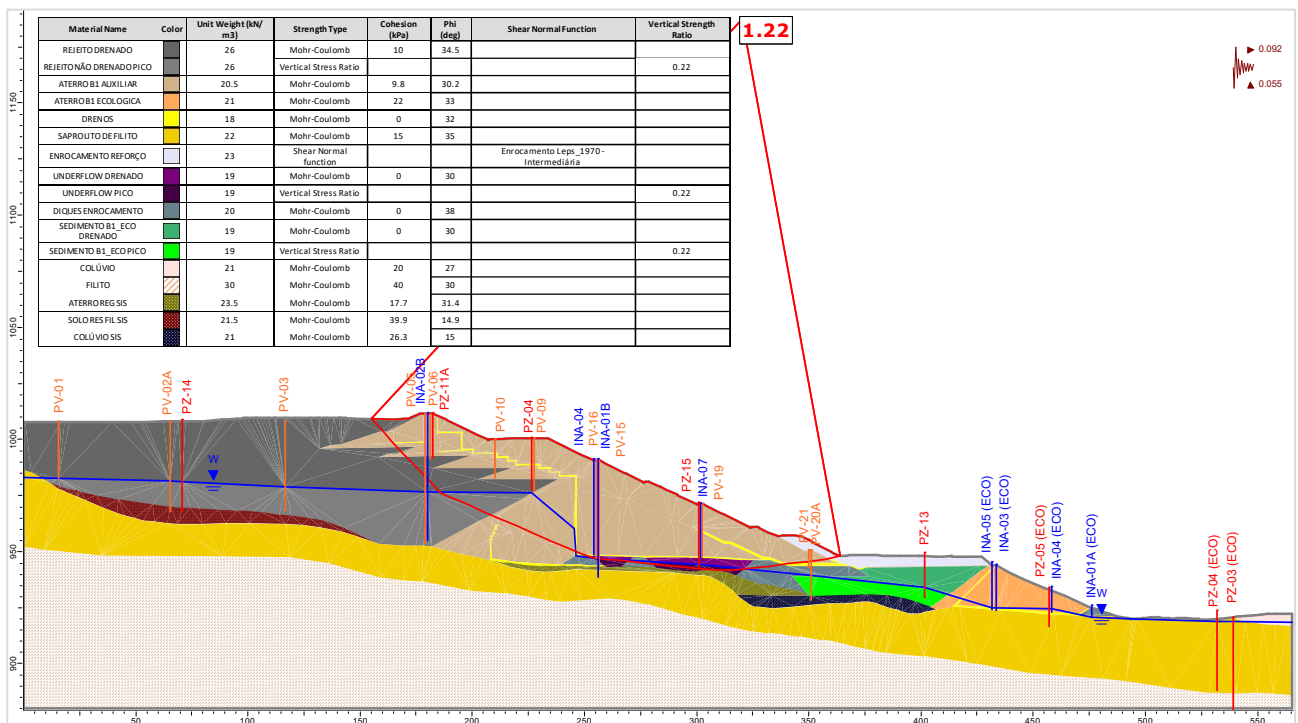
Figura 5.125 – Seção C-C' – Análise Não Drenada – Superfície de ruptura plano-circular otimizada – Freática 30/07/2024 – Razão de resistência não drenada de pico + sismo ↑ (critério CDA).
