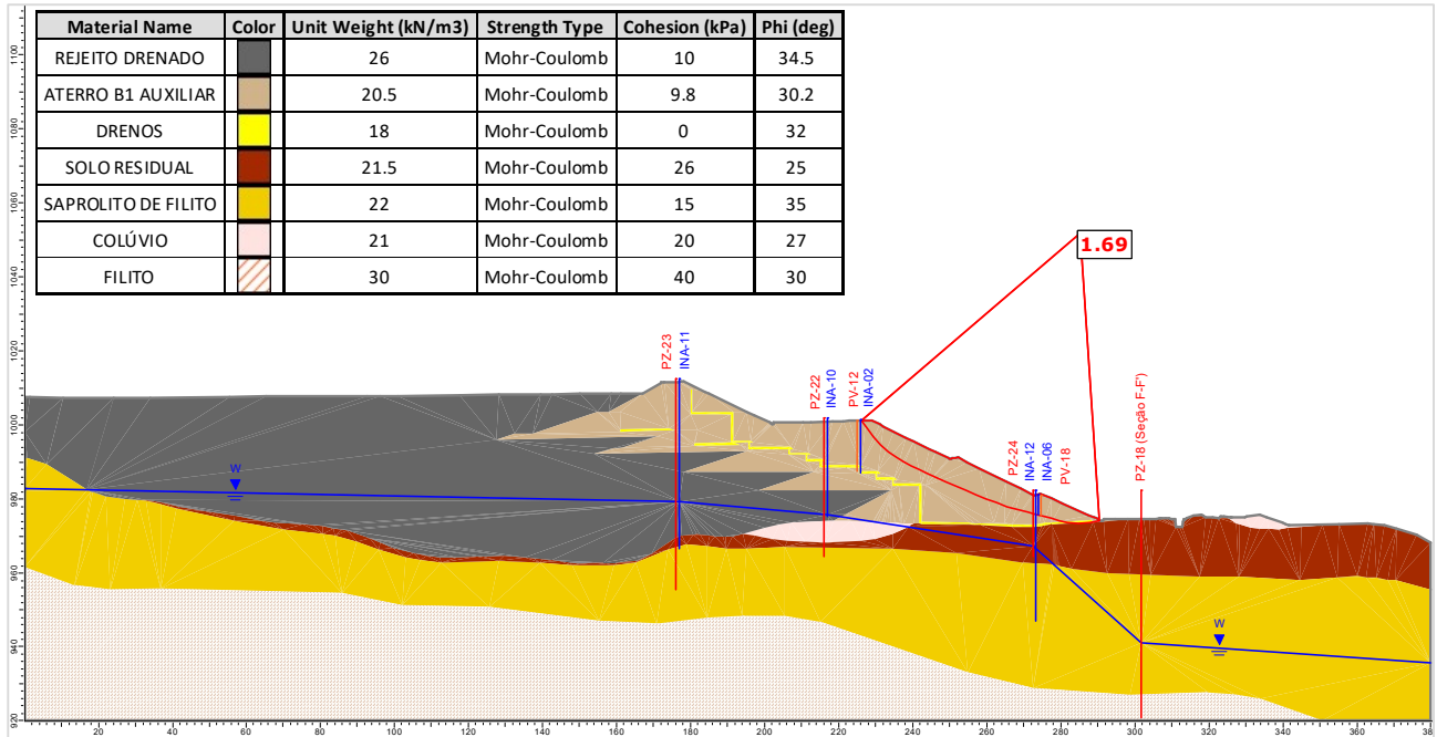
Figura 5.136 – Seção E-E' – Análise Drenada – Superfície de ruptura plano-circular otimizada – Freática 30/07/2024.
