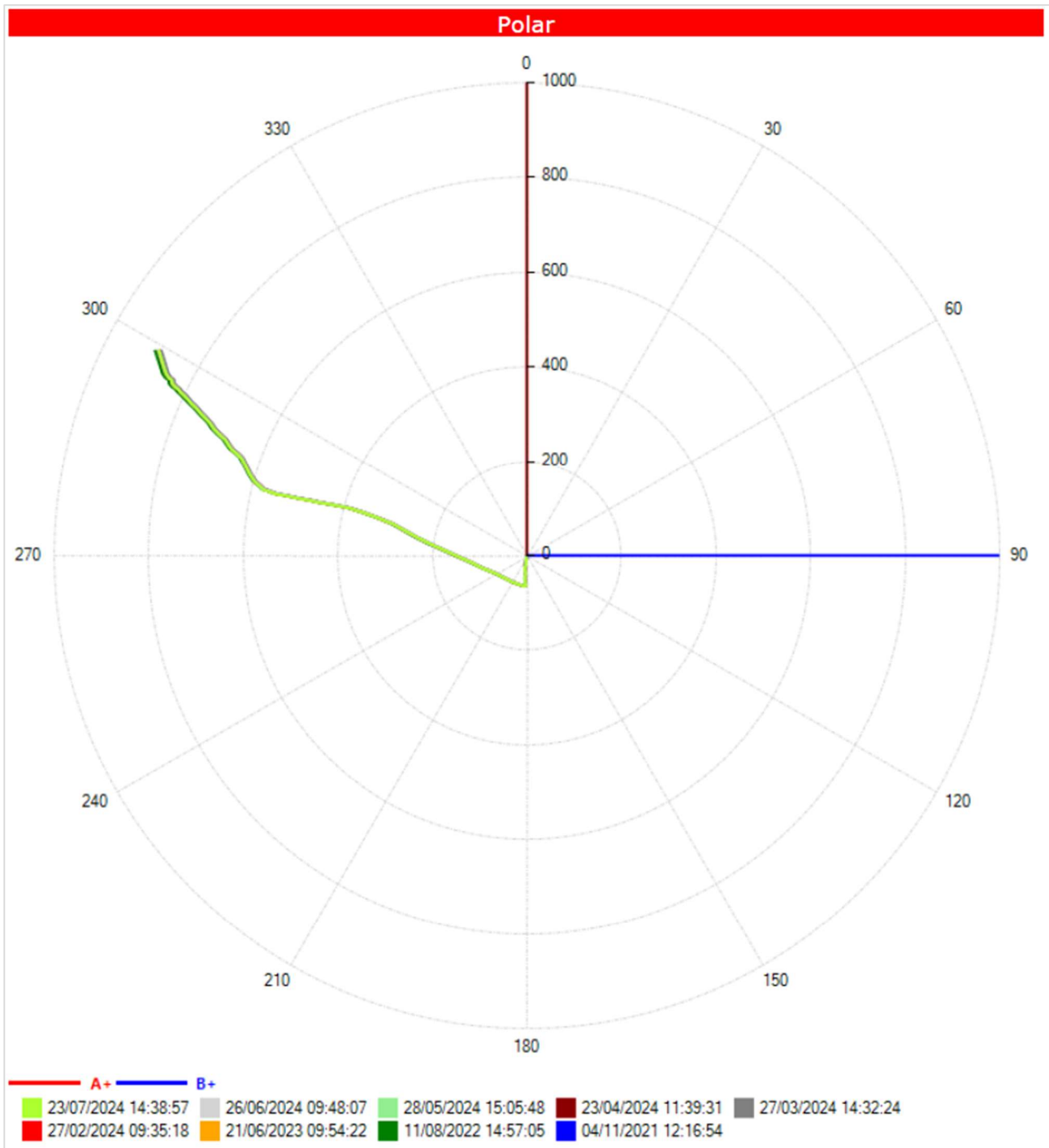
Figura 5.102 – Deslocamentos em relação a coordenadas polares acumulados do INC-01 (ref. 23/07/2024).
