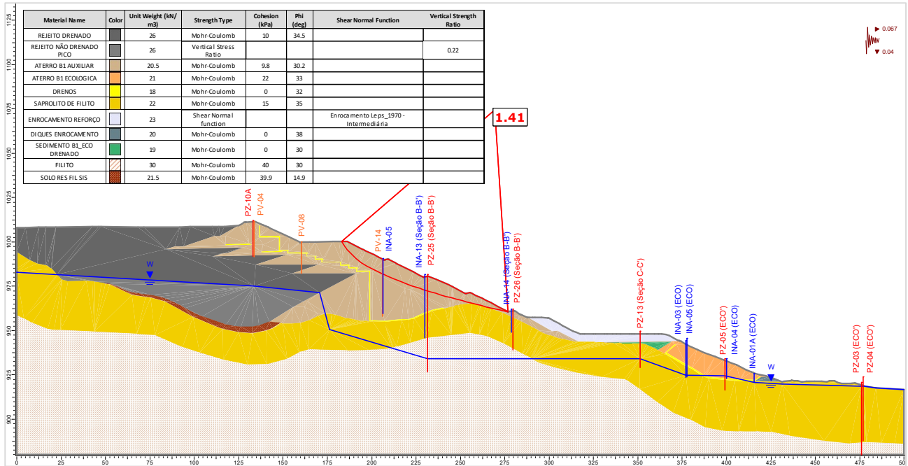
Figura 5.114 – Seção A-A’ – Análise Não Drenada – Superfície de ruptura plano-circular otimizada – Freática 30/07/2024 – Razão de resistência não drenada de pico + sismo ↓ (critério vida útil).
