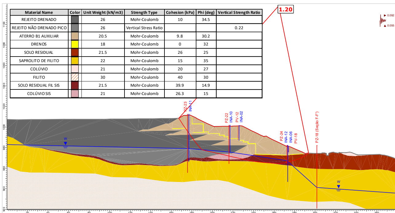
Figura 5.139 – Seção E-E' – Análise Não Drenada – Superfície de ruptura plano-circular otimizada – Freática 30/07/2024 – Razão de resistência não drenada de pico + sismo ↑ (critério CDA).
