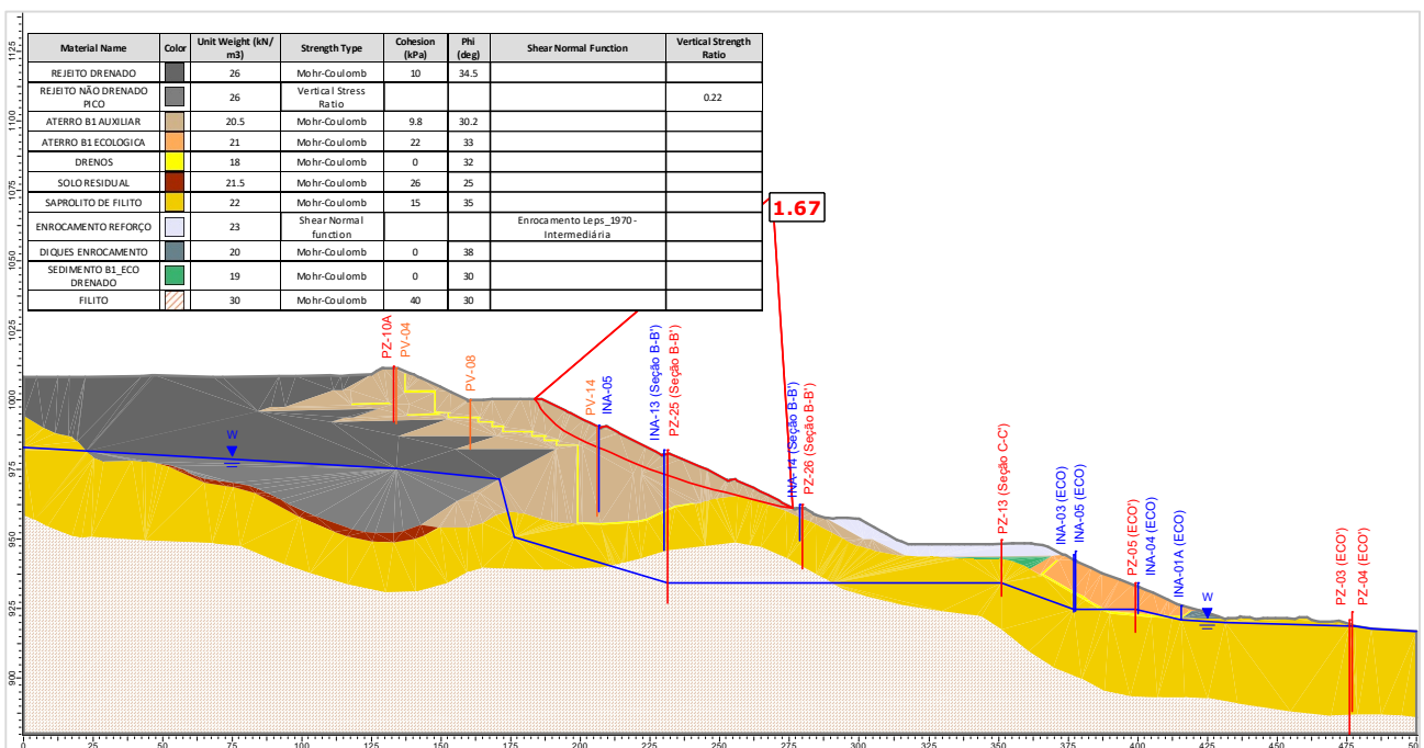
Figura 5.109 – Seção A-A' – Análise Não Drenada – Superfície de ruptura plano-circular otimizada – Freática 30/07/2024 – Razão de resistência não drenada de pico.
