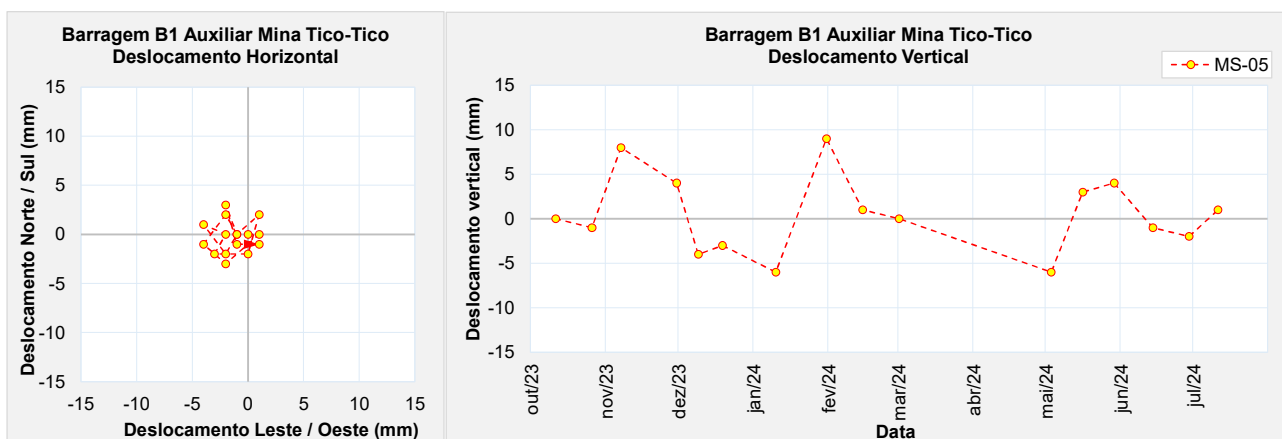
Figura 5.97 – Marco de controle de deformação – MS-05.
