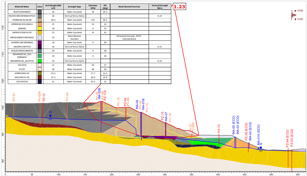
Figura 5.126 – Seção C-C' – Análise Não Drenada – Superfície de ruptura plano-circular otimizada – Freática 30/07/2024 – Razão de resistência não drenada de pico + sismo ↓ (critério CDA).
