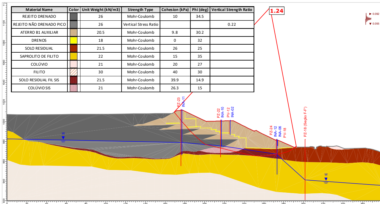
Figura 5.140 – Seção E-E' – Análise Não Drenada – Superfície de ruptura plano-circular otimizada – Freática 30/07/2024 – Razão de resistência não drenada de pico + sismo ↓ (critério CDA).
