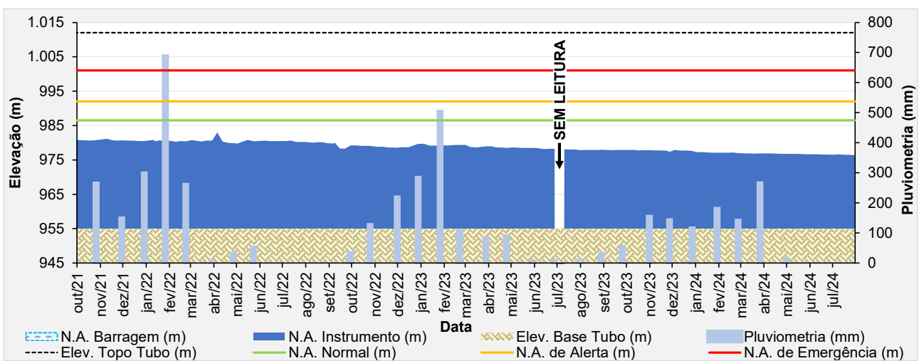
Figura 5.65 – Desempenho do indicador de nível d'água - INA-02B.
