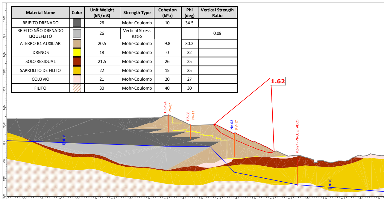
Figura 5.131 – Seção D-D' – Análise Não Drenada – Superfície de ruptura plano-circular otimizada – Freática 30/07/2024 – Razão de resistência não drenada liquefeita.
