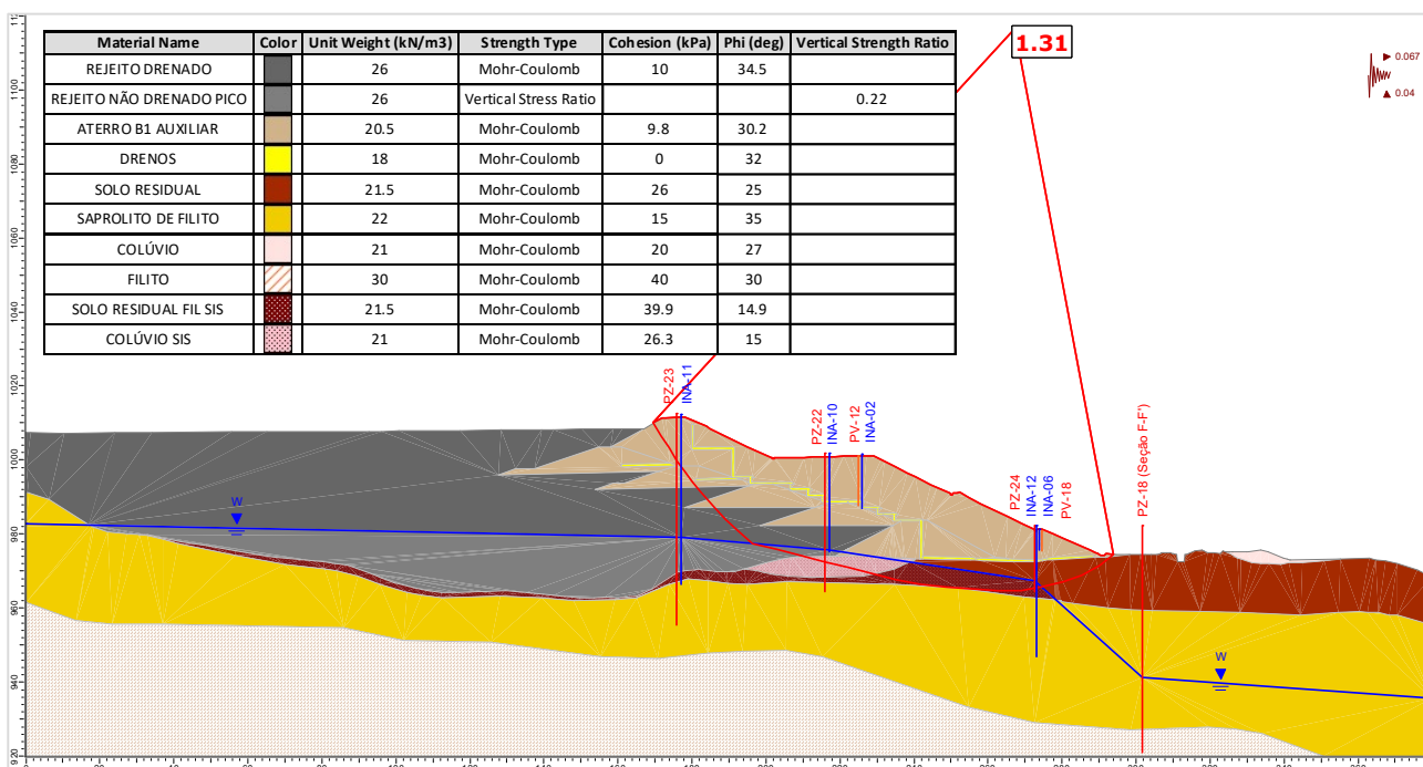
Figura 5.141 – Seção E-E' – Análise Não Drenada – Superfície de ruptura plano-circular otimizada – Freática 30/07/2024 – Razão de resistência não drenada de pico + sismo ↑ (critério vida útil).
