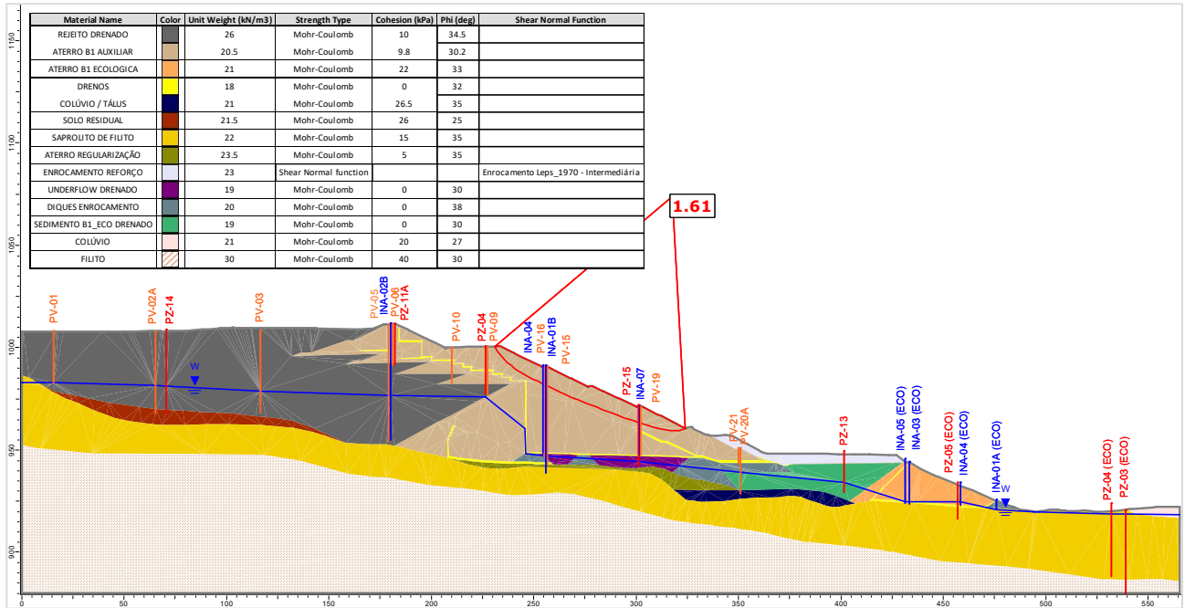
Figura 5.122 – Seção C-C' – Análise Drenada – Superfície de ruptura plano-circular otimizada – Freática 30/07/2024.
