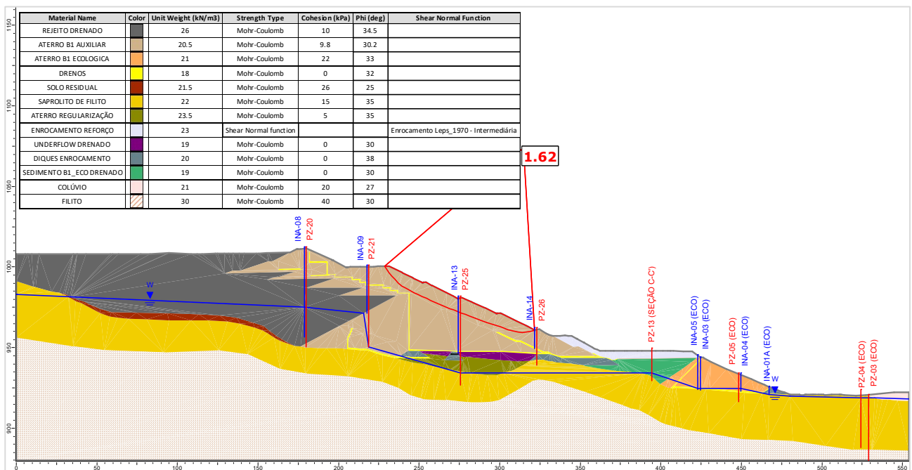
Figura 5.115 – Seção B-B’ – Análise Drenada – Superfície de ruptura plano-circular otimizada – Freática 30/07/2024.
