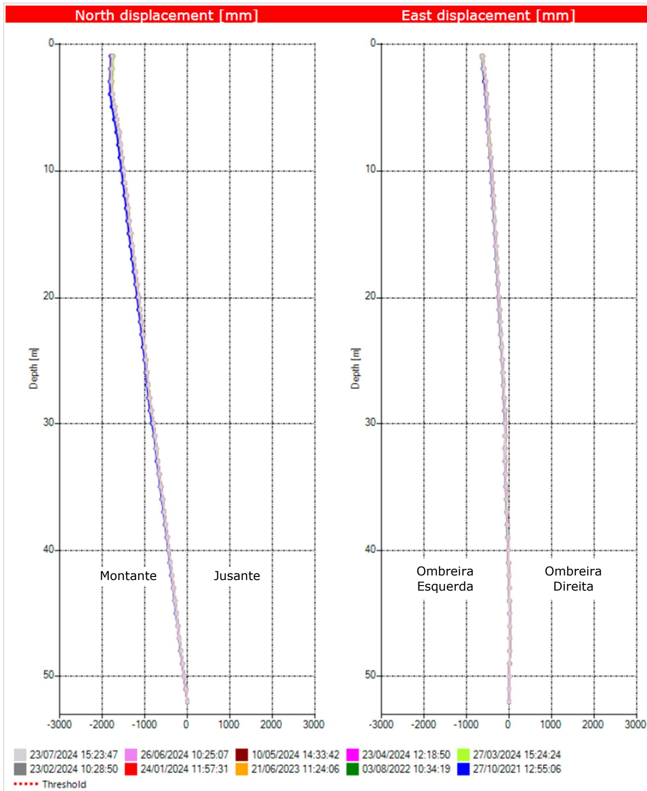
Figura 5.103 – Deslocamentos horizontais acumulados do INC-02 (ref. 23/07/2024).
