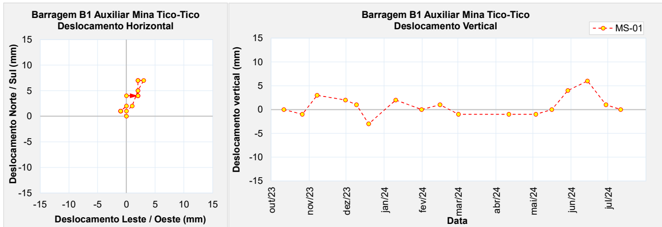
Figura 5.93 – Marco de controle de deformação – MS-01.
