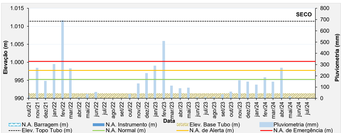
Figura 5.20 – Desempenho do piezômetro elétrico - PV-04.
