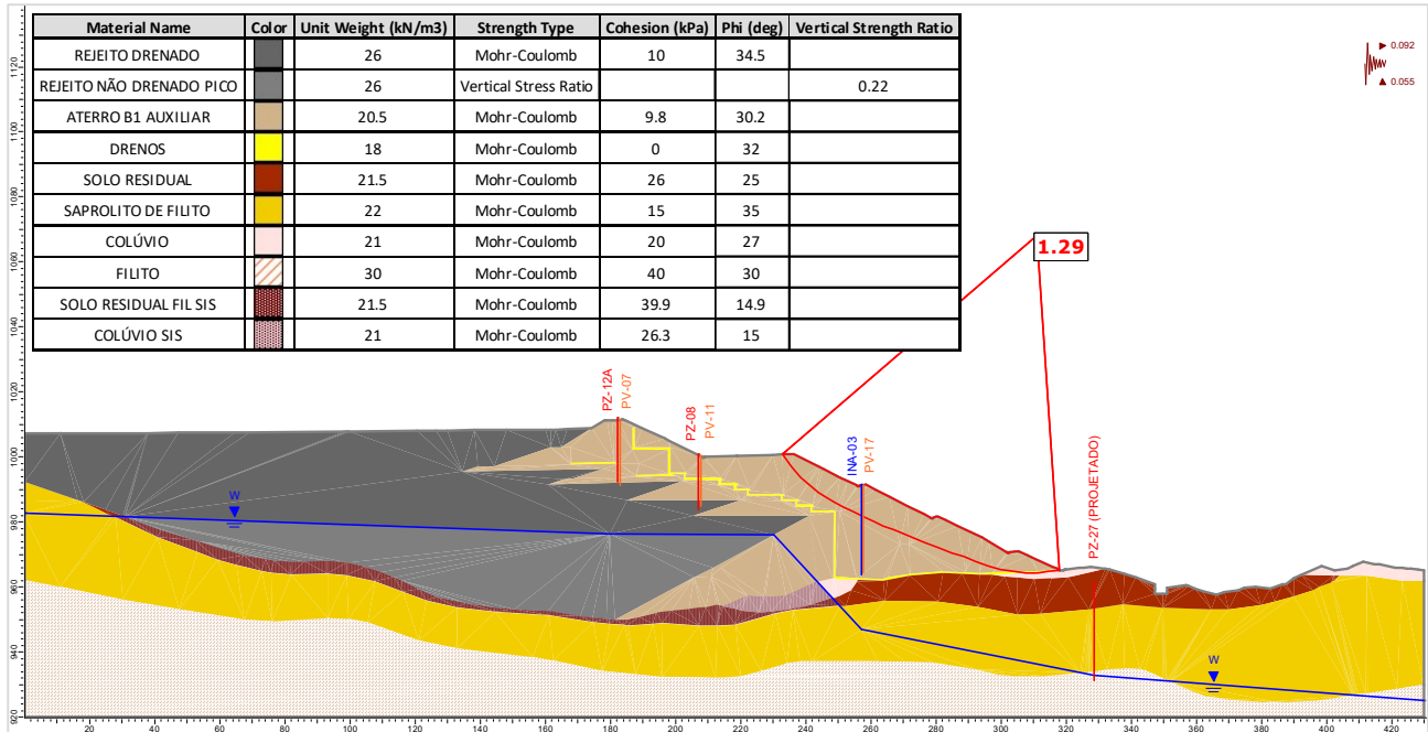
Figura 5.132 – Seção D-D' – Análise Não Drenada – Superfície de ruptura plano-circular otimizada – Freática 30/07/2024 – Razão de resistência não drenada de pico + sismo ↑ (critério CDA).
