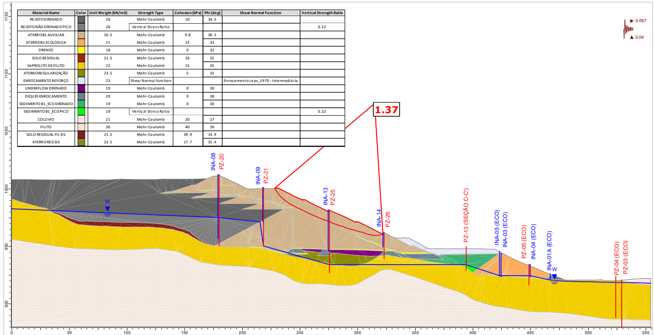
Figura 5.120 – Seção B-B' – Análise Não Drenada – Superfície de ruptura plano-circular otimizada – Freática 30/07/2024 – Razão de resistência não drenada de pico + sismo ↑ (critério vida útil).
