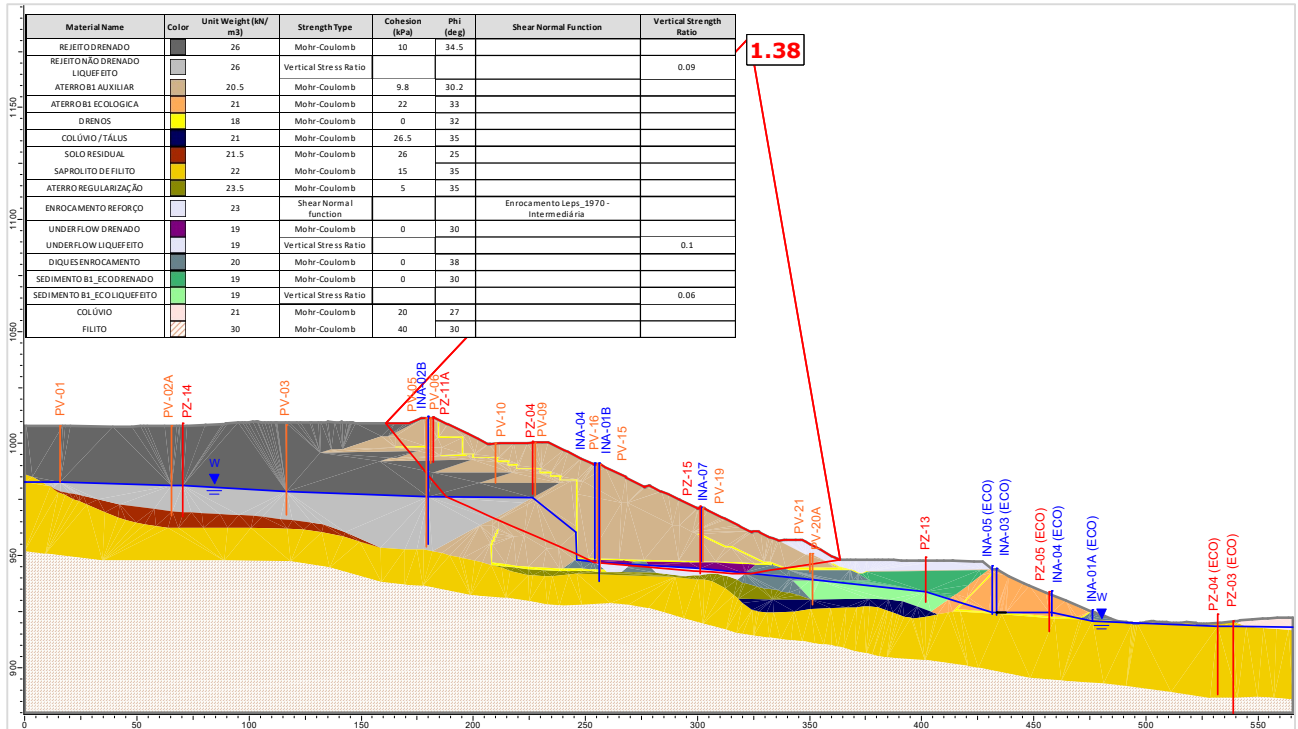
Figura 5.124 – Seção C-C' – Análise Não Drenada – Superfície de ruptura plano-circular otimizada – Freática 30/07/2024 – Razão de resistência não drenada liquefeita.
