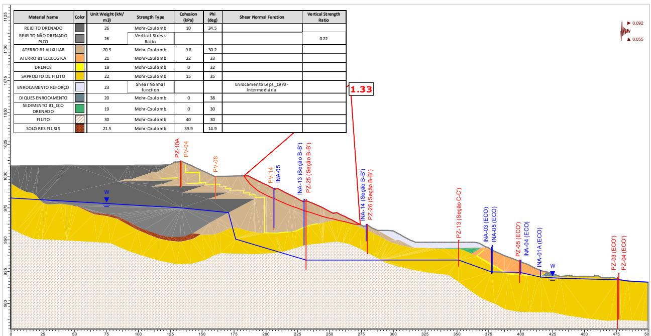
Figura 5.111 – Seção A-A' – Análise Não Drenada – Superfície de ruptura plano-circular otimizada – Freática 30/07/2024 – Razão de resistência não drenada de pico + sismo ↑ (critério CDA).
