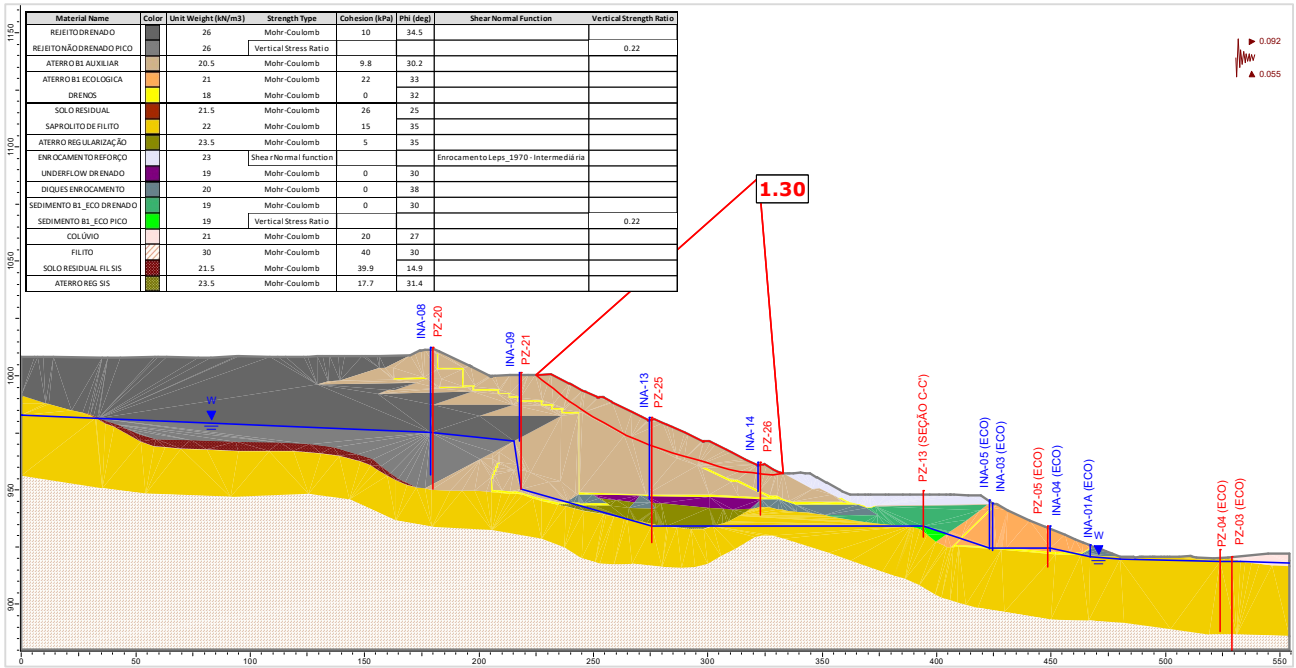
Figura 5.118 – Seção B-B' – Análise Não Drenada – Superfície de ruptura plano-circular otimizada – Freática 30/07/2024 – Razão de resistência não drenada de pico + sismo ↑ (critério CDA).
