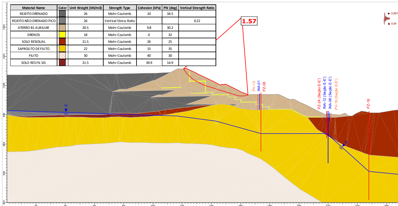
Figura 5.148 – Seção F-F' – Análise Não Drenada – Superfície de ruptura plano-circular otimizada – Freática 30/07/2024 – Razão de resistência não drenada de pico + sismo ↑ (critério vida útil).
