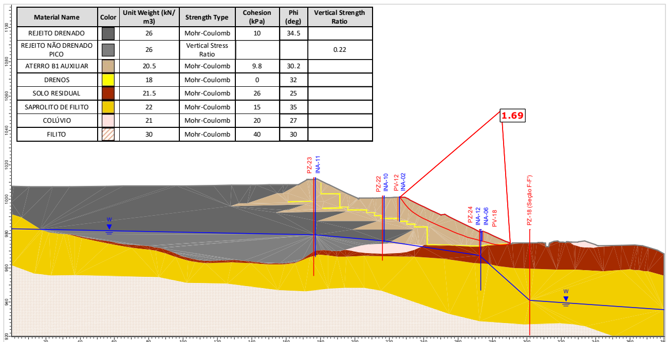
Figura 5.137 – Seção E-E' – Análise Não Drenada – Superfície de ruptura plano-circular otimizada – Freática 30/07/2024 – Razão de resistência não drenada de pico.
