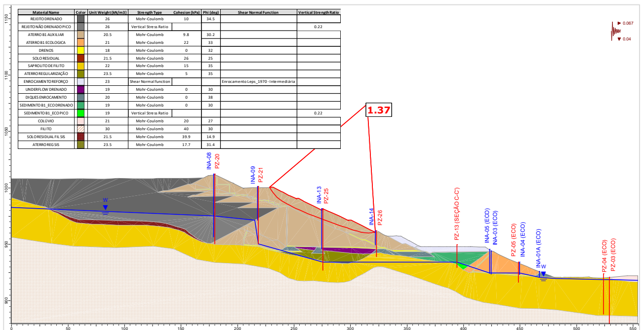
Figura 5.121 – Seção B-B' – Análise Não Drenada – Superfície de ruptura plano-circular otimizada – Freática 30/07/2024 – Razão de resistência não drenada de pico + sismo ↓ (critério vida útil).
