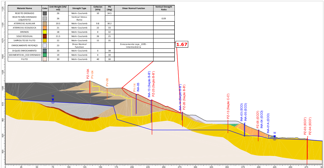
Figura 5.110 – Seção A-A' – Análise Não Drenada – Superfície de ruptura plano-circular otimizada – Freática 30/07/2024 – Razão de resistência não drenada liquefeita.
