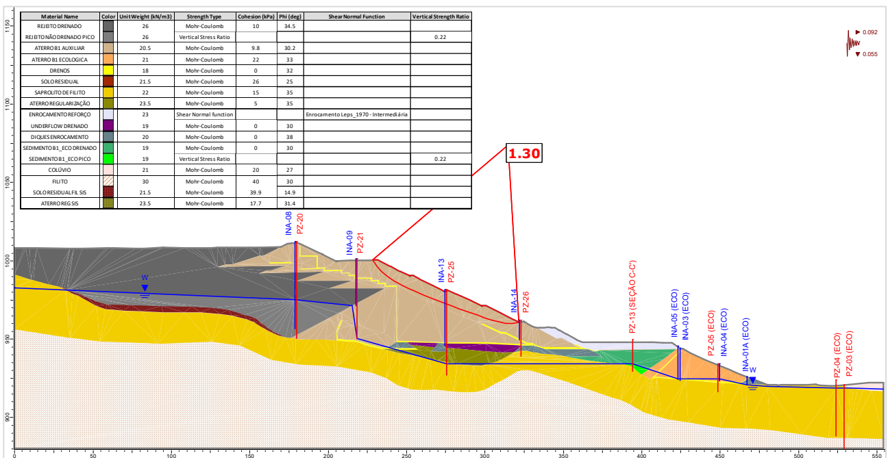
Figura 5.119 – Seção B-B' – Análise Não Drenada – Superfície de ruptura plano-circular otimizada – Freática 30/07/2024 – Razão de resistência não drenada de pico + sismo ↓ (critério CDA).
