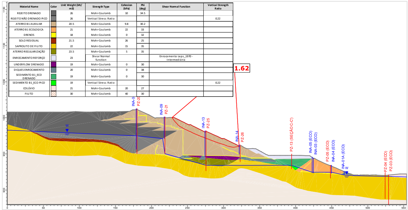
Figura 5.116 – Seção B-B' – Análise Não Drenada – Superfície de ruptura plano-circular otimizada – Freática 30/07/2024 – Razão de resistência não drenada de pico.
