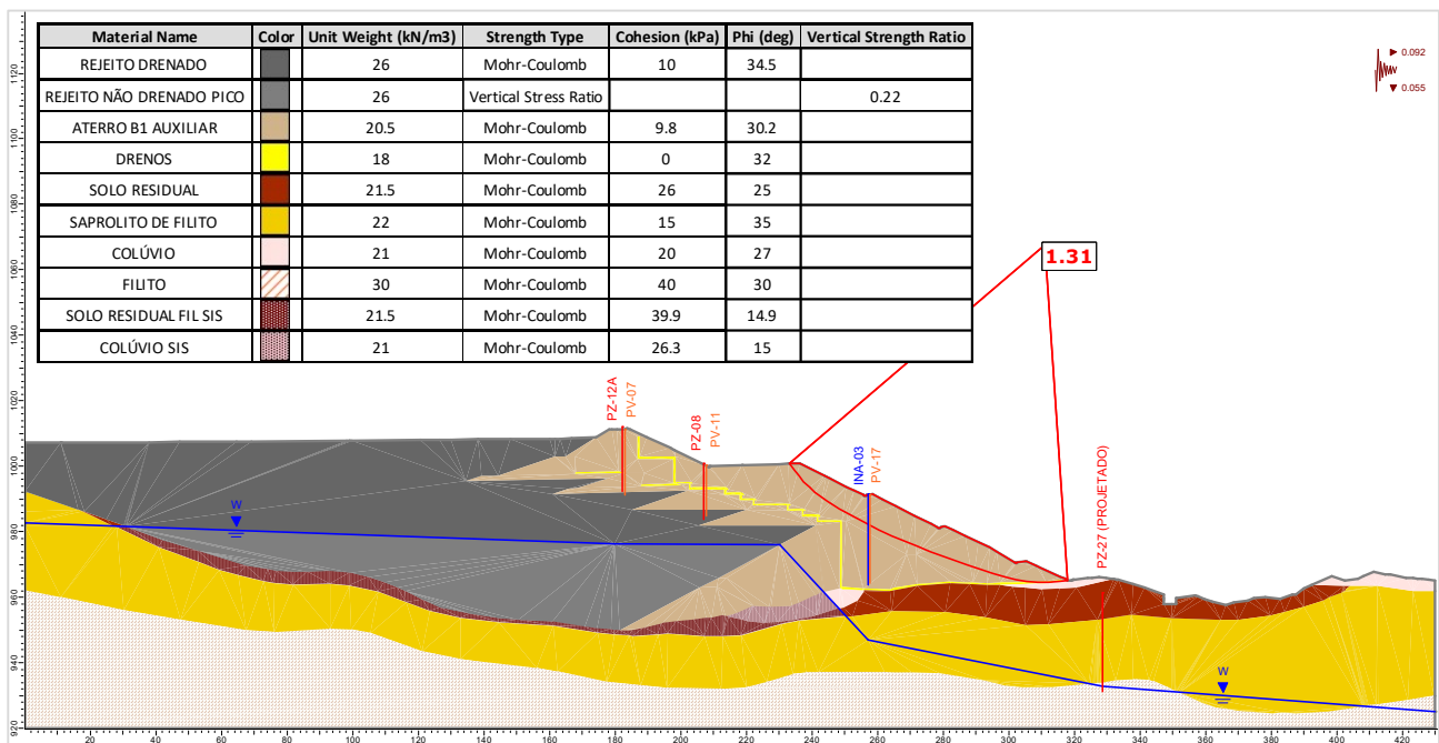
Figura 5.133 – Seção D-D' – Análise Não Drenada – Superfície de ruptura plano-circular otimizada – Freática 30/07/2024 – Razão de resistência não drenada de pico + sismo ↓ (critério CDA).
