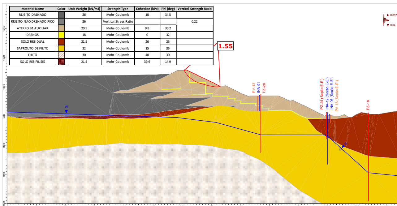
Figura 5.149 – Seção F-F' – Análise Não Drenada – Superfície de ruptura plano-circular otimizada – Freática 30/07/2024 – Razão de resistência não drenada de pico + sismo ↓ (critério vida útil).
