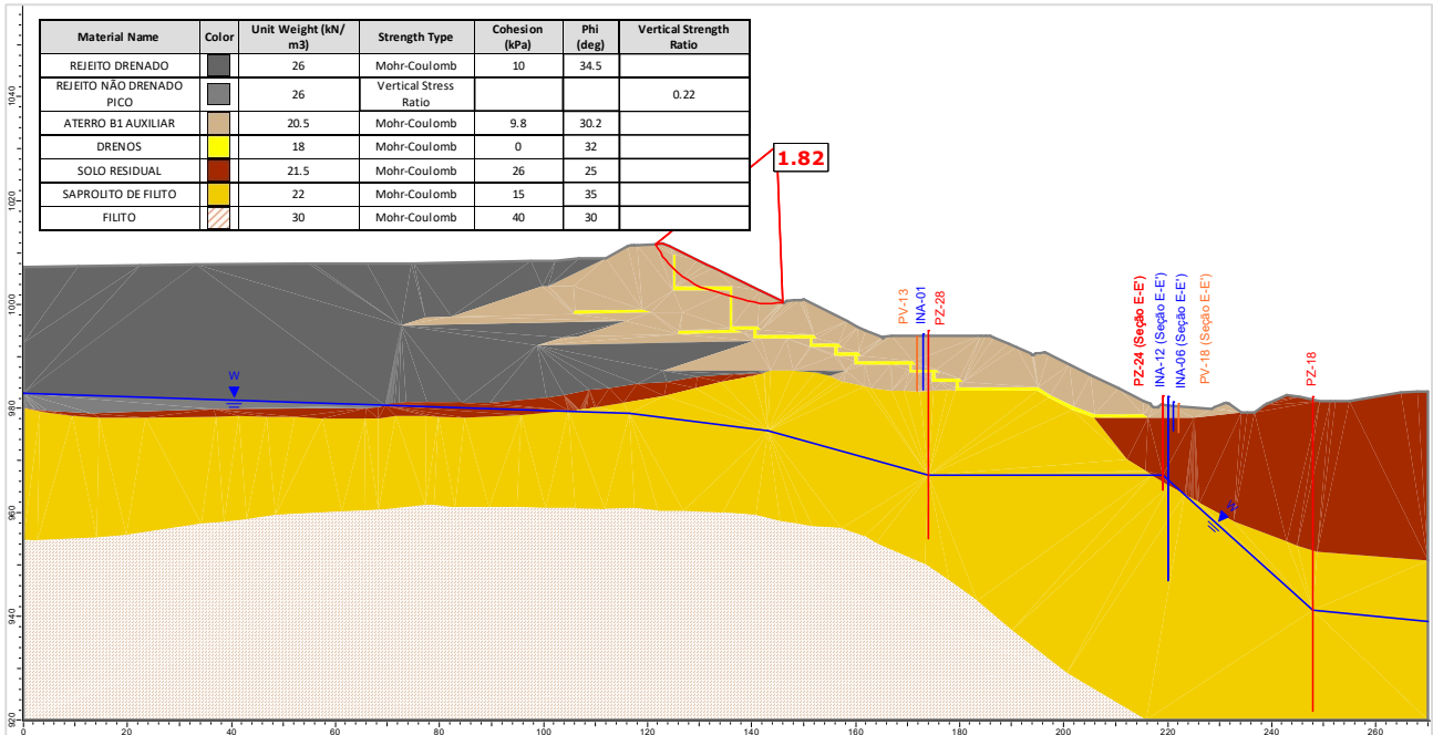
Figura 5.144 – Seção F-F' – Análise Não Drenada – Superfície de ruptura plano-circular otimizada – Freática 30/07/2024 – Razão de resistência não drenada de pico.
