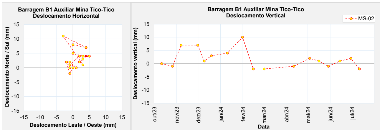
Figura 5.94 – Marco de controle de deformação – MS-02.
