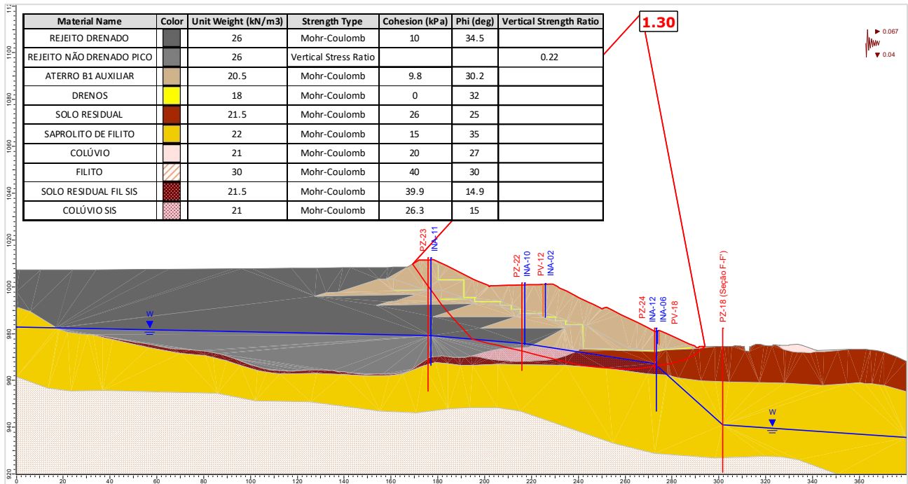
Figura 5.142 – Seção E-E' – Análise Não Drenada – Superfície de ruptura plano-circular otimizada – Freática 30/07/2024 – Razão de resistência não drenada de pico + sismo ↓ (critério vida útil).
