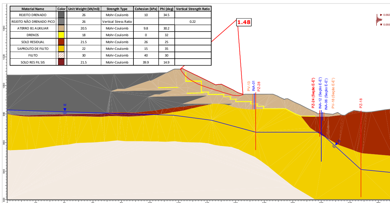
Figura 5.147 – Seção F-F' – Análise Não Drenada – Superfície de ruptura plano-circular otimizada – Freática 30/07/2024 – Razão de resistência não drenada de pico + sismo ↓ (critério CDA).
