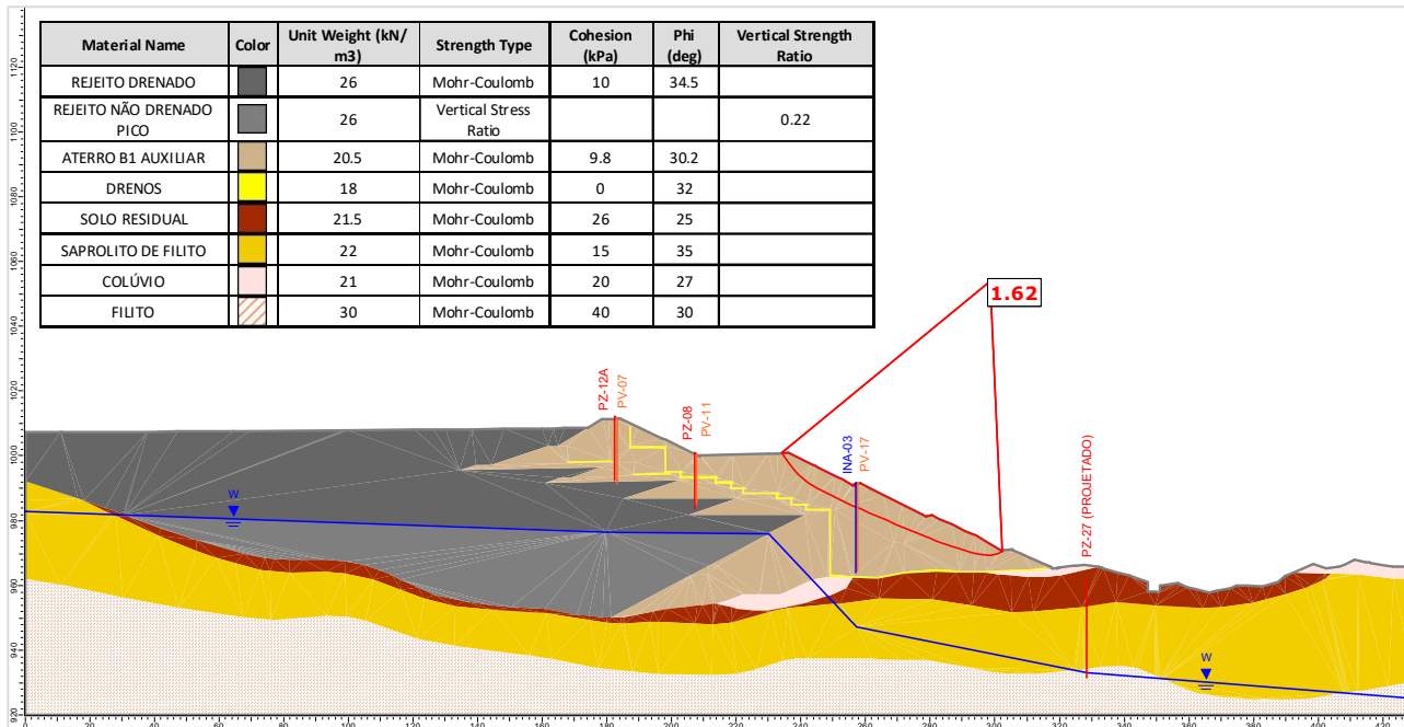
Figura 5.130 – Seção D-D' – Análise Não Drenada – Superfície de ruptura plano-circular otimizada – Freática 30/07/2024 – Razão de resistência não drenada de pico.
