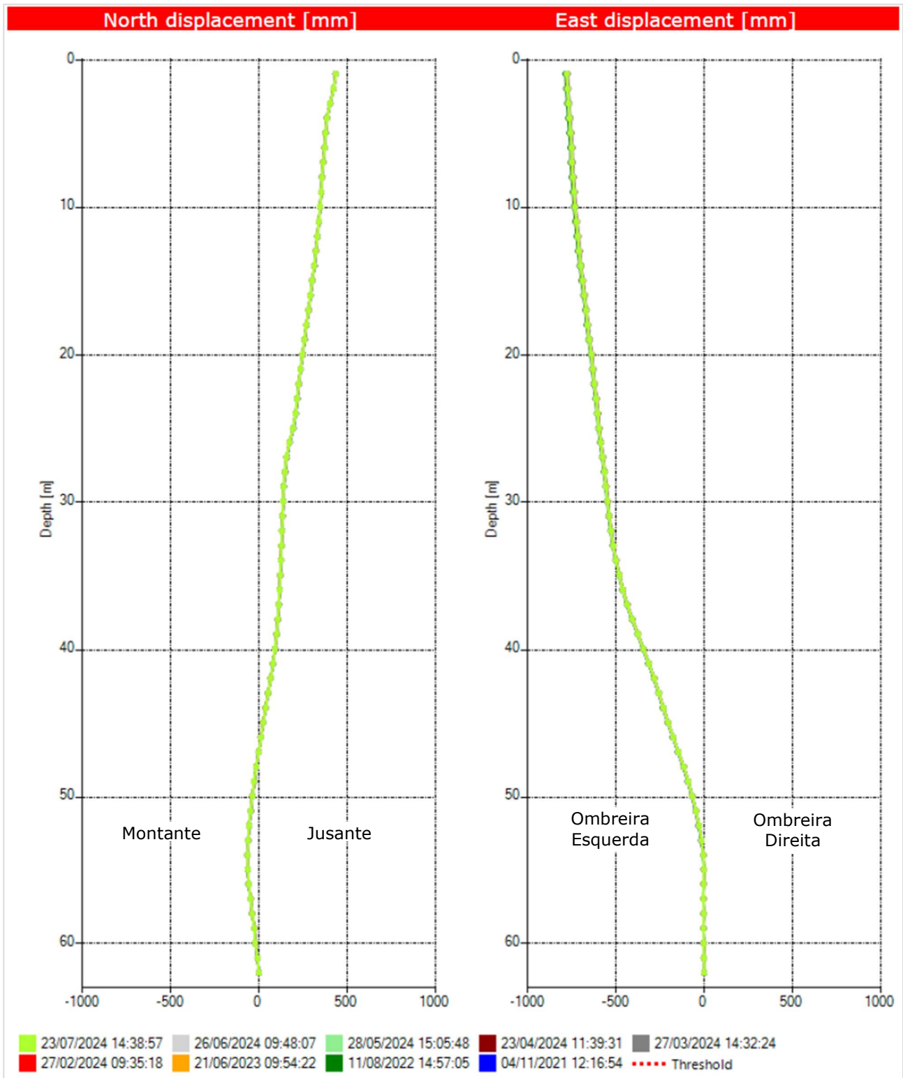
Figura 5.101 – Deslocamentos horizontais acumulados do INC-01 (ref. 23/07/2024).
