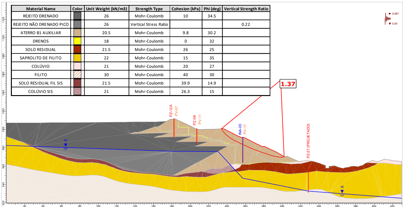
Figura 5.135 – Seção D-D' – Análise Não Drenada – Superfície de ruptura plano-circular otimizada – Freática 30/07/2024 – Razão de resistência não drenada de pico + sismo ↓ (critério vida útil).
