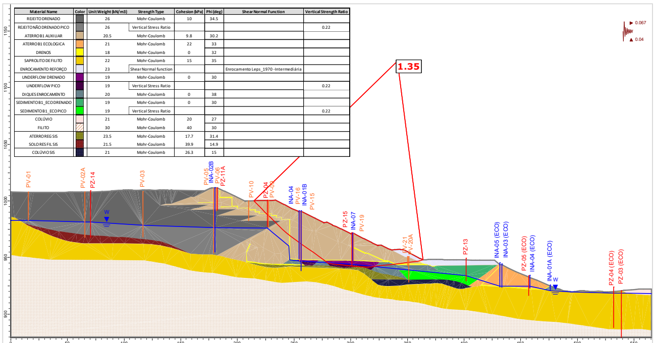
Figura 5.127 – Seção C-C' – Análise Não Drenada – Superfície de ruptura plano-circular otimizada – Freática 30/07/2024 – Razão de resistência não drenada de pico + sismo ↑ (critério vida útil).
