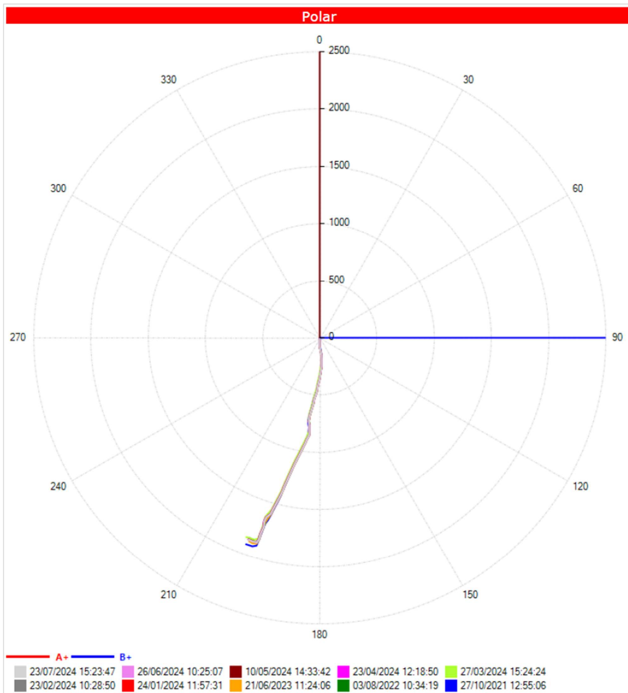
Figura 5.104 – Deslocamentos em relação a coordenadas polares acumulados do INC-02 (ref. 23/07/2024).
