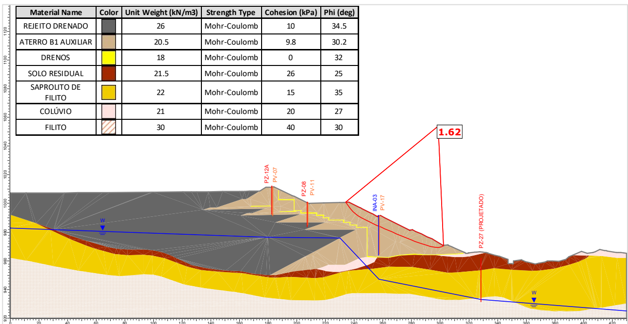
Figura 5.129 – Seção D-D' – Análise Drenada – Superfície de ruptura plano-circular otimizada – Freática 30/07/2024.
