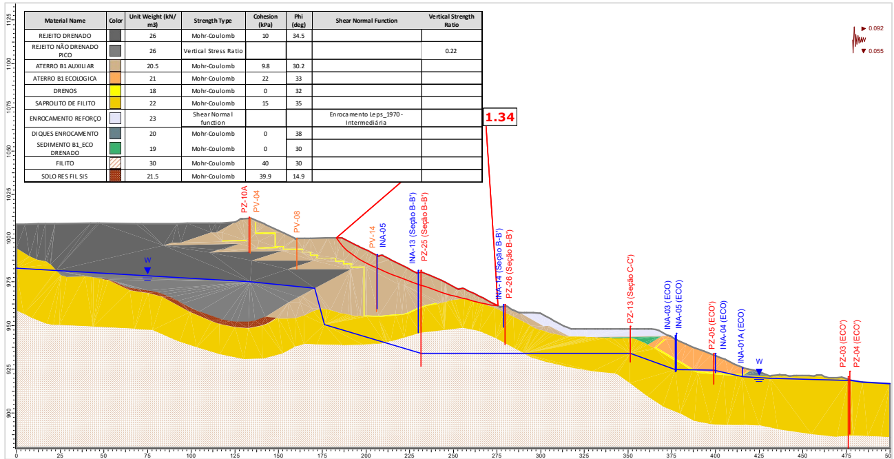
Figura 5.112 – Seção A-A' – Análise Não Drenada – Superfície de ruptura plano-circular otimizada – Freática 30/07/2024 – Razão de resistência não drenada de pico + sismo ↓ (critério CDA).
