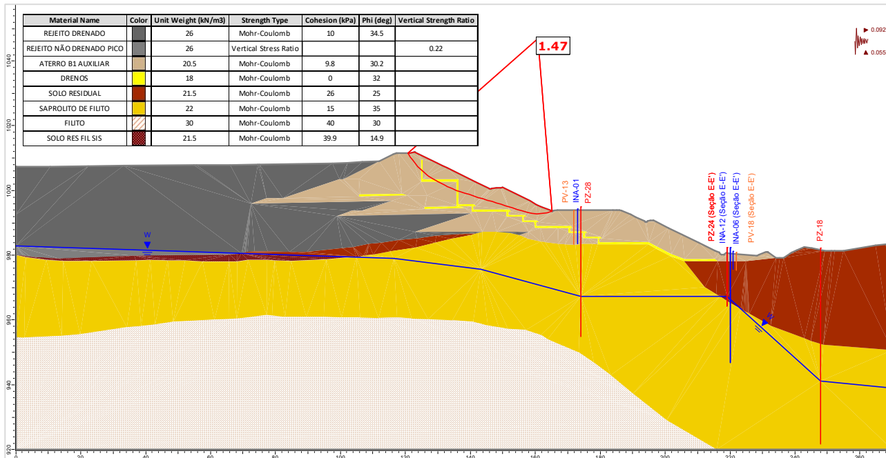
Figura 5.146 – Seção F-F' – Análise Não Drenada – Superfície de ruptura plano-circular otimizada – Freática 30/07/2024 – Razão de resistência não drenada de pico + sismo ↑ (critério CDA).
