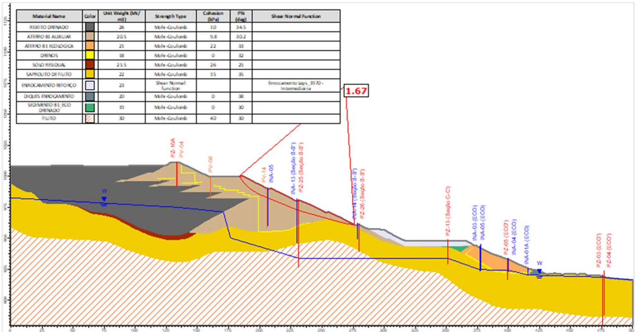
Figura 5.108 – Seção A-A' – Análise Drenada – Superfície de ruptura plano-circular otimizada – Freática 30/07/2024.
